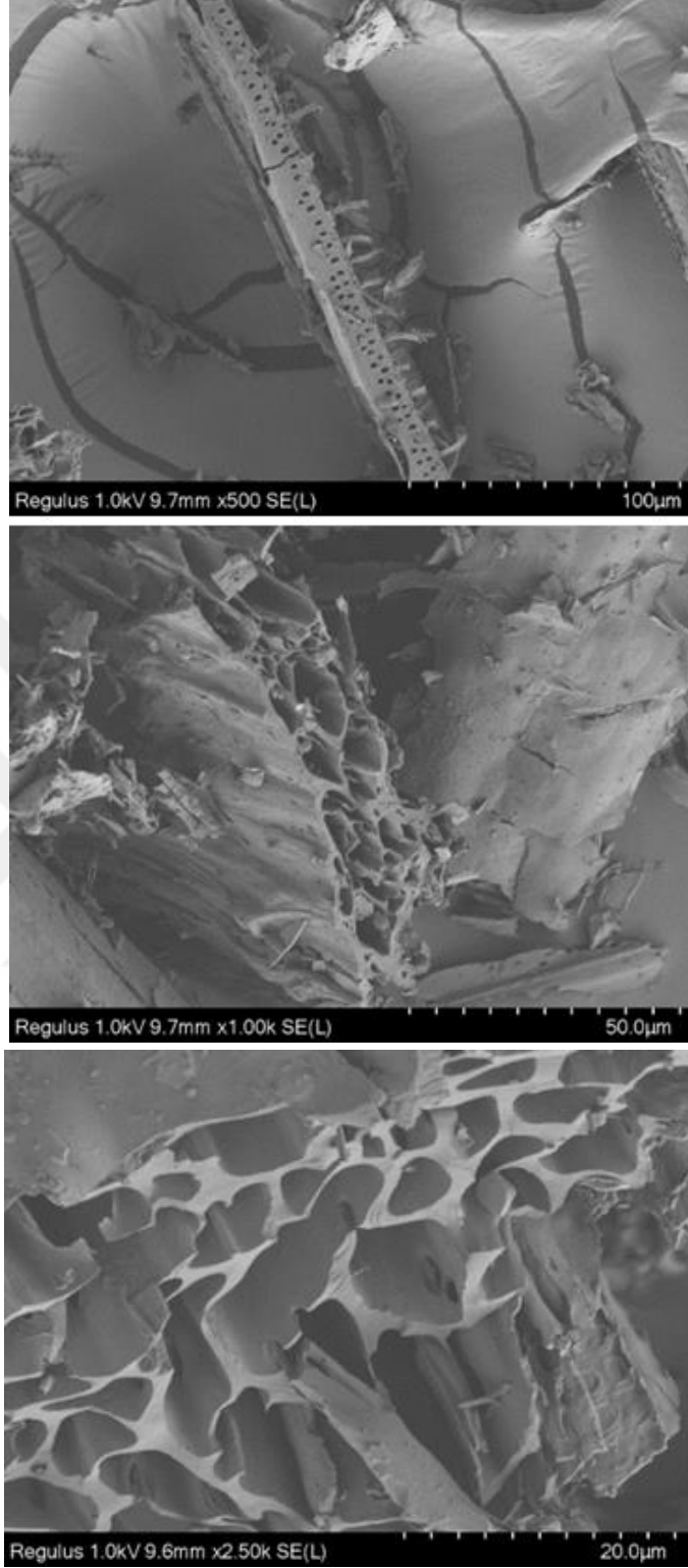
Şekil 7.54. Biyokütlenin 700°C sıcaklık ve 5 dk alıkonma süresiyle gerçekleştirilen hızlı pirolizinden elde edilen charın sırasıyla 500,1000 ve 2500 kez büyütülmüş SEM görüntüsü
