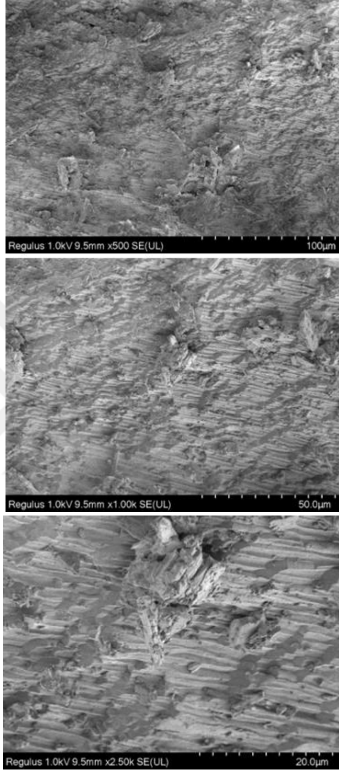
Şekil 7.3. Mussel Shell 'in sırasıyla 500,1000 ve 2500 kez büyütülmüş SEM görüntüsü
