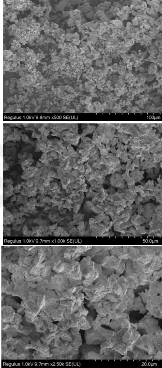
Şekil 7.7. 1000°C sıcaklıkta kalsine edilmiş Mussel Shell'in sırasıyla 500,1000 ve 2500 kez büyütülmüş SEM görüntüsü
