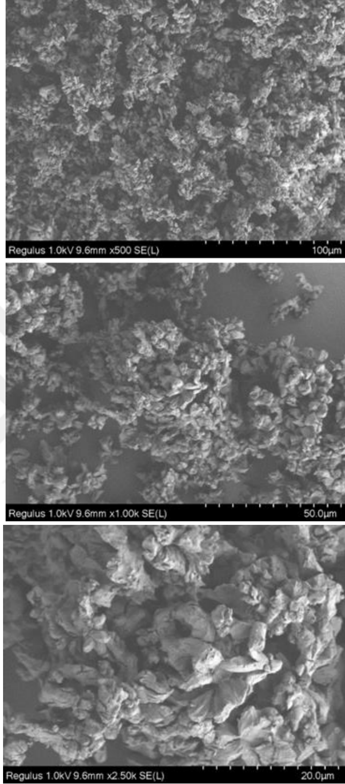
Şekil 7.8. 1000°C sıcaklıkta kalsine edilmiş Argopecten Gibbus Curved 'in sırasıyla 500,1000 ve 2500 kez büyütülmüş SEM görüntüsü
