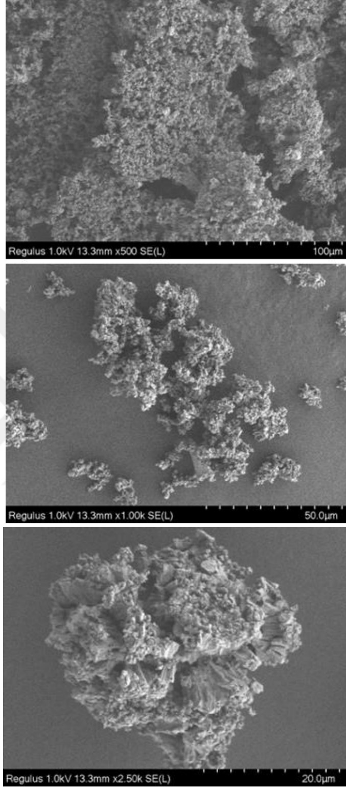
Şekil 7.9. Ticari CaO'ın sırasıyla 500,1000 ve 2500 kez büyütülmüş SEM görüntüsü
