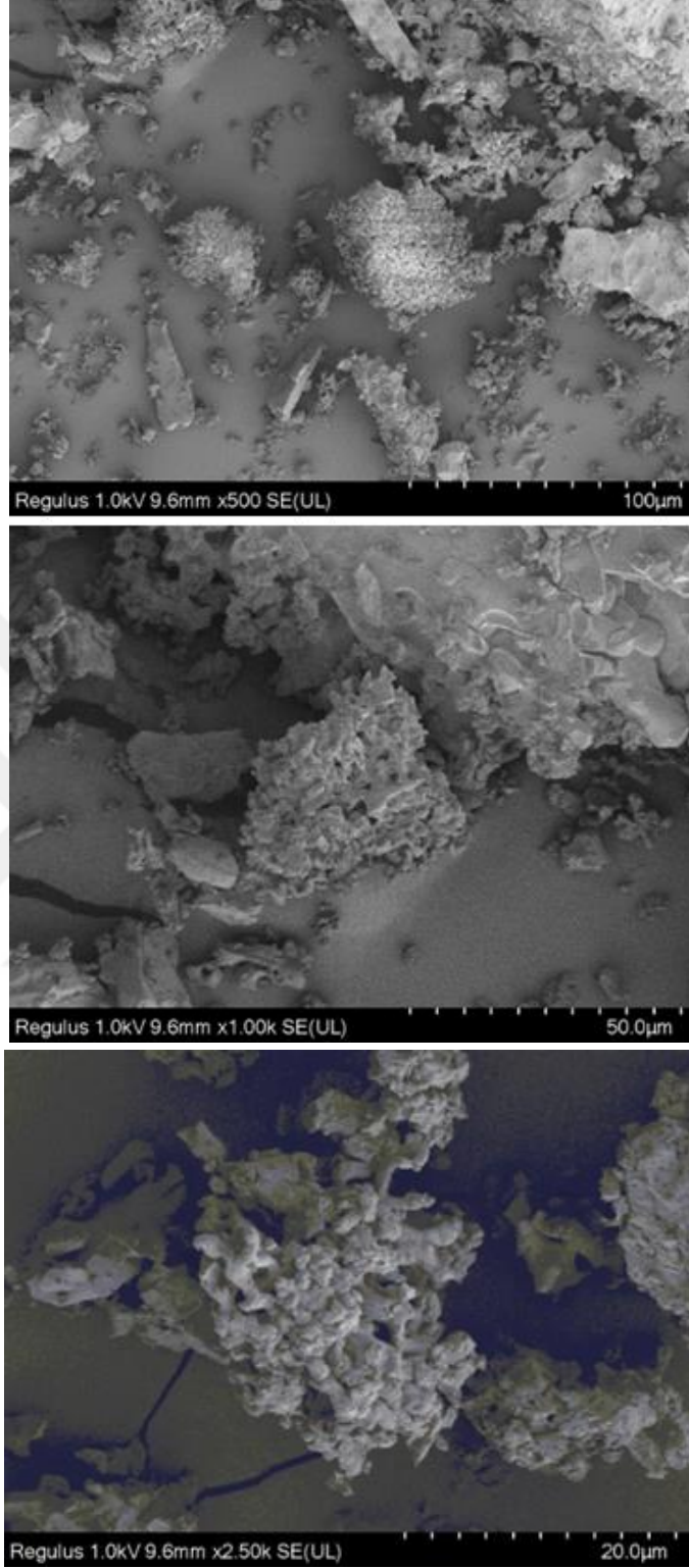
Şekil 7.5. 750°C sıcaklıkta kalsine edilmiş Mussel Shell'in sırasıyla 500,1000 ve 2500 kez büyütülmüş SEM görüntüsü
