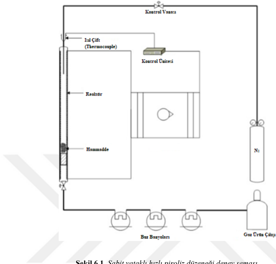
Şekil 6.1. Sabit yataklı hızlı piroliz düzeneği deney şeması
