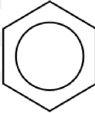
Şekil 7.39. Benzen bileşiği
