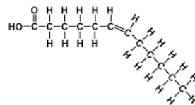
Şekil 7.41. Yağ asitleri
