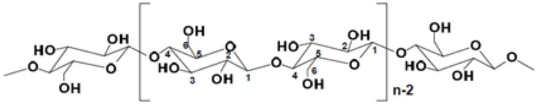
Şekil 2.4: Selülozun moleküler yapısı (Wei vd., 2015)
