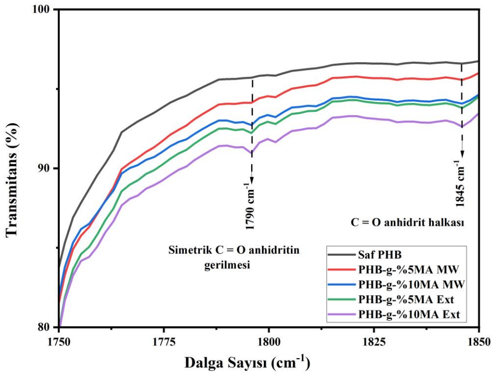
Şekil 4.16: PHB ve PHB-g-MA ilaveli karışımlarının FTIR grafiği maleik anhidrit grupları
