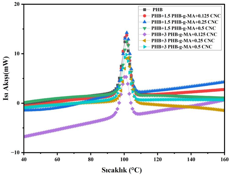
Şekil 4.47: Saf PHB ve PHB+P-g-MA+CNC kompozitlerinin DSC 2. soğutma eğrisi
