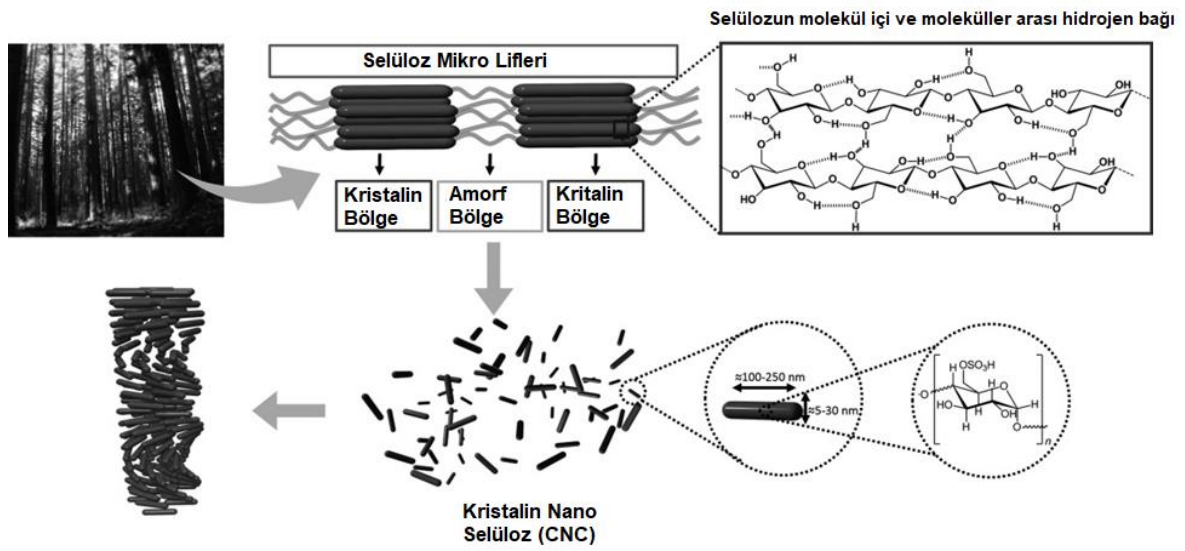
Şekil 2.5: Kristalin Nano selüloz üretim süreci (Giese vd., 2015)
