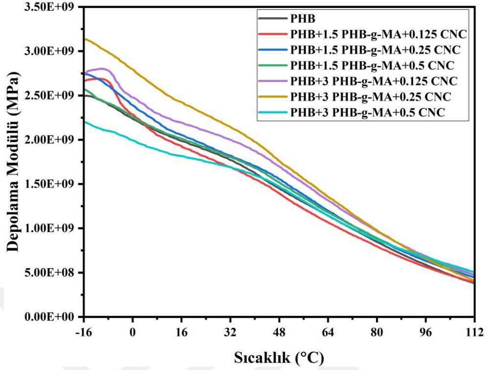
Şekil 4.67: Hızlandırılmış yaşlandırma testi sonrası PHB ve PHB+PHB-g-MA+CNC kompozitlerinin depolama modülü grafiği
