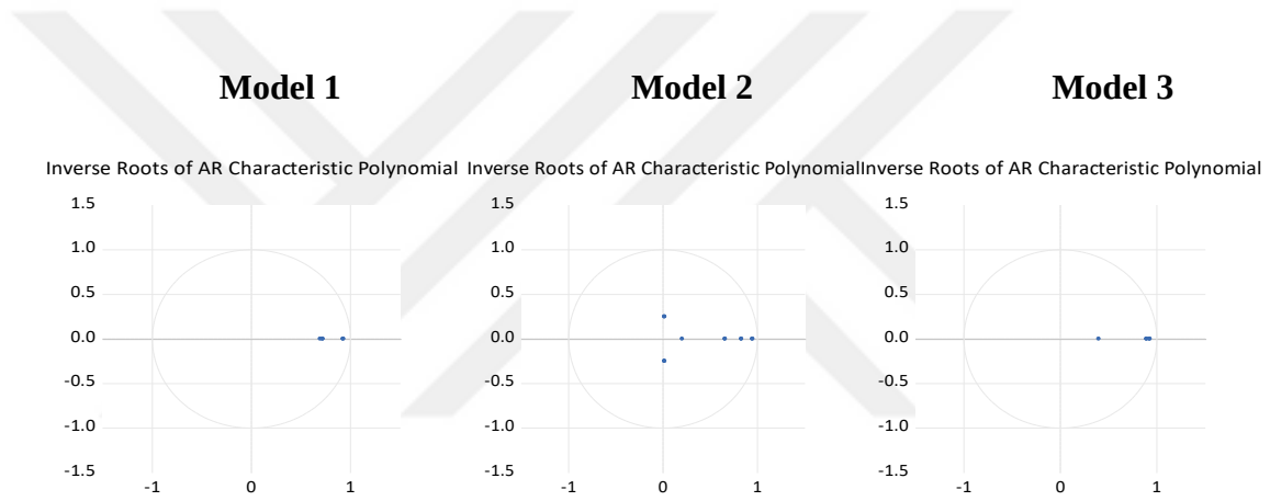
Şekil 1.7. AR Karakteristik Polinomun Ters Kökleri
