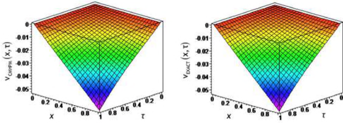
Şekil 5.2 Genelleştirilmiş Black-Scholes Denkleminin Çözümleri ve Kesirli Black-Scholes Denkleminin Homotopi Pertürbasyon Metodu ile Çözümlerinin Karşılaştırılması (Özdemir ve Yavuz [104])
