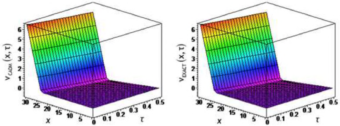
Şekil 5.1 Black-Scholes Denkleminin Çözümleri ve Kesirli Black-Scholes Denkleminin Adomian Ayırıştırma Metodu ile Çözümlerinin Karşılaştırılması (Özdemir ve Yavuz [104])
