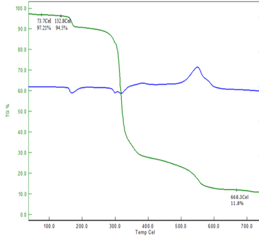
Şekil 201. I no'lu kompleks için TG-DTA
