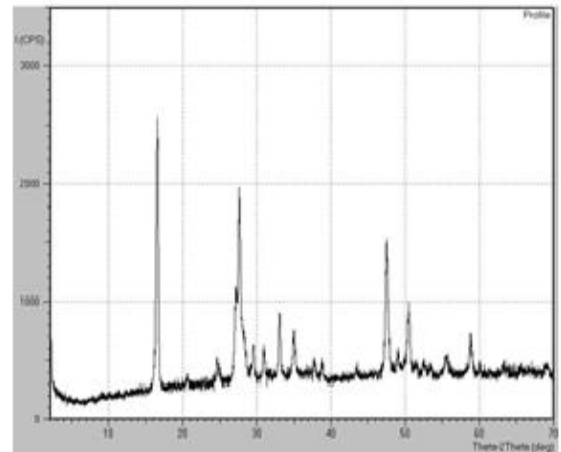
Şekil 96. XVI no'lu kompleks için XRD
