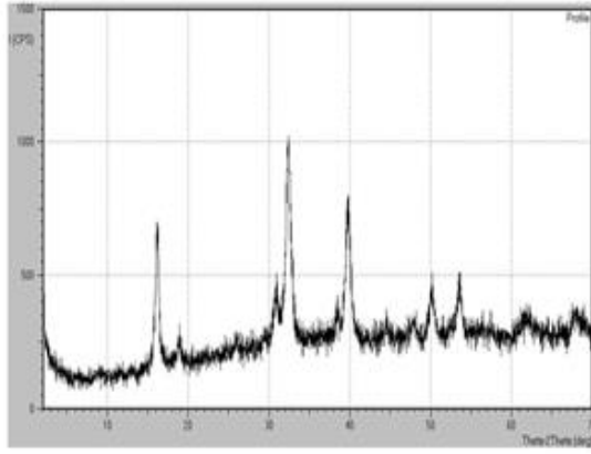
Şekil 87. VII no'lu kompleks için XRD
