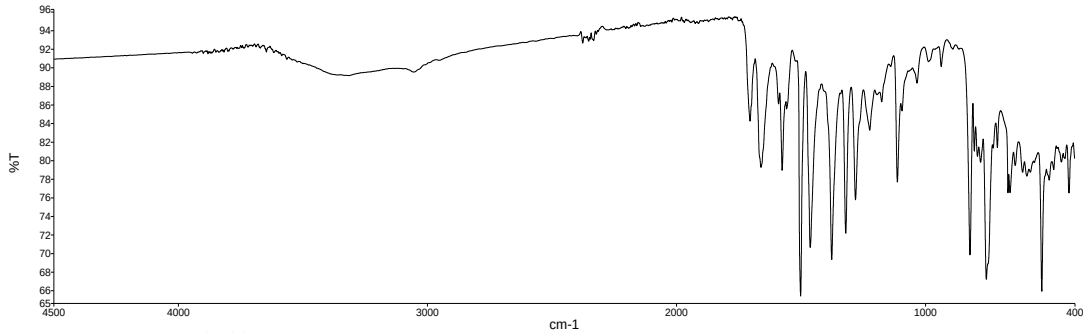
Şekil 44. IV no'lu kompleks için FTIR spektrumu.
