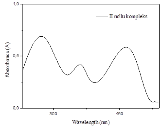
Şekil 2. II no'lu kompleks için UV.
