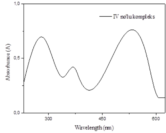
Şekil 4. IV no'lu kompleks için UV.
