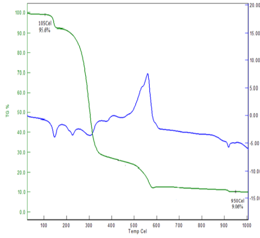
Şekil 205. V no'lu kompleks için TG-DTA
