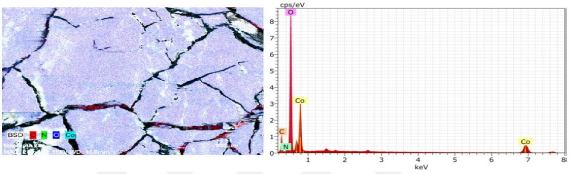
Şekil 125. V no'lu kompleks için EDX.
