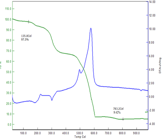
Şekil 218. XVIII no'lu komp. için TG-DTA
