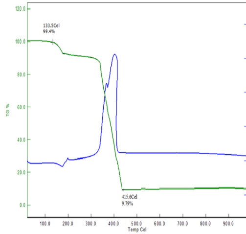
Şekil 209. X no'lu kompleks için TG-DTA
