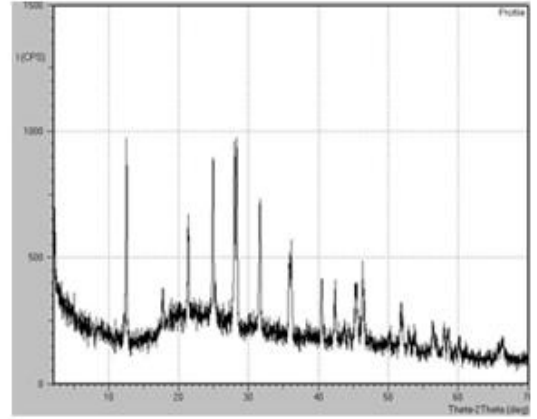
Şekil 82. II no'lu kompleks için XRD
