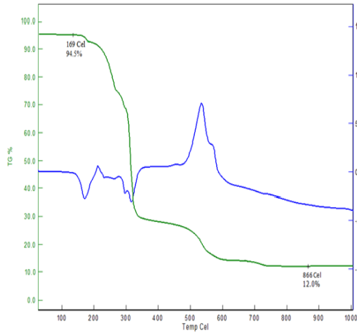
Şekil 235. XXXV no'lu komp. için TG-DTA
