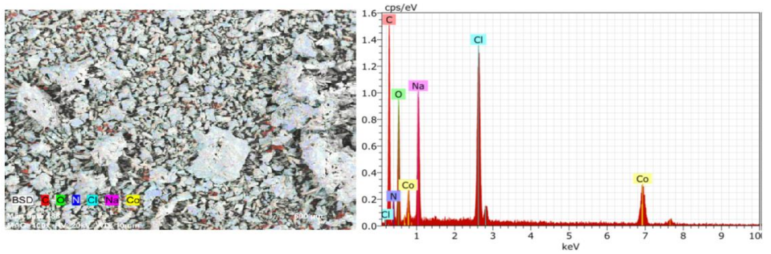
Şekil 141. XXI no'lu kompleks için EDX.
