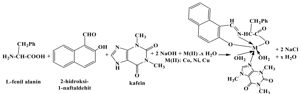
Şekil 4.22. Kafeinin imin 5 varlığında Kobalt(II), Nikel(II) ve Bakır(II) kompleks bileşiklerinin eldesi.
