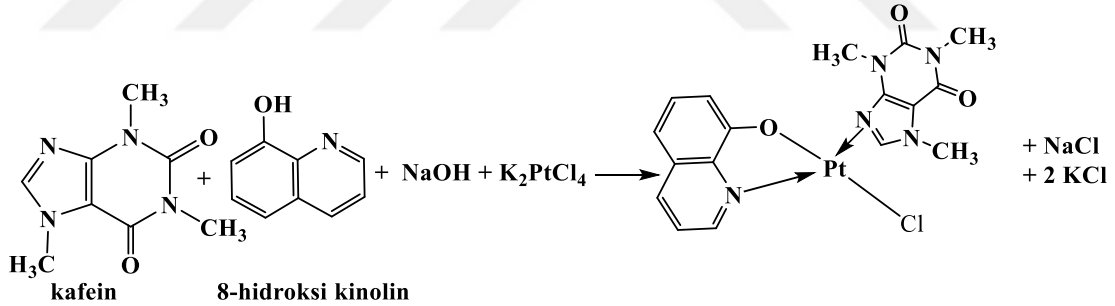
Şekil 4.3. Kafeinin 8-hidroksikinolin varlığında Platin(II) kompleks bileşiğinin eldesi.
