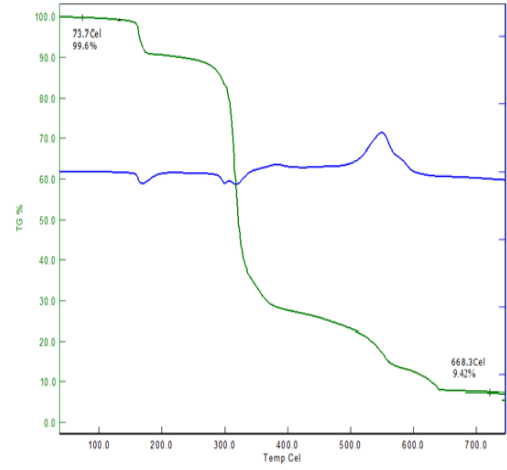
Şekil 217. XVII no'lu komp. için TG-DTA
