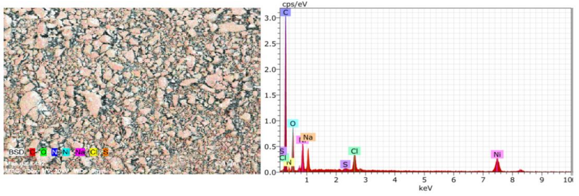
Şekil 145. XXV no'lu kompleks için EDX.
