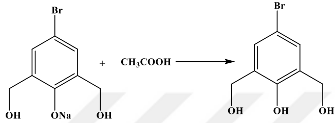
Şekil 4.13. BBHMP (L 1 ) eldesi.
