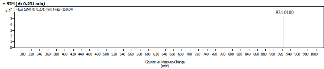
Şekil 5.13. XIII no'lu kompleks bileşiğin LC-MS spektrum grafiği.
