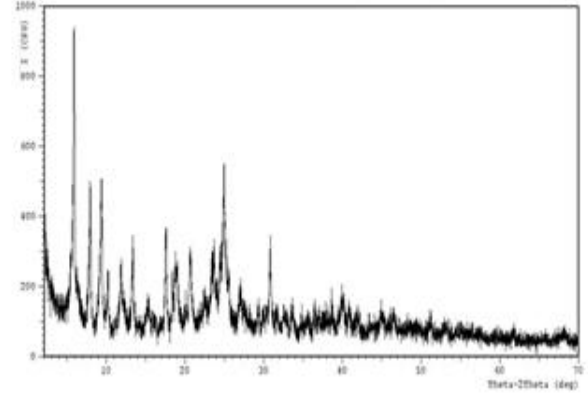
Şekil 114. XXXIV no'lu komp. için XRD
