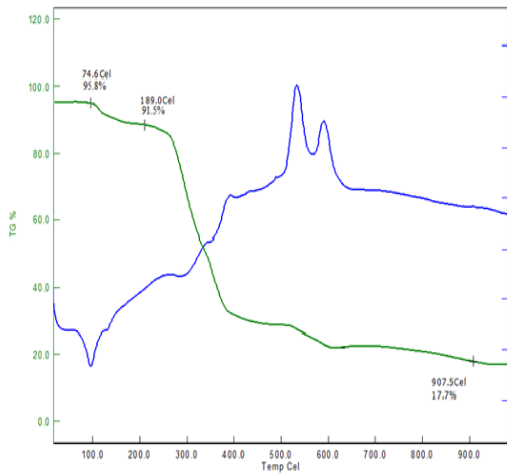
Şekil 221. XXI no'lu komp. için TG-DTA
