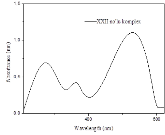
Şekil 22. XXII no'lu kompleks için UV.
