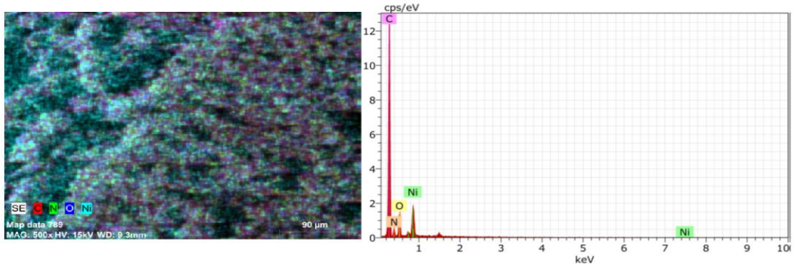
Şekil 122. II no'lu kompleks için EDX.
