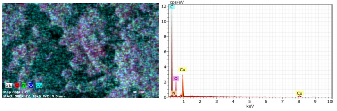
Şekil 157. XXXVII no'lu kompleks için EDX.
