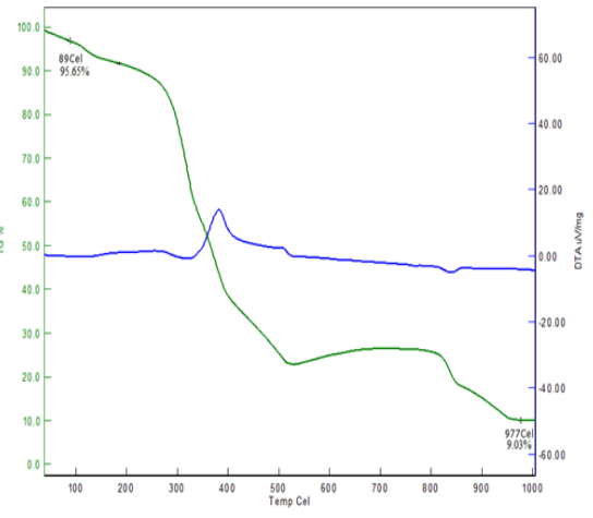
Şekil 206. VI no'lu komp. için TG-DTA
