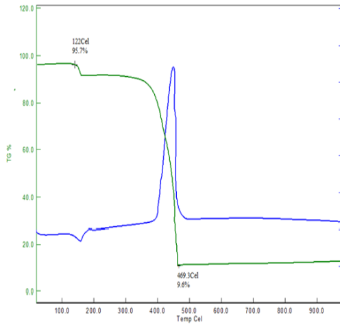
Şekil 205. V no'lu kompleks için TG-DTA
