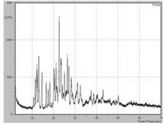
Şekil 106. XXVI no'lu kompleks için XRD
