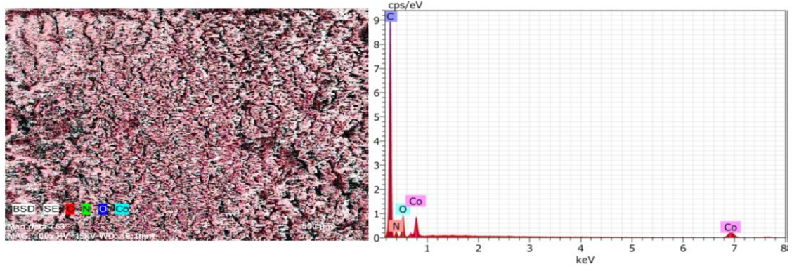
Şekil 121. I no'lu kompleks için EDX.
