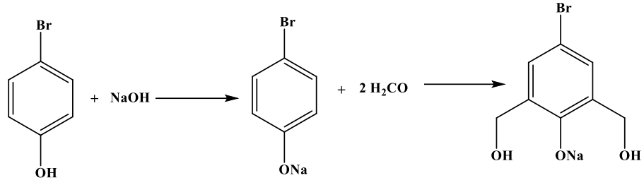
Şekil 4.12. Sodyum p-brom-2,6-bis(hidroksimetil)fenolün eldesi.
