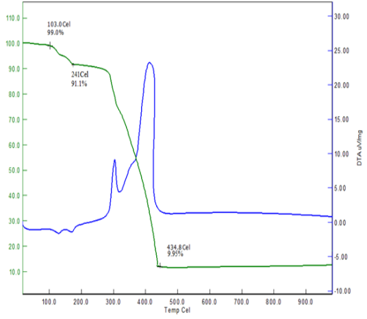
Şekil 218. XVIII no'lu komp. için TG-DTA
