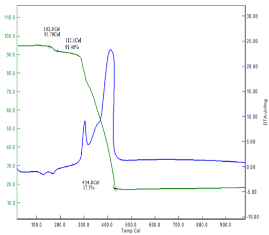
Şekil 222. XXII no'lu komp. için TG-DTA
