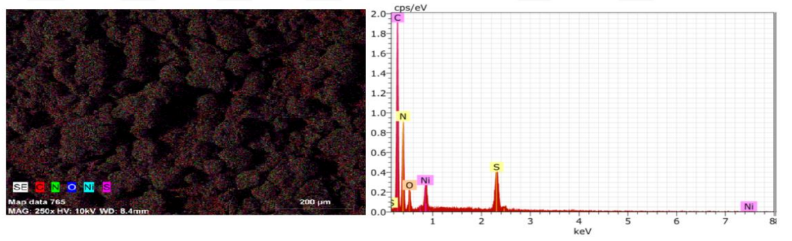
Şekil 134. XIV no'lu kompleks için EDX.
