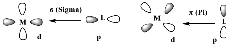
Şekil 2.3. \pi verici ligandlar L \rightarrow M ( \sigma bağı), L \rightarrow M ( \pi bağı).
