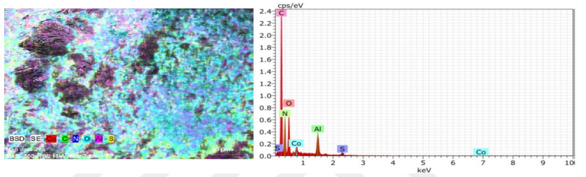
Şekil 133. XIII no'lu kompleks için EDX.
