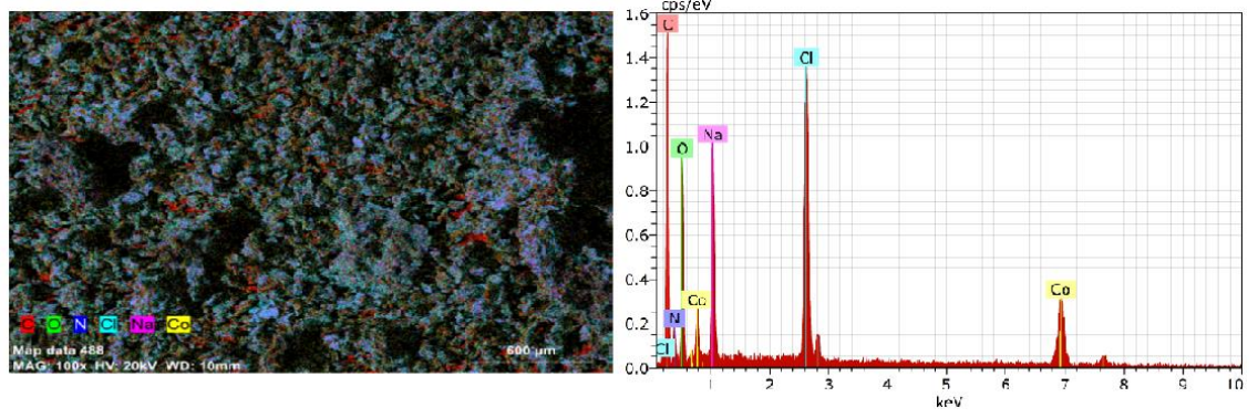
Şekil 148. XXVIII no'lu kompleks için EDX.
