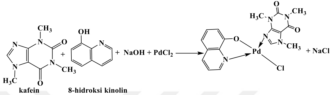
Şekil 4.2. Kafeinin 8-hidroksikinolin varlığında Palladyum(II) kompleks bileşiğinin eldesi.
