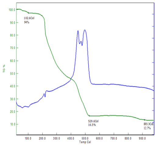
Şekil 237. XXXVII no'lu komp. TG-DTA
