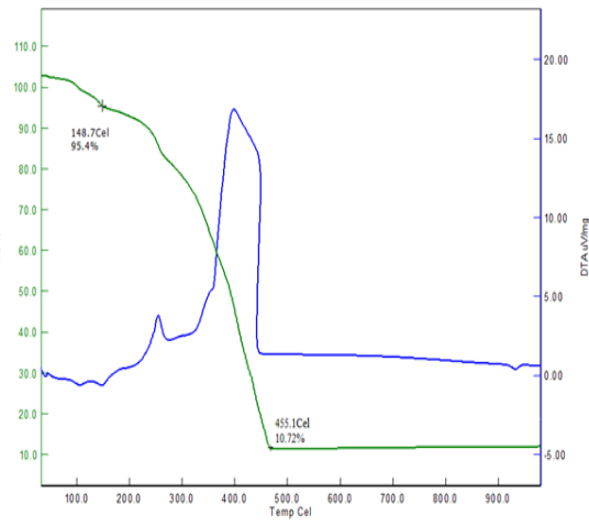
Şekil 210. XI no'lu komp. için TG-DTA
