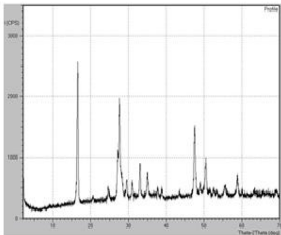
Şekil 101. XXI no'lu kompleks için XRD
