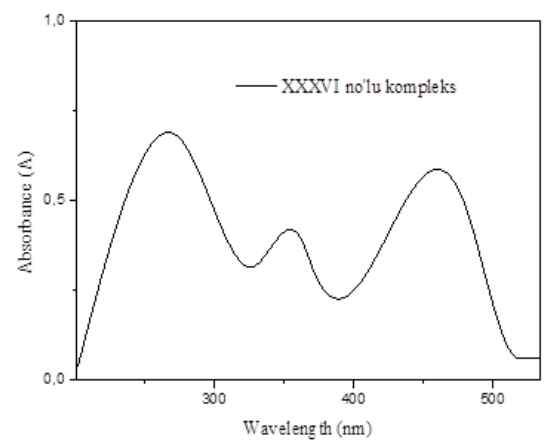
Şekil 36. XXXVI no'lu kompleks için UV.
