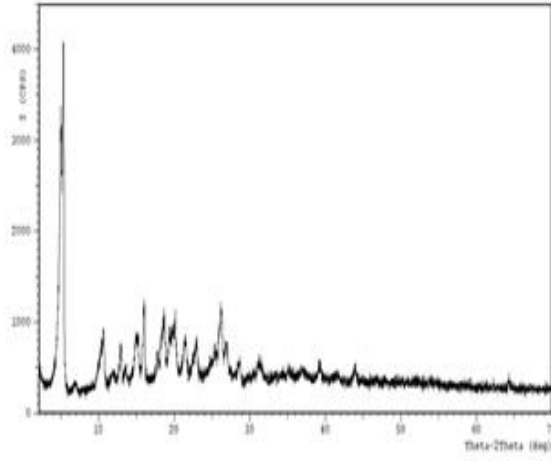
Şekil 117. XXXVII no'lu komp. için XRD
