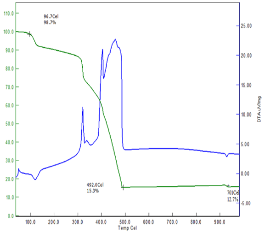
Şekil 206. VI no'lu komp. için TG-DTA
