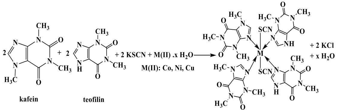
Şekil 4.8. Kafeinin teofilin ve KSCN varlığında Kobalt(II), Nikel(II) ve Bakır(II) kompleks bileşiklerinin eldesi.
