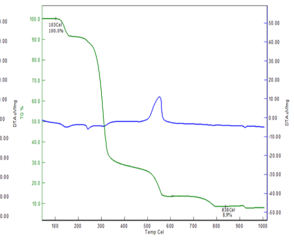
Şekil 216. XVI no'lu komp. için TG-DTA
