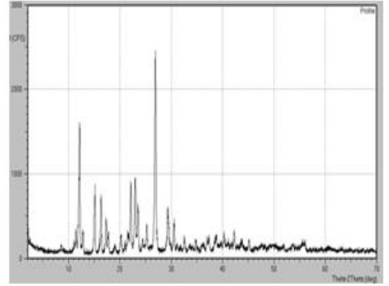
Şekil 88. VIII no'lu kompleks için XRD
