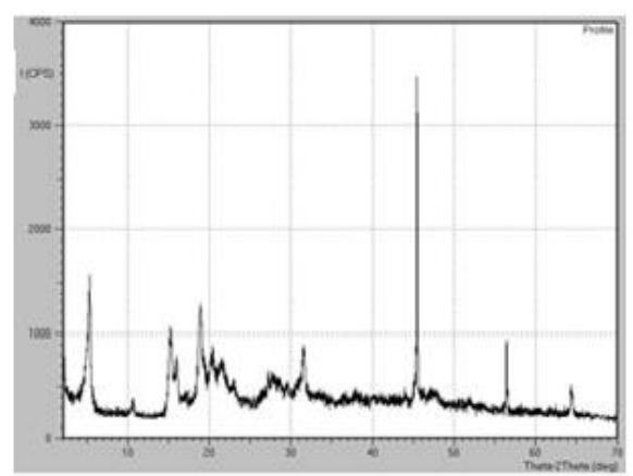
Şekil 110. XXX no'lu kompleks için XRD
