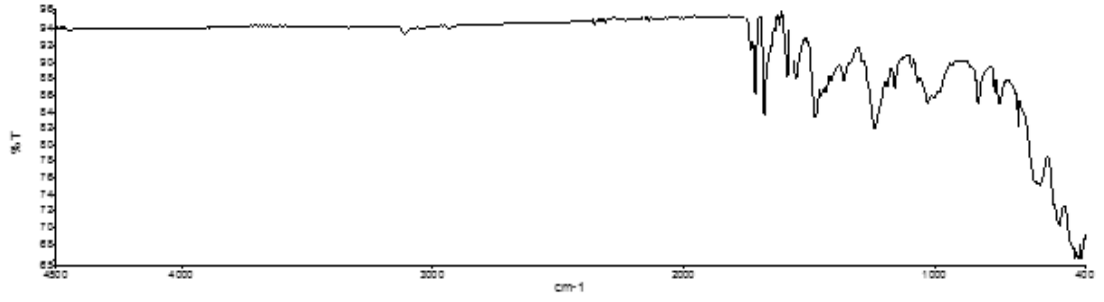
Şekil 45. V no'lu kompleks için FTIR spektrumu.
