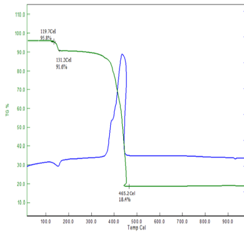
Şekil 223. XXIII no'lu kom. için TG-DTA Şekil 224. XXIV no'lu komp. için TG-DTA
