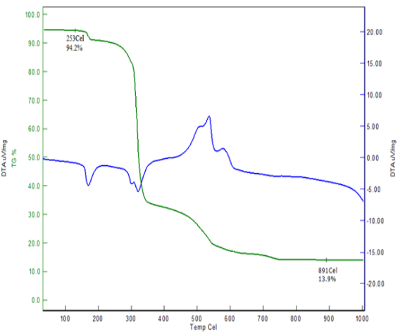
Şekil 238. XXXVIII no'lu komp. TG-DTA
