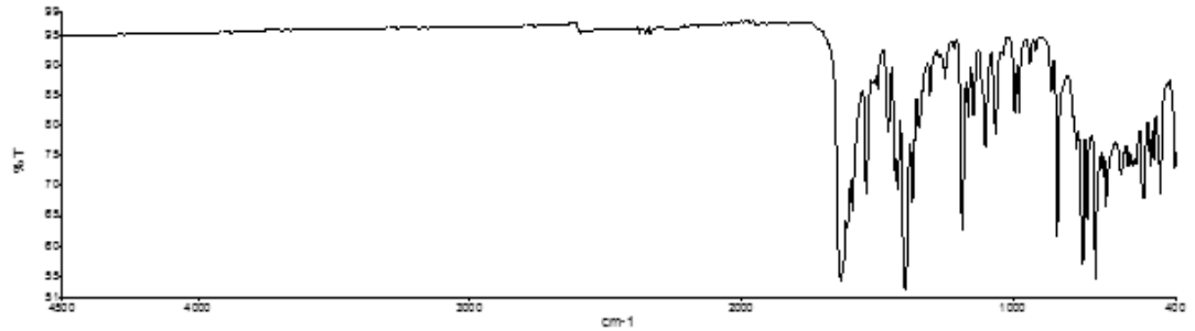
Şekil 77. XXXVII no'lu kompleks için FTIR spektrumu.
