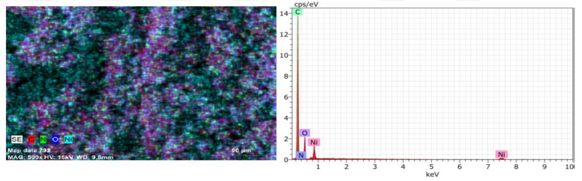
Şekil 159. XXXIX no'lu kompleks için EDX.
