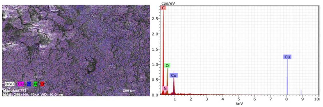
Şekil 153. XXXIII no'lu kompleks için EDX.
