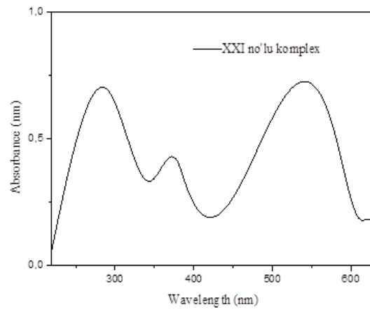
Şekil 21. XXI no'lu kompleks için UV.
