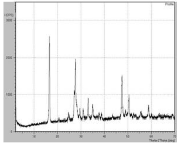
Şekil 92. XII no'lu kompleks için XRD
