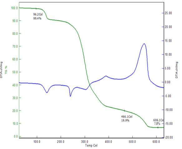
Şekil 212. XII no'lu komp. için TG-DTA
