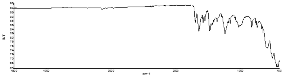
Şekil 46. VI no'lu kompleks için FTIR spektrumu.
