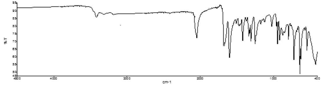
Şekil 59. XIX no'lu kompleks için FTIR spektrumu.
