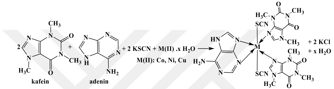
Şekil 4.7. Kafeinin adenin ve KSCN varlığında Kobalt(II), Nikel(II) ve Bakır(II) kompleks bileşiklerinin eldesi.
