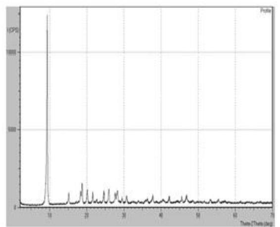
Şekil 102. XXII no'lu kompleks için XRD
