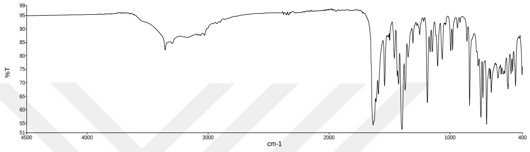
Şekil 79. XXXIX no'lu kompleks için FTIR spektrumu.
