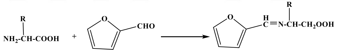
Şekil 4.15. Furfuraldehit varlığında aminoasitlerin Schiff bazlarının eldesi.
