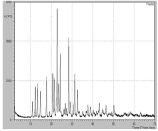
Şekil 94. XIV no'lu kompleks için XRD
