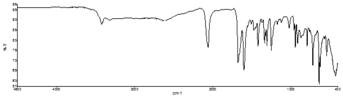
Şekil 56. XVI no'lu kompleks için FTIR spektrumu.
