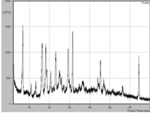
Şekil 81. I no'lu kompleks için XRD
