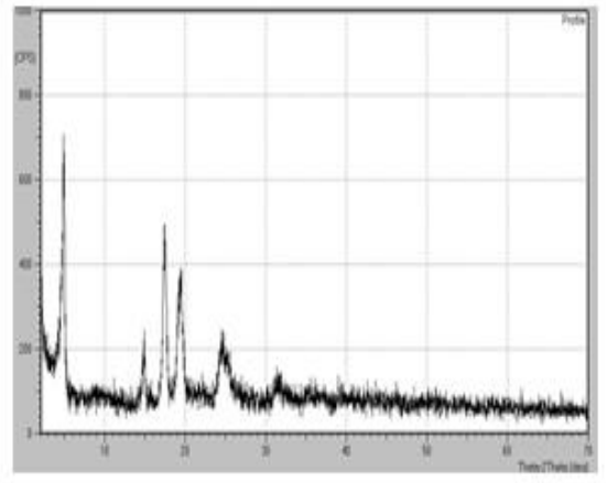
Şekil 118. XXXVIII no'lu komp. için XRD
