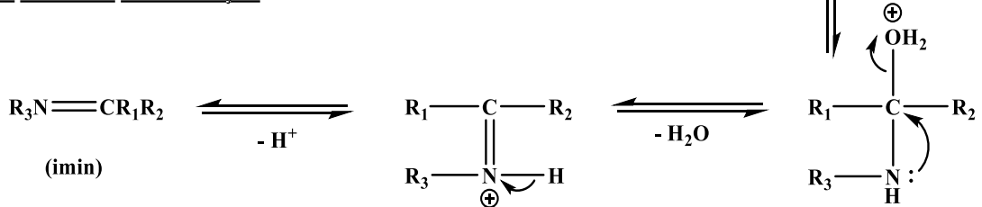
Şekil 2.6. Schiff bazları sentezi (Khan vd., 2021).
