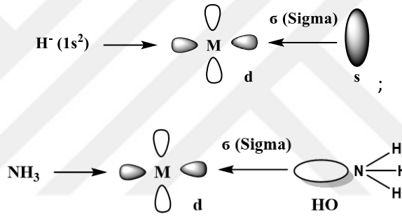
Şekil 2.2. \sigma bağı içeren ligandlar L \rightarrow M ( \sigma bağı).
