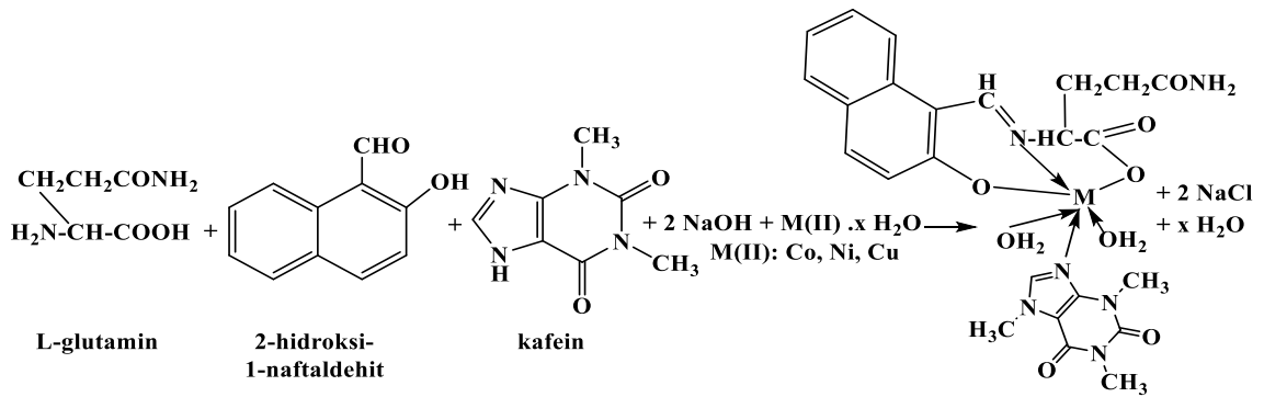
Şekil 4.23. Kafeinin imin 6 varlığında Kobalt(II), Nikel(II) ve Bakır(II) kompleks bileşiklerinin eldesi.
