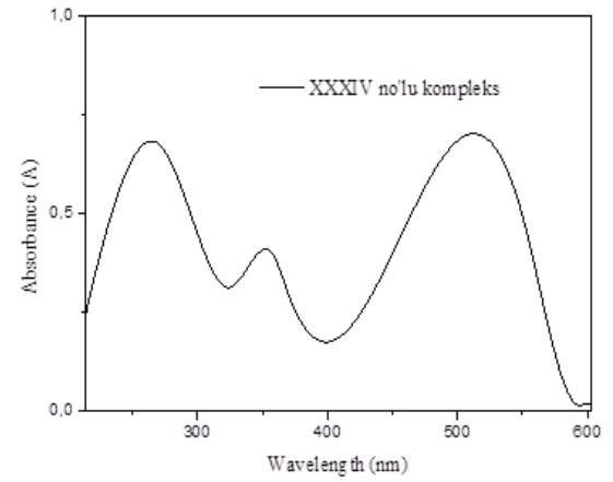
Şekil 34. XXXIV no'lu kompleks için UV.
