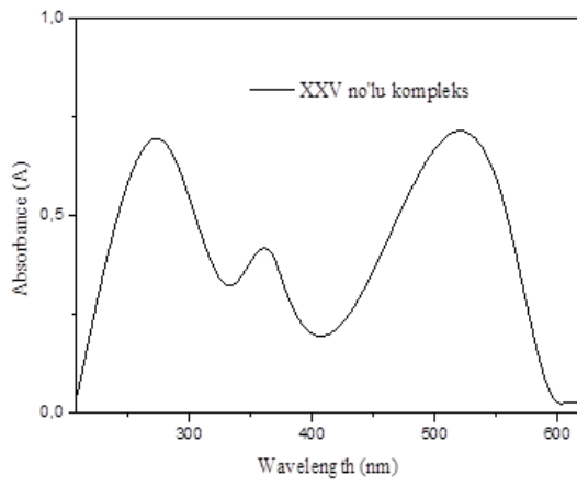
Şekil 25. XXV no'lu kompleks için UV.
