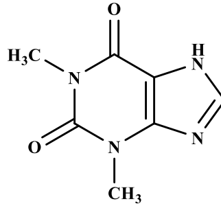
Şekil 2.17. Teofilin ( C_7H_8N_4O_2 ).
