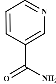
Şekil 2.15. Nikotinamid ( C_6H_5NO_2 ).
