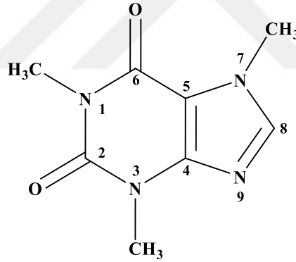
Şekil 2.8. Kafein ( C_8H_{10}N_4O_2 ).
