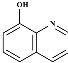
Şekil 2.12. 8-Hidroksikinolin ( \text{C}_9\text{H}_7\text{NO} ).
