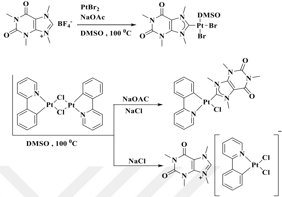
Şekil 2.11. Kafeinin Pt(II) kompleksi (Hu vd., 2011).
