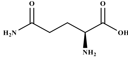
Şekil 2.22. L-Glutamin ( C_5H_{10}N_2O_3 ).
