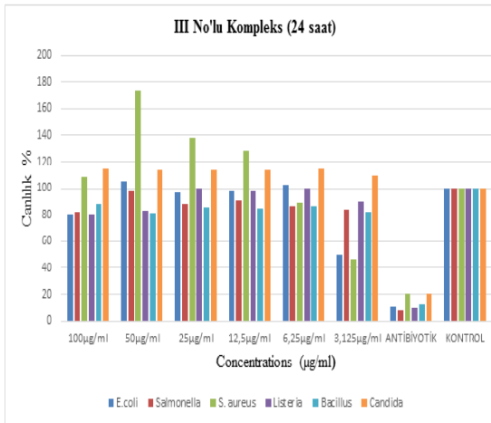
Şekil 243. III no'lu kompleks için antimikrobial analiz.
