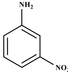
Şekil 2.18. m-Nitroanilin ( C_6H_6N_2O_2 ).
