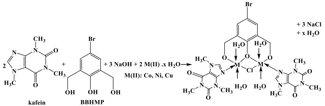
Şekil 4.14. Kafeinin BBHMP varlığında Kobalt(II), Nikel(II) ve Bakır(II) kompleks bileşiklerinin eldesi.
