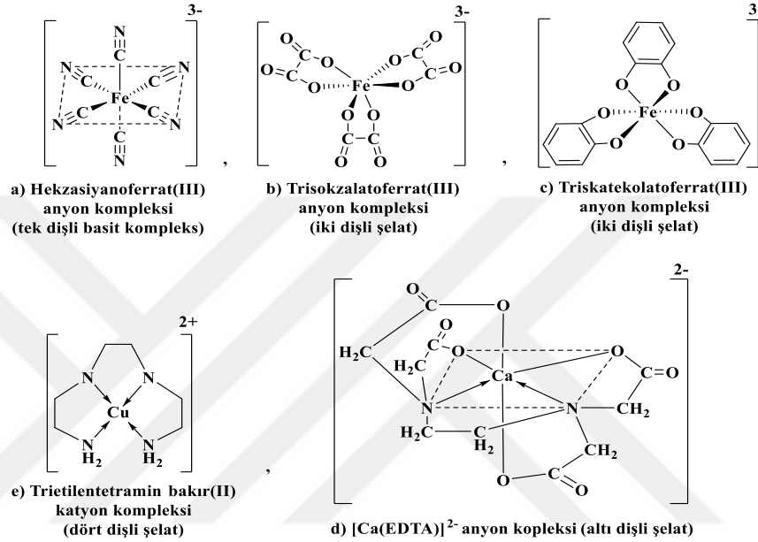
Şekil 2.1. Bazı şelat kompleksi örnekleri.
