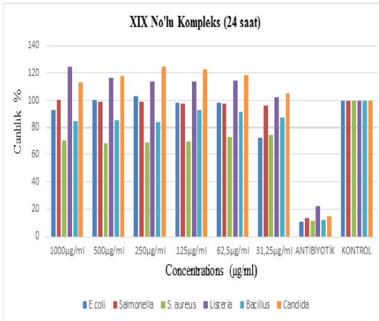
Şekil 246. XIX no'lu kompleks için antimikrobia analiz.
