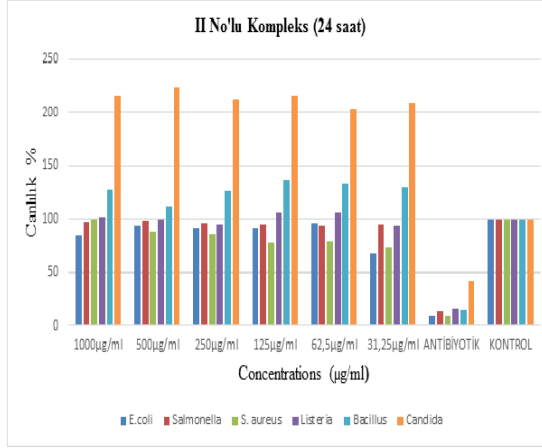
Şekil 242. II no'lu kompleks için antimikrobial analiz.
