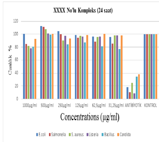
Şekil 255. XXXX no'lu kompleks için antimikrobal analiz.
