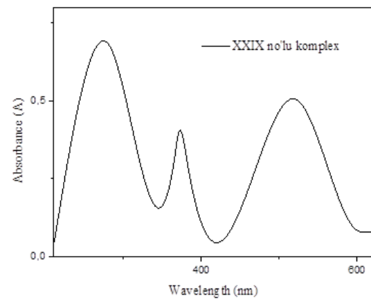
Şekil 29. XXIX no'lu kompleks için UV.
