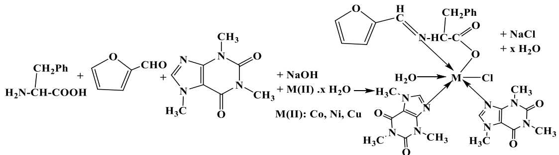
Şekil 4.18. Kafeinin imin 2 varlığında Kobalt(II), Nikel(II) ve Bakır(II) kompleks bileşiklerinin eldesi.
