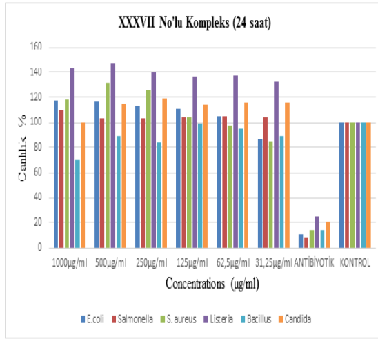
Şekil 253. XXXVII no'lu kompleks için antimikrobal analiz.
