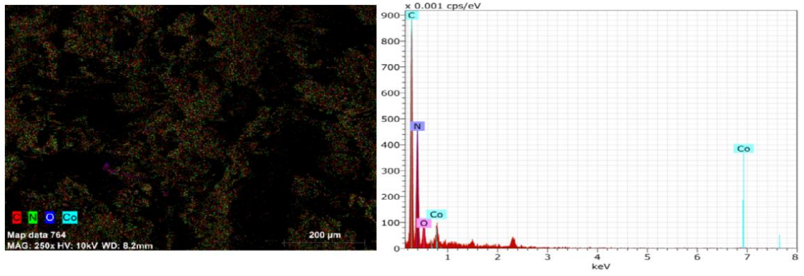
Şekil 136. XVI no'lu kompleks için EDX.
