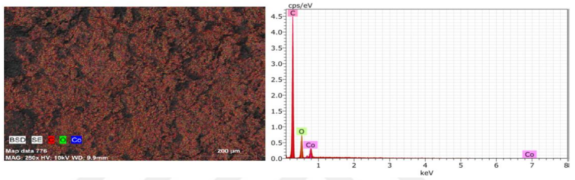
Şekil 158. XXXVIII no'lu kompleks için EDX.
