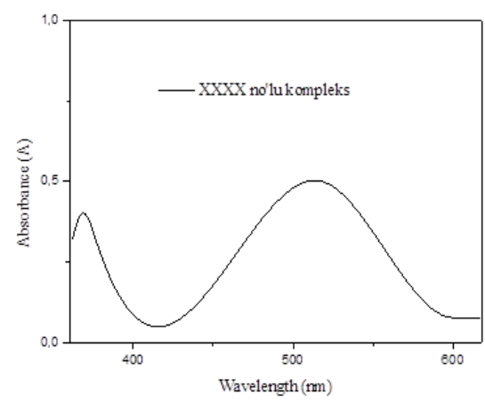
Şekil 40. XXXX no'lu kompleks için UV.
