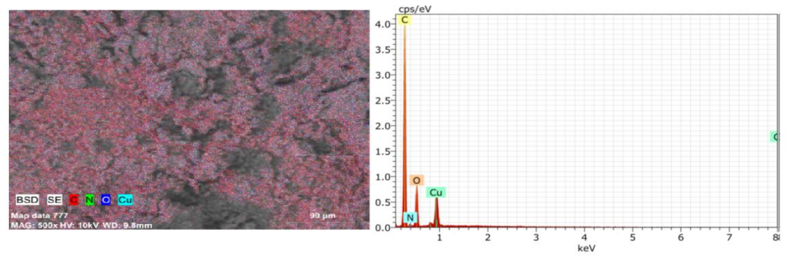
Şekil 147. XXVII no'lu kompleks için EDX.
