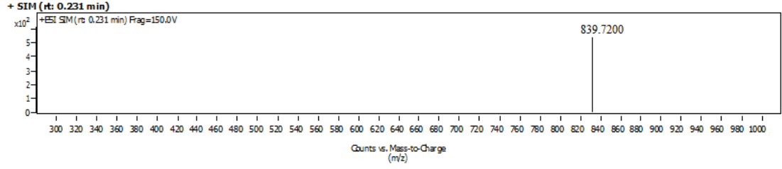
Şekil 5.17. XVII no'lu kompleks bileşiğin LC-MS spektrum grafiği.
