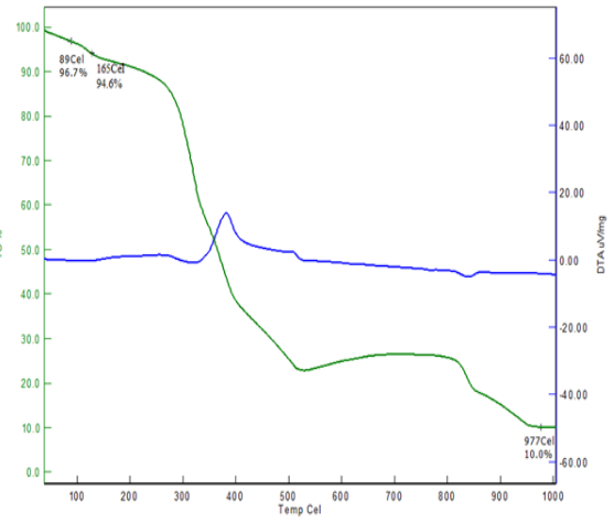
Şekil 225. XXV no'lu komp. için TG-DTA Şekil 226. XXVI no'lu komp. için TG-DTA
