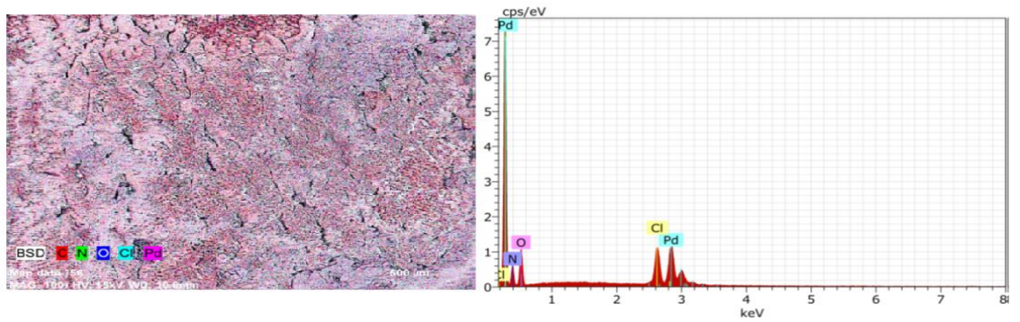
Şekil 123. III no'lu kompleks için EDX.
