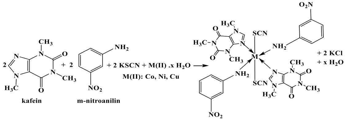
Şekil 4.9. Kafeinin m-nitroanilin ve KSCN varlığında Co(II), Ni(II) ve Cu(II) kompleks bileşiklerinin eldesi.
