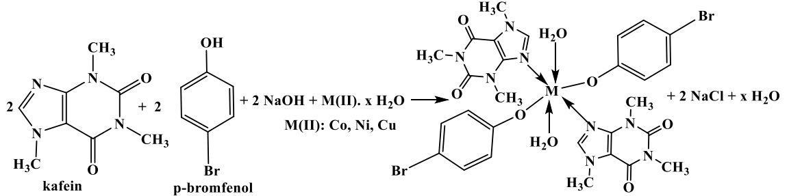
Şekil 4.4. Kafeinin p-bromfenol varlığında Kobalt(II), Nikel(II) ve Bakır(II) kompleks bileşiklerinin eldesi.
