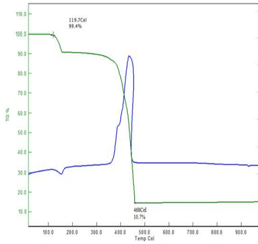
Şekil 211. XI no'lu kompleks için TG-DTA
