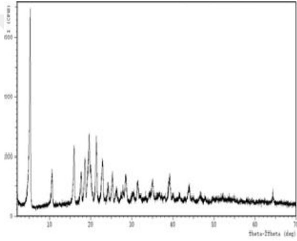
Şekil 105. XXV no'lu kompleks için XRD
