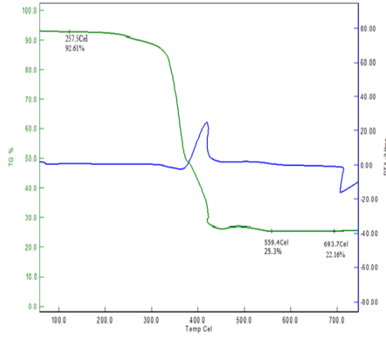
Şekil 201. I no'lu kompleks için TG-DTA
