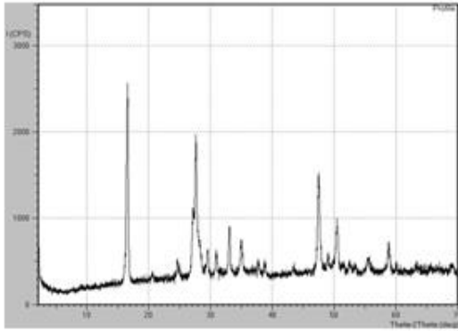
Şekil 113. XXXIII no'lu kompleks için XRD
