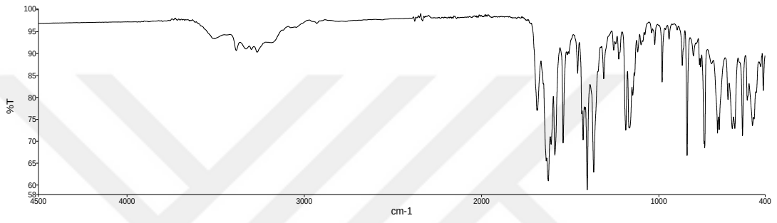
Şekil 71. XXXI no'lu kompleks için FTIR spektrumu.
