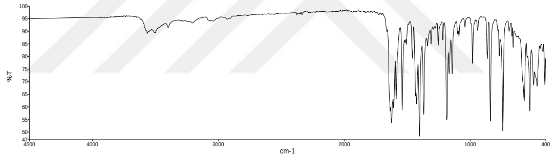
Şekil 80. XXXX no'lu kompleks için FTIR spektrumu.
