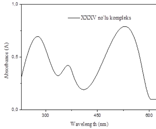
Şekil 35. XXXV no'lu kompleks için UV.
