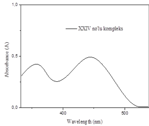
Şekil 24. XXIV no'lu kompleks için UV.
