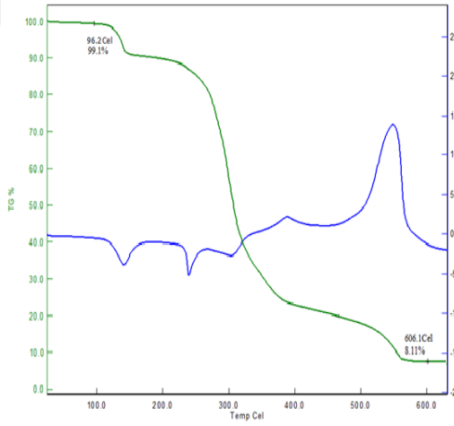
Şekil 211. XI no'lu kompleks için TG-DTA
