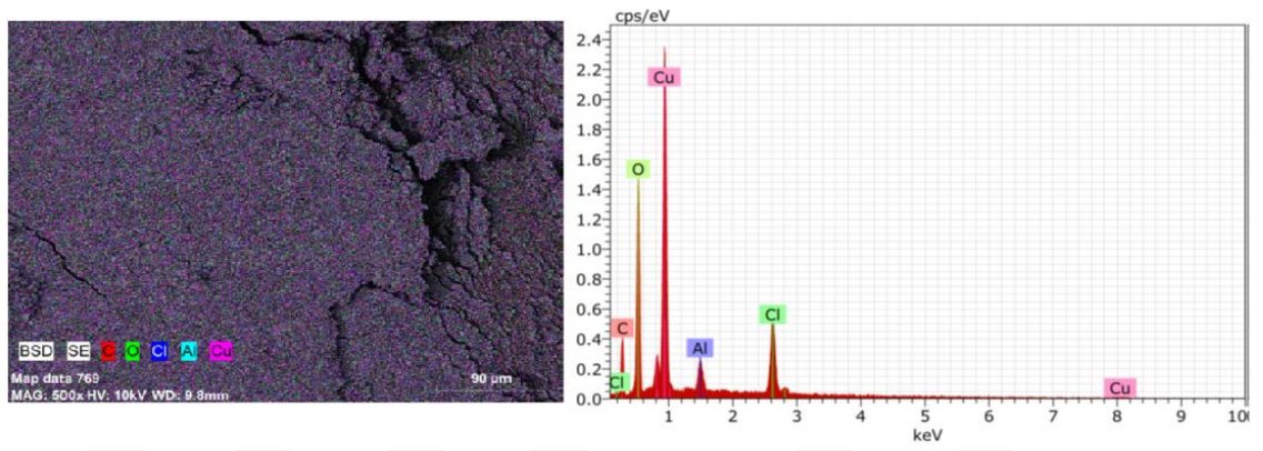
Şekil 143. XXIII no'lu kompleks için EDX.
