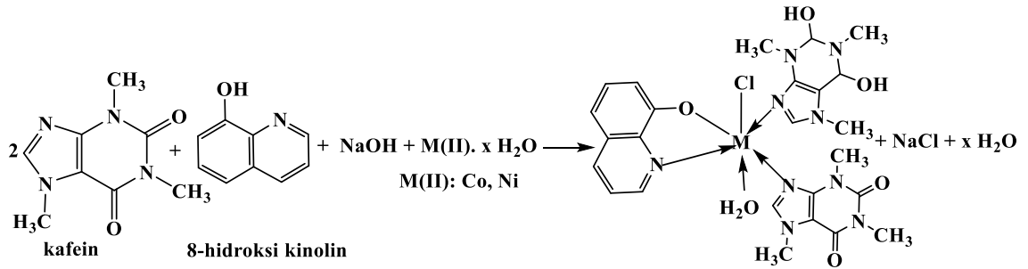
Şekil 4.1. Kafeinin 8-hidroksikinolin varlığında Kobalt(II) ve Nikel(II) kompleks bileşiklerinin eldesi.
