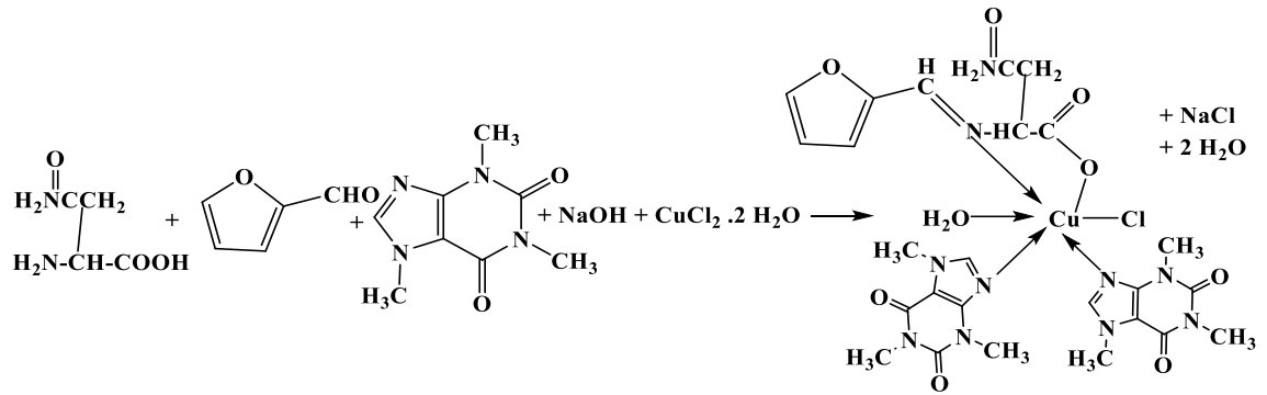
Şekil 4.17. Kafeinin imin 1 varlığında Bakır(II) kompleks bileşiğinin eldesi.
