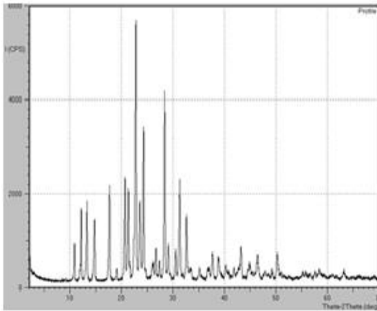
Şekil 95. XV no'lu kompleks için XRD
