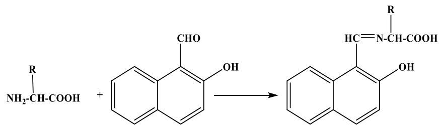
Şekil 4.16. 2-hidroksi-1-naftaldehit varlığında aminoasitlerin Schiff bazlarının eldesi.
