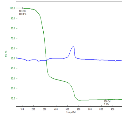
Şekil 215. XV no'lu komp. için TG-DTA
