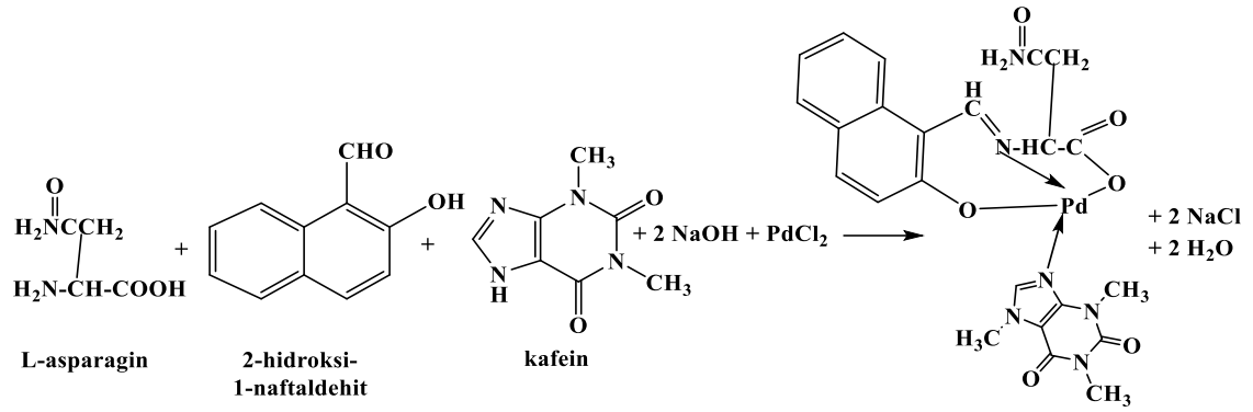
Şekil 4.21. Kafeinin imin 4 varlığında Palladyum(II) kompleks bileşiğinin eldesi.
