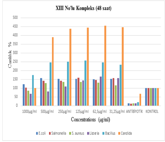
Şekil 245. XIII no'lu kompleks için antimikrobia analiz
