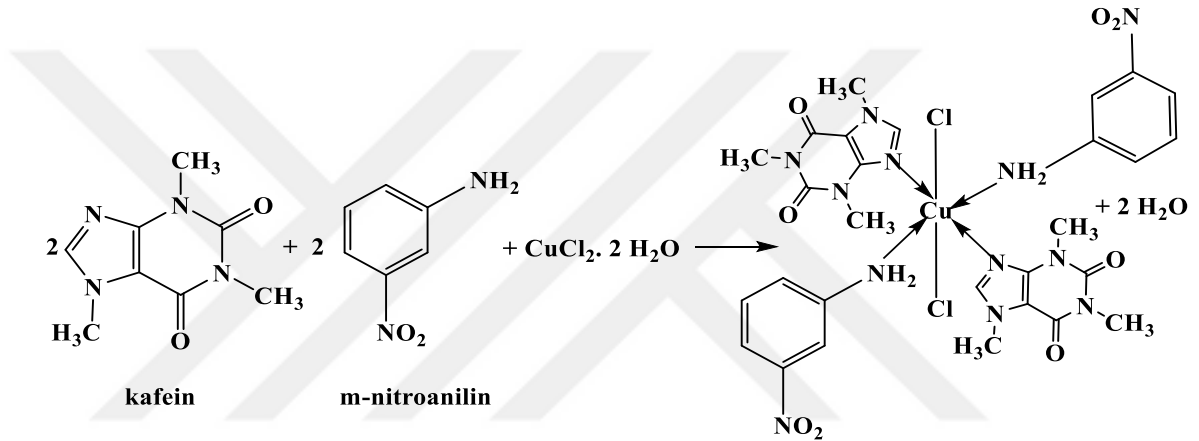
Şekil 4.11. Kafeinin m-nitroanilin varlığında Bakır(II) kompleks bileşiğinin eldesi.
