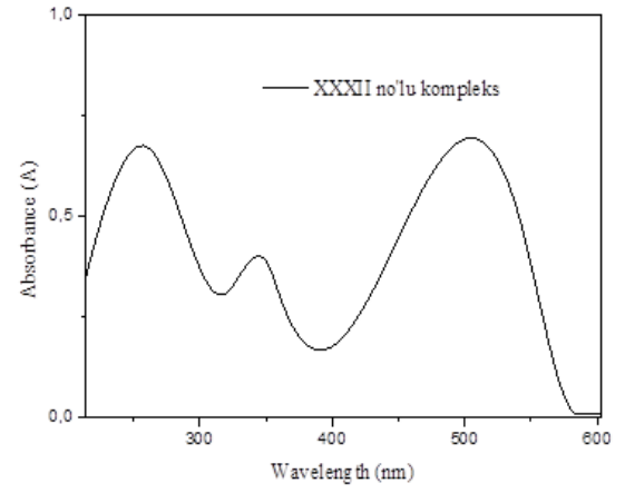
Şekil 32. XXXII no'lu kompleks için UV.
