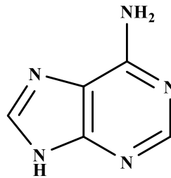
Şekil 2.16. Adenin ( C_5H_5N_5 ).
