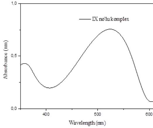
Şekil 9. IX no'lu kompleks için UV.
