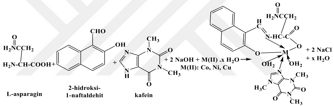
Şekil 4.20. Kafeinin imin 4 varlığında Kobalt(II), Nikel(II) ve Bakır(II) kompleks bileşiklerinin eldesi.
