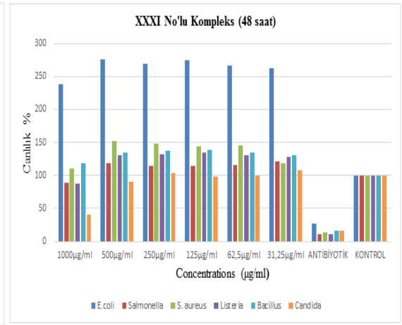
Şekil 247. XXXI no'lu kompleks için antimikrobial analiz.
