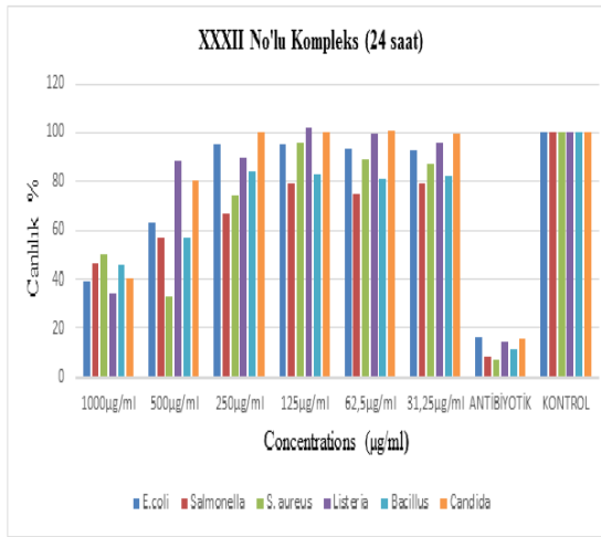
Şekil 248. XXXII no'lu kompleks için antimikrobial analiz.
