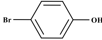
Şekil 2.13. p-Bromfenol ( C_6H_5BrO ).
