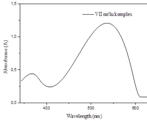
Şekil 7. VII no'lu kompleks için UV.
