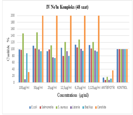
Şekil 244. IV no'lu kompleks için antimikrobia analiz.
