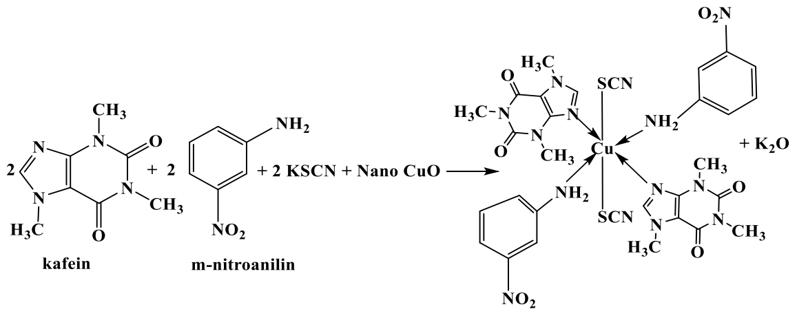
Şekil 4.10. Kafeinin m-nitroanilin ve KSCN varlığında nano Bakır(II) kompleks bileşiğinin eldesi.
