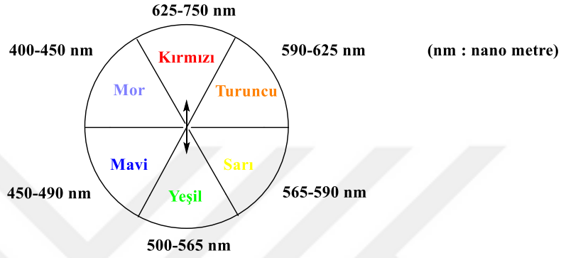
Şekil 2.7. Renk çemberi.
