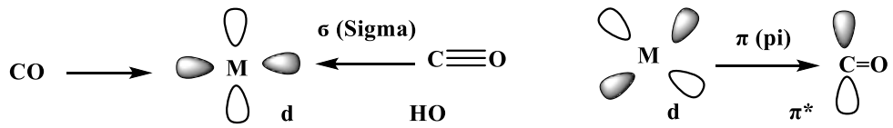
Şekil 2.5. Düşük enerjili \pi^* orbitalleri olan ligandlar.
