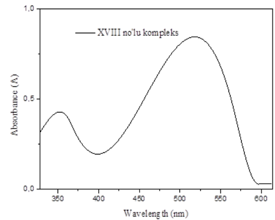
Şekil 18. XVIII no'lu kompleks için UV.
