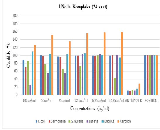
Şekil 241. I no'lu kompleks için antimikrobial analiz.
