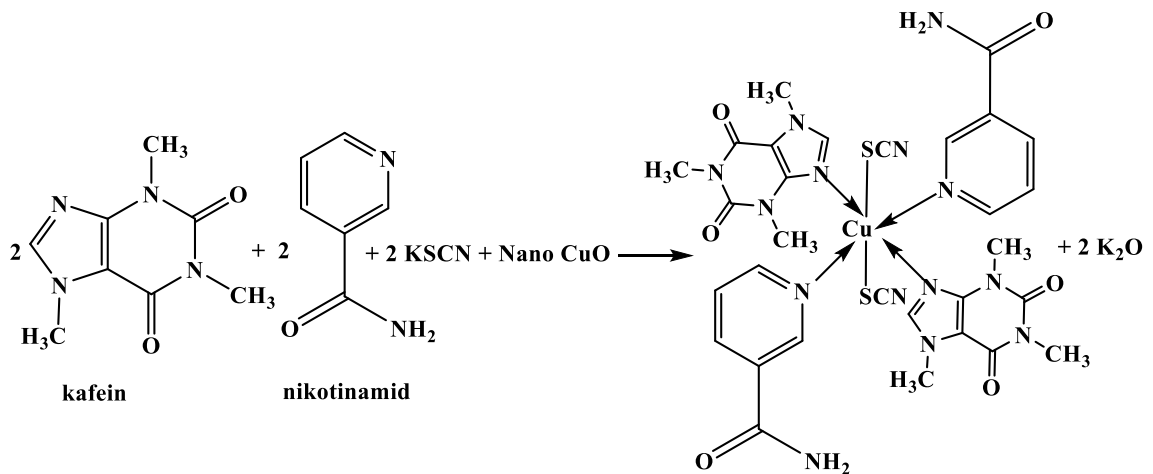
Şekil 4.6. Kafeinin nikotinamid ve KSCN varlığında nano Bakır(II) kompleks bileşiğinin eldesi.
