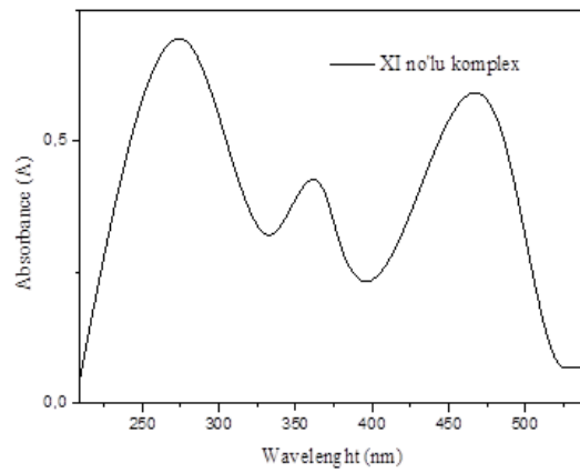
Şekil 11. XI no'lu kompleks için UV.
