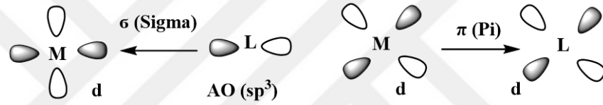
Şekil 2.4. \pi alıcı ligandlar, L \rightarrow M ( \sigma bağı), M \rightarrow L ( \pi bağı) (Geri bağlanma).
