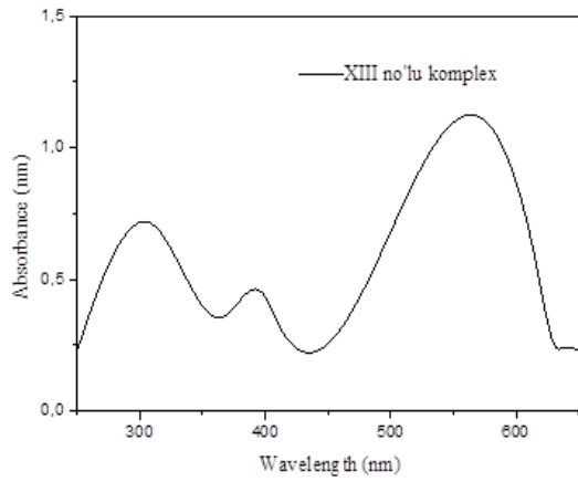
Şekil 13. XIII no'lu kompleks için UV.
