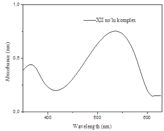
Şekil 12. XII no'lu kompleks için UV.
