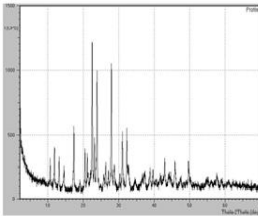
Şekil 85. V no'lu kompleks için XRD
