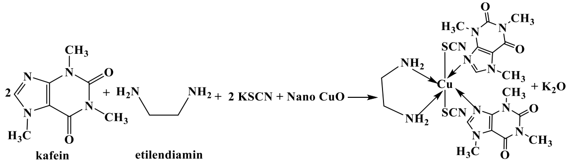
Şekil 4.5. Kafeinin etilendiamin ve KSCN varlığında nano Bakır(II) kompleks bileşiğinin eldesi.
