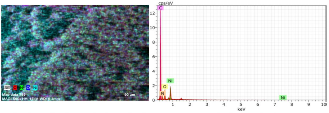
Şekil 137. XVII no'lu kompleks için EDX.
