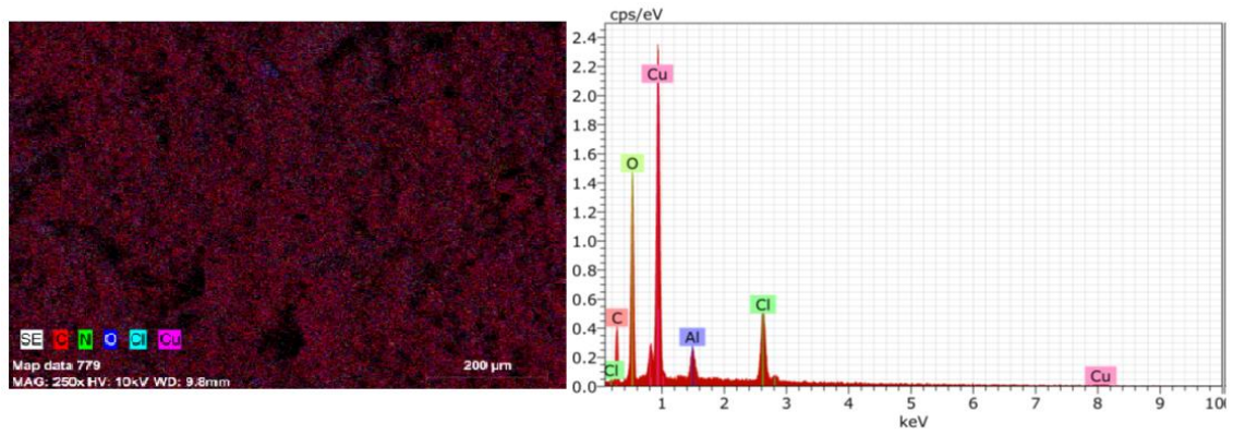
Şekil 138. XVIII no'lu kompleks için EDX.
