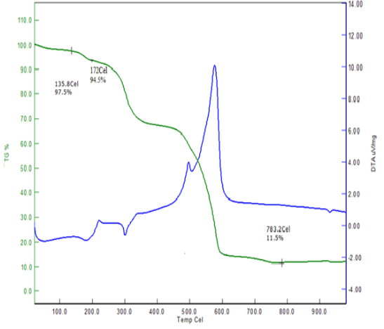
Şekil 202. II no'lu kompleks için TG-DTA
