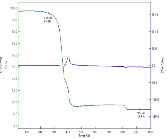
Şekil 236. XXXVI no'lu komp. TG-DTA
