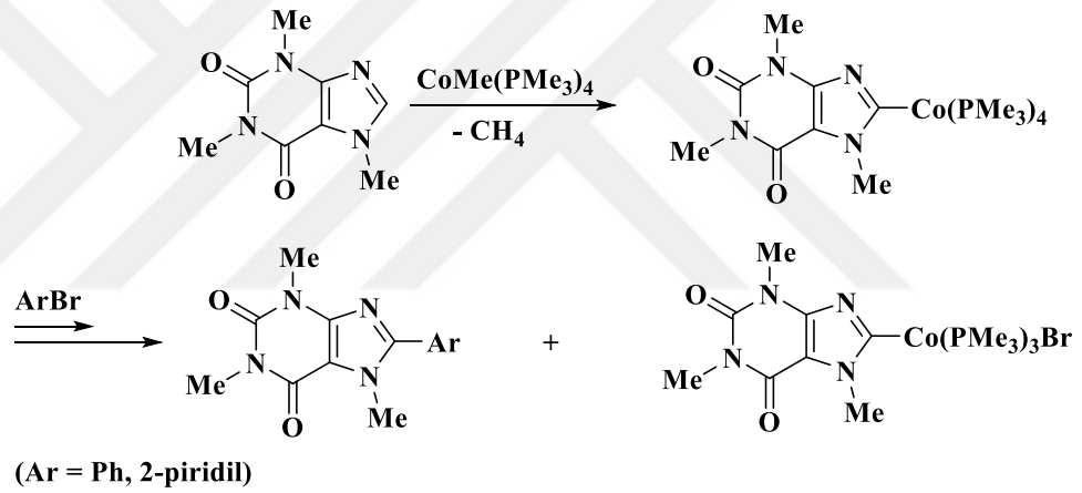
Şekil 2.10. Kafeinin Co(II) kompleksi (Saker ve Farina, 2010).
