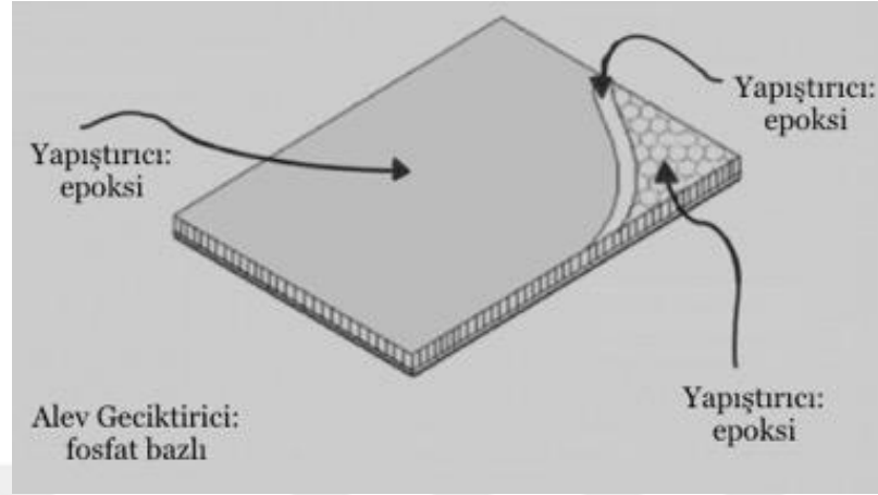
Şekil 26: Petek Sandviç Panel Bileşenleri (Santos ve diğ., 2016).
