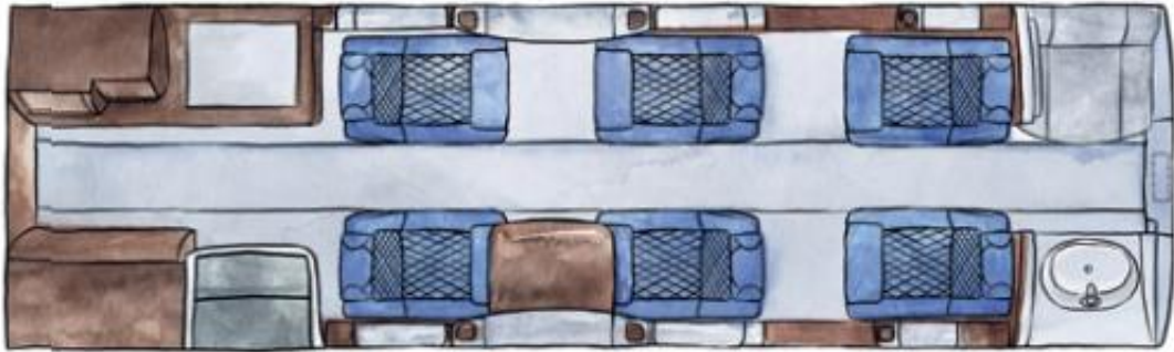
Şekil 36: Embraer Phenom 300E Standart Yerleşim Planı (URL-31).
