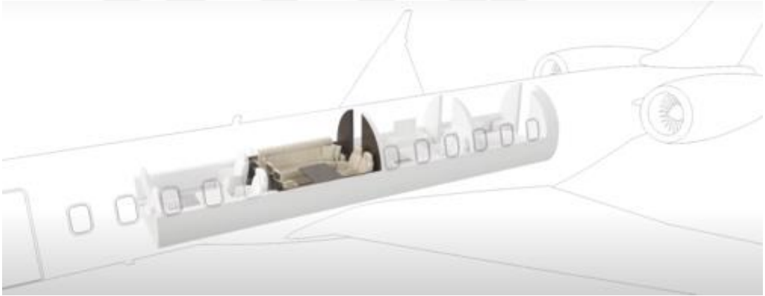
Şekil 68: Bombardier Global 7500 İkinci Zoning Alanı, Karşılıklı Yerleştirilmiş Dört Yolcu Koltuğu ve Üçlü Koltuk Düzeni (URL-37).
