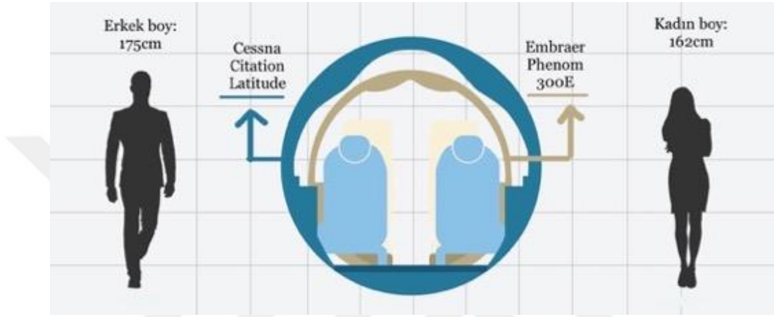
Şekil 121: Cessna Citation Latitude ve Embraer Phenom 300E Karşılaştırmalı Kabin Kesitleri.
