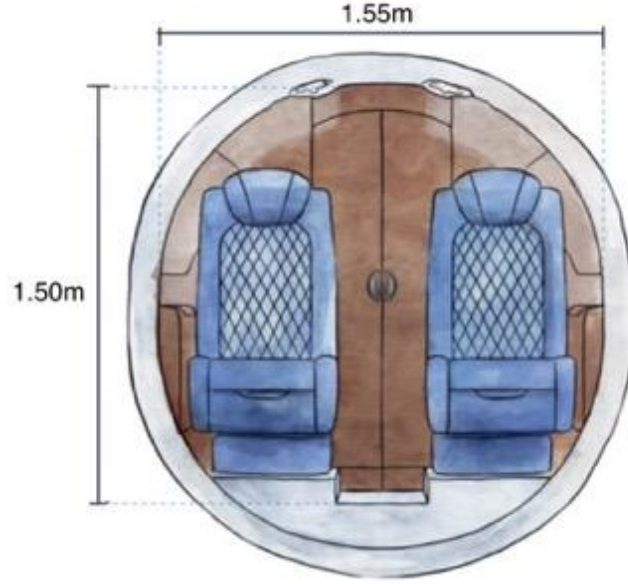
Şekil 35: Embraer Phenom 300E Kabin Kesit Görünüşü (URL-31).
