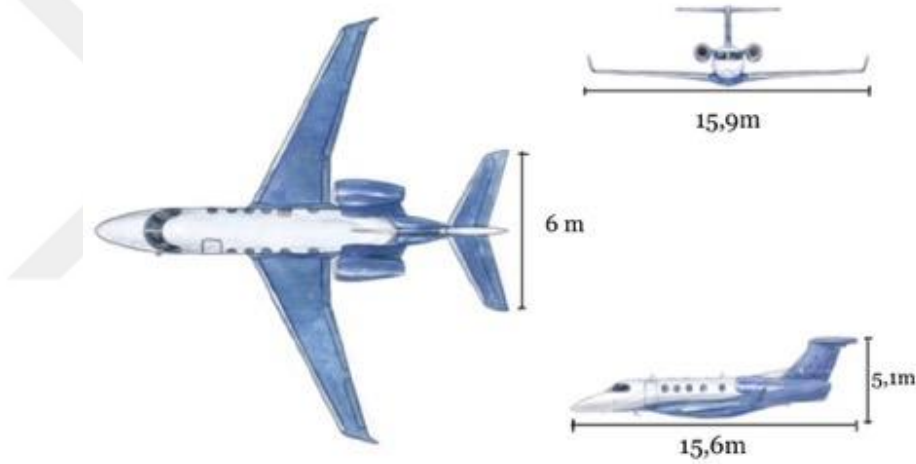
Şekil 34: Embraer Phenom 300E Plan ve Görünüş Çizimleri (URL-31).
