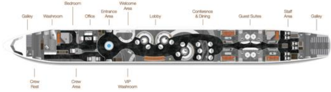
Şekil 116: Airbus ACJ330neo “Enjoy Extra Personal Space” Yerleşim Planı (URL-48).
