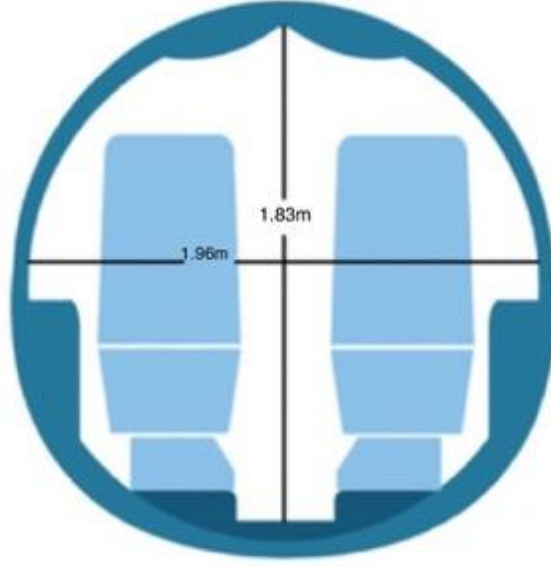
Şekil 52: Cessna Citation Latitude Kabin Kesit Görünüşü (URL-35).
