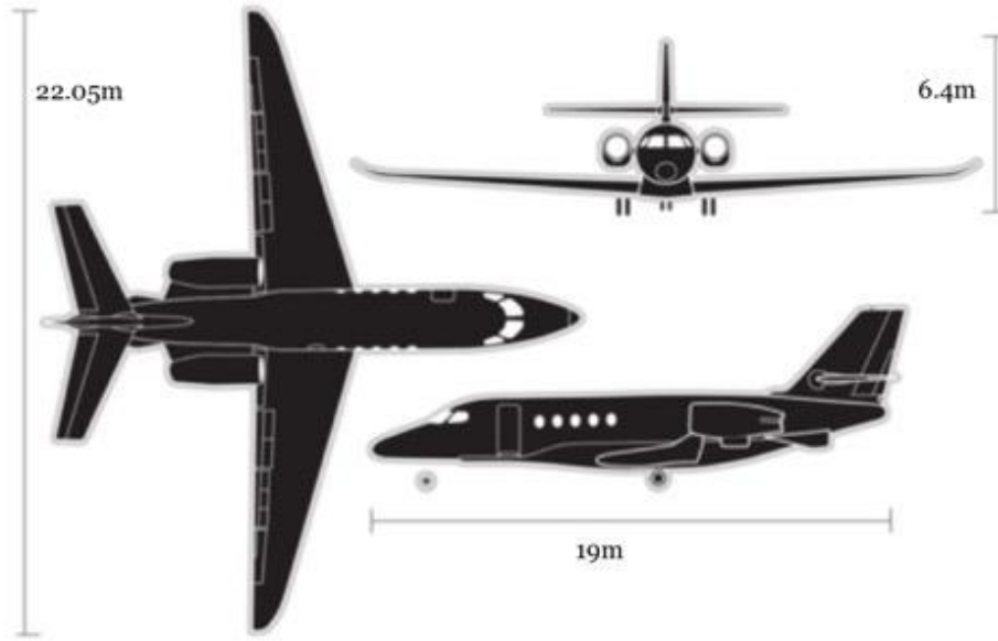
Şekil 51: Cessna Citation Latitude Plan ve Görünüş Çizimleri (URL-33 ).
