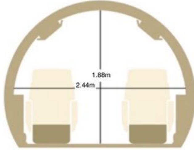
Şekil 61: Bombardier Global 7500 Kabin Kesit Görünüşü (URL-38).
