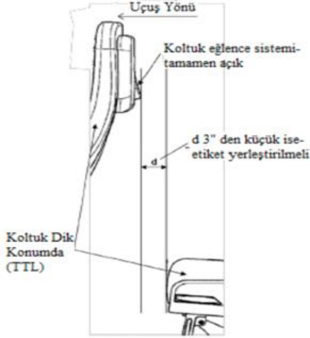
Şekil 18: A 350 Modeli İçin Airbus Firması Tarafından Belirlenen Koltuk Standardı (Criou, 2016).
