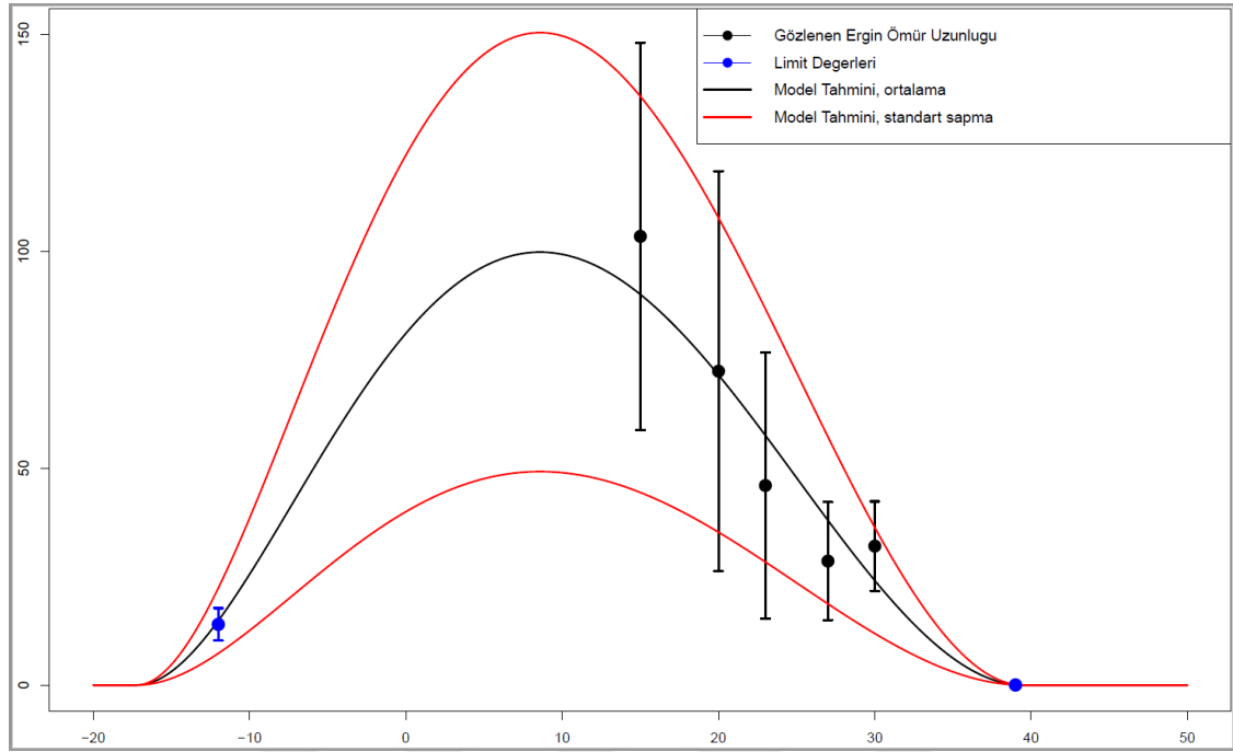
Şekil 4.1.4.2. Sıcaklığa bağlı ergin ömür uzunluğu ve model tahmini
