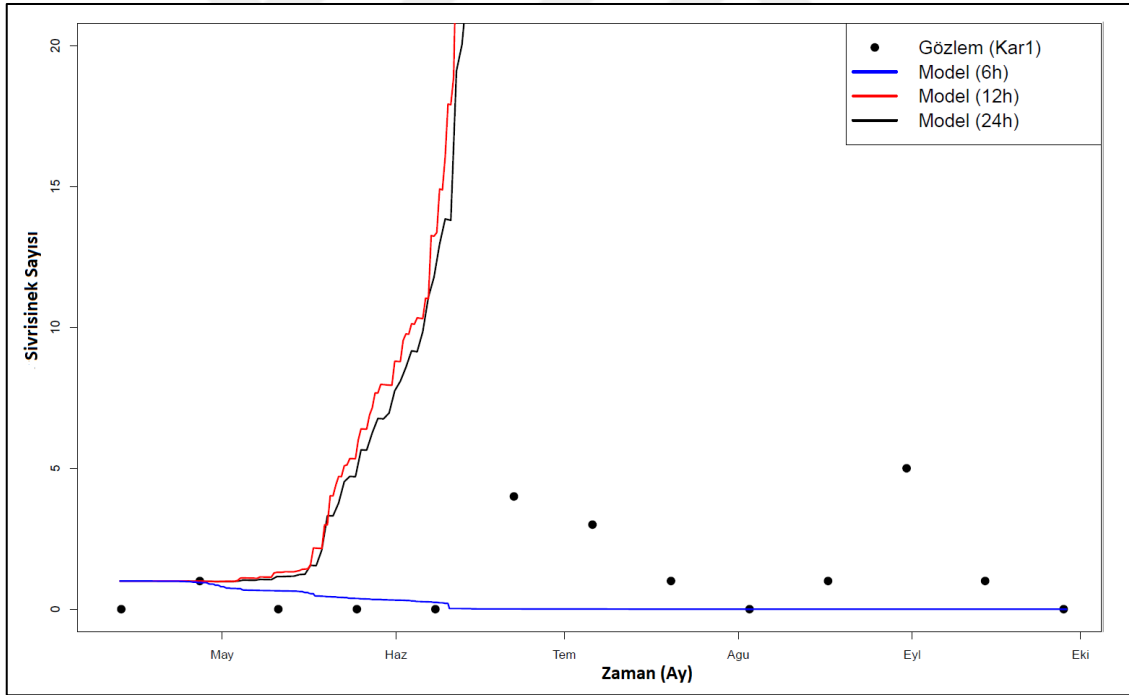
Şekil 4.4.1.1. Kar1 data logger sıcaklığı ile çalıştırılan model ve Kar1 tuzağı popülasyon dinamiği karşılaştırması
