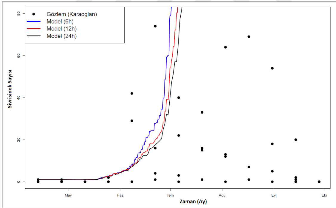
Şekil 4.4.1.6. Kar6 data logger sıcaklığı ile çalıştırılan model ve Karaoglan bölgesindeki tüm tuzaklardaki popülasyon dinamiği karşılaştırması
