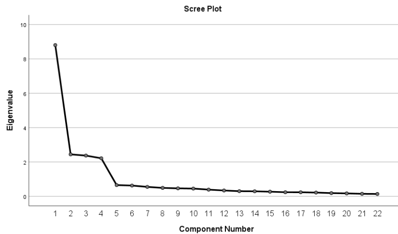
Şekil 3.4: Scree Plot Grafiği
