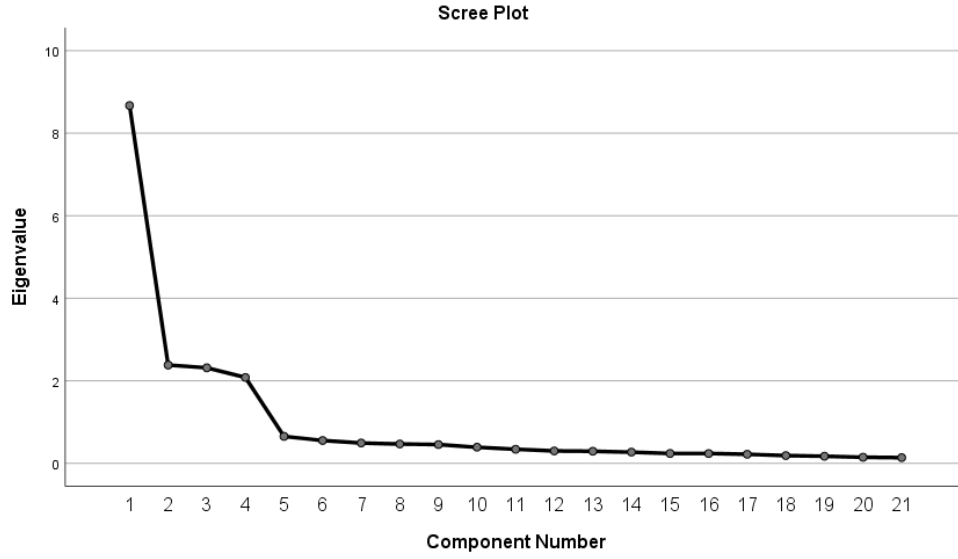
Şekil 3.6: Scree Plot Grafiği 2
