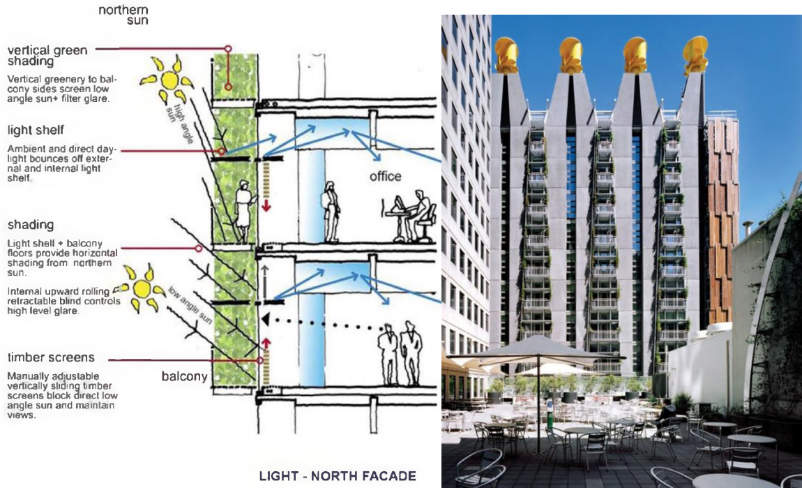
Şekil 5.16: Kuzey Cephesinde Bulunan Balkonların Çalışma Prensibi (Pearce, 2006) ve Balkonlar (Snape, 2013)
