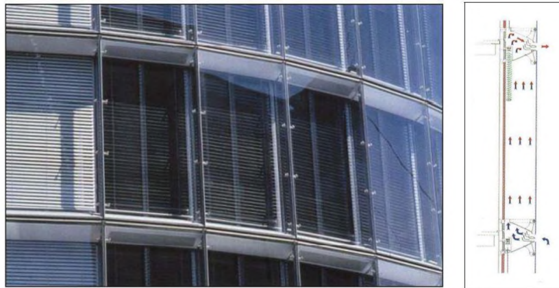
Şekil 4.14: Kutu Tipi Çift Tabaka Cephe Örneği, RWE Binası (Gür N. V., 2007)
