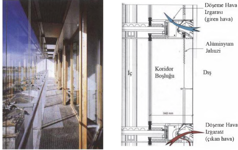
Şekil 4.13: Koridor Tipi Çift Tabaka Cephe Örneği, Staddtor Binası (Ünalan & Tokman, 2011)
