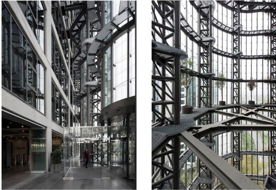
Şekil 4.12: Çok Katlı Çift Tabaka Cephe Örneği- Maslak No.1 Ofis Binası (Maslak No/1, 2014)
