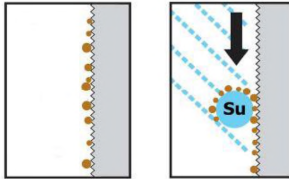
Şekil 4.21: Lotus özellikli cephede kendini temizleme mekanizması (STO, 2005)
