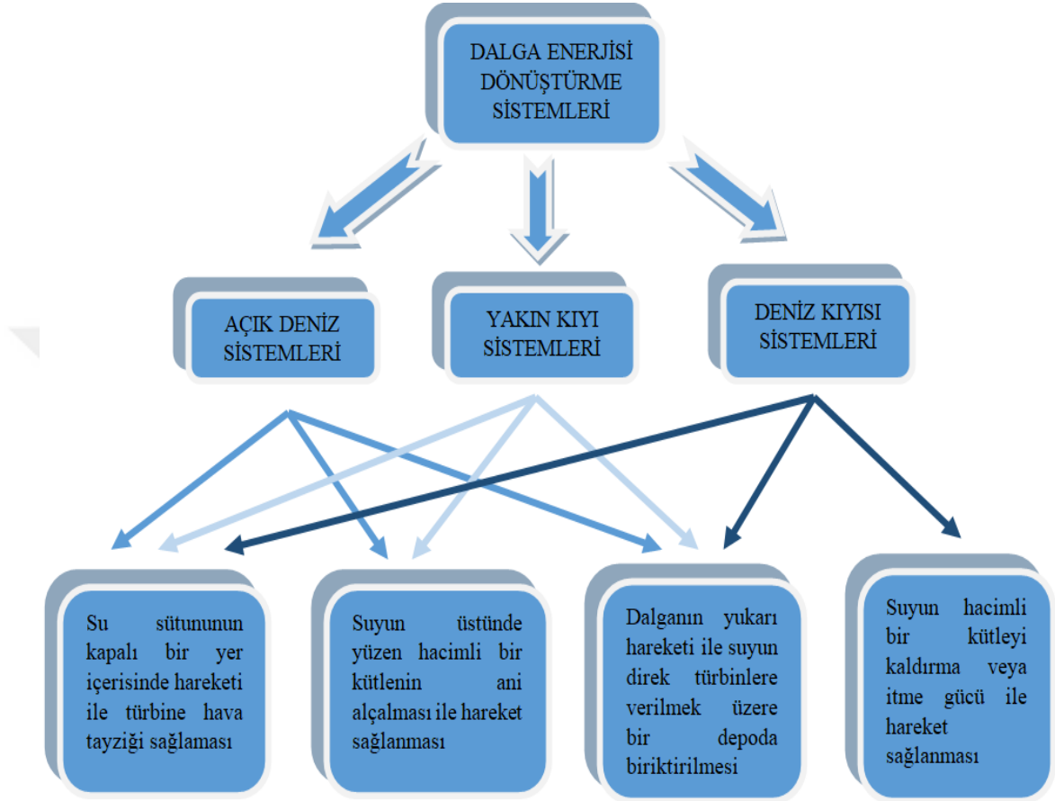
Şekil 1. Dalga enerji dönüştürücüleri sistemleri ve işlemleri
