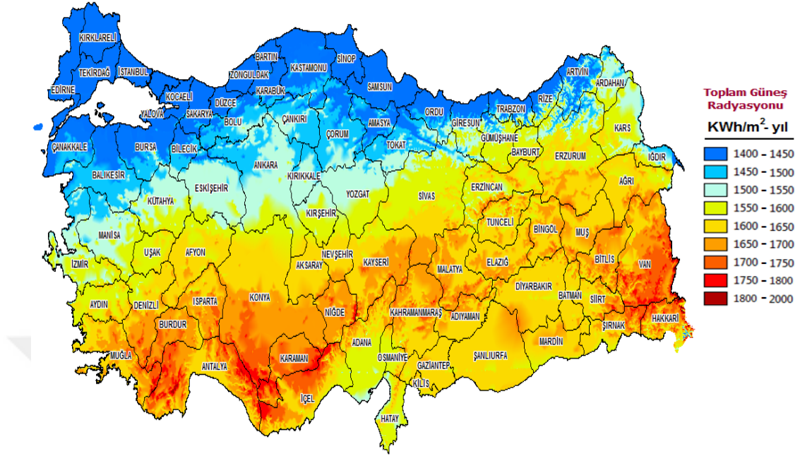
Şekil 4. Türkiye'nin Toplam Güneş Radyasyonu
