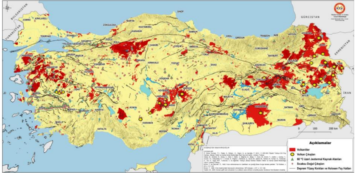
Şekil 3. Jeotermal Kaynaklar ve Volkanik Alanlar Haritası
