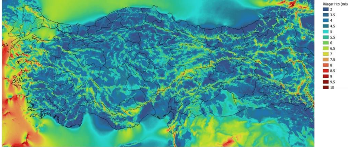
Şekil 2. Türkiye Ortalama Rüzgâr Hızları Haritası
