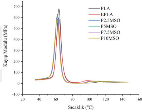
Şekil 3.42: MSO katkılı PLA malzemelerin sıcaklığa bağlı E'' değişimi
