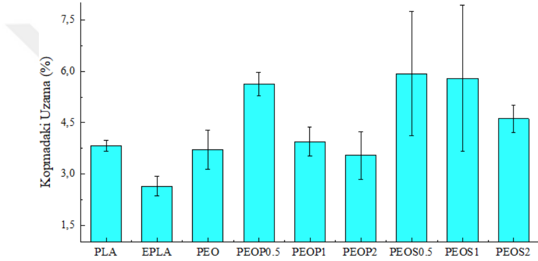
Şekil 3.28: PLAG-MAH ve Silan katkılı PEO malzemelerin kopmadaki yüzde uzaması
