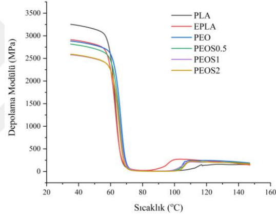
Şekil 3.50: Silan katkılı PEO kompozitlerinin sıcaklığa bağlı E' değişimi
