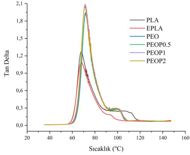
Şekil 3.49: PLAG-MAH katkılı PEO kompozitlerinin sıcaklığa bağlı Tan Delta değişimi
