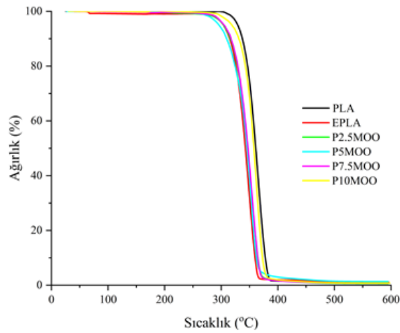
Şekil 3.54: MOO katkılı PLA malzemelerin TGA termogramları
