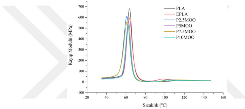
Şekil 3.39: MOO katkılı PLA malzemelerin sıcaklığa bağlı E" değişimi
