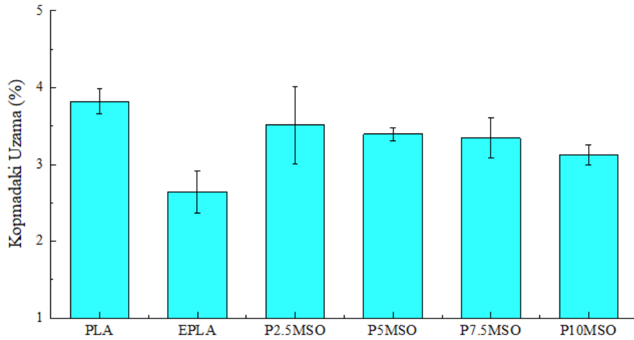
Şekil 3.21: MSO katkılı PLA malzemelerin kopmadaki yüzde uzaması
