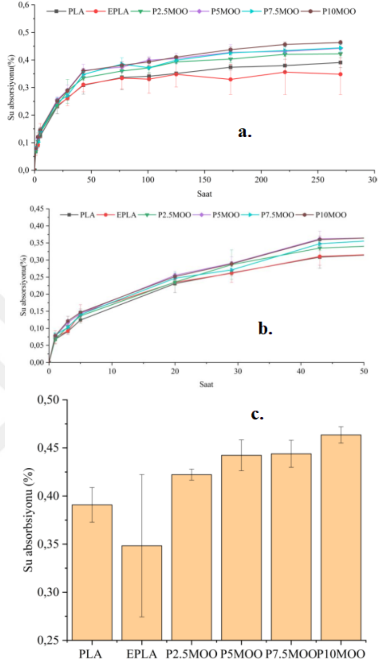
Şekil 3.73: MOO katkılı PLA malzemelerin su absorpsiyon grafikleri
