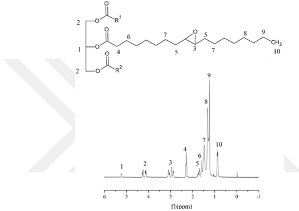
Şekil 3.2: ESBO yağının H-NMR spektrumu ve yapısal gösterimi
