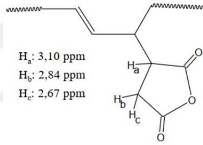
Şekil 3.4: Maleik anhidrit protonlarının NMR kimyasal kaymaları
