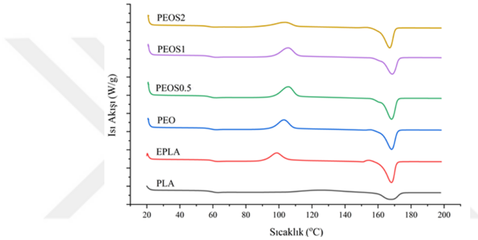
Şekil 3.63: Silan katkılı PEO kompozitlerinin DSC termogramları
