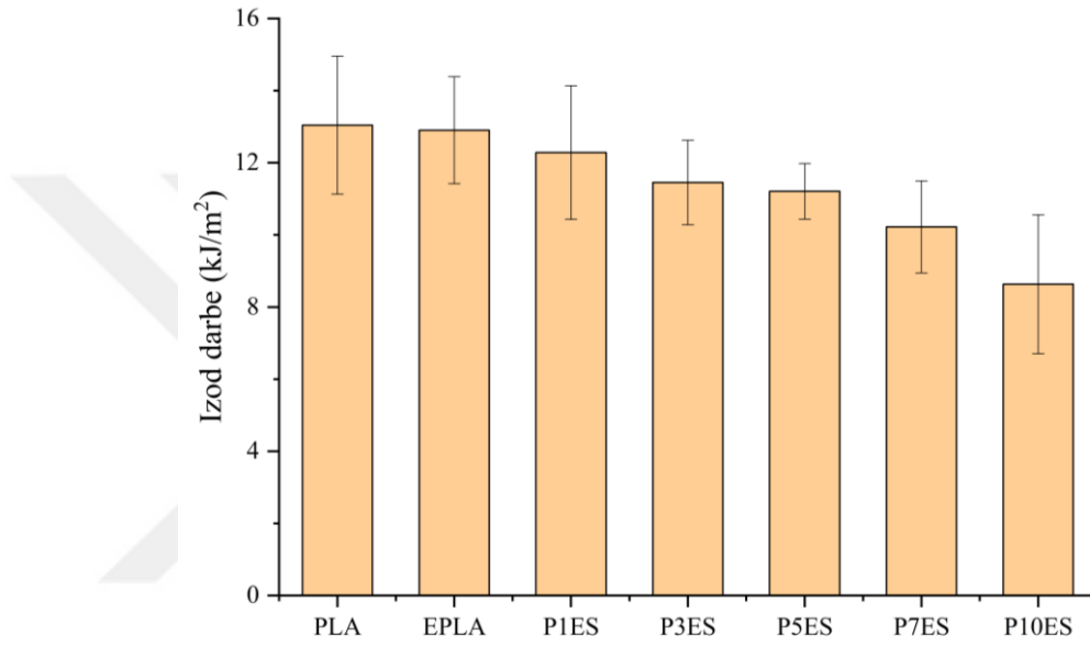
Şekil 3.32: ES dolgulu PLA malzemelerin çentiksiz Izod darbe sonuçları
