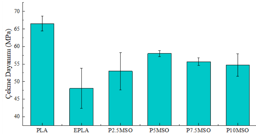
Şekil 3.19: MSO katkılı PLA malzemelerin maksimum çekme dayanımı
