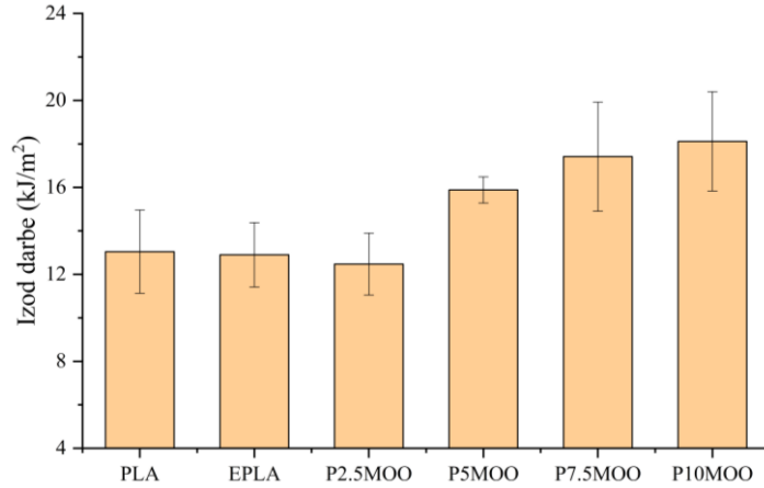
Şekil 3.31: MOO katkılı PLA malzemelerinin çentiksiz Izod darbe sonuçları
