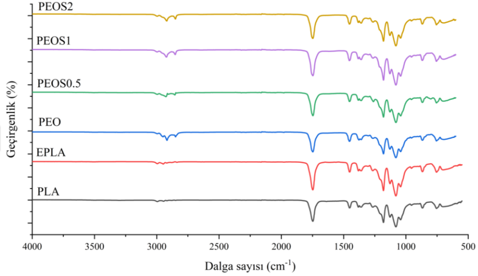
Şekil 3.69: Silan katkılı PEO kompozitlerin FTIR spektrumları
