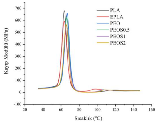
Şekil 3.51: Silan katkılı PEO kompozitlerinin sıcaklığa bağlı E'' değişimi
