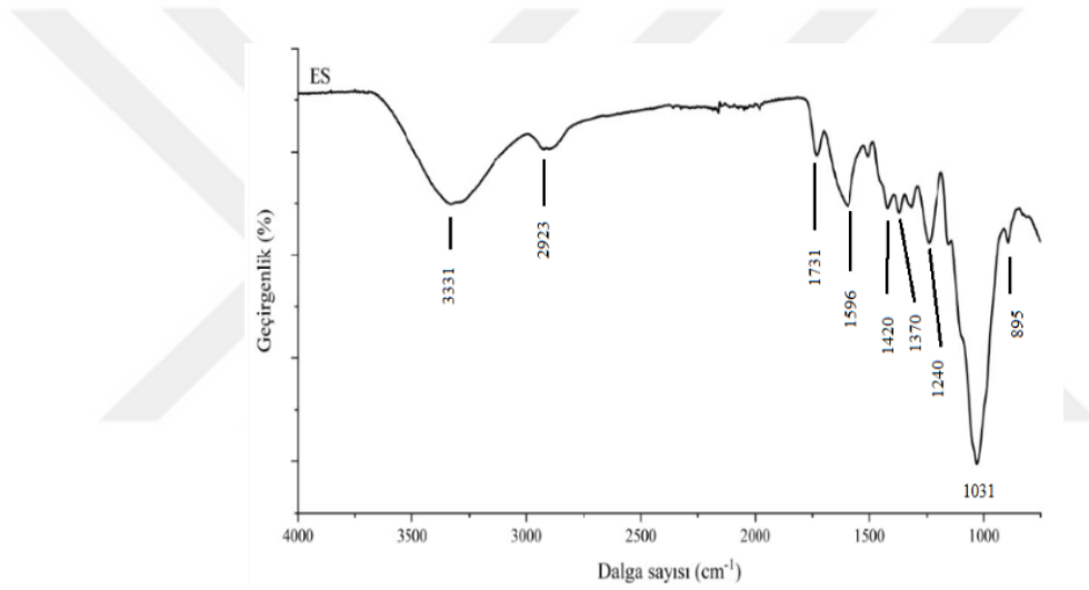
Şekil 3.8: ES doğal lifin FTIR Spektrumu
