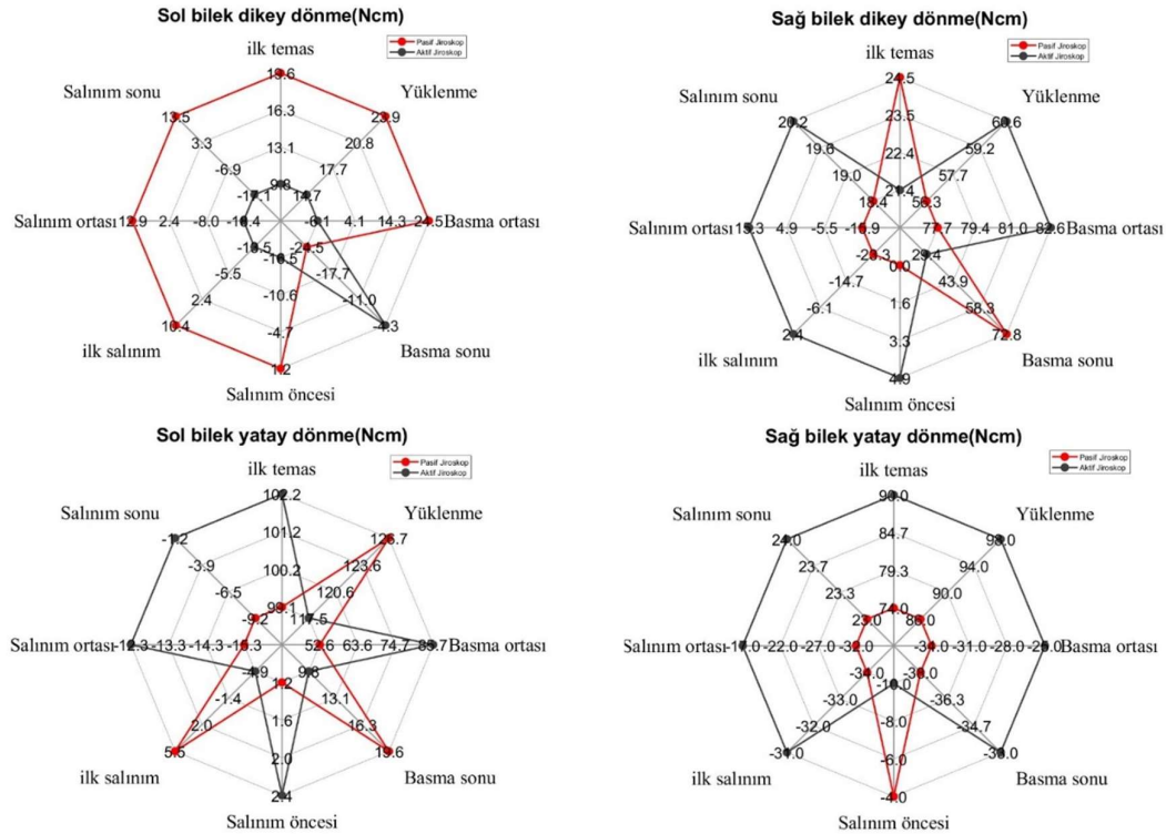
Şekil 4.10. Sağa dönme hareketinde yürüme fazlarına göre motor tork değişimleri.
