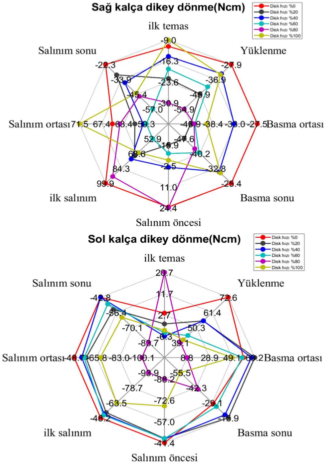
Şekil 4.7. Sağ ve sol kalça dikey dönme hareketine ait tork radar diyagramı.
