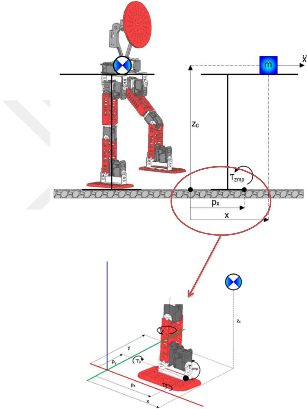
Şekil 3.9. Sıfır moment noktası ve kütle ağırlık merkezi transfer gösterimi.
