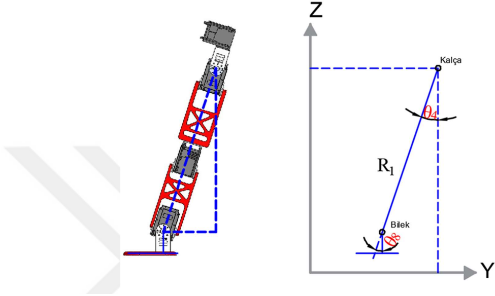
Şekil 3.7. Robot bacağının bilek kalça eklem uzunlukları ve açıları.
