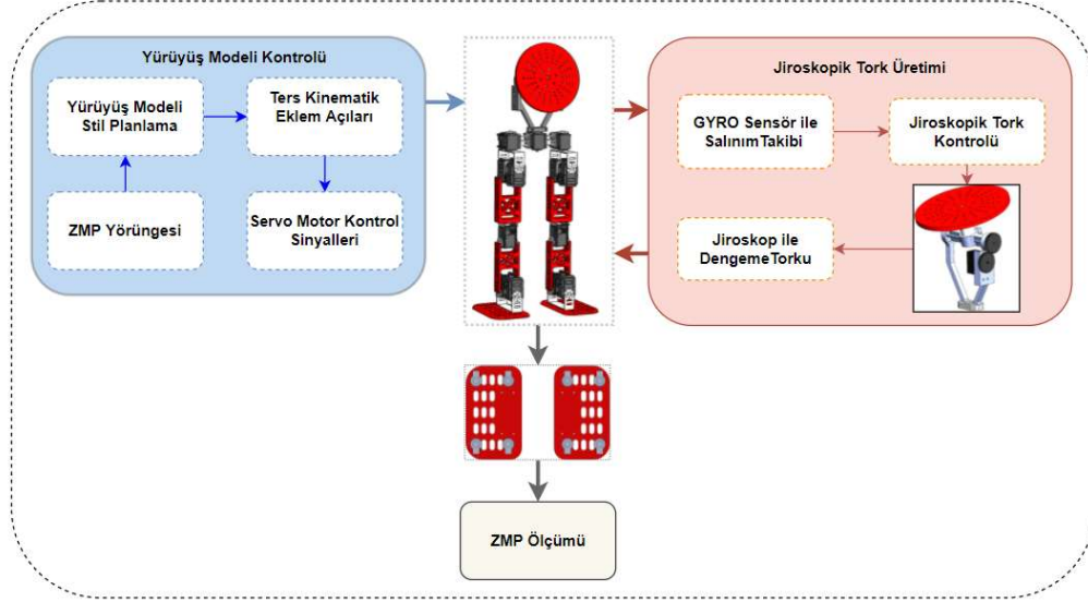
Şekil 3.22. İki ayaklı robotun jiroskop mekanizması ile kontrollü blok diyagramı.
