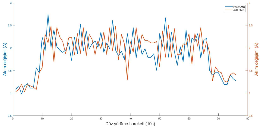
Şekil 4.16. İki ayaklı robotun akım değişimleri
