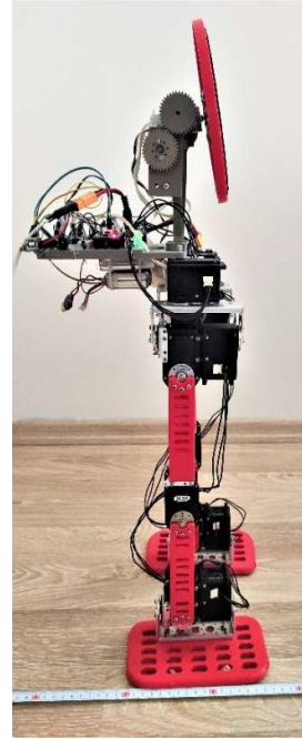
Şekil 3.3. Jiroskop mekanizmalı iki ayaklı robot tasarımı ve boyutları.
