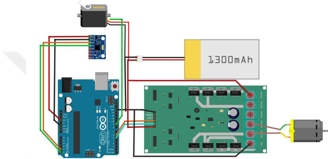
Şekil 3.25. Kontrol edilebilir momentli jiroskop mekanizması devre şeması.
