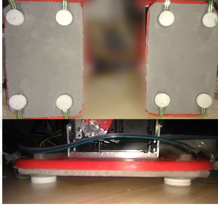
Şekil 3.11. Robot ayak tabanında FSR bağlantıları.
