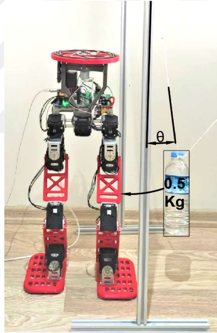
Şekil 4.14. İki ayaklı robotun serbest düşme ile bozucu yük uygulanması.
