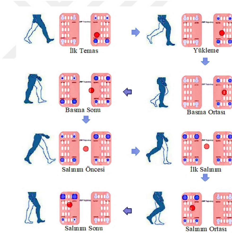
Şekil 3.16. İki ayaklı robotun yürüme fazlarında FSR'ye göre ZMP değişimi simülasyonu.
