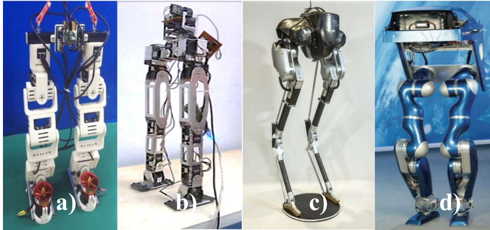
Şekil 3.1. İki ayaklı robot tasarım örnekleri. a) (Liu vd., 2018), b) (Olçay & Özkurt, 2017), c) (Reher vd., 2019), d) (Ott vd., 2011)
