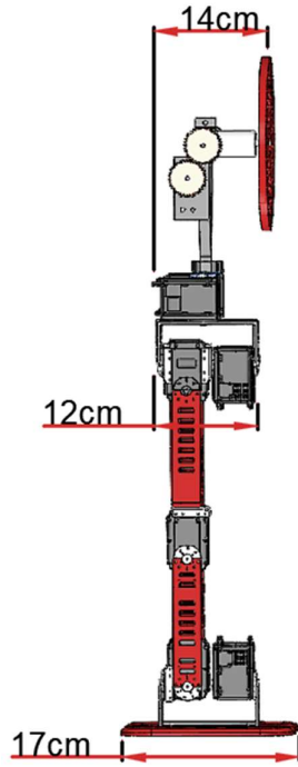
Şekil 3.3. Jiroskop mekanizmalı iki ayaklı robot tasarımı ve boyutları.
