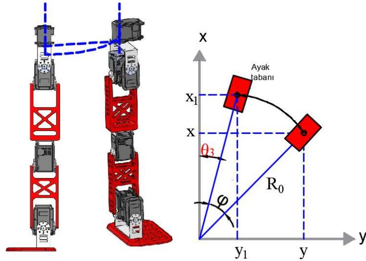
Şekil 3.8. Bacak üst görünüşü eklem uzunlukları ve açıları.
