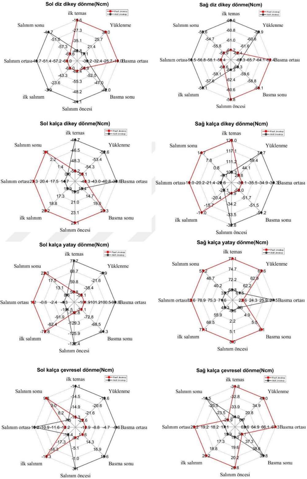
Şekil 4.13. Sola dönme hareketinde yürüme fazlarına göre motor tork değişimleri.
