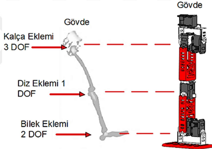
Şekil 3.2. İnsan bacağı eklem yapısı ile tasarlanan iki ayaklı robotun eklem yapısı.
