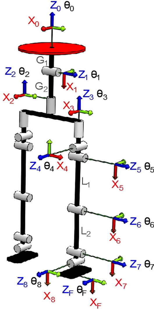
Şekil 3.5. İki ayaklı robot 3 boyutlu modeli ve serbestlik dereceleri.
