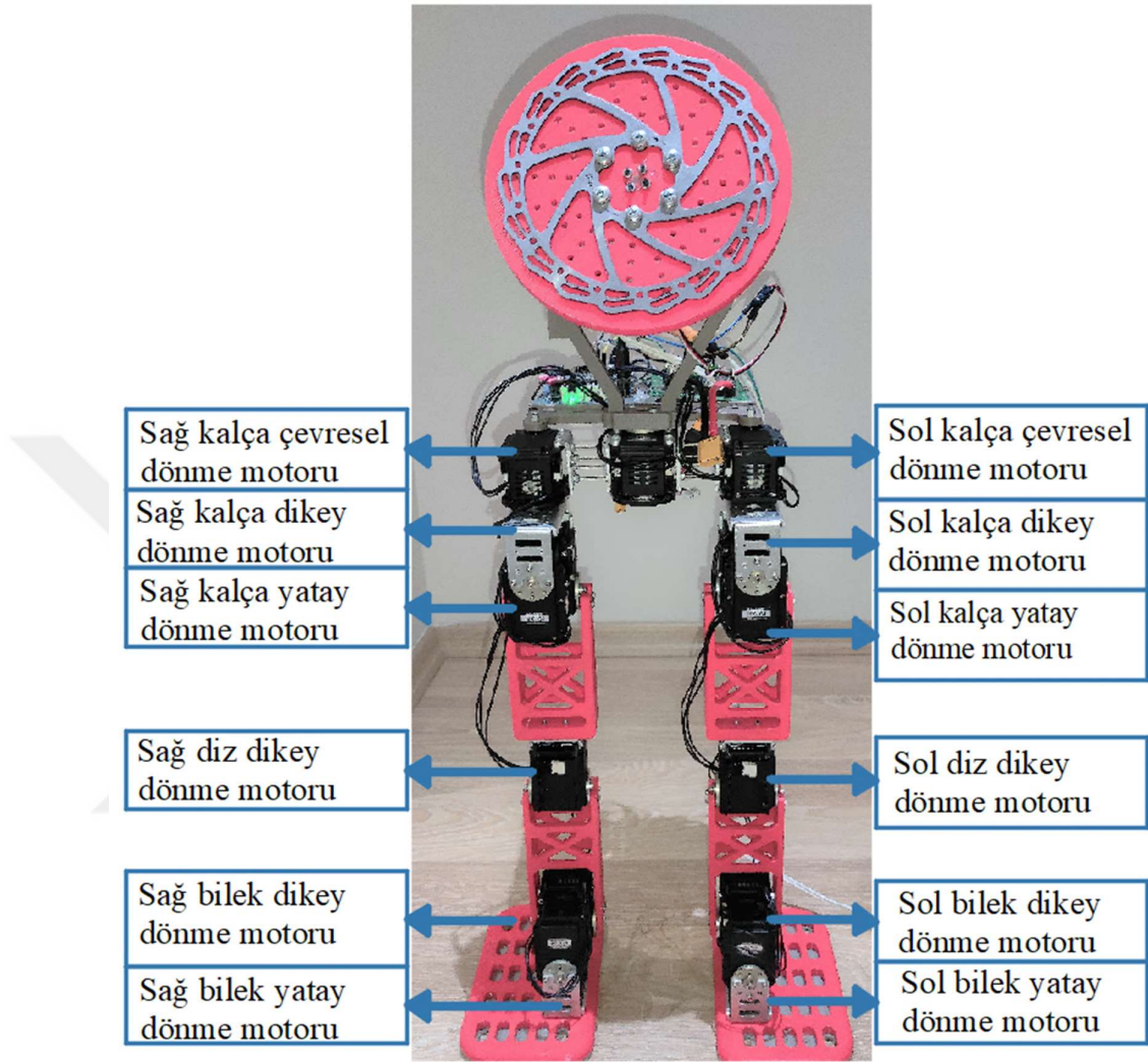
Şekil 3.24. İki ayaklı robotun eklem motor tanımları.
