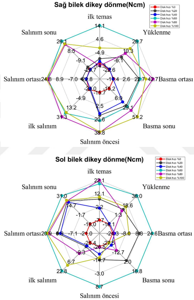
Şekil 4.4. Sağ ve sol bileklerin dikey dönme hareketine ait tork radar diyagramı.
