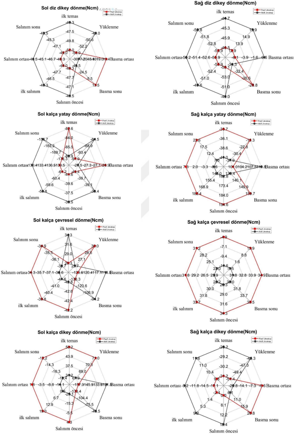
Şekil 4.11. Sağa dönme hareketinde yürüme fazlarına göre motor tork değişimleri.
