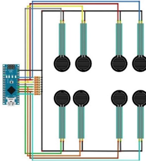
Şekil 3.12. FSR Arduino nano devre şeması.
