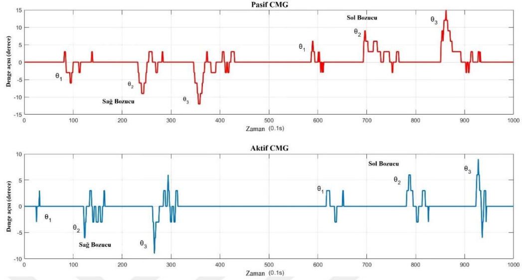
Şekil 4.15. Jiroskoplu iki ayaklı robotun serbest düşme ile bozucu yük uygulanması.
