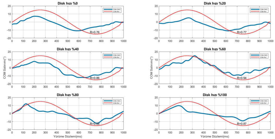
Şekil 4.1. Jiroskopik tork etkisi ile COM salınımları değişimi.
