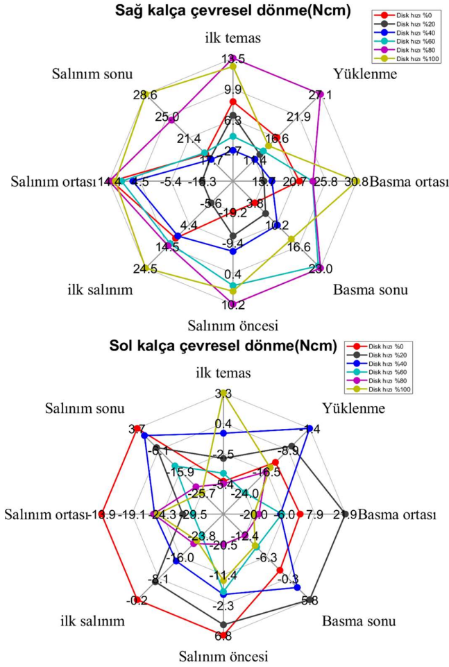
Şekil 4.9. Sağ ve sol kalça çevresel dönme hareketine ait tork radar diyagramı.
