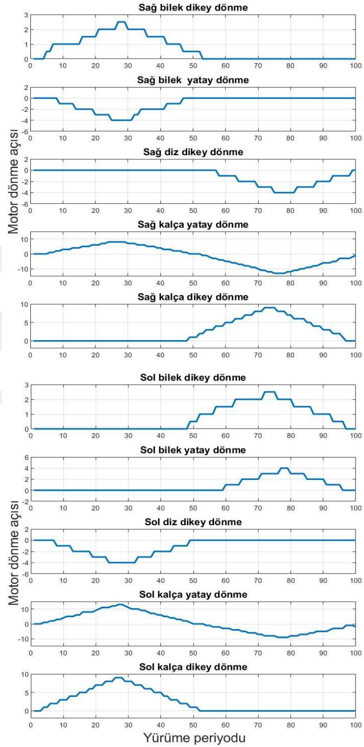
Şekil 3.23. Bir adıma ait düz yürüme eklem açısı değişimleri.
