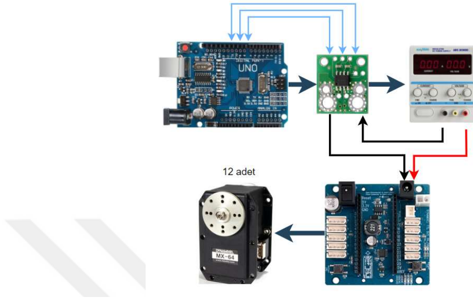
Şekil 4.17. Pololu ACS711EX akım sensör ve bağlantı blok şeması
