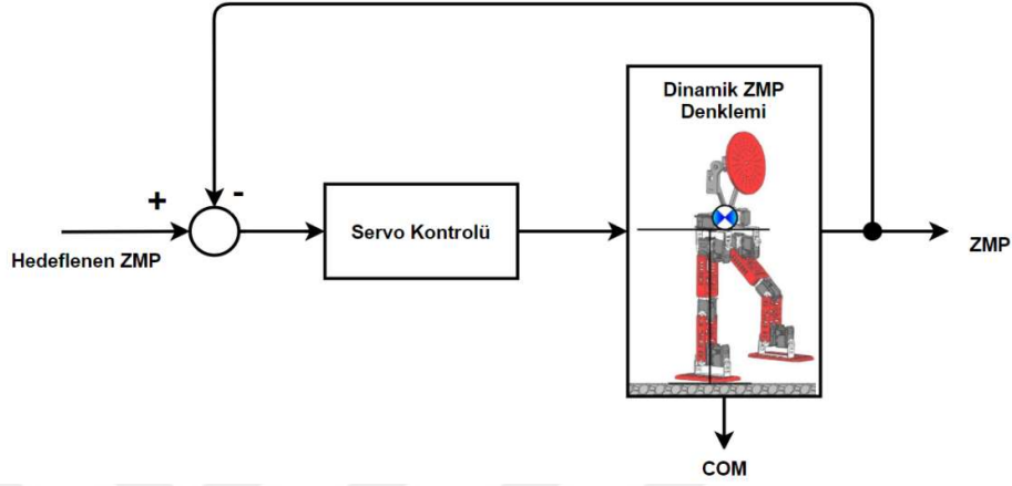
Şekil 3.10. ZMP ve COM kontrol bloğu.
