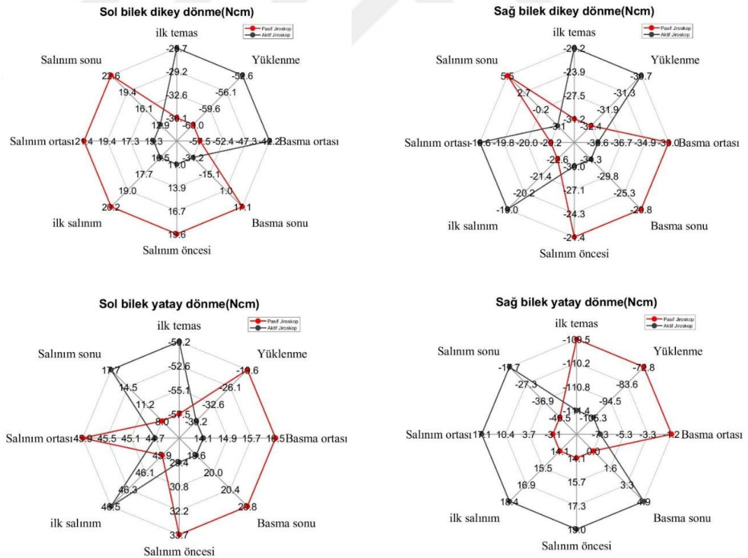
Şekil 4.12. Sola dönme hareketinde yürüme fazlarına göre motor tork değişimleri.
