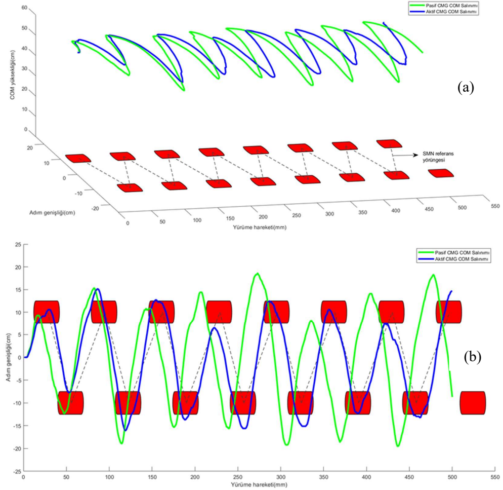
Şekil 4.2. Jiroskop etkisinin yürüme hareketi salınımları üzerindeki etkisi.
