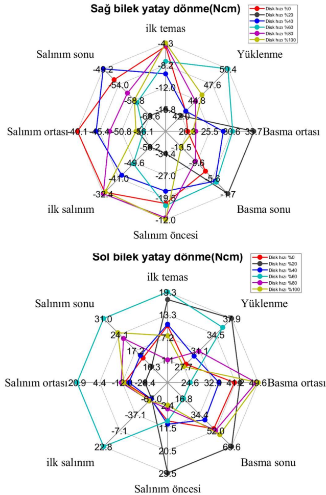
Şekil 4.5. Sağ ve sol bileklerin yatay dönme hareketine ait tork radar diyagramı.
