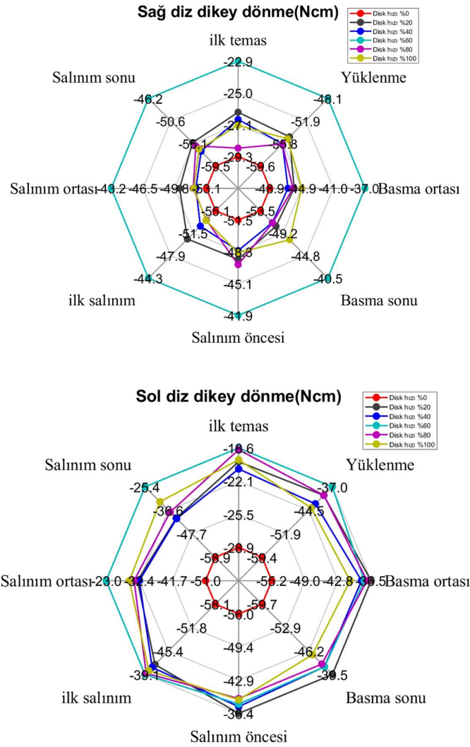
Şekil 4.6. Sağ ve sol diz dikey dönme hareketine ait tork radar diyagramı.
