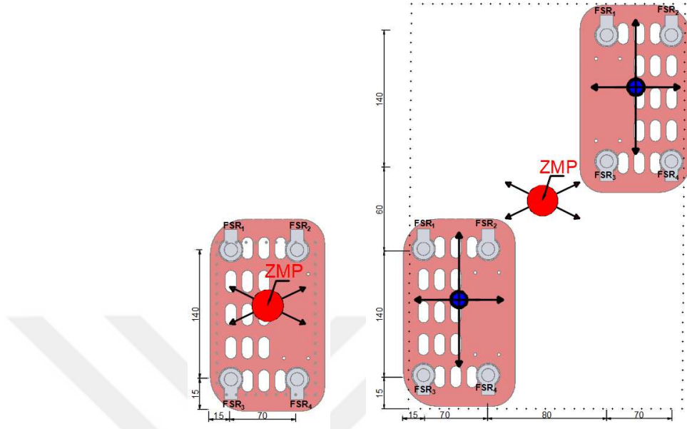
Şekil 3.13. Robot ayak tabanı FSR konumları ve ölçüleri.
