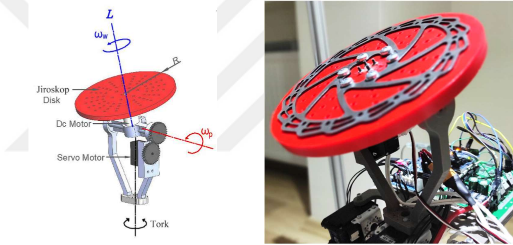
Şekil 3.4. Jiroskop mekanizması ve değişkenleri.
