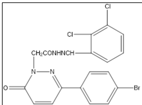
Şekil 4.6. 6-(4-Bromofenil) -3(2H)-piridazinon-2-asetil-2-(2,4-diklorofenilbenzal) hidrazon IVf
