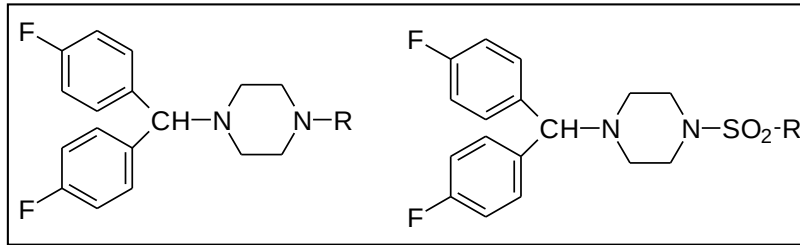
Şekil 1.8. 1-[Bis(4-florofenil) metil] piperazin türevi antibakteriyal bileşikler
