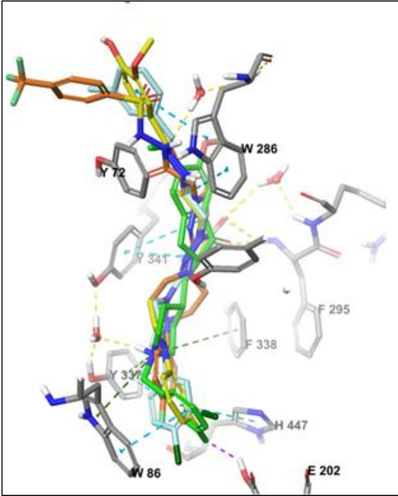
Şekil 2.37. Donazepilın AChE enziminin aktif bölgesi ile etkileşiminin moleküler modelleme çalışması ile gösterimi
