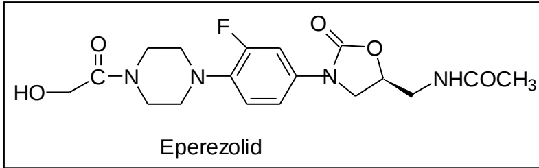
Şekil 1.6. Eperozolid yapısı
