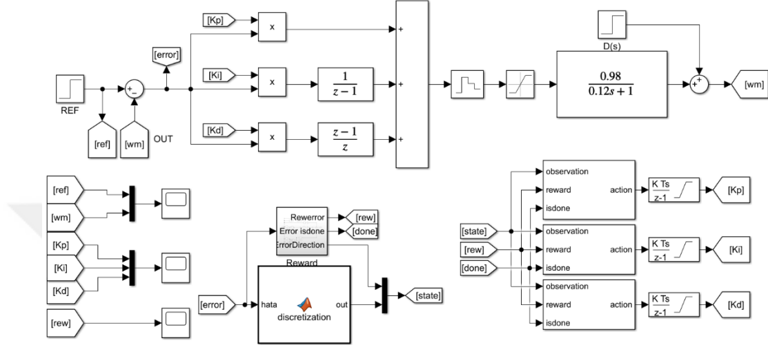
Şekil 3.11. Üç Ajanlı Çalışma Benzetimi
