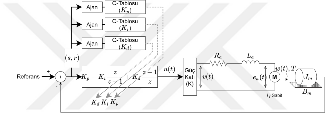
Şekil 3.3. Üç Ajanlı Q-Öğrenme Tabanlı PID
