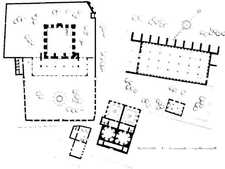
Plan 1. İzmir Pertev Paşa Külliyesi vaziyet planı (Vakıflar Genel Müdürlüğü)
