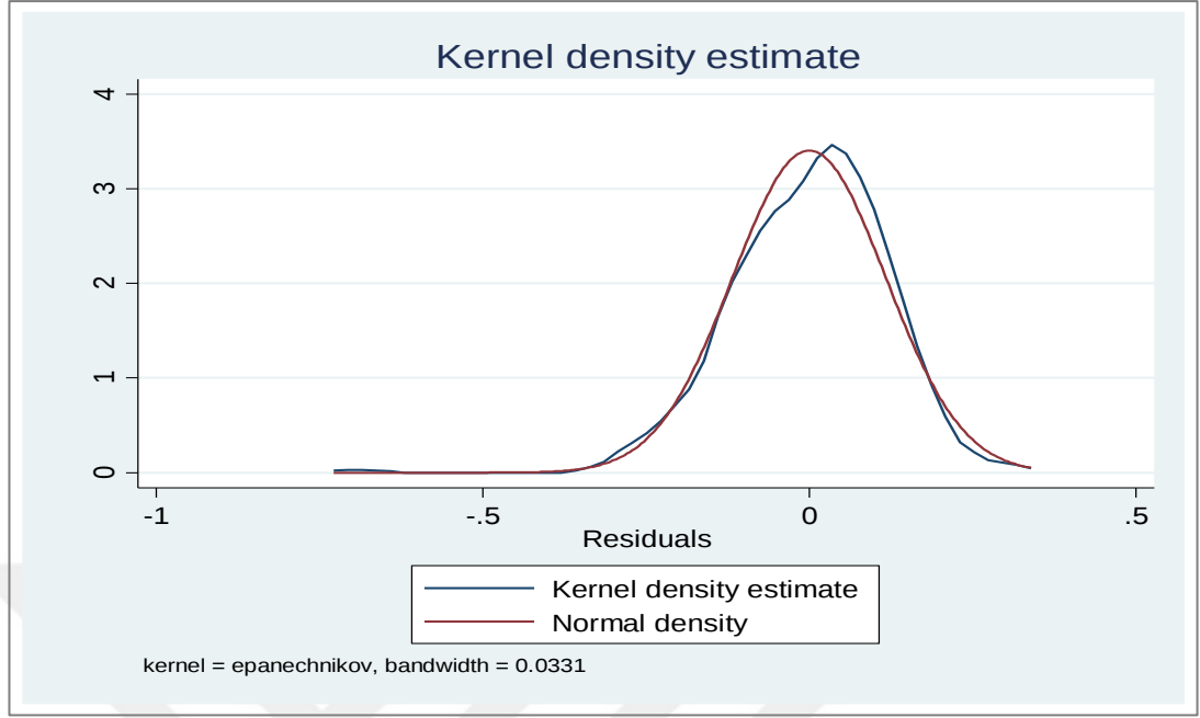
Şekil 2: Normal Dağılımın Şekli
