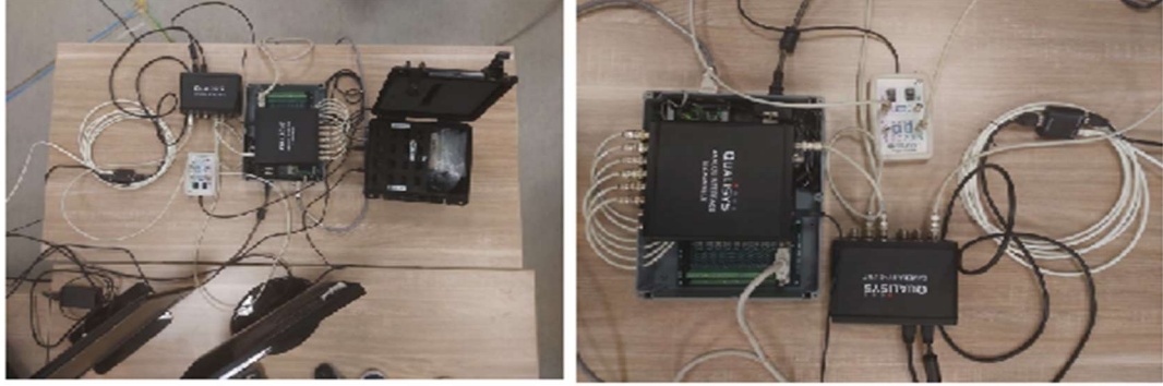
Resim 3.10. Qualisys kamera senkronizasyon ünitesi.
