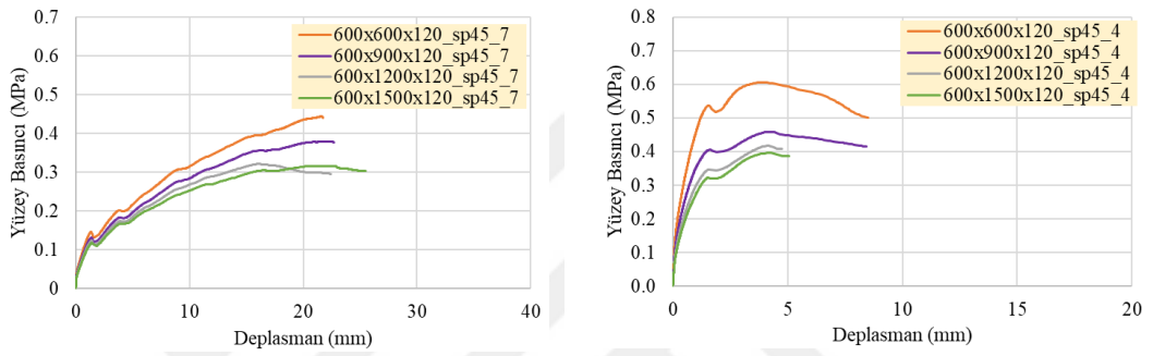
Şekil 4.113: En boy oranının 2 farklı sınır koşuluna etkisi
