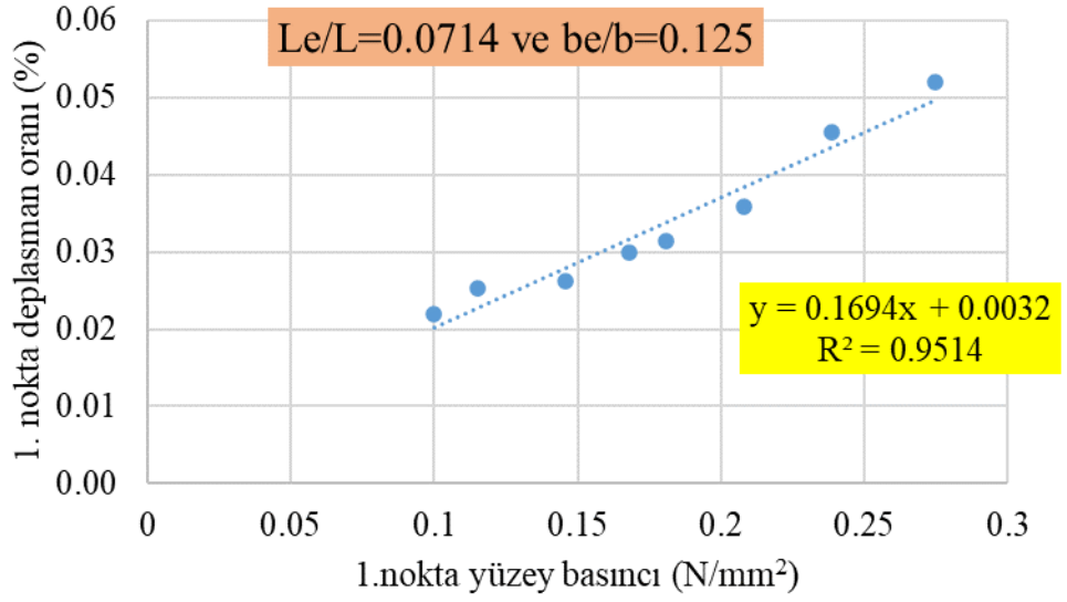
Şekil 5.41: L_e/L = 0.0714 ve b_e/b = 0.125 için 1 noktadaki deplasman oranı-yüzey basıncı ilişkisi (Şekil 35'in alt grupları)
