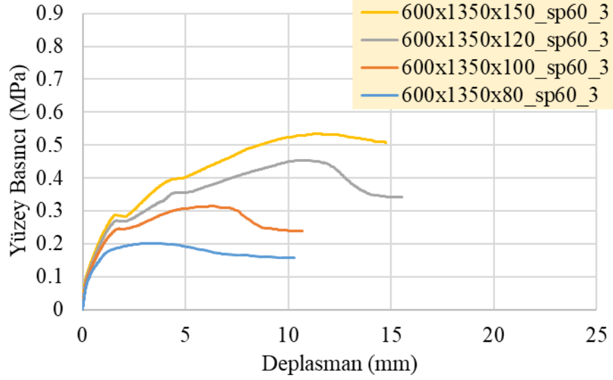
Şekil 4.86: SP60 malzemeden oluşan ve 3 numaralı sınır şartına sahip 600x1350 mm panellerin her bir kalınlık için yüzey basıncı deplasman ilişkisi
