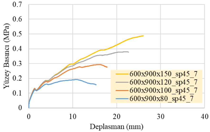
Şekil 4.58: SP45 malzemedan oluşarı ve 7 numaralı sınır şartına sahip 600x900 mm panellerin her bir kalınlık için yüzey basıncı deplasman ilişkisi
