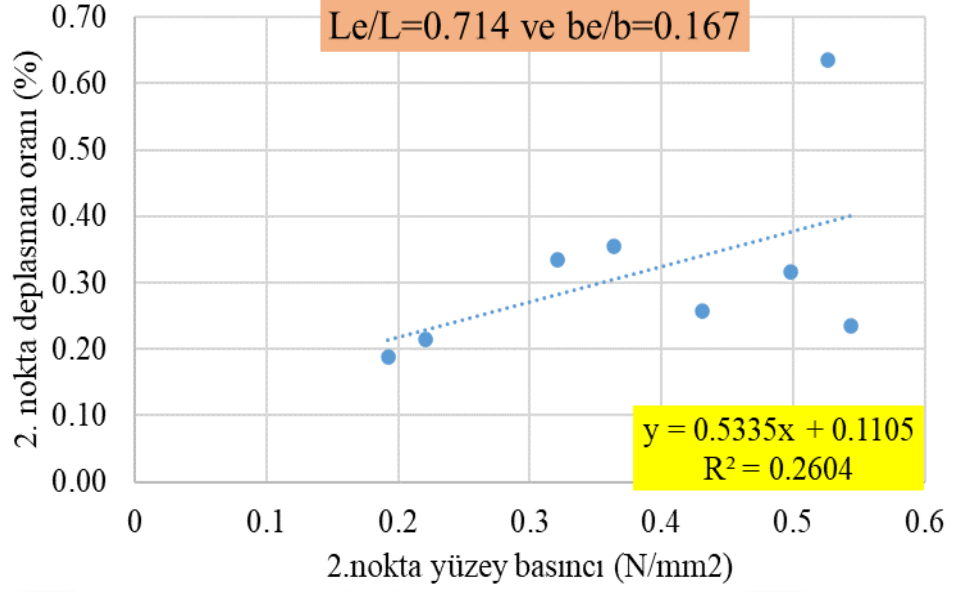
Şekil 5.111: L_e/L=0.0714 ve b_e/b=0.167 için 2. noktadaki deplasman oranı-yüzey basıncı ilişkisi (Şekil 106'nın alt grupları)
