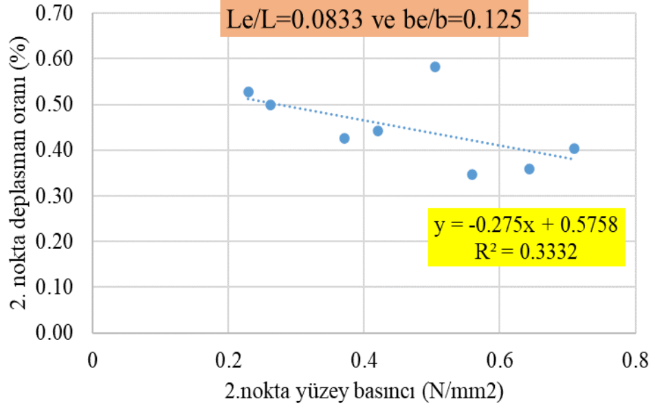
Şekil 5.114: L_e/L=0.083 ve b_e/b=0.125 için 2. noktadaki deplasman oranı-yüzey basıncı ilişkisi (Şekil 110'un alt grupları)
