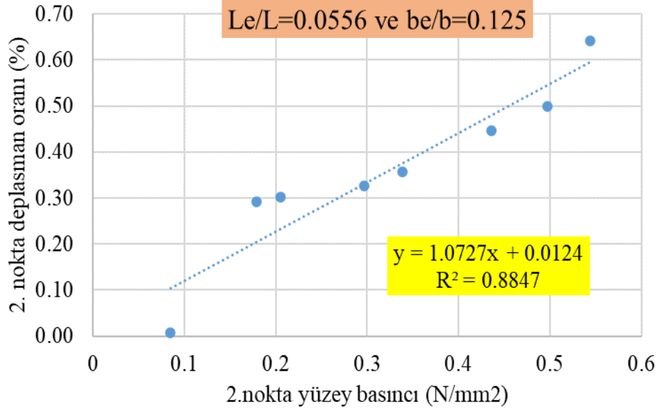
Şekil 5.104: L_e/L=0.056 ve b_e/b=0.125 için 2. noktadaki deplasman oranı-yüzey basıncı ilişkisi (Şekil 100'ün alt grupları)
