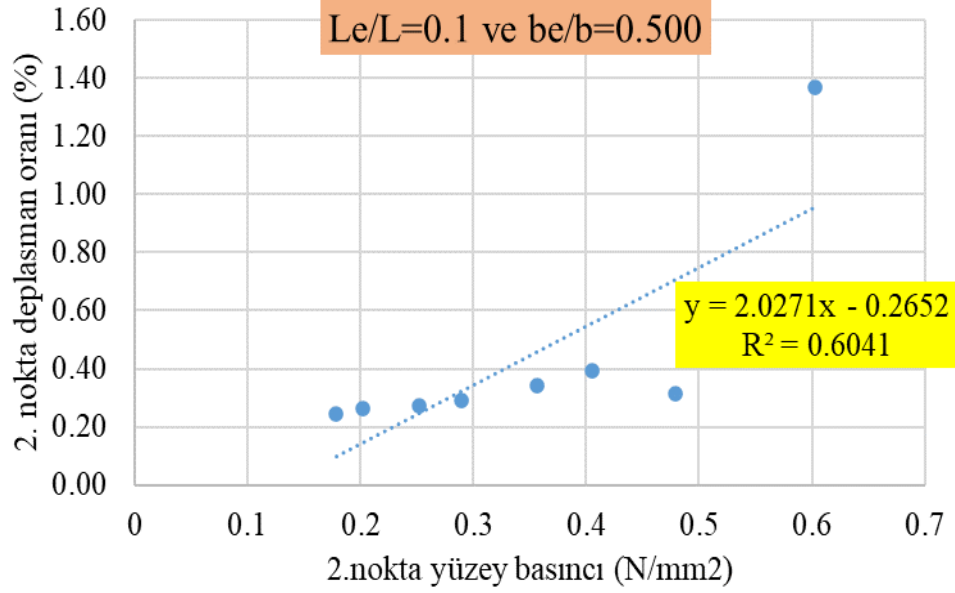
Şekil 5.120: L_e/L=0.1 ve b_e/b=0.500 için 2. noktadaki deplasman oranı-yüzey basıncı ilişkisi (Şekil 113'ün alt grupları)
