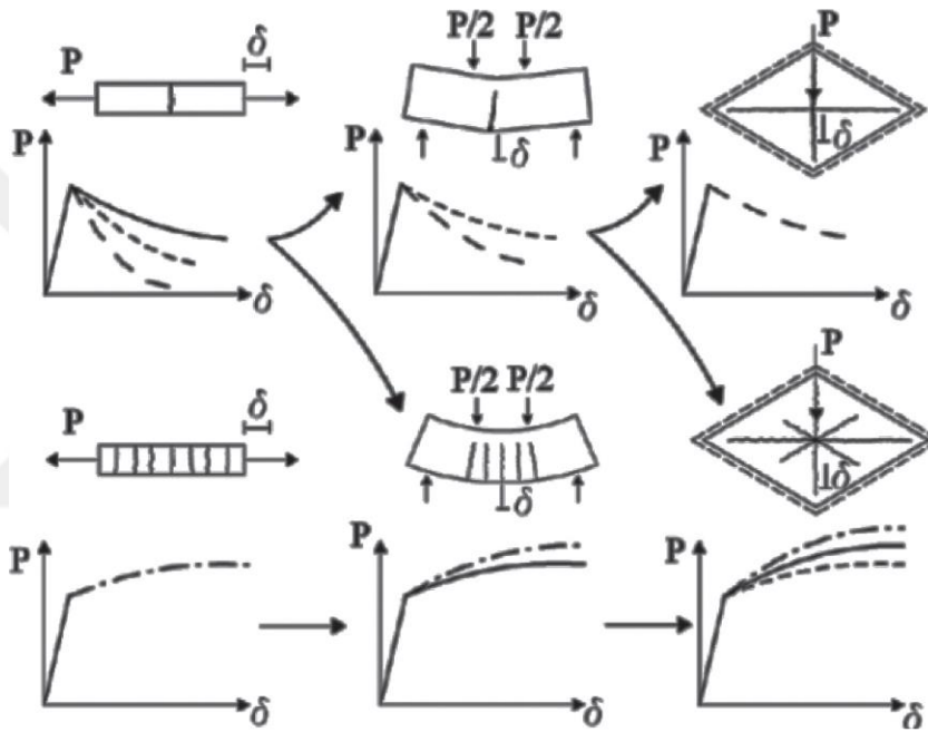
Şekil 2.16: Gerilim, eğilme ve bir sistem altındaki FRC'de gerilim yumuşatma ve gerilim sertleşme şemaları (Model Kodu 2010 [fib 2013]). İlk üçü gerilim yumuşatma davranışını gösterir; alttaki üç gerilim sertleşmesi tepkisini gösterir
