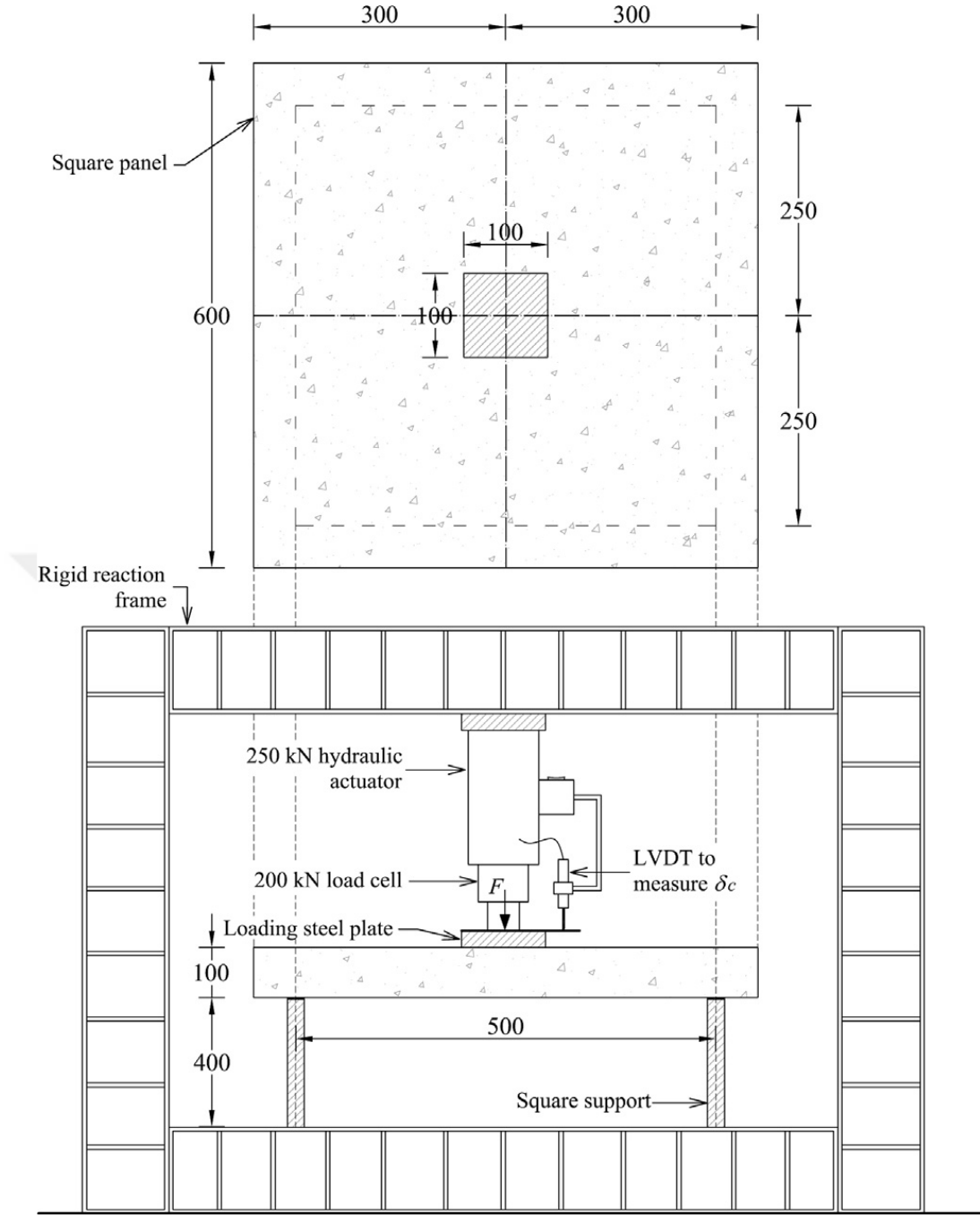
Şekil 4.20: Test düzeneği
