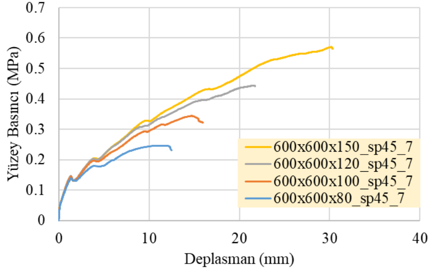
Şekil 4.57: SP45 malzemedan oluşarı ve 7 numaralı sınır şartına sahip 600x600 mm panellerin her bir kalınlık için yüzey basıncı deplasman ilişkisi
