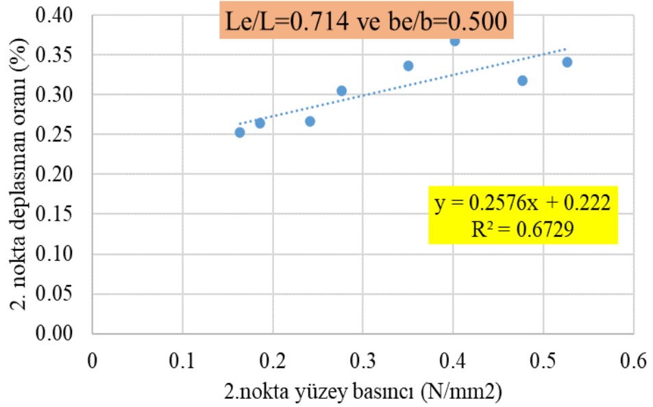
Şekil 5.112: L_e/L=0.0714 ve b_e/b=0.500 için 2.noktadaki deplasman oranı-yüzey basıncı ilişkisi (Şekil 106'nın alt grupları)
