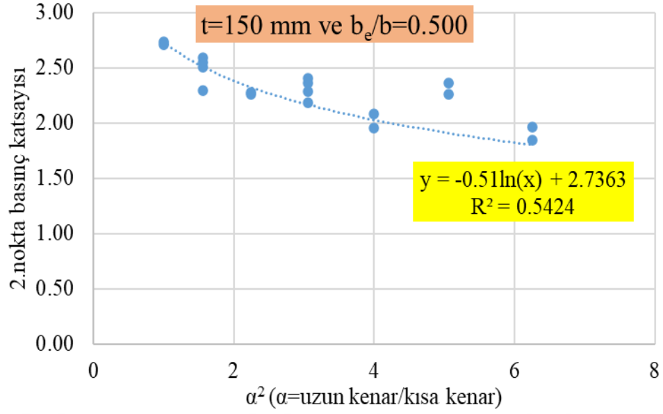
Şekil 5.99: t=150 mm ve b_e/b = 0.500 olan paneller için göçme noktasındaki basınç katsayısının \alpha^2 ile değişimi
