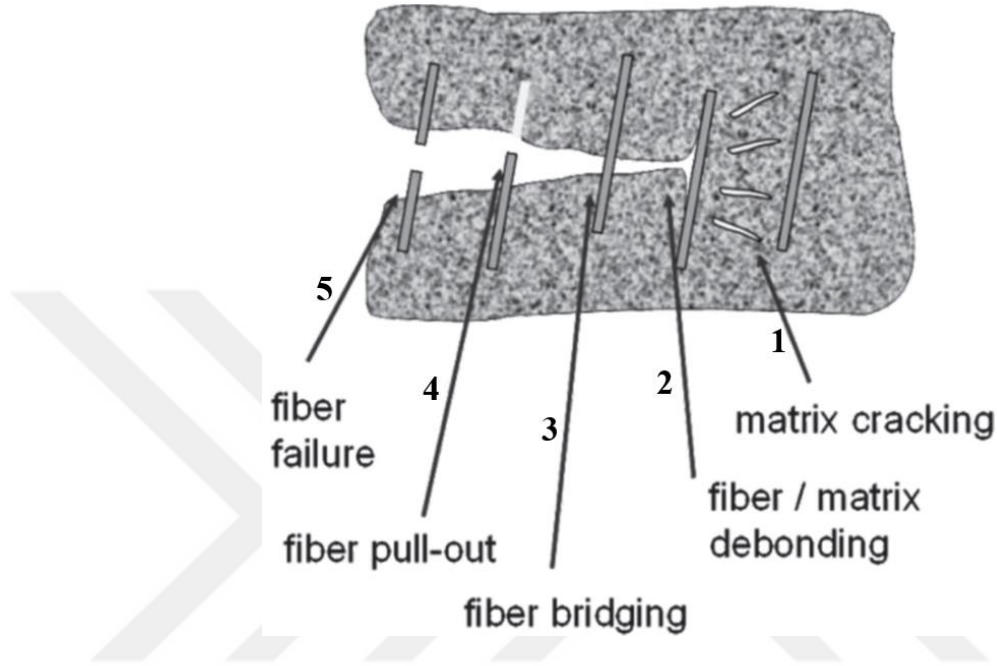
Şekil 2.11: Fiber takviyesinin çalıştığı mekanizmanın şemaları
