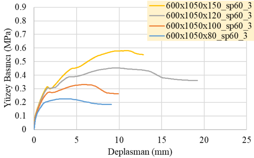
Şekil 4.84: SP60 malzemeden oluşan ve 3 numaralı sınır şartına sahip 600x1050 mm panellerin her bir kalınlık için yüzey basıncı deplasman ilişkisi
