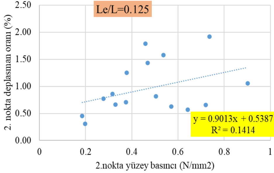
Şekil 5.125: L_e/L=0.125 için 2. noktadaki deplasman oranı-yüzey basıncı ilişkisi
