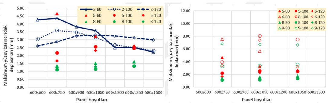
Şekil 4.110: Nihai taşıma kapasitesinde gözlenen orta açıklık sehmindeki değişim
