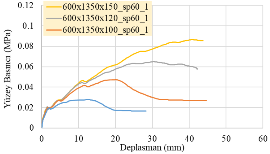
Şekil 4.72: SP60 malzemeden oluşan ve 1 numaralı sınır şartına sahip 600x1350 mm panellerin her bir kalınlık için yüzey basıncı deplasman ilişkisi
