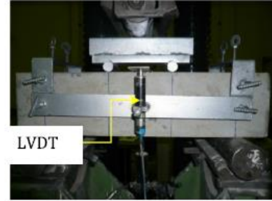
Şekil 4.4: Betonun mekanik özellikleri için test düzeneği
