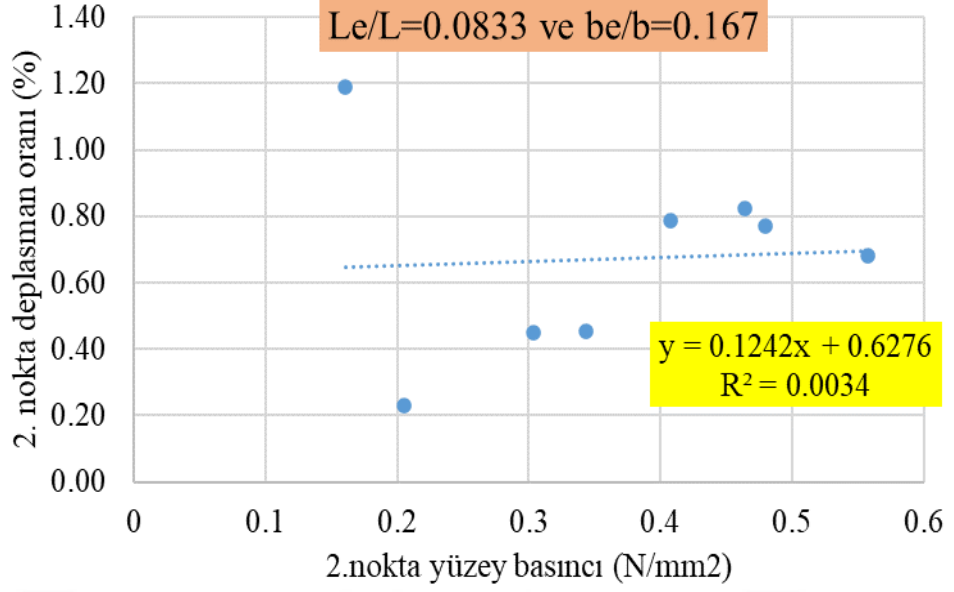
Şekil 5.115: L_e/L=0.0833 ve b_e/b=0.167 için 2. noktadaki deplasman oranı-yüzey basıncı ilişkisi (Şekil 110'un alt grupları)
