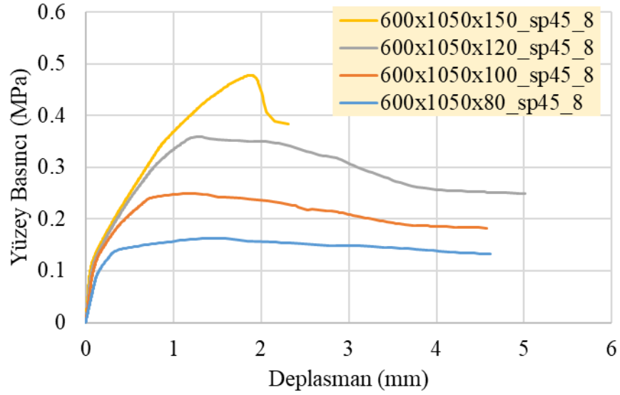
Şekil 4.62: SP45 malzemedan oluşan ve 8 numaralı sınır şartına sahip 600x1050 mm panellerin her bir kalınlık için yüzey basıncı deplasman ilişkisi
