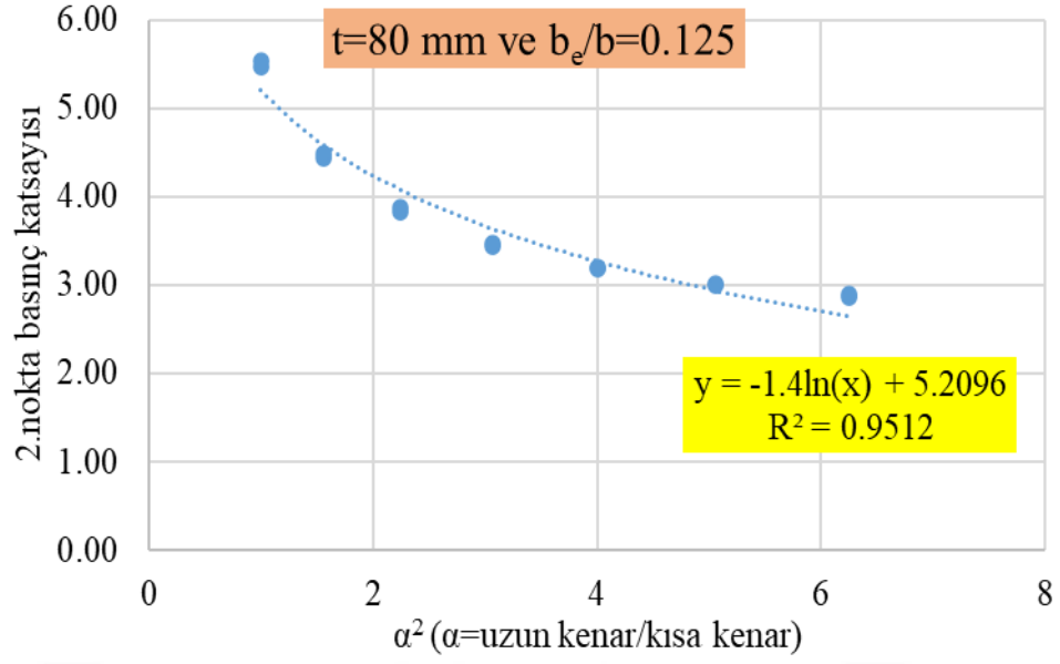
Şekil 5.81: t=80 mm ve b_e/b = 0.125 olan paneller için geçme noktasındaki basınç katsayısının \alpha^2 ile değişimi
