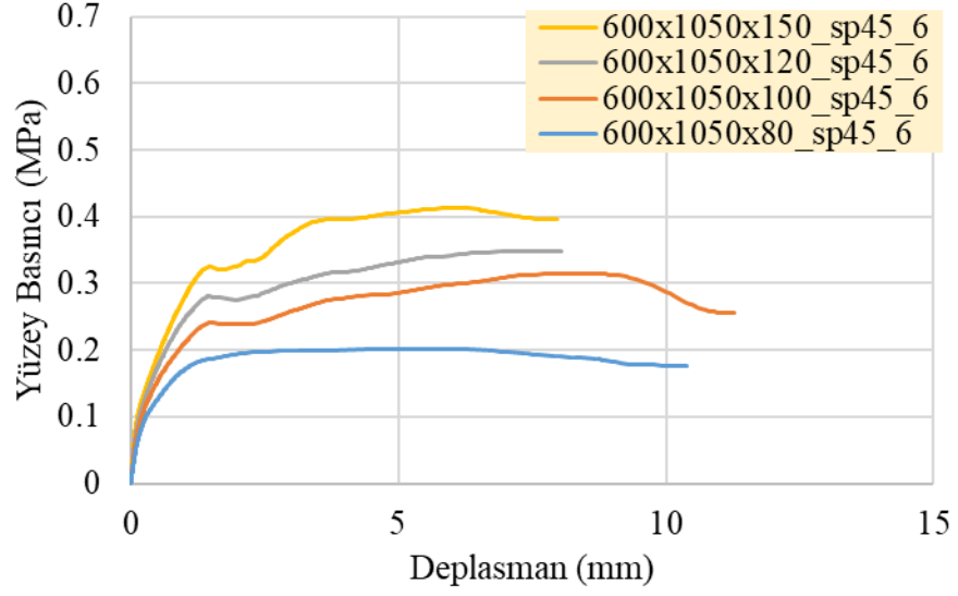
Şekil 4.55: SP45 malzemeden oluşan ve 6 numaralı sınır şartına sahip 600x1050 mm panellerin her bir kalınlık için yüzey basıncı deplasman ilişkisi
