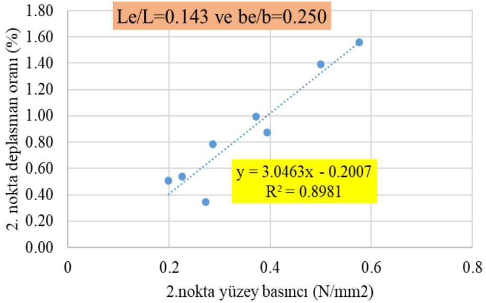
Şekil 5.130: L_e/L=0.143 ve b_e/b=0.250 için 2. noktadaki deplasman oranı-yüzey basıncı ilişkisi (Şekil 127'in alt grupları)
