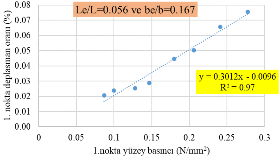
Şekil 5.36: L_e/L = 0.056 ve b_e/b = 0.167 için 1 noktadaki deplasman oranı-yüzey basıncı ilişkisi (Şekil 29'un alt grupları)
