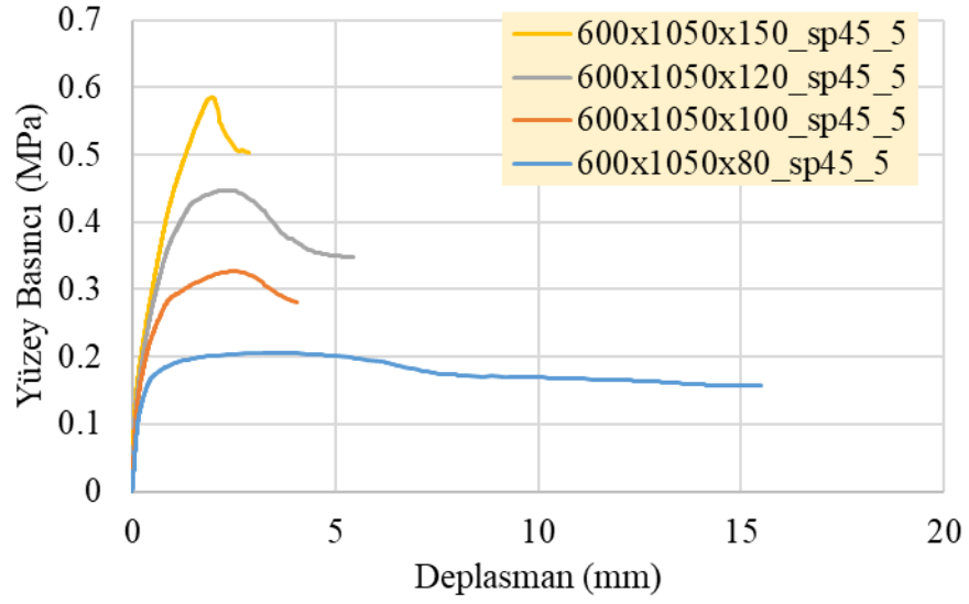
Şekil 4.52: SP45 malzemeden oluşan ve 5 numaralı sınır şartına sahip 600x1050 mm panellerin her bir kalınlık için yüzey basıncı deplasman ilişkisi
