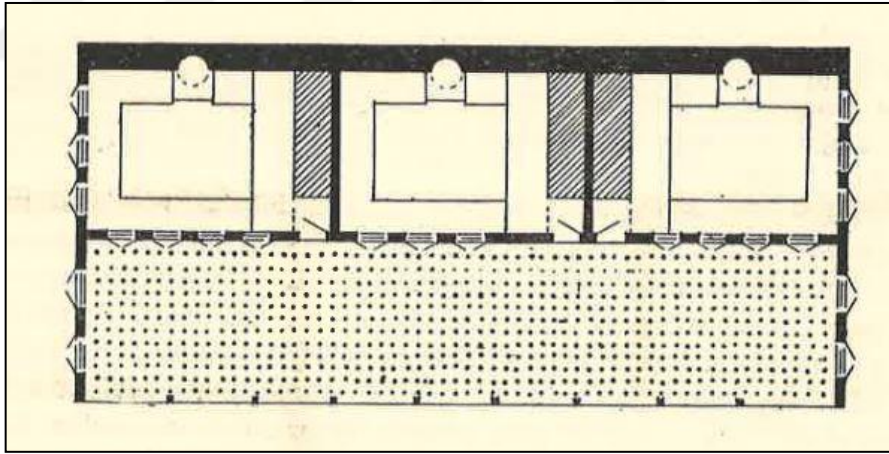
Şekil 60. Sedat Hakkı Eldem- Türk Evi- ideal dış sofalı plan tipi (Eldem, 1954).
