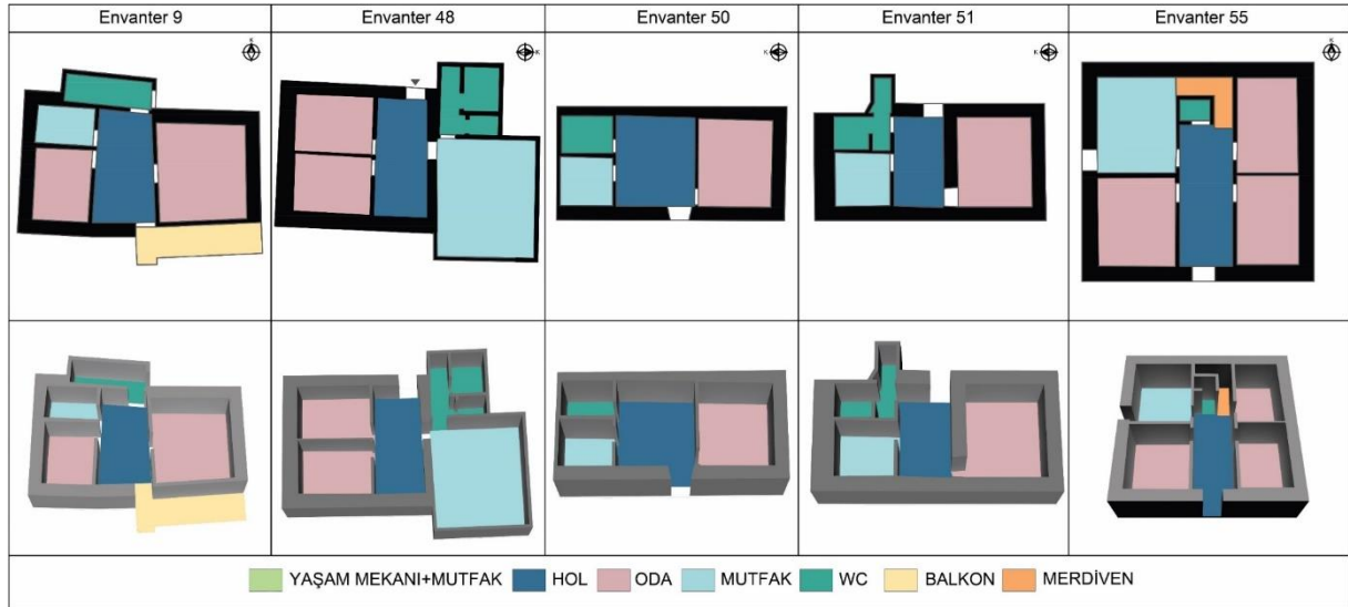
Şekil 63. Sırakonaklar iç sofalı ev tipine uygun ev planları.
