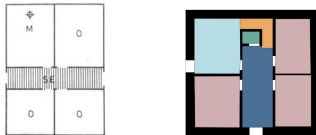
Şekil 64. Sırasıyla, Doğu Karadeniz konutlarındaki basit aşhaneli tip (Sümerkan, 1991), Sırakonaklardaki dış sofalı plan tipine uygun tip.
