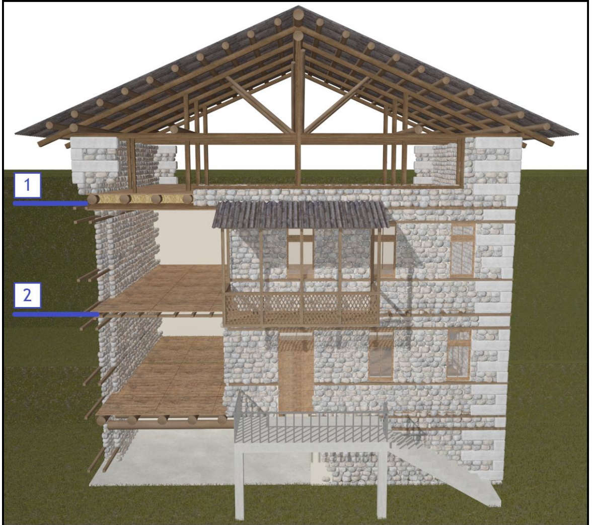
Şekil 119. Yapım sistemi.
