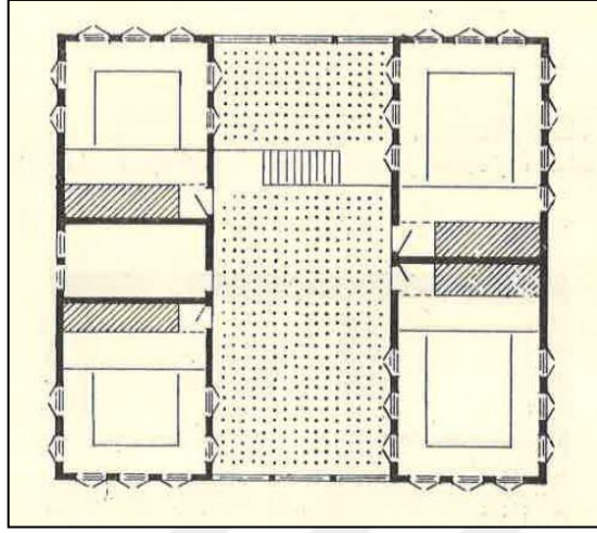
Şekil 62. Sedat Hakkı Eldem- Türk Evi- ideal iç sofalı plan tipi (Eldem, 1954).
