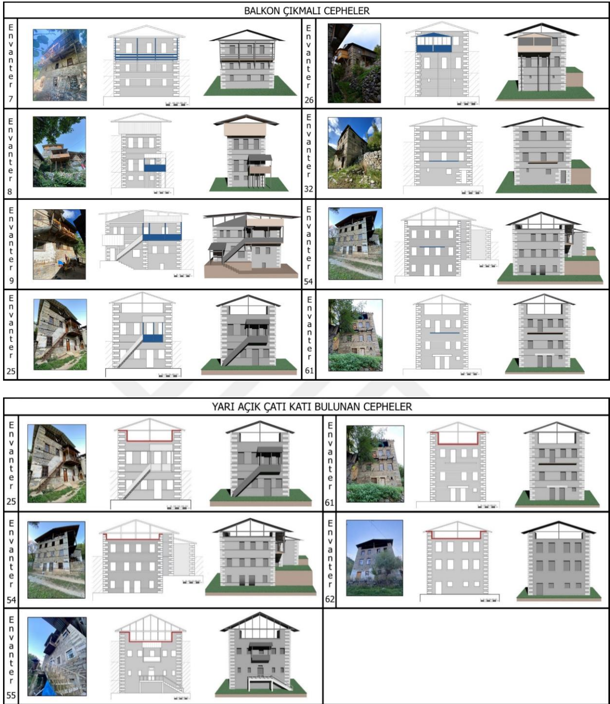
Şekil 95. Cephe tipolojileri (Devamı)
