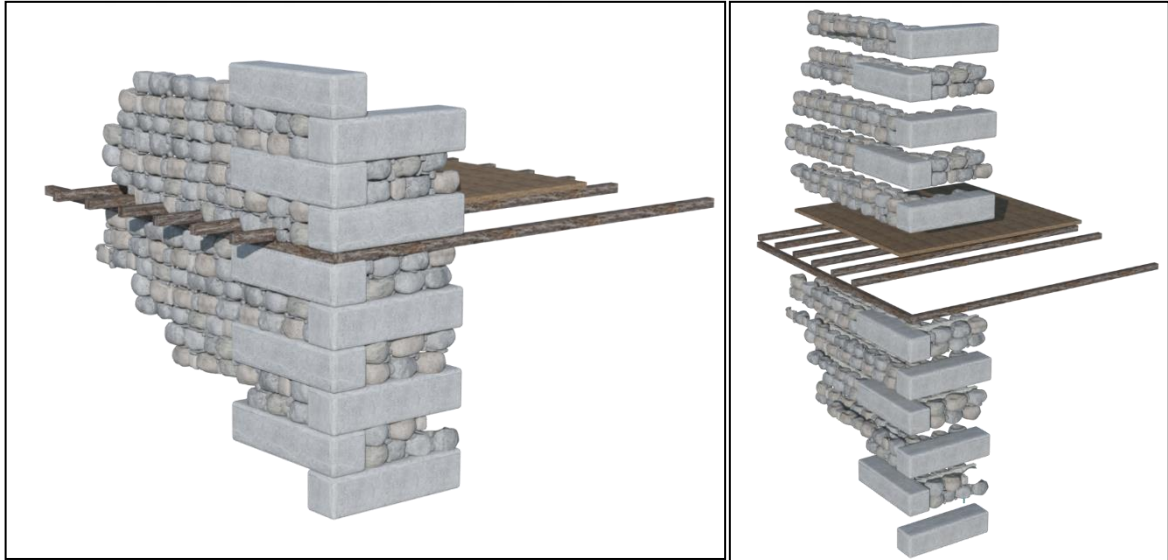
Şekil 115. Duvar sistemi.
