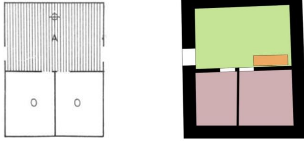
Şekil 64. Sırasıyla, Doğu Karadeniz konutlarındaki basit aşhaneli tip (Sümerkan, 1991), Sırakonaklardaki dış sofalı plan tipine uygun tip.
