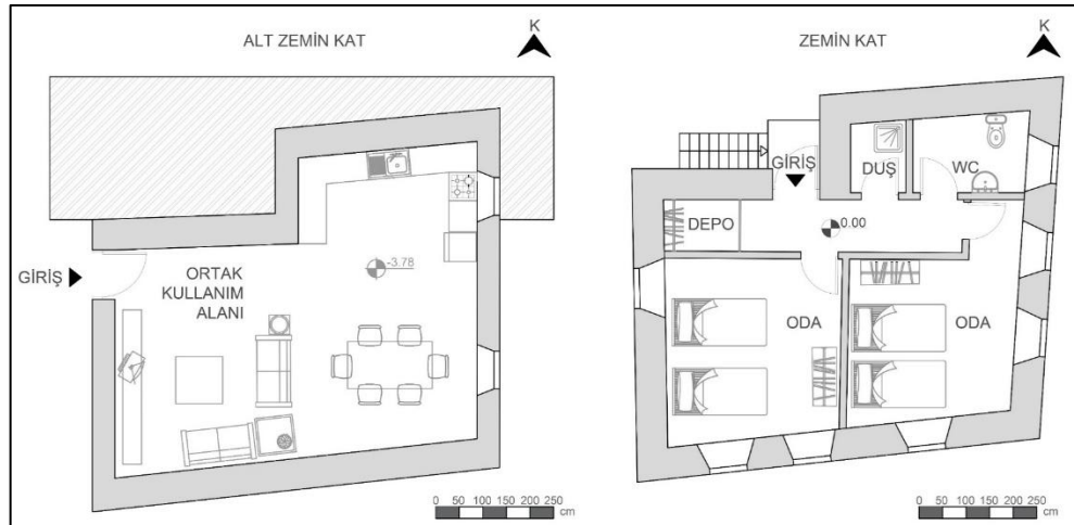
Şekil 133. 52 envanter nolu kullanılmayan yapının pansiyona dönüştürülmesi.
