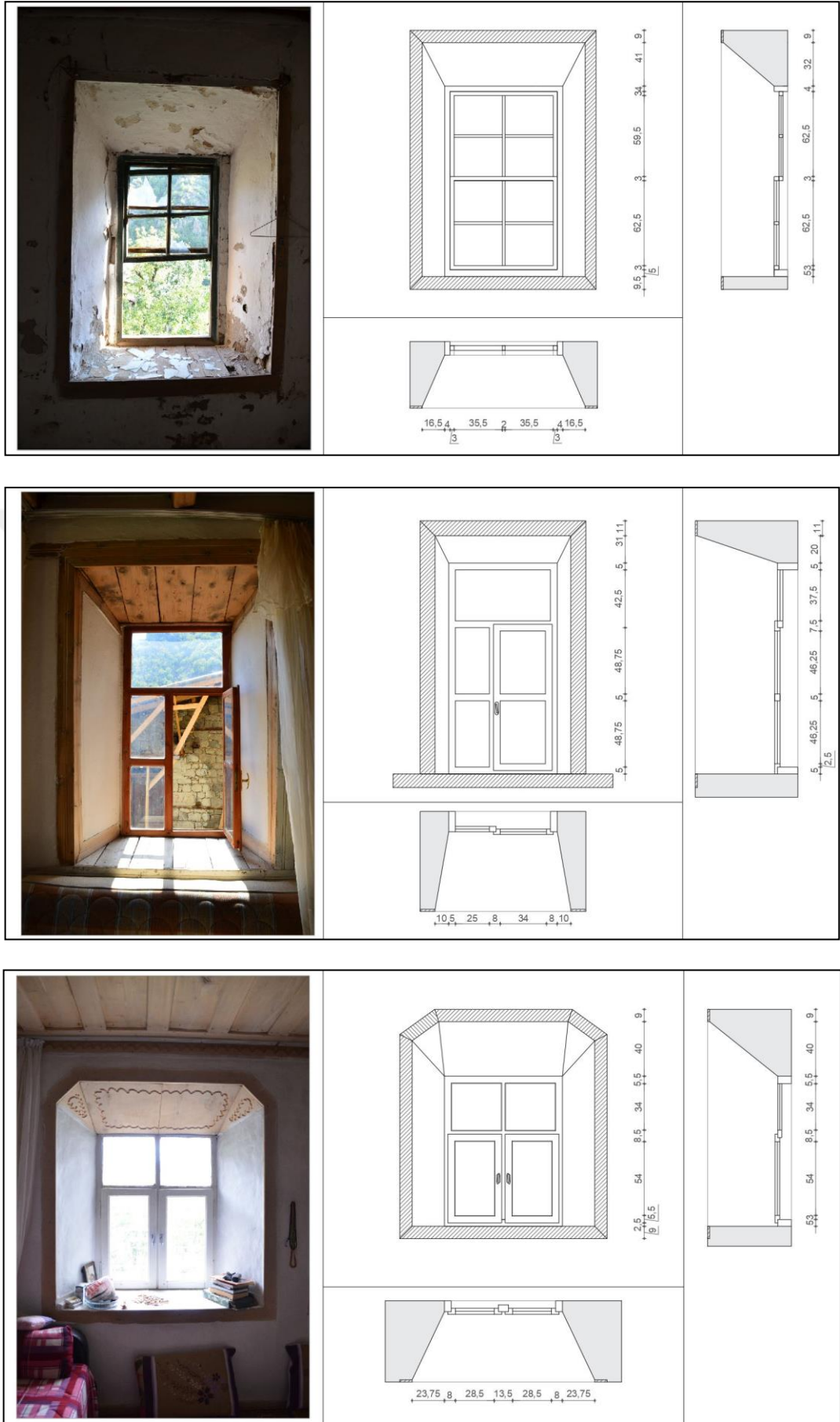
Şekil 103. Çeşitli pencere tipleri (Devamı)
