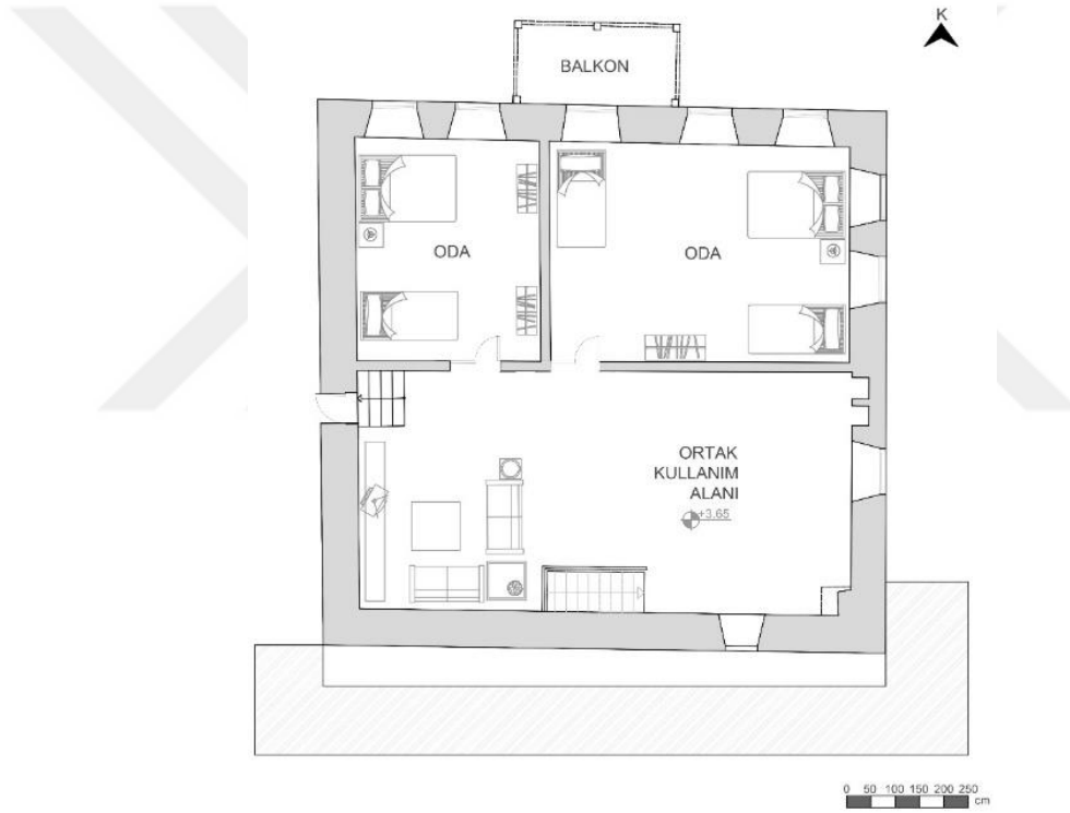
Şekil 134. 55 envanter nolu yapının kullanılmayan birinci katının pansiyona dönüştürülmesi.
