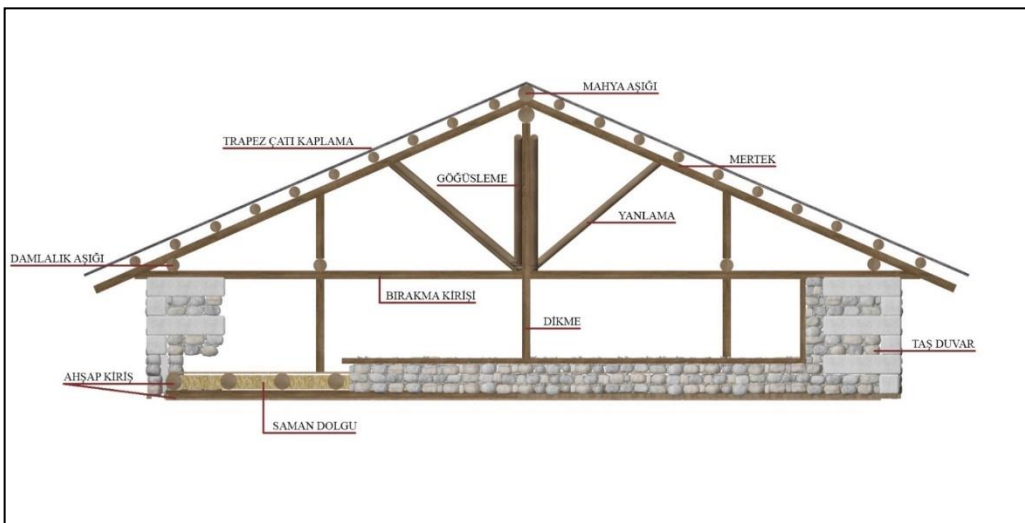
Şekil 122. Çatı sistemi.
