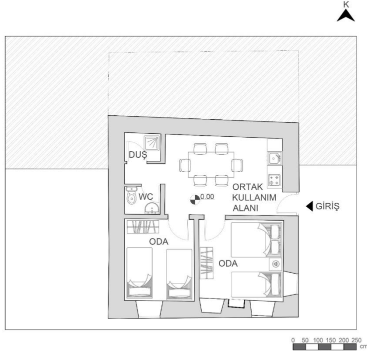
Şekil 132. 26 envanter nolu yapının kullanılmayan zemin katının pansiyona dönüştürülmesi.
