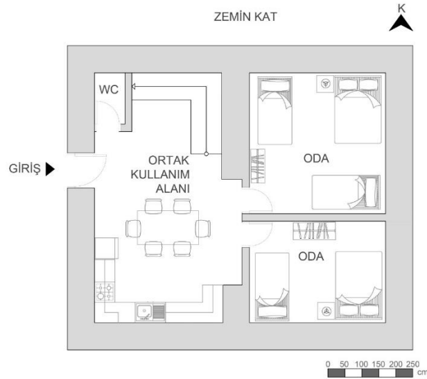
Şekil 135. 65 envanter nolu kullanılmayan yapının pansiyona dönüştürülmesi.
