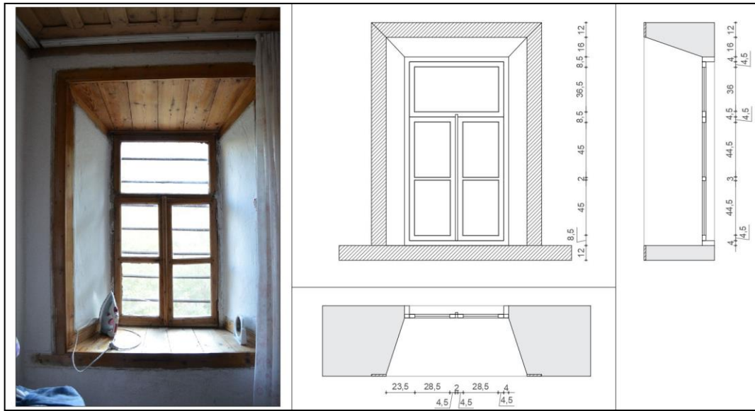
Şekil 103. Çeşitli pencere tipleri.
