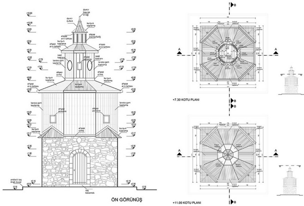
Şekil 5.14. Sivas Saat Kulesi Rölöve Plan ve Görünüş (Sekamimarlık)
