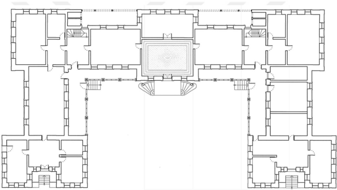
Şekil 5.47. Sivas Sanayi Mektebi Zemin Kat Planı (Bulut, 2006)
