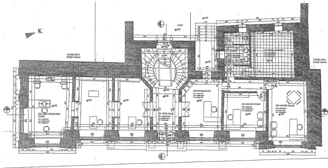
Şekil 5.57. Ziya Bey Yazma Eserler Kütüphanesi Zemin Kat Planı (Bulut, 2006; Bayındırlık Müdürlüğü Arşivi)
