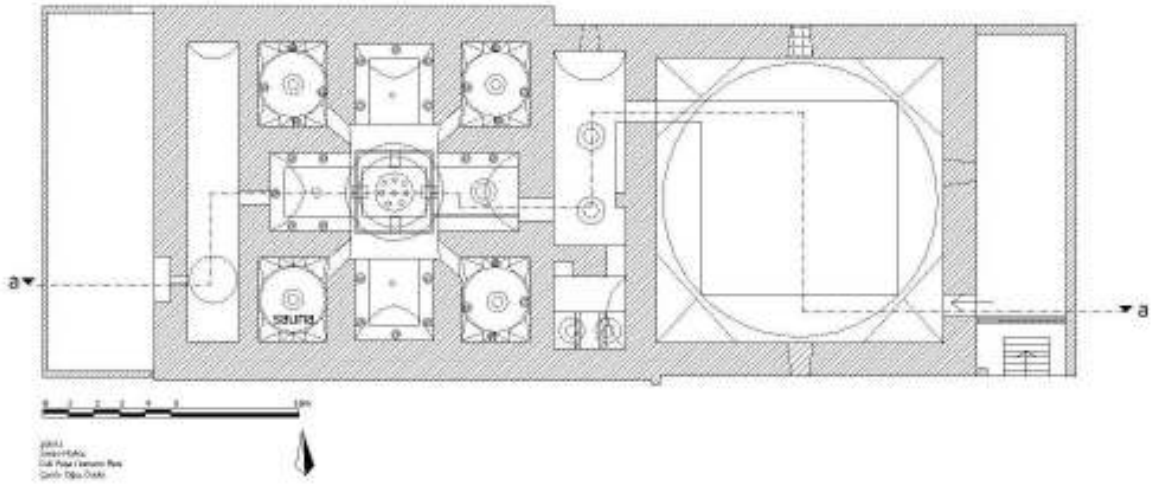
Şekil 5.44. Eski Paşa Hamamı Planı (Önder, 2007)
