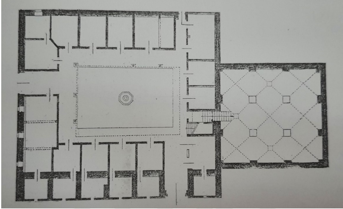
Şekil 4.37. Sivas Subaşı Hanı Planı (Bilget- Denizli, 1998)
