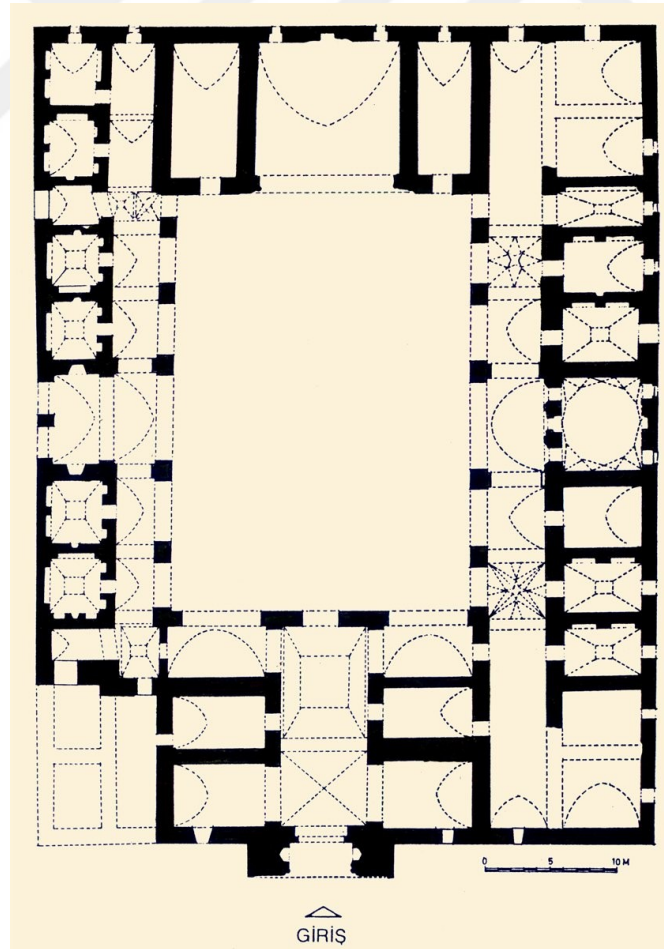
Şekil 3.13. Şifaiye Medresesi (Darüşşifa) Planı (Cantay, 2002)
