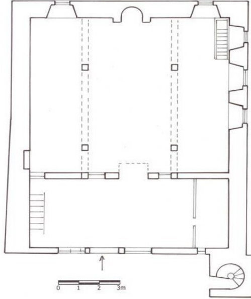
Şekil 4.16. Zincirli Minare Cami Planı (Ünsal, 2006)
