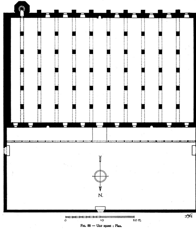
Şekil 3.7. Sivas Ulu Cami Planı (Gabriel Arşivi)
