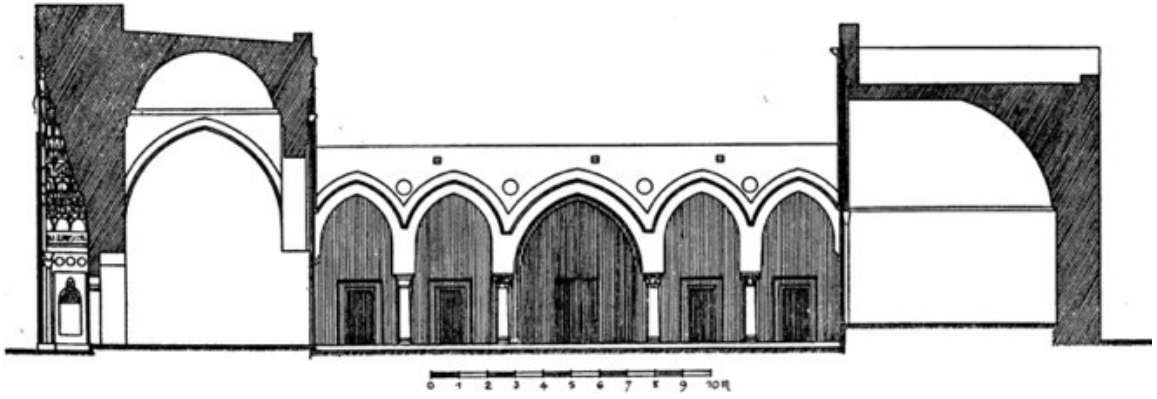
FIG. 97. — MÉDRESSÉ DE MUZAFFER BARUDJIRI : Coupe longitudinale.
