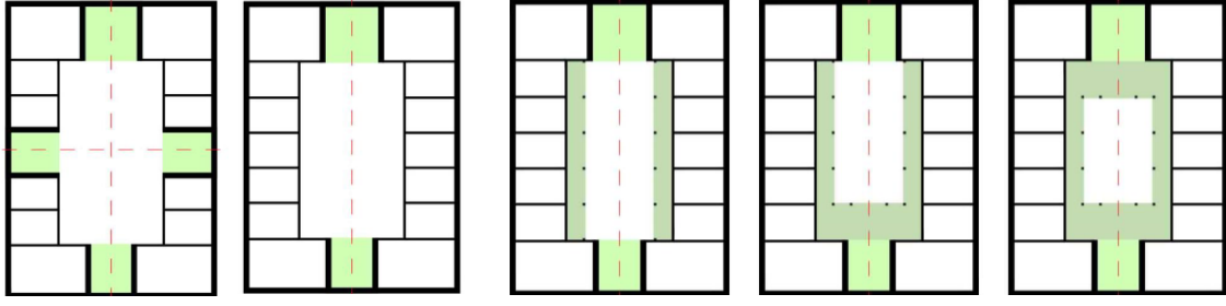
Şekil 3.6. Soldaki İki ve Dört Eyvanlı Plan Tipleri, Sağdaki ise Revak Tipleri Şematik Gösterimi (Meral, 2021)
