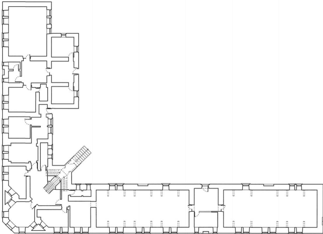
Şekil 5.54. Sivas Jandarma Binası Zemin Kat Planı (Bulut, 2006)
