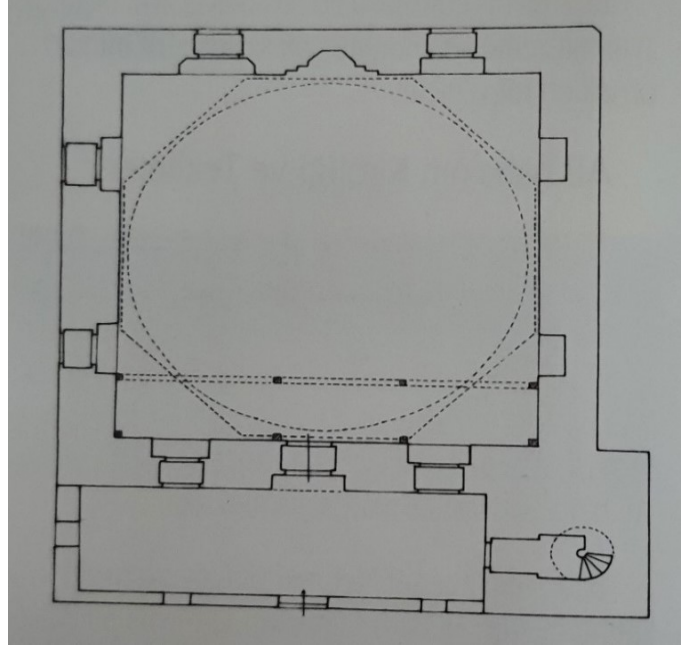
Şekil 4.8. Sivas Kale Cami Planı (Denizli,1998)
