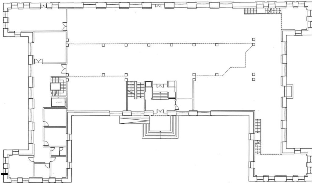
Şekil 5.40. Sivas Sanayi Mektebi Demir Atölyesi Zemin Kat Planı (Bulut, 2006; Bayındırlık Müdürlüğü Arşivi)
