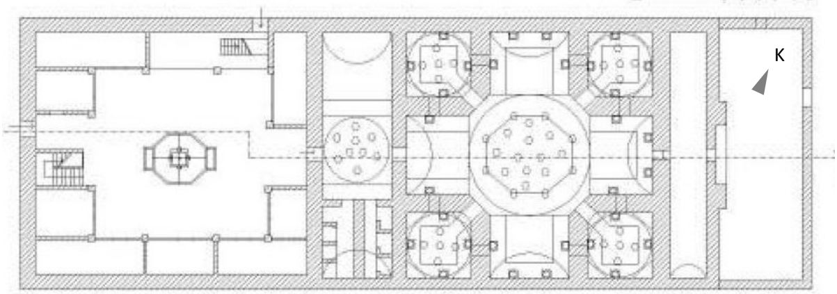
Şekil 5.52. Eski Paşa Hamamı Planı (Önder, 2007)
