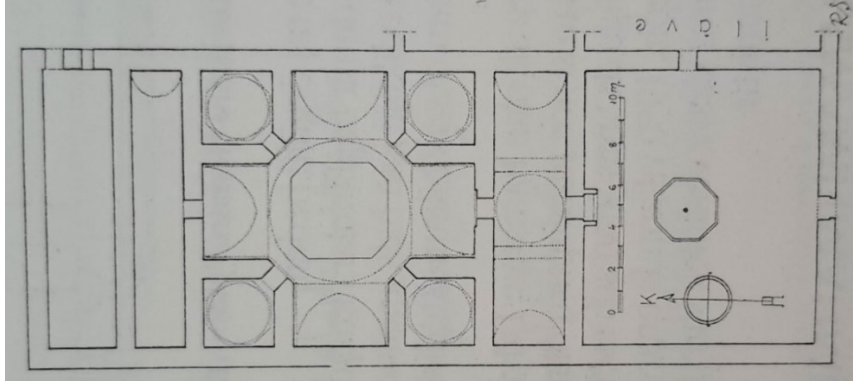
Şekil 4.27. Mehmet Ali Hamamı Planı (Bilget- Denizli, 1998)
