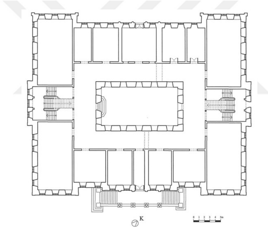
Şekil 5.37. Mülki İdadi Binası Zemin Kat Planı (Bulut, 2006; Bayındırlık Müdürlüğü Arşivi)
