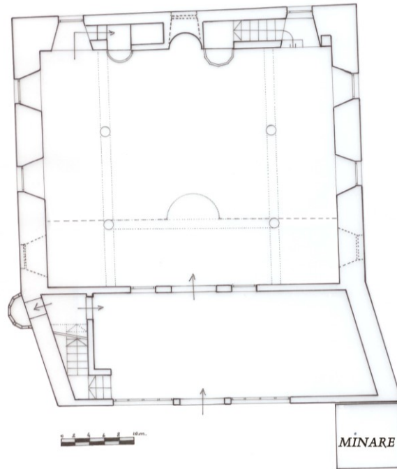
Şekil 4.18. Sivas Örtmeli Cami Planı (Ünsal, 2006)
