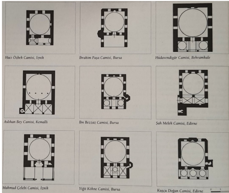
Şekil 4.2. Tek Kubbeli Cami Yapılarından Bazılarının Planları (Kuban, 2021)
