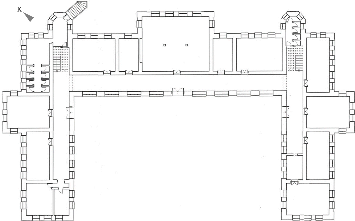
Şekil 5.63. Sivas Erkek Öğretmen Okulu (Selçuk Anadolu Lisesi) Zemin Kat Planı (Bulut, 2006)
