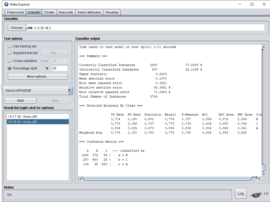
Şekil 4.5. Yüzdesel parçalama J48 algoritmasının Weka'daki sonucu
