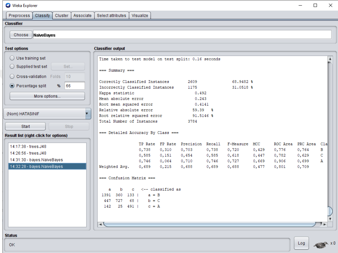
Şekil 4.7. Yüzdesel parçalama Naive Bayes algoritmasının Weka’daki sonucu
