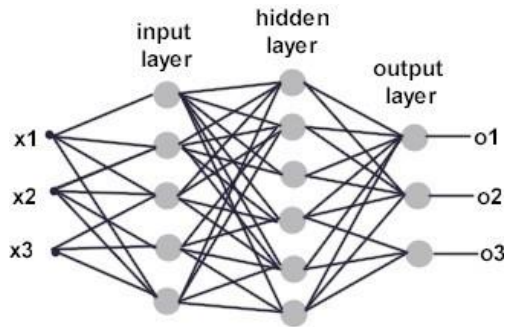
Şekil 3.19. Multilayer perceptron katmanları
