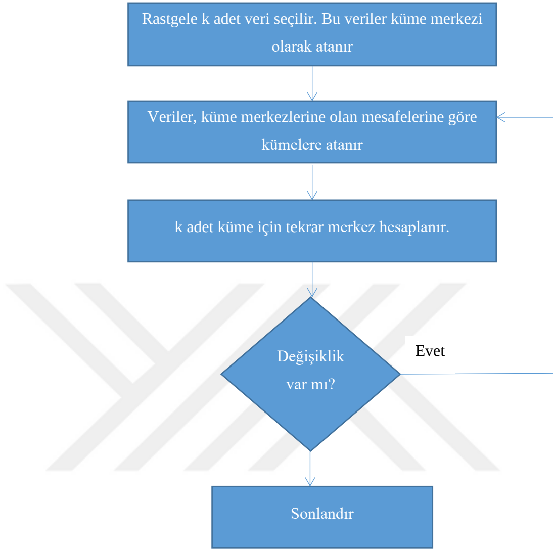
Şekil 3.8. Kümeleme iş akışı
