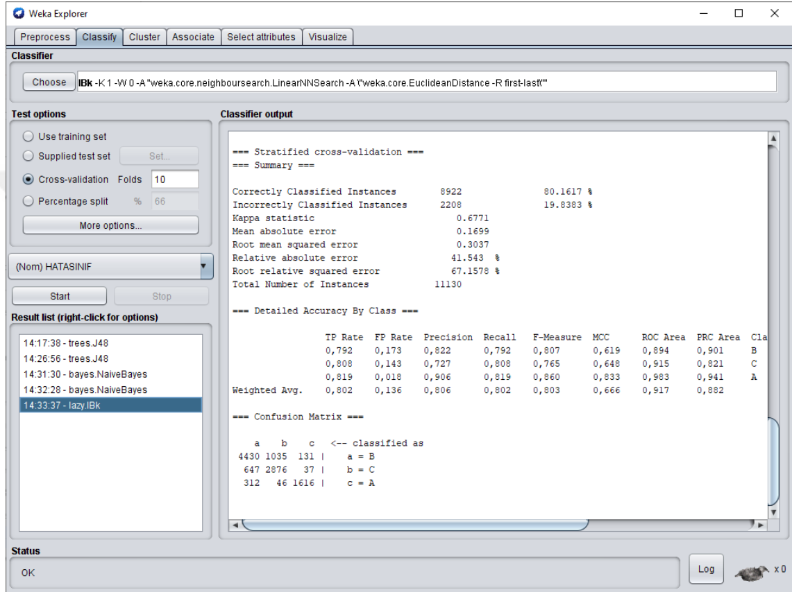
Şekil 4.8. Çapraz doğrulama K-NN algoritmasının Weka’deki sonucu
