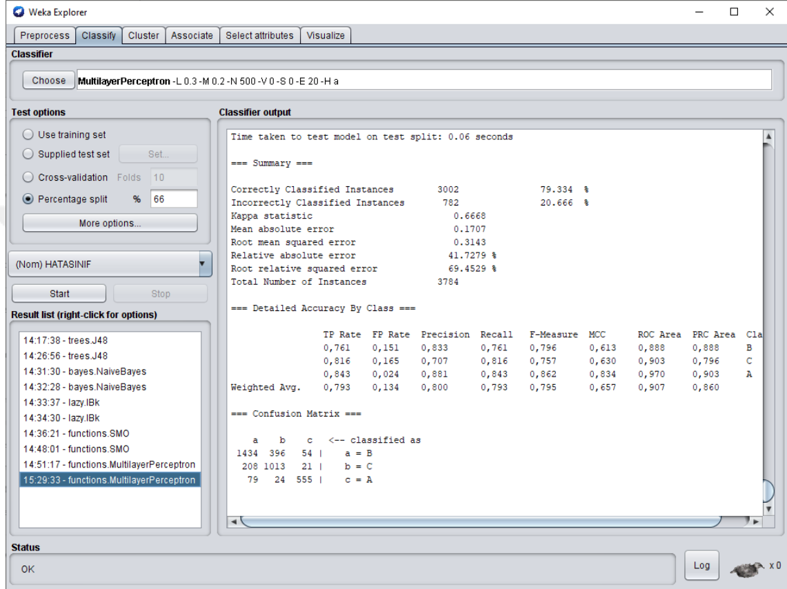
Şekil 4.13. Yüzdesel parçalama Multilayer Perceptron algoritmasının Weka'daki sonucu
