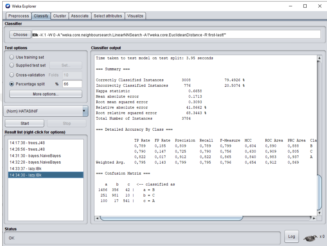
Şekil 4.9. Yüzdesel parçalama K-NN algoritmasının Weka’daki sonucu
