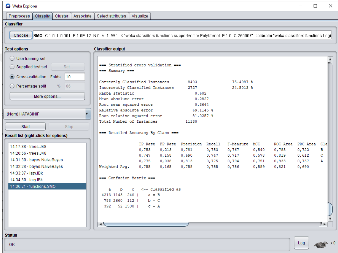
Şekil 4.10. Çapraz doğrulama SVM algoritmasının Weka'daki sonucu
