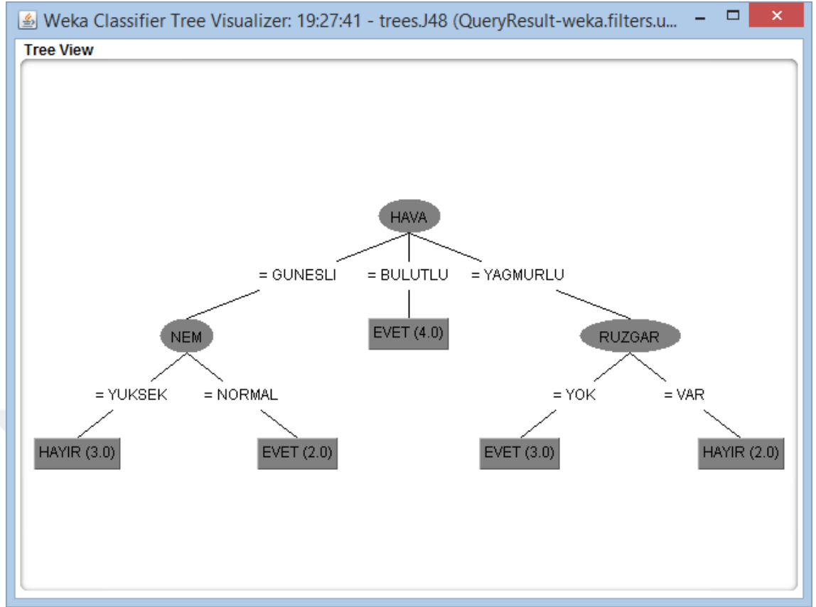
Şekil 3.5. Veri setinin Weka'daki ağaç görünümü
