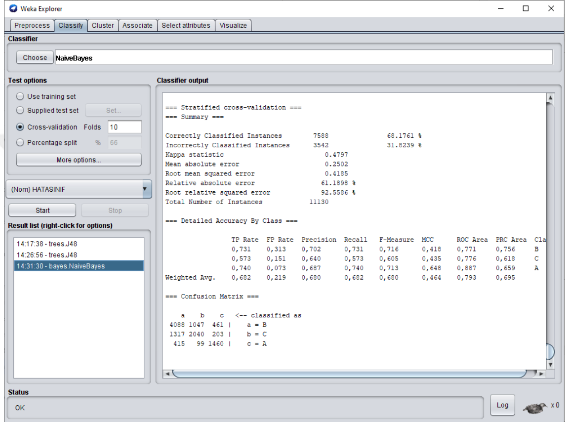
Şekil 4.6. Çapraz doğrulama Naive Bayes algoritmasının Weka’daki sonucu
