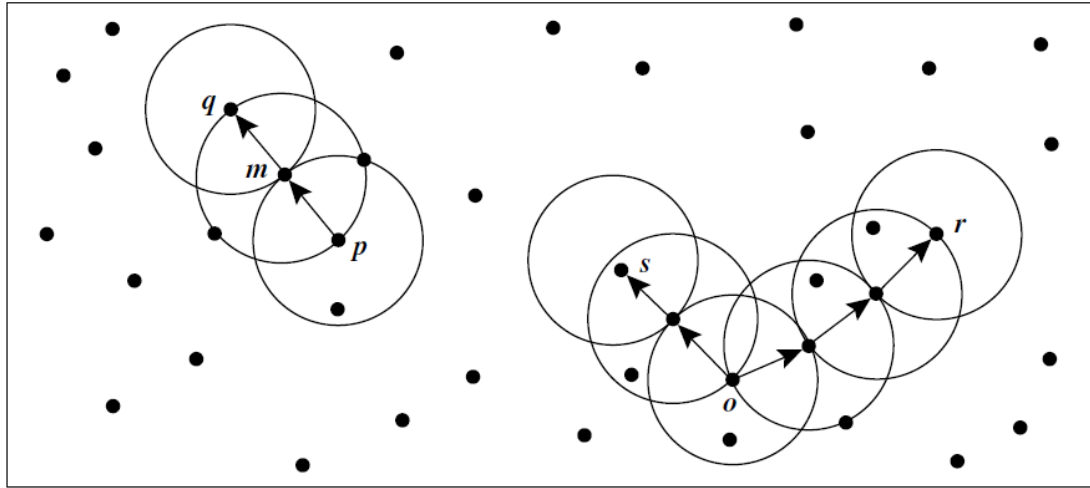
Şekil 3.11. Dbscan yöntemi
