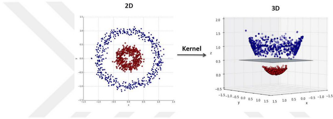
Şekil 3.17. Polynominal kernel
