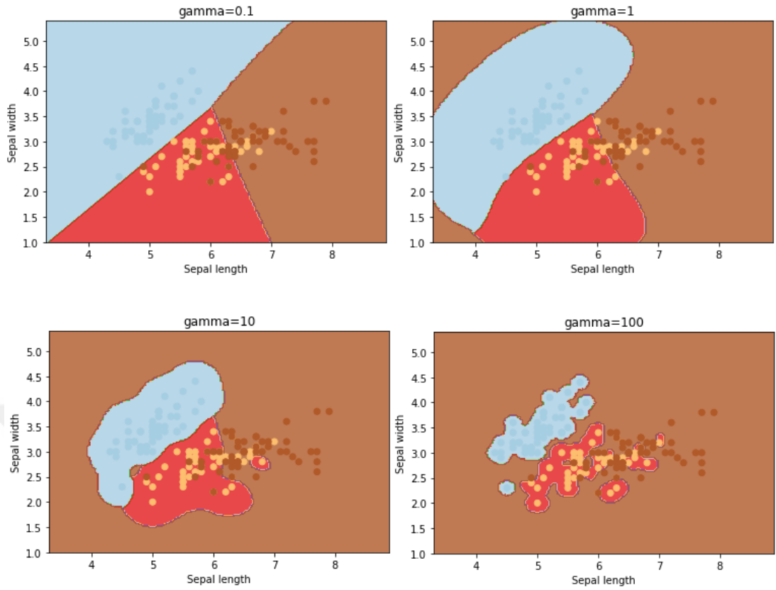
Şekil 3.18. Gaussian kernel
