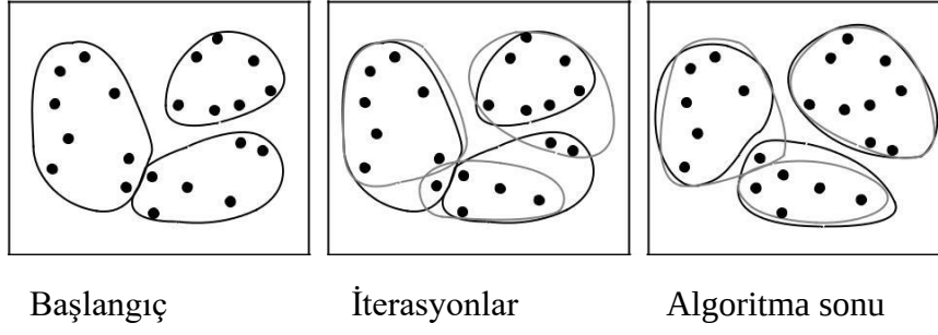
Şekil 3.9. k-means algoritması
