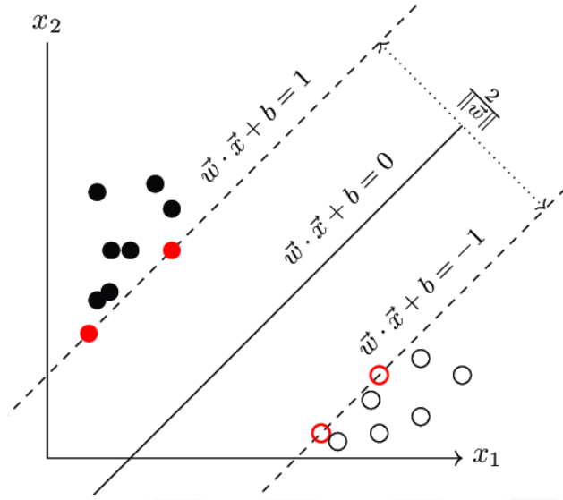
Şekil 3.15. SVM vektörleri ve marginler
