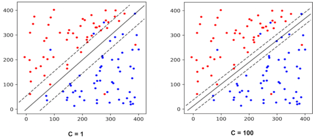
Şekil 3.16. Verilerin vektörlere göre ayrılması
