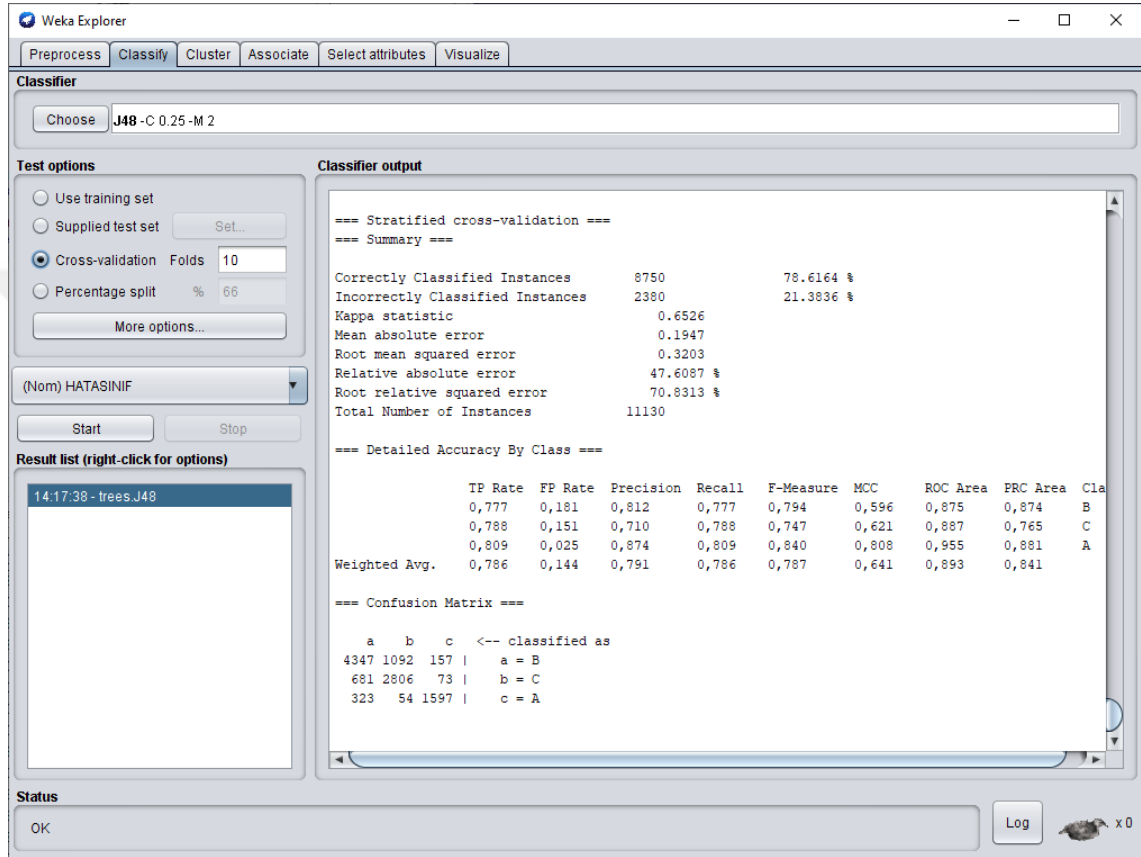
Şekil 4.4. Çapraz doğrulama J48 algoritmasının Weka'daki sonucu
