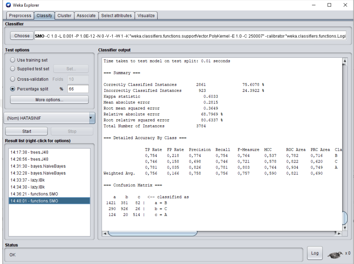
Şekil 4.11. Yüzdesel parçalama SVM algoritmasının Weka’daki sonucu
