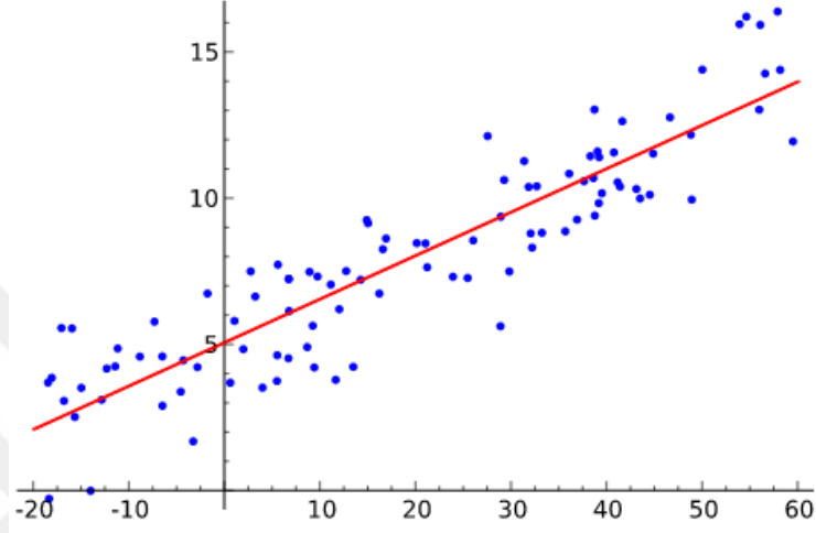
Şekil 3.6. Tahmin fonksiyonu
