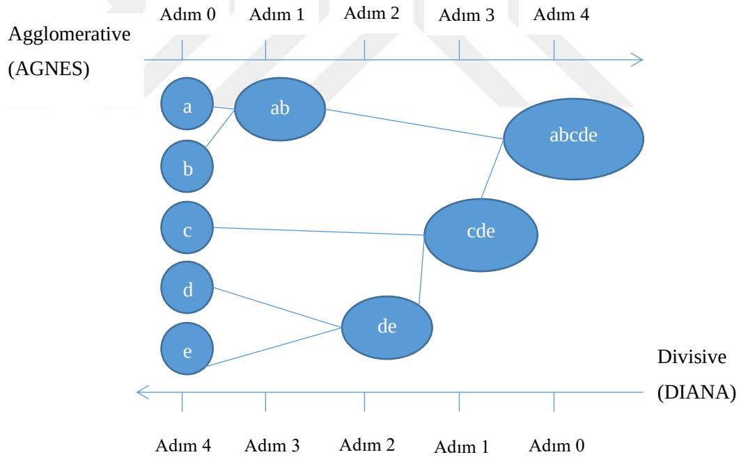
Şekil 3.10. Agnes ve Diana metotları
