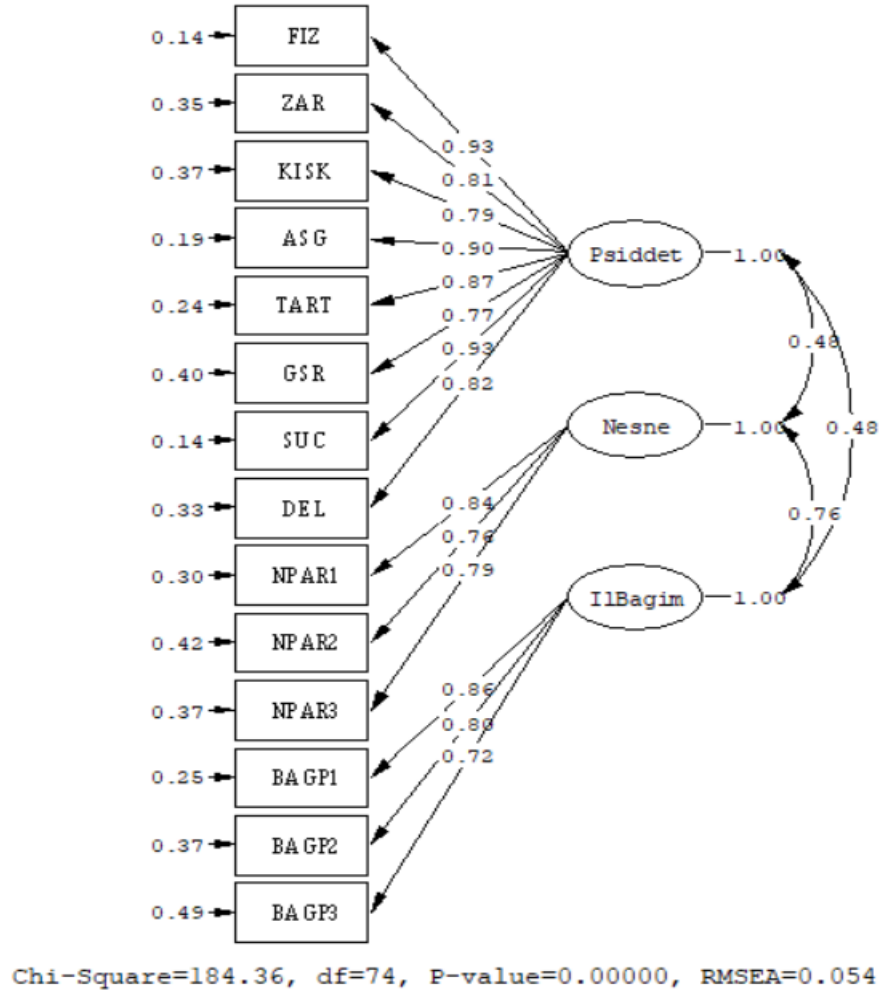
Şekil 3. Ölçme Modeline Ait Standardize Edilmiş Yol Katsayıları
