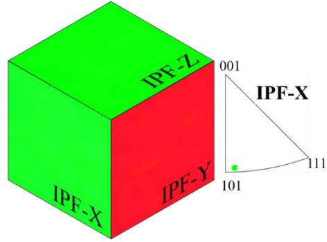
e) 110-NiCoCr-WQ/Failure
