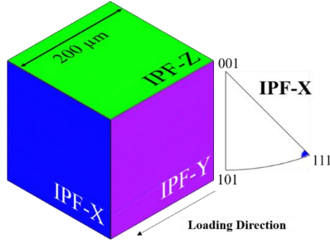
b) 111-NiCoCr-WQ/Failure
