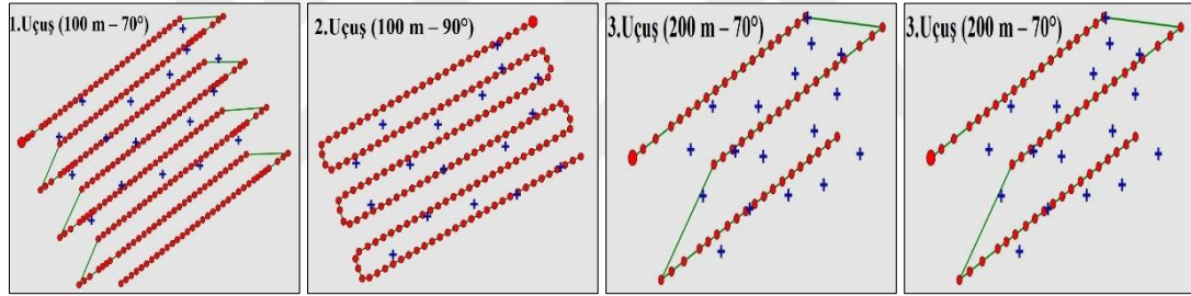
Şekil 4.3: Fotoğraf çekim noktaları ve arazi noktaları
