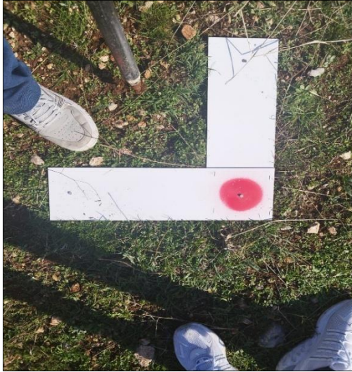
Şekil 4.1: Arazide işaretlenen nokta görünümü Şekil 4.2: Arazide işaretlenen noktaların konumları
