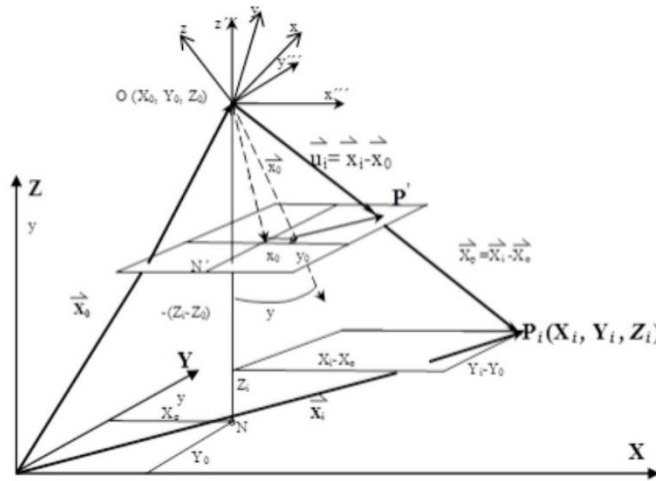
Şekil 3.2: Fotogrametri matematiksel modeli
