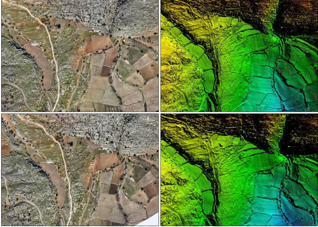
Şekil 4.7: Üretilen ortofoto ve sayısal yüzey modelleri
