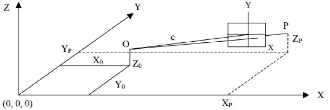
Şekil 3.3: Yersel fotogrametrik izdüşüm modeli
