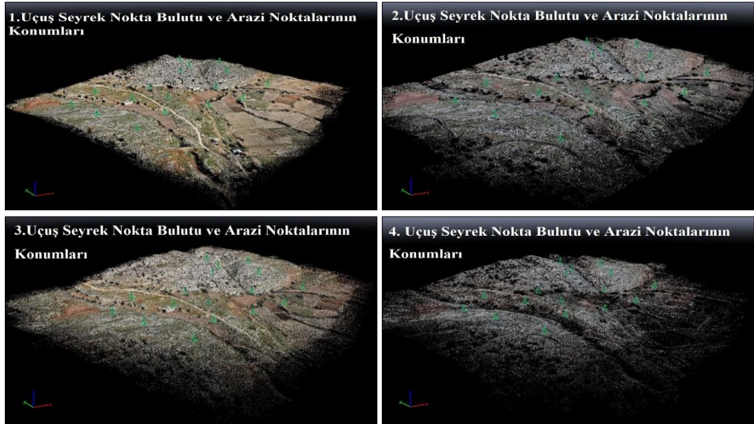
Şekil 4.4: Uçuşların seyrek nokta bulutu ve arazi noktalarının konumları
