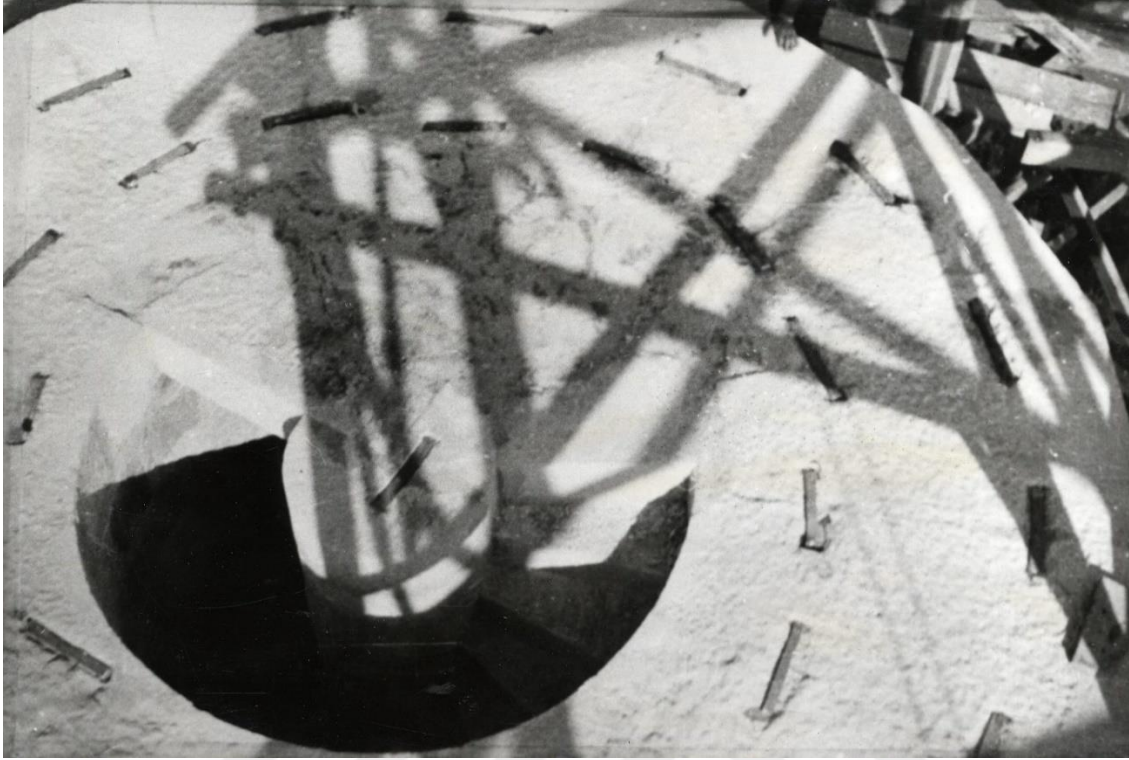
Resim 27: Selimiye Camii minaresinde kenet uygulaması 635
