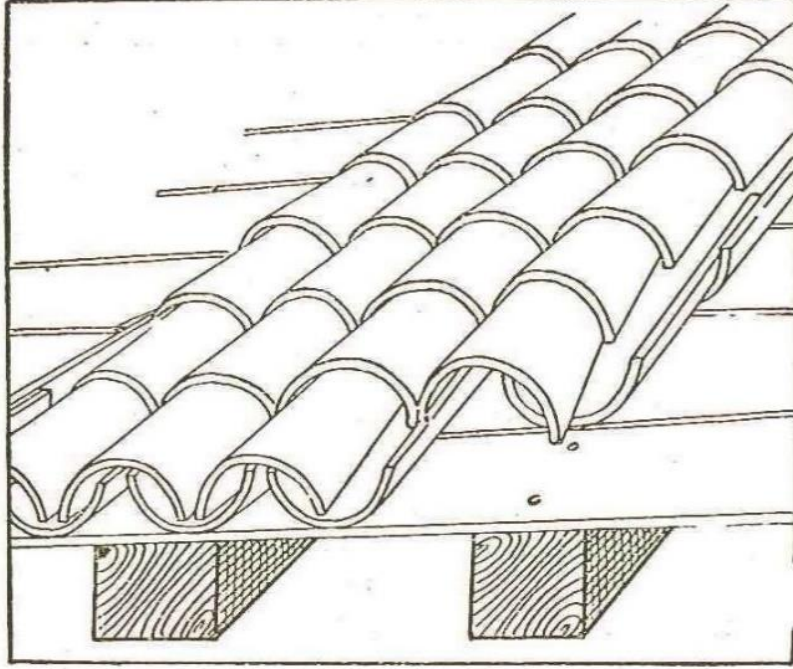
Resim 29: Kiremitlerin çatıdaki düzeni 678
