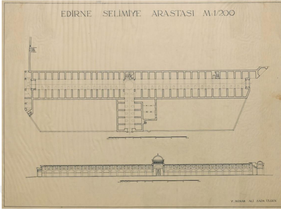
Çizim 2: Arasta ve Sıbyan Mektebi'nin plan ve kesiti 72
