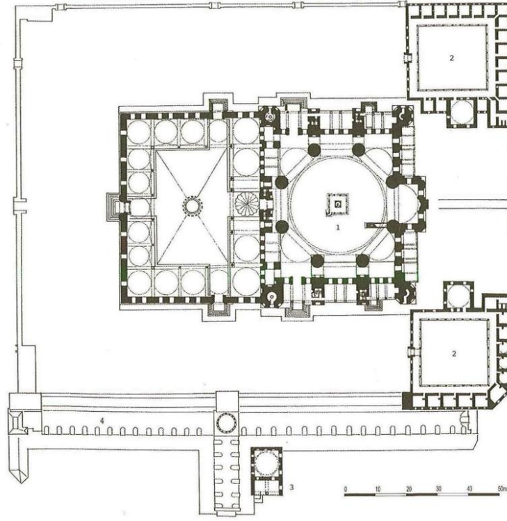
Çizim 1: Selimiye Külliyesi Vaziyet Planı: 1. Cami, 2. Medreseler, 3. Sıbyan Mektebi, 4. Arasta 61
