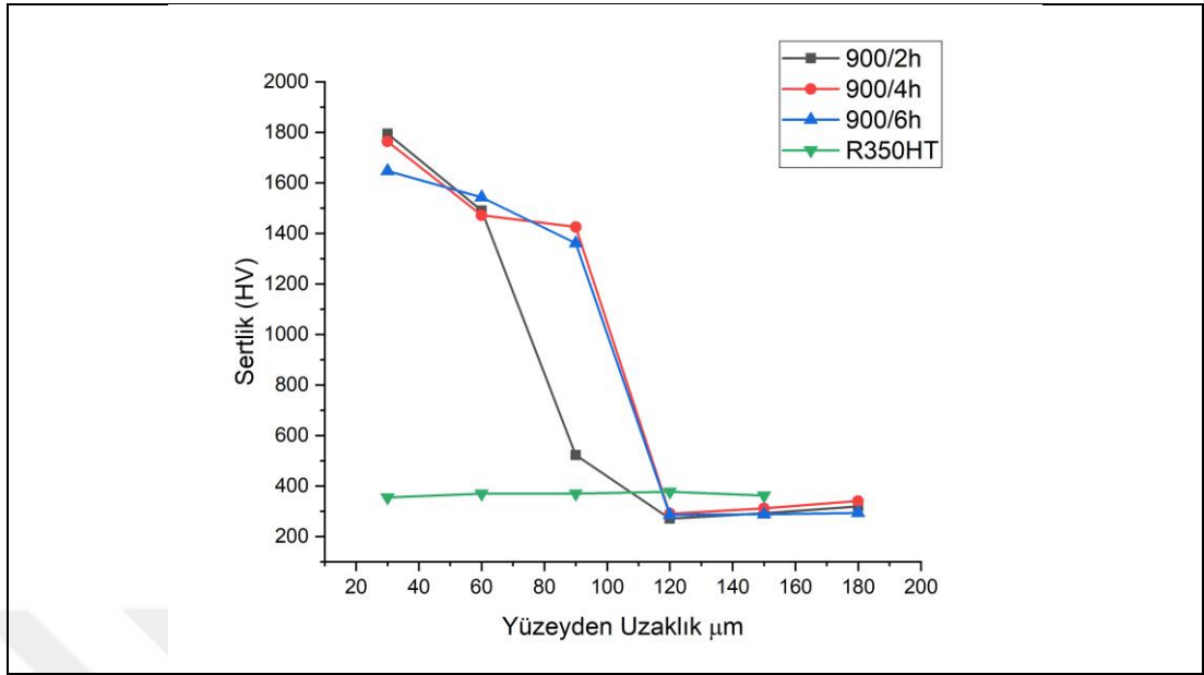
Şekil 39: Sertlik değişim grafiği (900 °C'de borlanan numuneler ve R350HT için)
