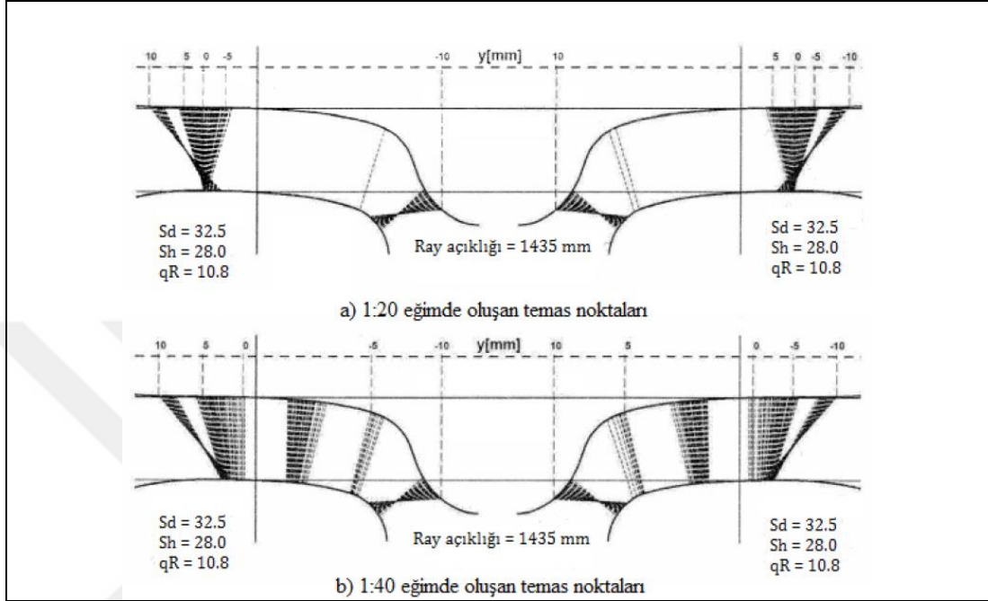
Şekil 5: Farklı eğimlerde Ray-Teker temas noktaları [10]
