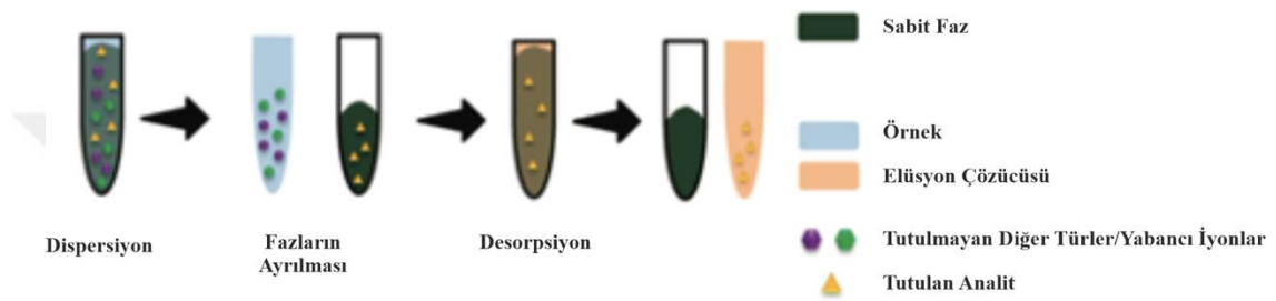
Şekil 2.8: Dispersif katı faz ekstraksiyon yöntemi şematik gösterimi (Socas Rodríguez ve diğ. 2015)
