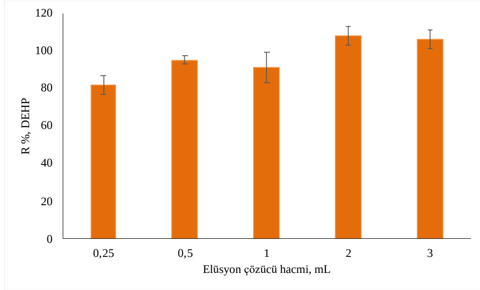
Şekil 6.11: Elüsyon çözücü hacminin ekstraksiyona etkisi (model çözeltide 1 ppm DEHP, 15 mg katı faz, 10 mL örnek hacmi, %50MeOH-%50ACN elüsyon çözücüsü, pH 8’de vorteks ile 3 dakika ve 1600 rpm çalkalama)
