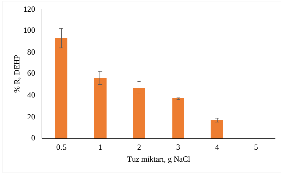
Şekil 6.14: Tuz miktarının ekstraksiyona etkisi (model çözeltide 1 ppm DEHP, 15 mg katı faz, 10 mL örnek hacmi, %50MeOH-%50ACN hacminde 0,5 mL elüsyon çözücüsü, pH 8’de vorteks ile 3 dakika ve 1600 rpm çalkalama)
