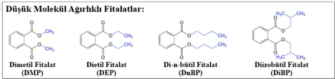
Şekil 2.3: Düşük molekül ağırlıklı fitalatlar (Juneau 2021)
