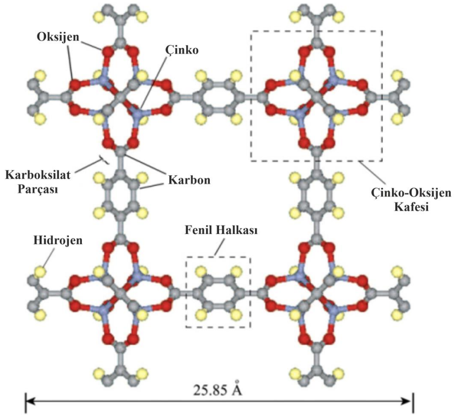
Şekil 3.2: MOF-5 kübik yapısı (Huang ve diğ. 2006)
