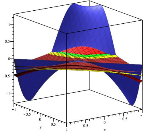
Şekil 4.2. H_n(h; \xi, \rho) operatörünün h(\xi, \rho) = \sin(\pi(\xi + \rho))(\xi^2 + \rho^2) fonksiyonuna farklı n değerleri için yaklaşımı.
