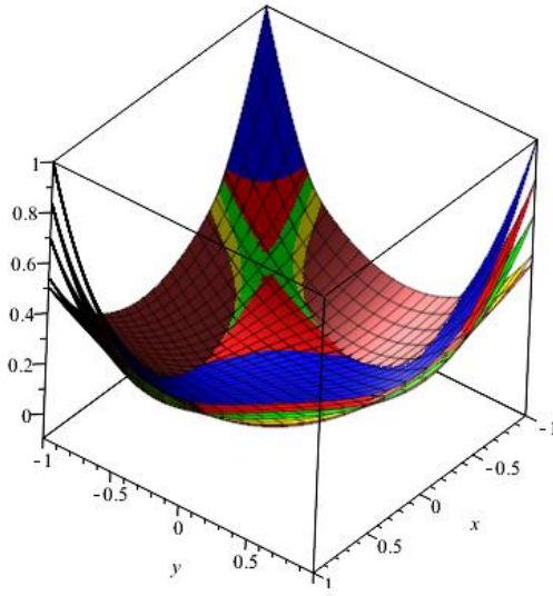
Şekil 4.4. E_n(h; \xi, \varrho) operatörünün h(\xi, \varrho) = |\xi^2 \varrho^2| fonksiyonuna farklı n değerleri için yaklaşımı.
