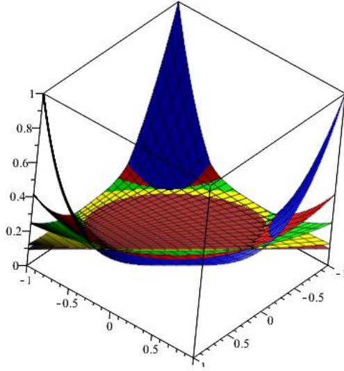
Şekil 4.3. H_n(h; \xi, \rho) operatörünün h(\xi, \rho) = |\xi^2 \rho^2| fonksiyonuna farklı n değerleri için yaklaşımı.
