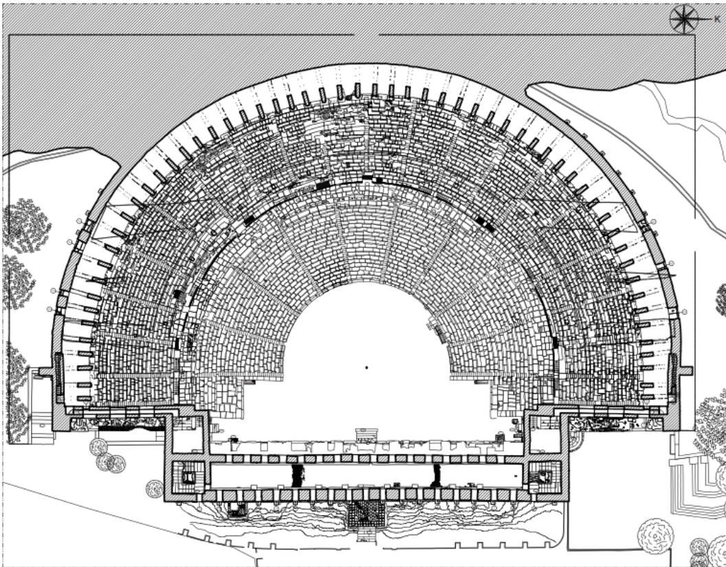
Şekil 3.3. Aspendos Antik Tiyatrosu +19.40 kotu planı
