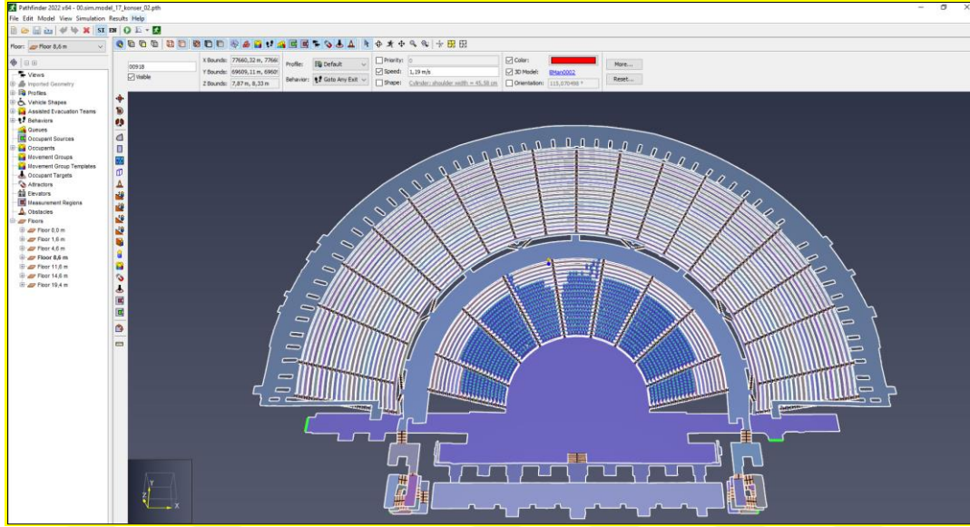
Şekil 3.18. Senaryo 00 Pathfinder benzetim modeli
