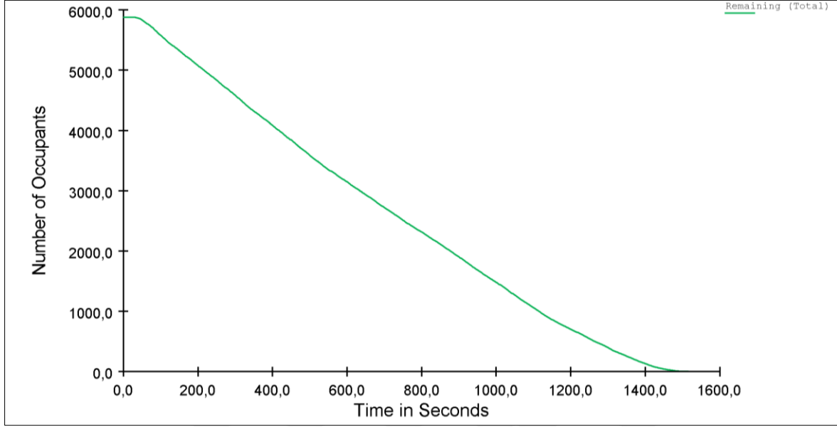
Şekil 4.4. Yapıda bulunan kullanıcı sayısı-zaman grafiği
