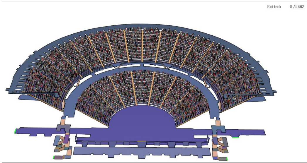
Şekil 3.14. Pathfinder benzetim modelinde tam kapasite doluluk durumu
