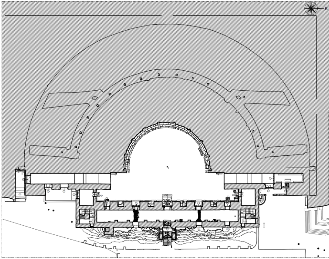
Şekil 3.1. Aspendos Antik Tiyatrosu 0.00 kotu planı
