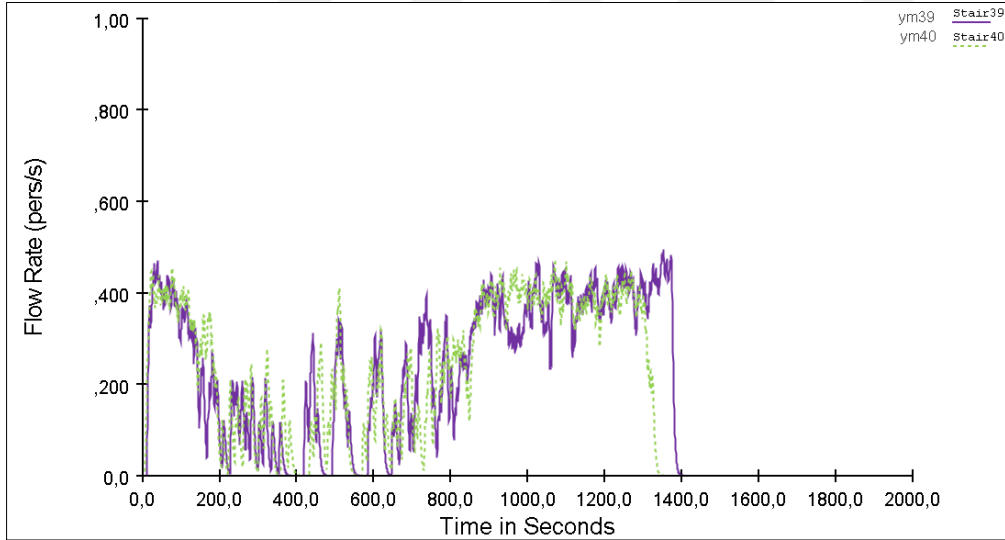
Şekil 4.8. ym39 ve ym40 merdivenlerindeki akış hızı
