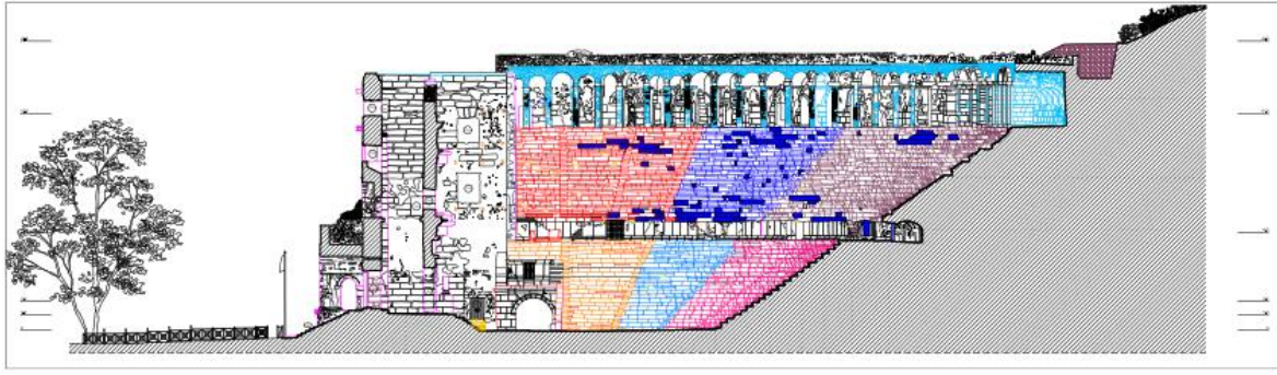
Şekil 3.4. Aspendos Antik Tiyatrosu doğu batı yönünden kesiti
