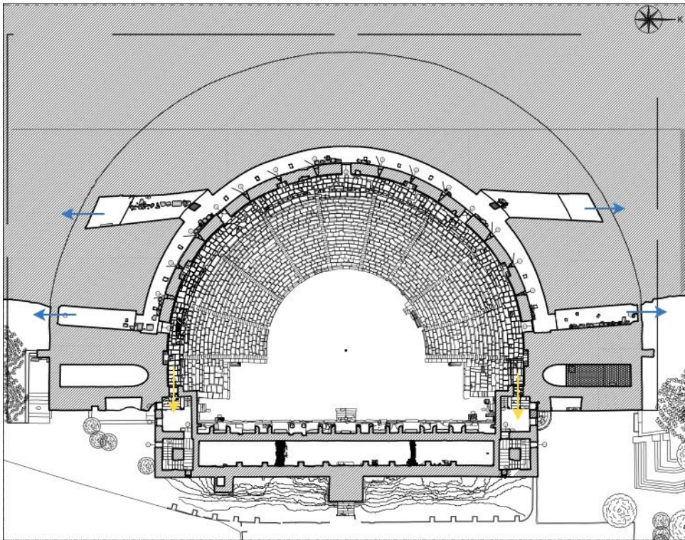
Şekil 3.11. 0.00 kotu çıkışları
