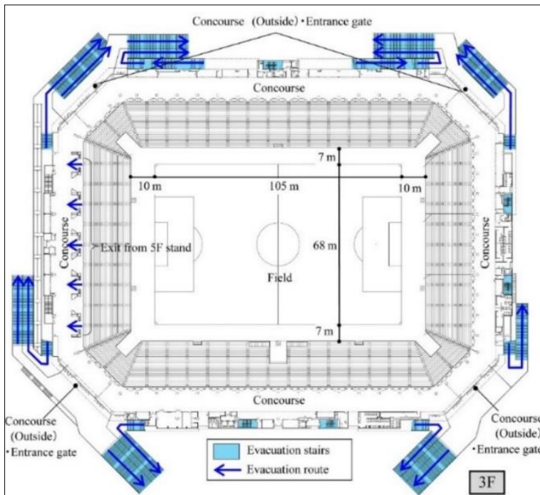
Şekil 2.17. Tahliye yolları ve çıkışların gösterildiği 3F kat planı (Minegishi & Takeichi, 2018)
