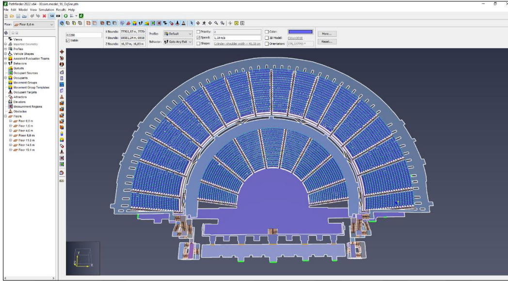
Şekil 3.21. Senaryo 02a Pathfinder benzetim modeli
