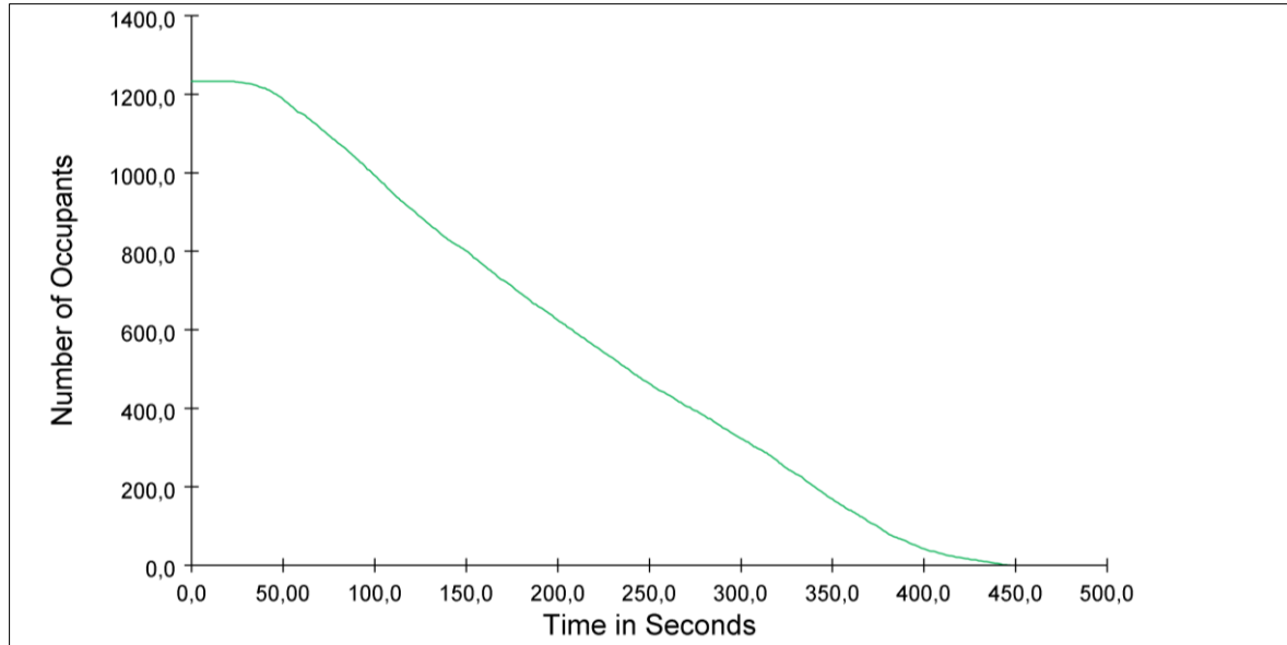
Şekil 4.1. Yapıda bulunan kullanıcı sayısı-zaman grafiği
