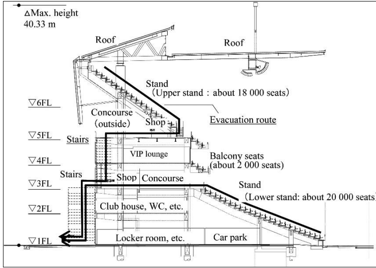
Şekil 2.16. Yapının kesiti üzerinde gösterilen tahliye yolu (Minegishi & Takeichi, 2018)
