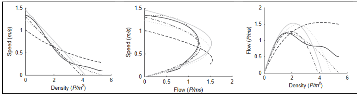
Şekil 2.7. Kullanıcı akışı ve yürüme hızı, kullanıcı yoğunluğu ve yürüme hızı, kullanıcı akışı ve kullanıcı yoğunluğu arasındaki ilişkiler (Daamen vd., 2005)
