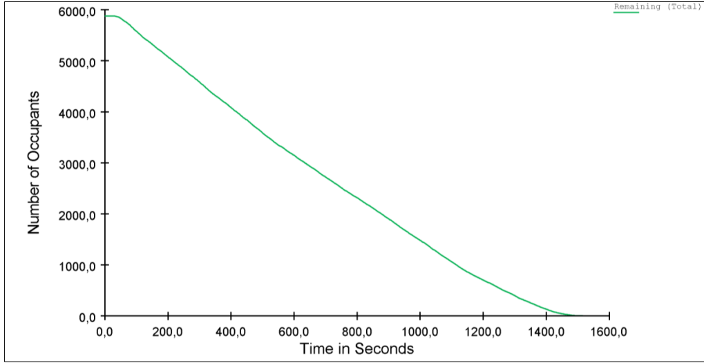
Şekil 4.9. Yapıda bulunan kullanıcı sayısı-zaman grafiği
