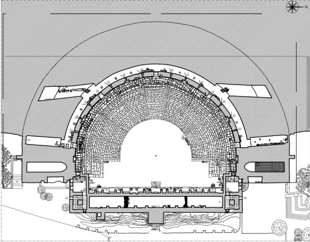
Şekil 3.2. Aspendos Antik Tiyatrosu +8.60 kotu planı
