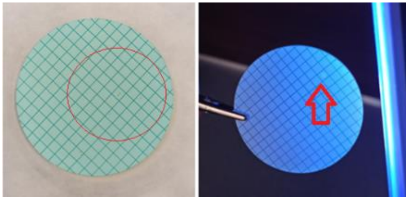
Resim 4.7. Tespit edilen toplam koloni (solda) ve Pseudomonas aeruginosa (sağda)
