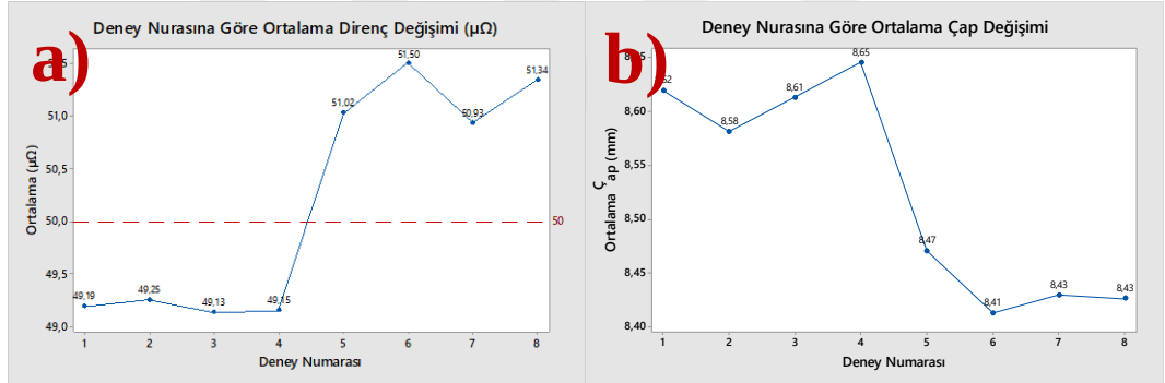
Şekil 6.1.1: a) Deney Numarasına Göre Direnç (μΩ) Değişimi, b) Deney Numarasına Göre Ortalama Çap Değişimi
