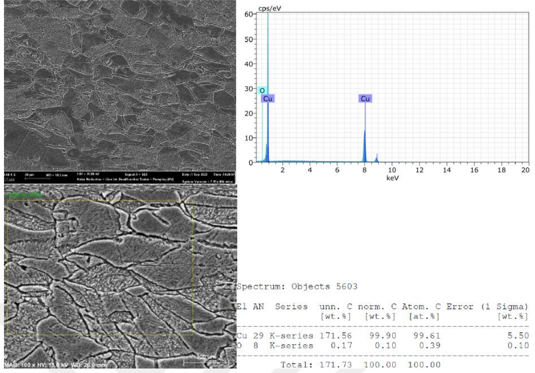
Şekil 5.5.12: 8. Deney-KB2-1500X (En Yüksek Sertlik Değeri)
