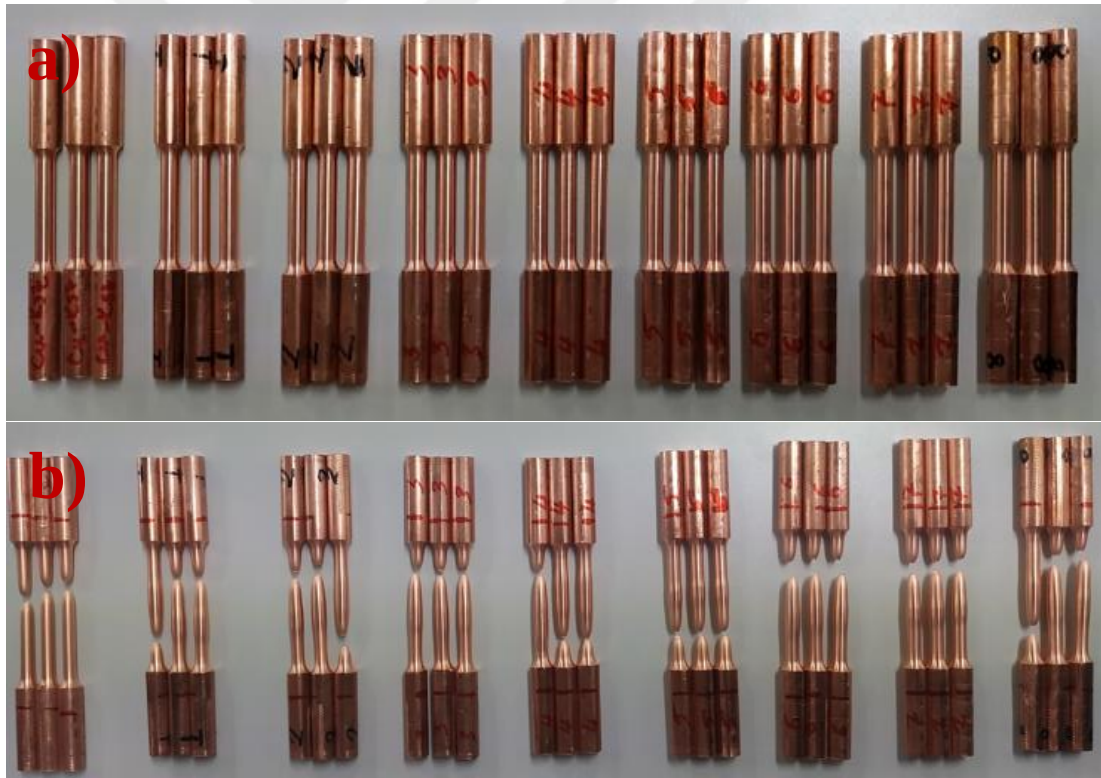
Şekil 5.4.1: Çekme numunelerinin a) Çekme deneyi öncesindeki görüntüsü, b) Çekme deneyi yapıldıktan sonraki görüntüsü ve kopma noktaları
