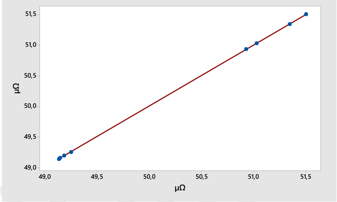
Şekil 5.2.3.1: Direnç değişiminde deneysel sonuçlarla tahmin edilen sonuçların karşılaştırılması
