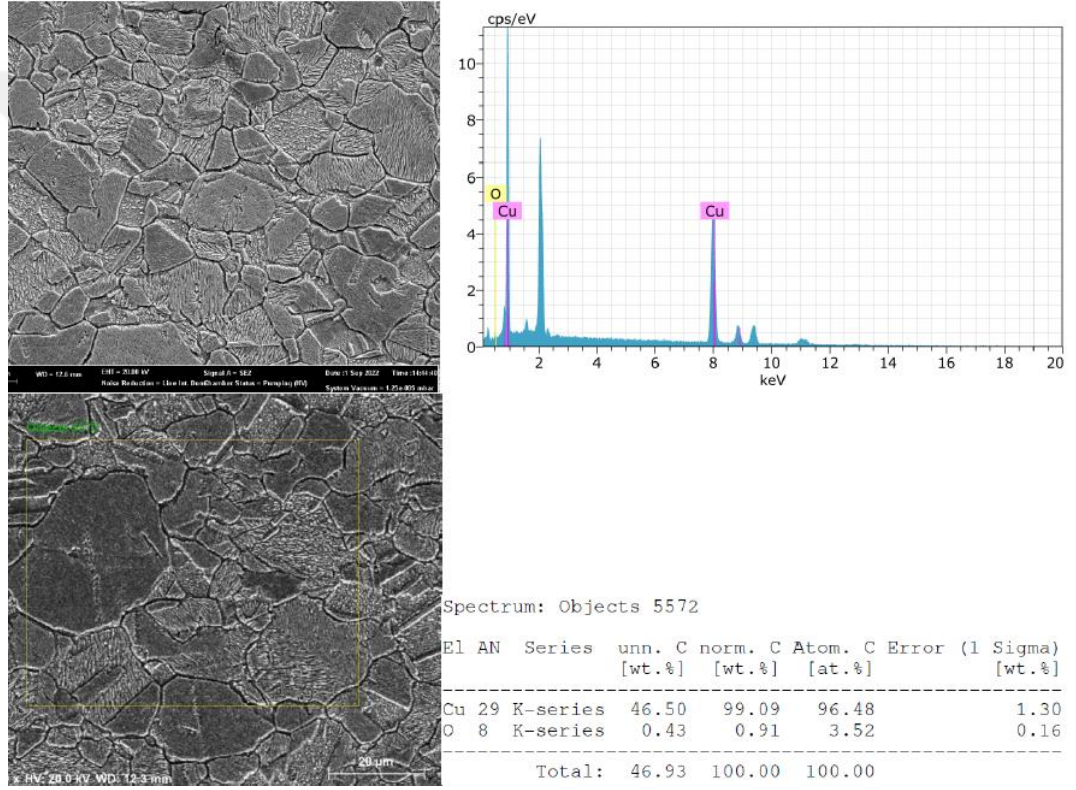
Şekil 5.5.17: 4. Deney-KB4-1500X (En Yüksek Sertlik Değeri)
