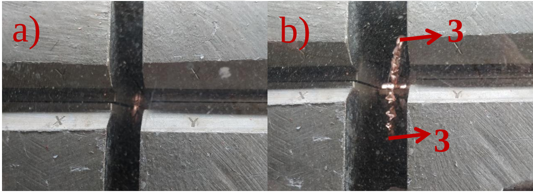
Şekil 4.2.1.4: Soğuk Basıncılı Kaynak Yapımının İşlem Sırası-2 a) Makine kaynak yapmaya başlamış ve ilk vuruş tamamlanmış halinin görüntüsü b) Makine kaynak yapmaya başlamış ve 6 vuruş tamamlanmış halinin görüntüsü
