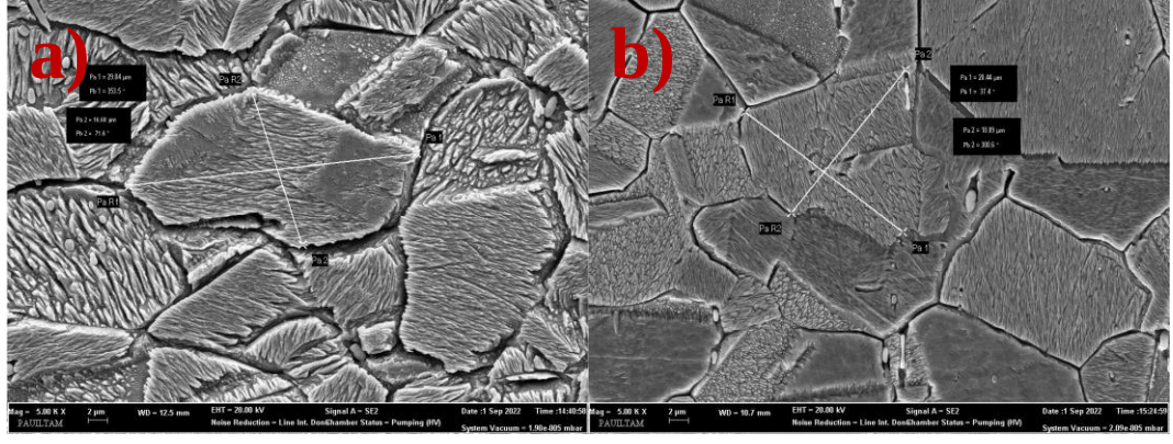
Şekil 5.5.16: a) 4. Deney-KB3-5000X (En Yüksek Sertlik Değeri), b) 7. Deney-KB3-5000X (En Düşük Sertlik Değeri)
