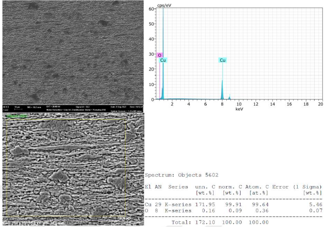
Şekil 5.5.8: 8. Deney-KB1-1500X (En Yüksek Direnç)
