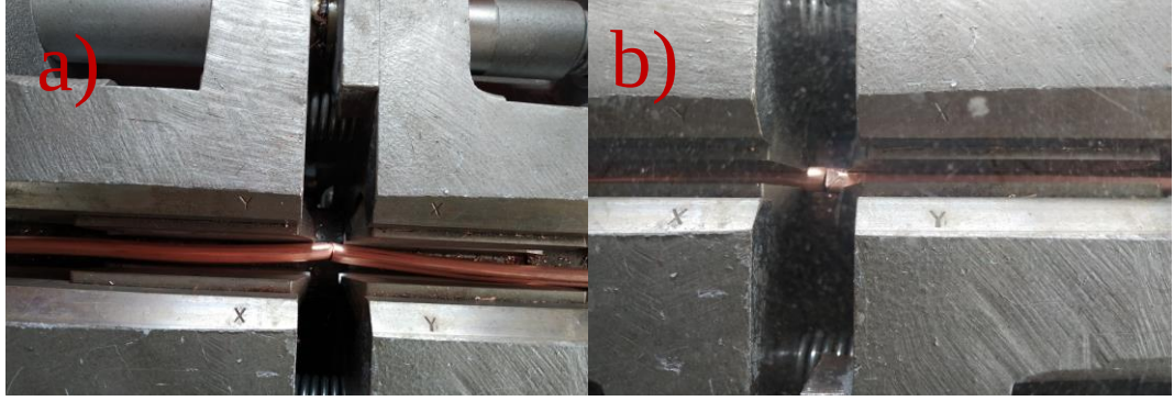
Şekil 4.2.1.3: Soğuk Basıncılı Kaynak Yapımının İşlem Sırası-1 a) Makine boş pozisyonda bakır yükleme işlemi b) Makine yükleme pozisyonuna getirilerek malzemelerin yanlardan sürülme işlemi
