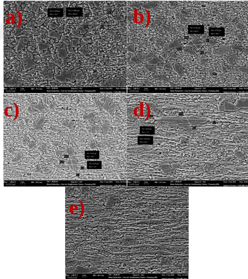
Şekil 5.5.9: a) 2. Deney-KB1-5000X (En İyi Çekme Mukavemet Değeri), b) 3. Deney-KB1-5000X (En Kötü Çekme Mukavemet Değeri), c) 5. Deney-KB1-5000X (En Düşük Sertlik), d) 6. Deney-KB1-5000X (En Yüksek Sertlik), e) 8. Deney-KB1-5000X (En Yüksek Direnç)
