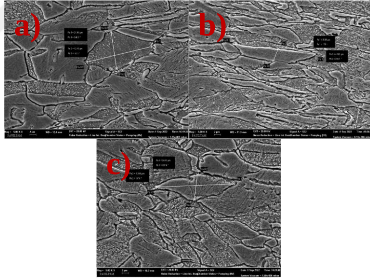
Şekil 5.5.13: a) 3. Deney-KB2-5000X (En Düşük Sertlik Değeri), b) 6. Deney-KB2-5000X (En Düşük Sertlik Değeri), c) 8. Deney-KB2-5000X (En Yüksek Sertlik Değeri)
