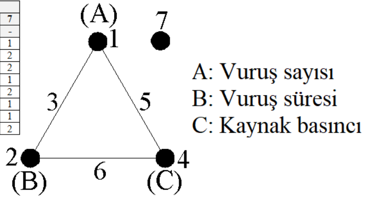
Şekil 5.1: Faktör ve etkileşimlerin lineer grafik yöntemiyle ortogonal dizinin sütunlarına aktarılması
