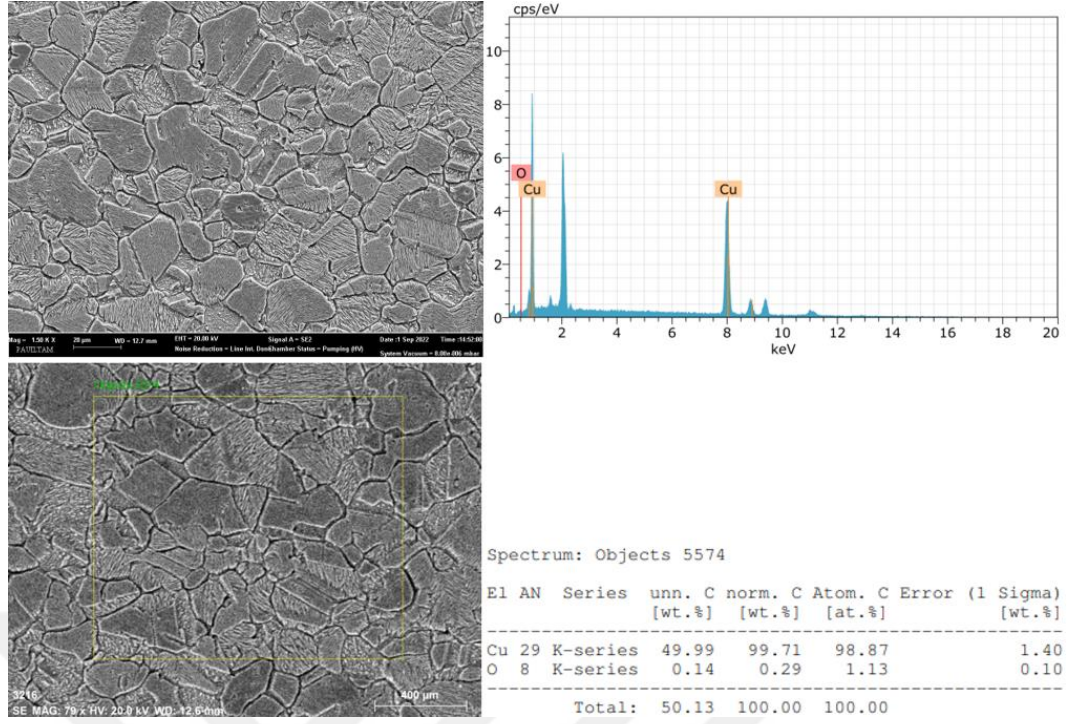
Şekil 5.5.23: 4.Deney-KB6-1500X (En Yüksek Sertlik Değeri)
