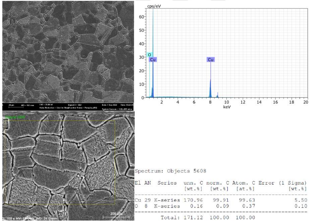
Şekil 5.5.24: 7. Deney-KB6-1500X (En Düşük Sertlik Değeri)
