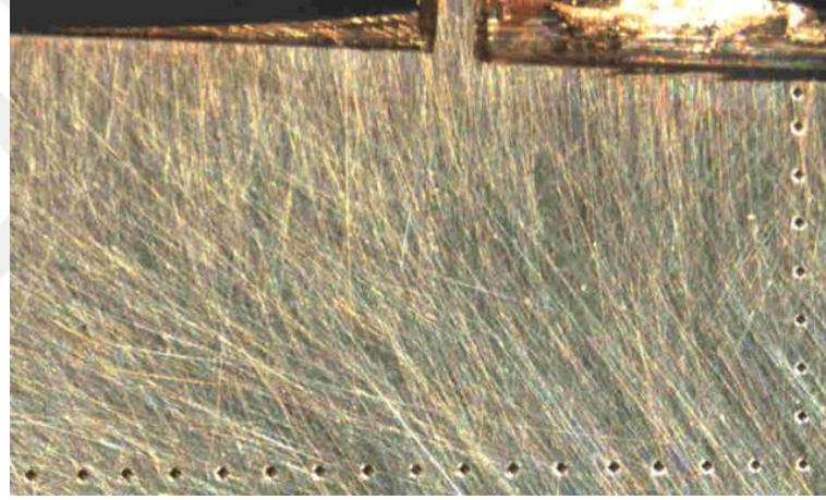
Şekil 4.5.11: Sıcak kalıba alınmış ve mikro sertlik ölçümü yapılmış numune örneği-1X
