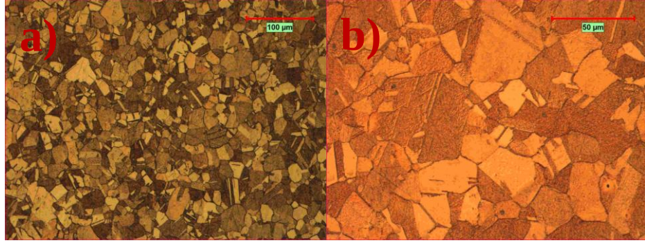
Şekil 5.5.1: a) Cu-ETP malzemenin 200X büyütmedeki kaynaksız iç yapı görüntüsü, b) Cu-ETP malzemenin 500X büyütmedeki kaynaksız iç yapı görüntüsü
