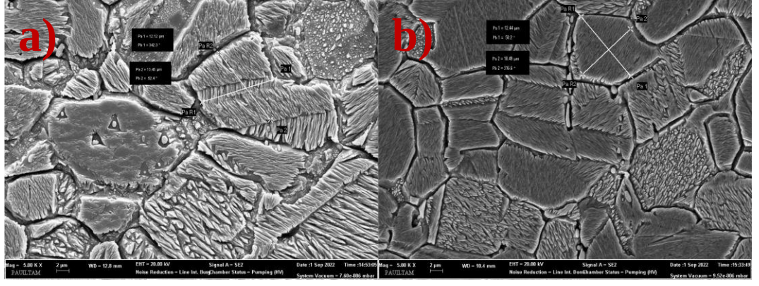
Şekil 5.5.25: a) 4. Deney-KB6-5000X (En Yüksek Sertlik Değeri), b) 7. Deney-KB6-5000X (En Düşük Sertlik Değeri)
