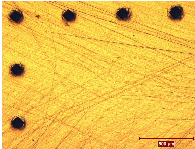
Şekil 4.5.12: Mikro sertlik ölçümü yapılmış numune örneği-50X
