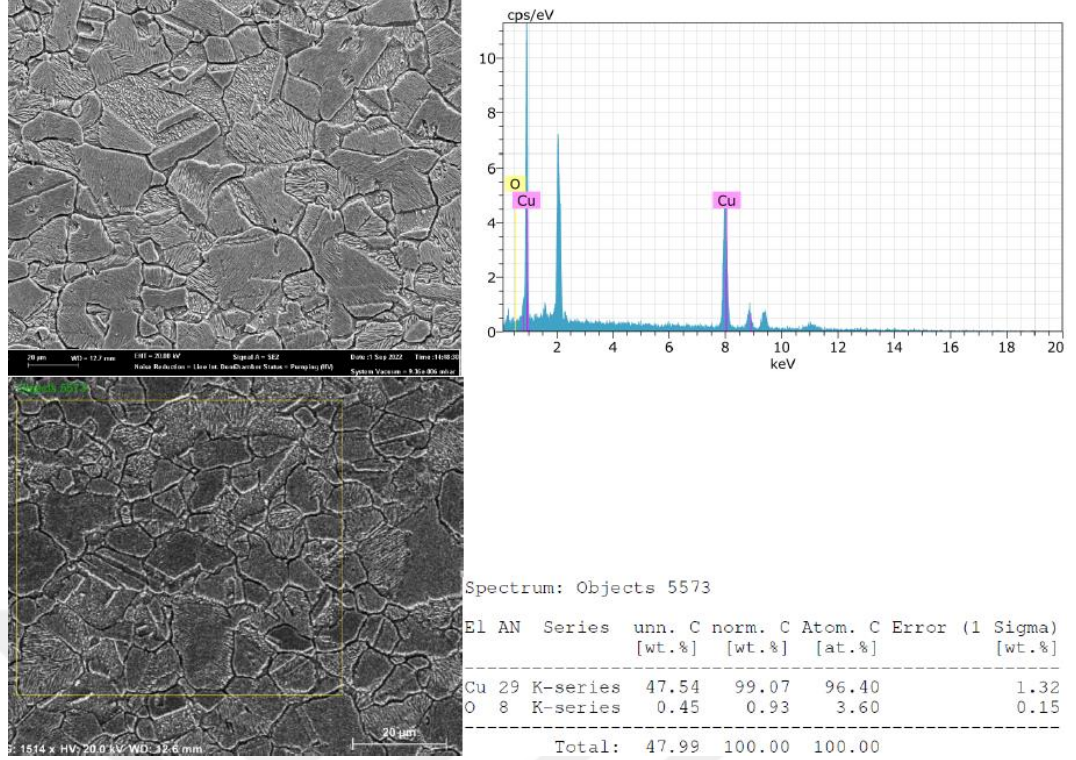
Şekil 5.5.20: 4. Deney-KB5-1500X (En Yüksek Sertlik Değeri)
