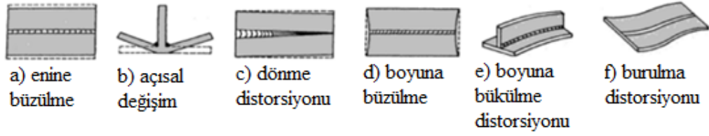
Şekil 3.28. Çeşitli kaynak distorsiyonu türleri [37].
