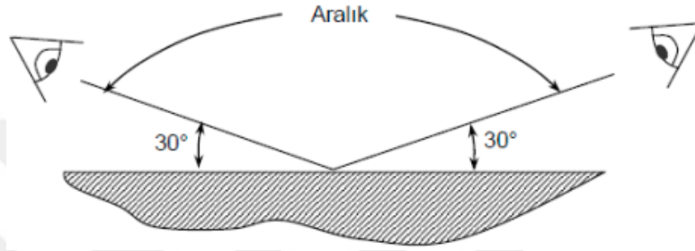
Şekil 4.1. Muayene açısı [48].
