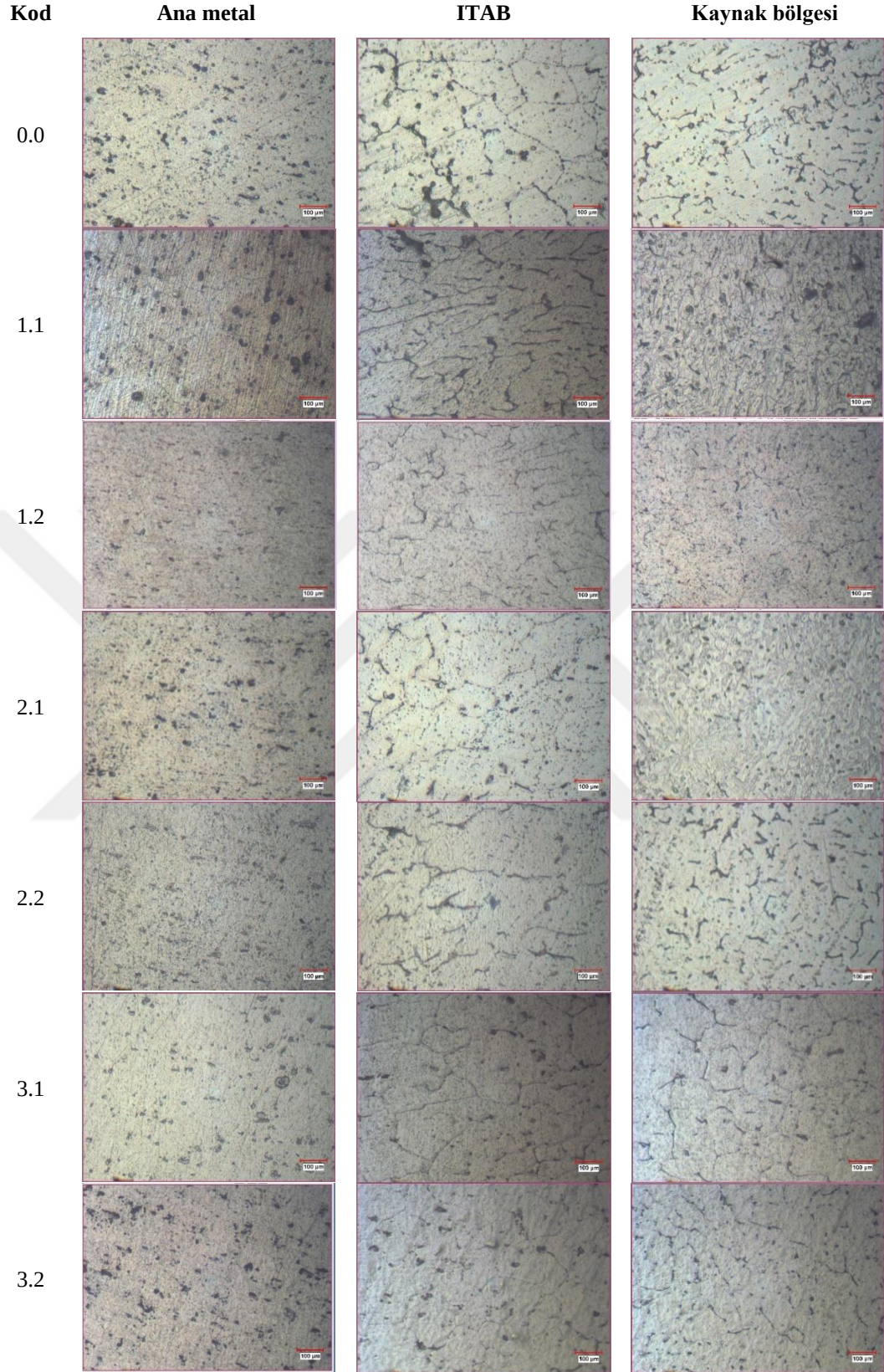
Şekil 6.11. Kaynak tamiri yapılmamış MIG kaynağının ve MIG ve TIG kaynaklarıyla tamiraty yapılmış numunelerin 50X büyütmedeki mikroyapı görüntüleri.
