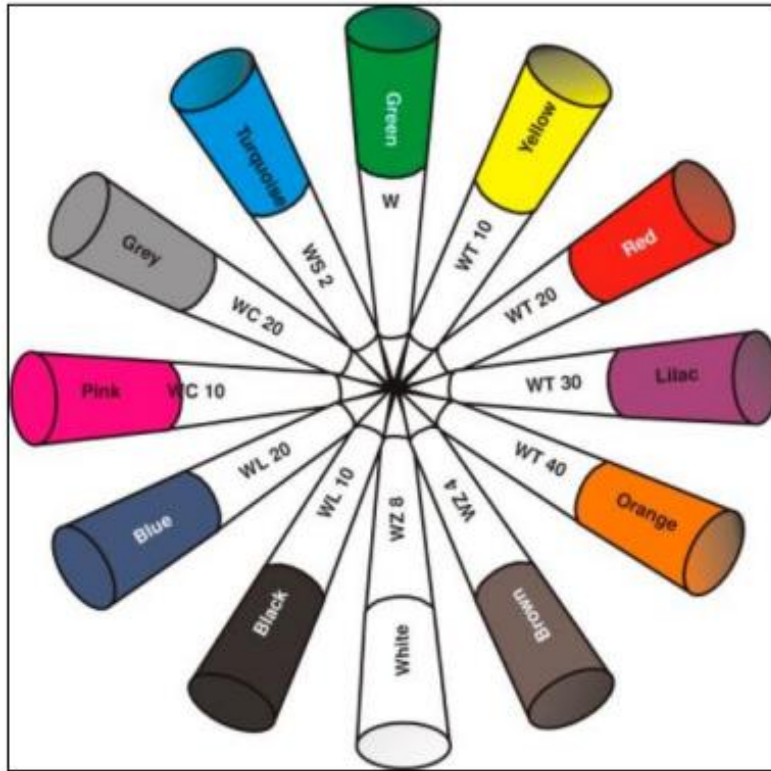
Şekil 3.16. Renklerine göre DIN standardı ile tanımlanan elektrotlar [28].
