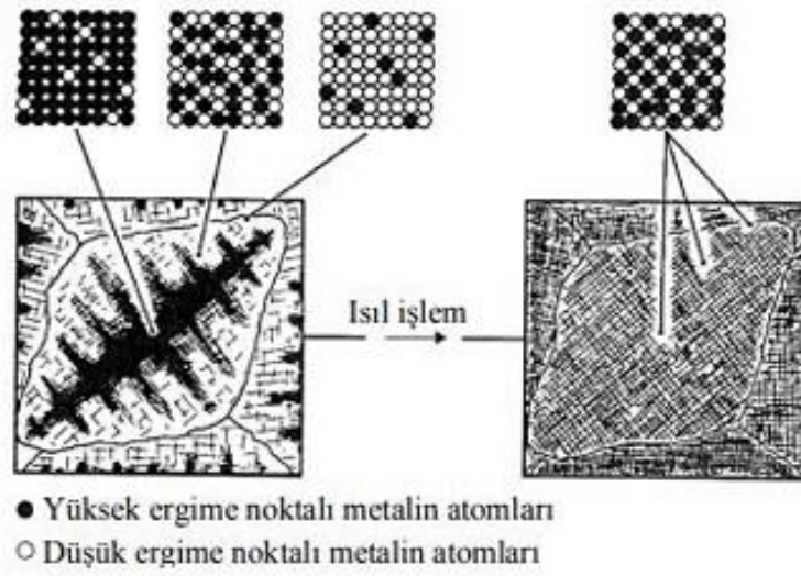
Şekil 2.2. Çekirdeklenmiş bir katı çözeltilde bileşimin farklılık göstermesi [12].
