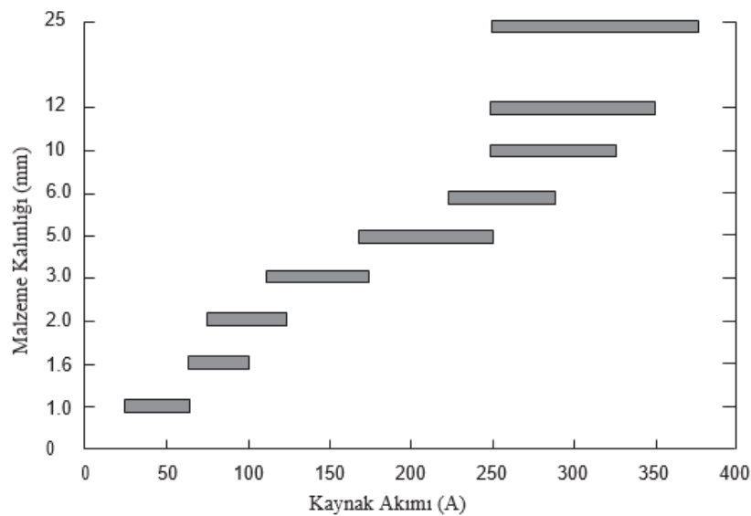
Şekil 3.17. Çeşitli malzeme kalınlıkları için tipik TIG akım aralıkları [30].
