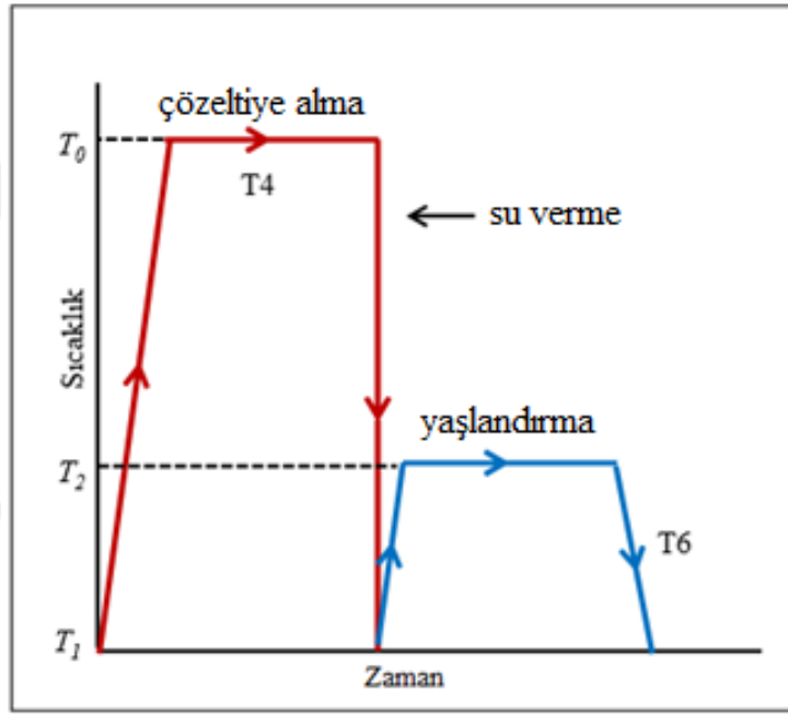
Şekil 2.7. T6 ısı işleminde çökeltme sertleşmesinin iki aşaması. [21].
