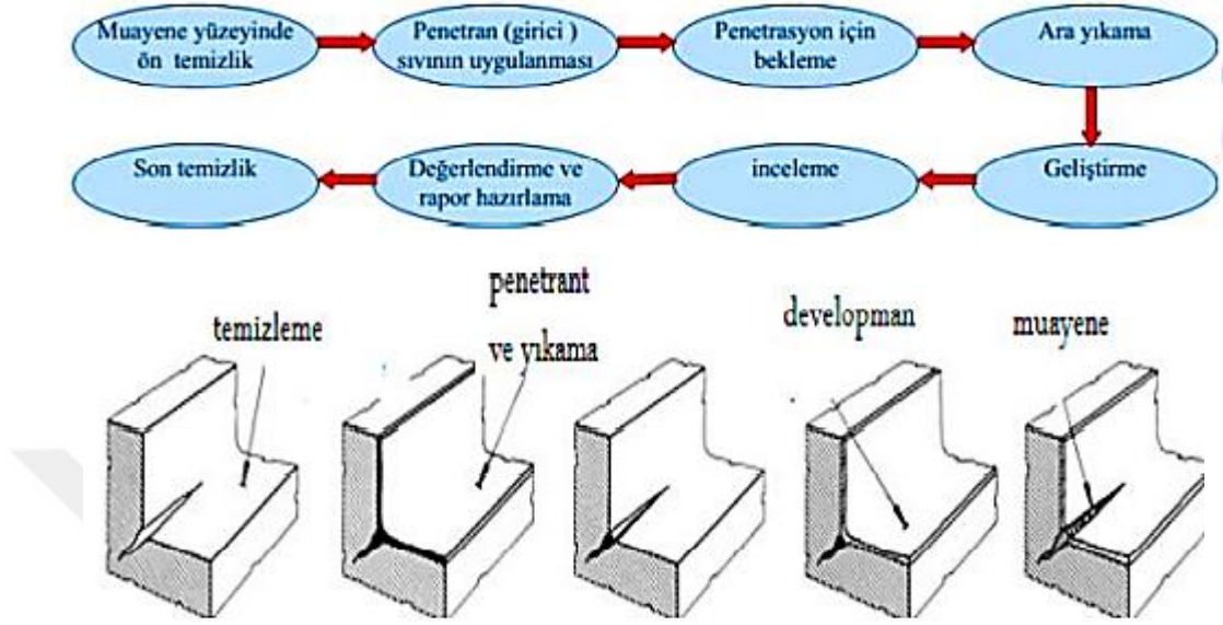
Şekil 4.5. Penetrant testi işlem sırası [48].
