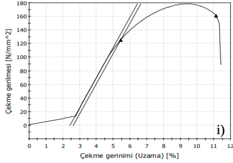
Şekil 6.7. a) ve b) 0.0, c) ve d) 1.1, e) ve f) 1.2, g) ve h) 2.1, i) ve j) 2.2, k) ve l) 3.1, m) ve n) 3.2 numaralı numunelerin çekme ve eğme testi grafikleri.
