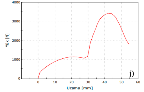
Şekil 6.7. a) ve b) 0.0, c) ve d) 1.1, e) ve f) 1.2, g) ve h) 2.1, i) ve j) 2.2, k) ve l) 3.1, m) ve n) 3.2 numaralı numunelerin çekme ve eğme testi grafikleri.
