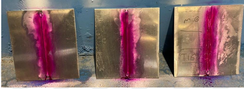
Şekil 6.2. Penetrant uygulama.
