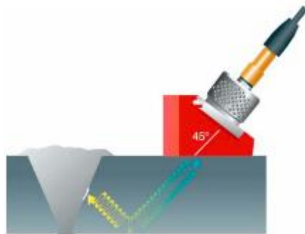
Şekil 4.6. Propla kaynaklı parçanın hata tespiti [49].
