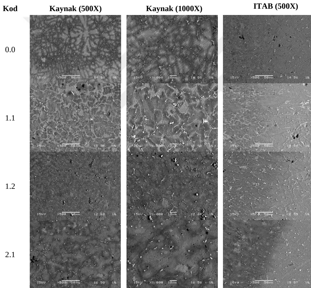
Şekil 6.12. Kaynak tamiri yapılmamış ve 3 kez tamiraty yapılmış numunelerin ITAB bölgelerinden alınan 500X büyütmedeki ve kaynak bölgelerinden alınan 500X ve 1000X büyütmedeki SEM görüntüleri.
