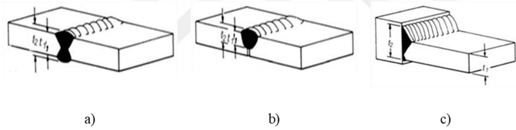
Şekil 3.22. Alın kaynağında boğaz kalınlığı: (a) tam kalem alın kaynağı, (b) kısmi alın kaynağı, (c) T-alın kaynağı [30].
