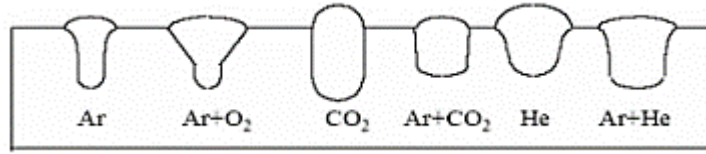
Şekil 3.19. Farklı gazların ve karışımlarının kaynak dikişi ve nüfuziyete etkisi [29].
