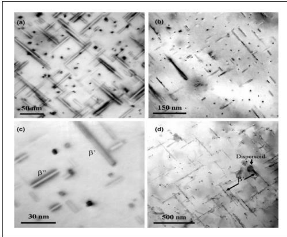
řekil 2.5. (a), (c) \beta'' (iğne řeklinde) ve (b), (d) \beta' (çubuk řeklinde) çökeltilerini gösteren transmisyon elektron mikroskop görüntüsü [18].
