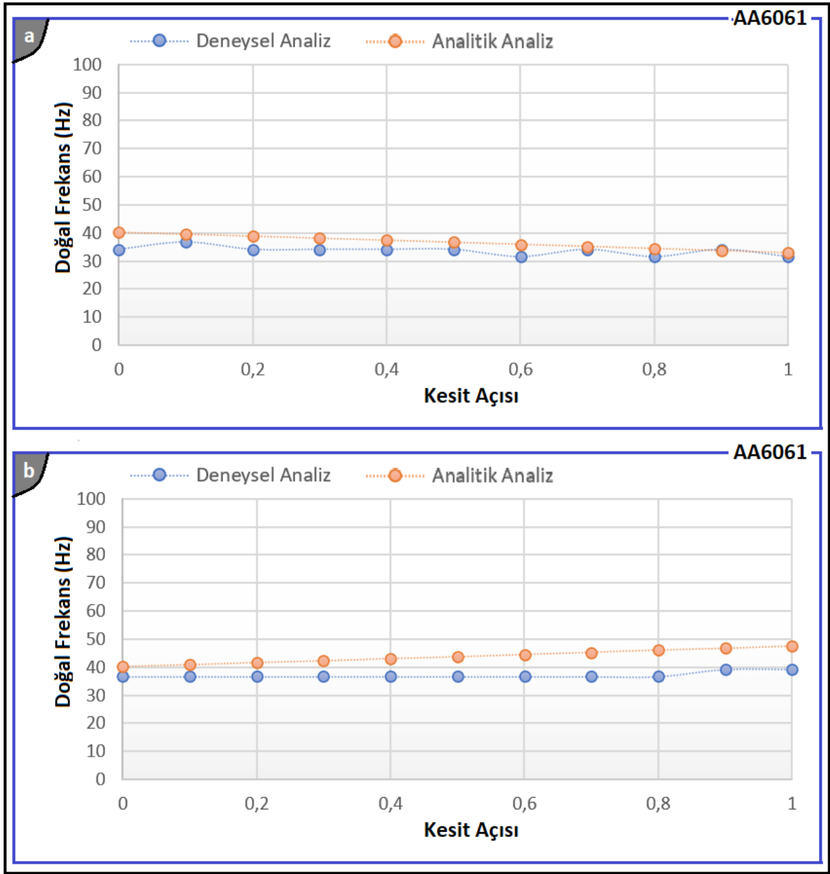
Şekil 5.7: AA6061 Al alaşım serisine ait sığ-kriyojenik soğutma ve ısıt işlem sonrası deneysel ve analitik doğal frekans değerleri, a) Kısa kenar sabit uzun kenar serbest numune serisi, b) Uzun kenar sabit kısa kenar serbest numune serisi.
