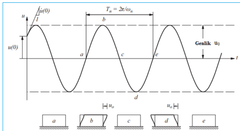
Şekil 3.1: Sönümsüz bir sistemin serbest titreşiminin yer değişimi-zaman eğrisini şematik gösterimi (Dagdelen ve Ruhani 2018).
