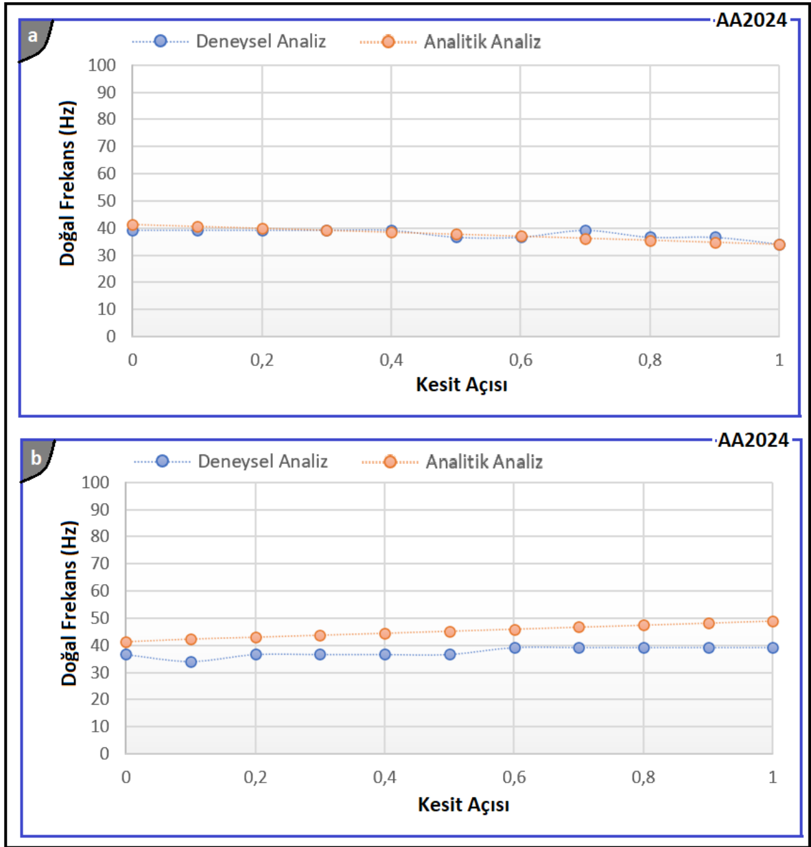
Şekil 5.6: AA2024 Al alaşım serisine ait sıg-kriyojenik soğutma ve ısıt işlem sonrası deneysel ve analitik doğal frekans değerleri, a) Kısa kenar sabit uzun kenar serbest numune serisi, b) Uzun kenar sabit kısa kenar serbest numune serisi.
