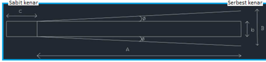
Şekil 4.15: 1. Seri test numunesinin ankastre test düzeneğine bağlanma konumu.
