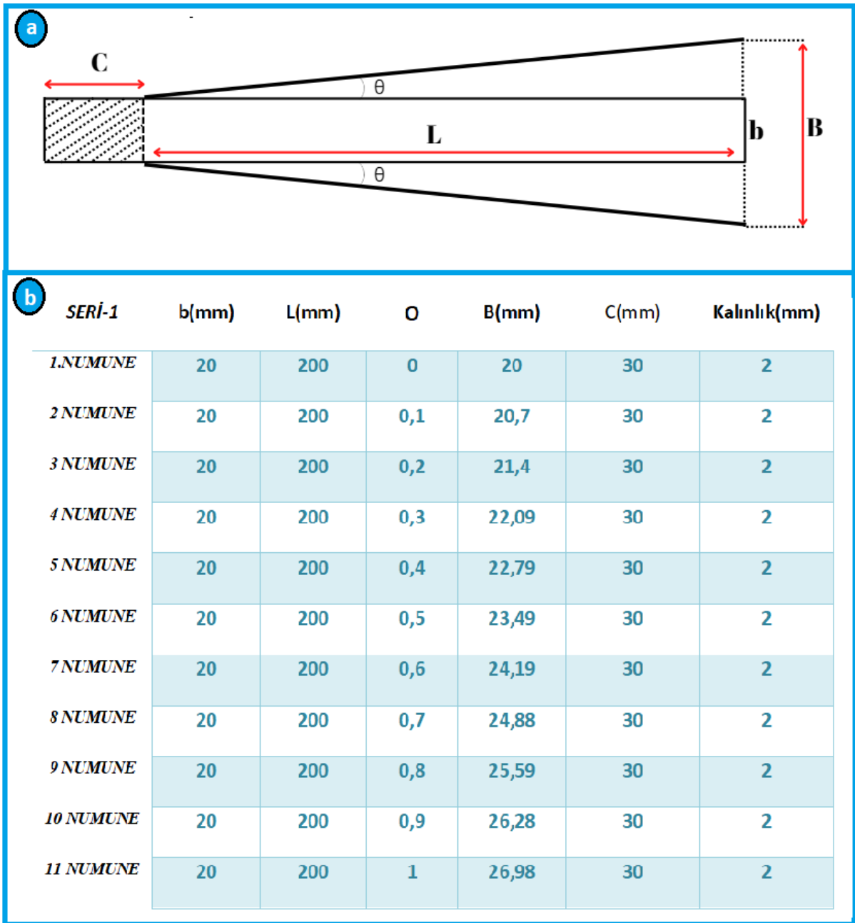
Şekil 4.4: Dar kenar test numune serisi, a) Numune şematik gösterimi, b) Numune boyut bilgisi.
