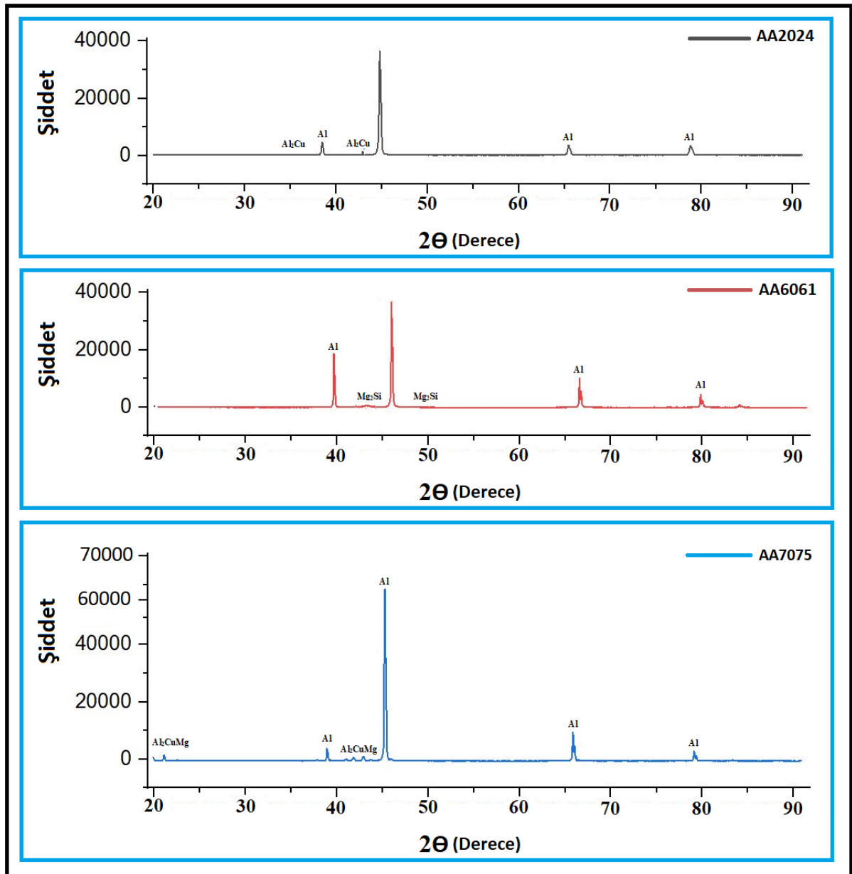
Şekil 5.13: AA2024, AA6061 ve AA7075 Al alaşım serilerine uygulanan çözündürme + su verme + sığ- kriyojenik ve yaşlandırma ısıt işlemleri sonrası XRD analiz verileri.
