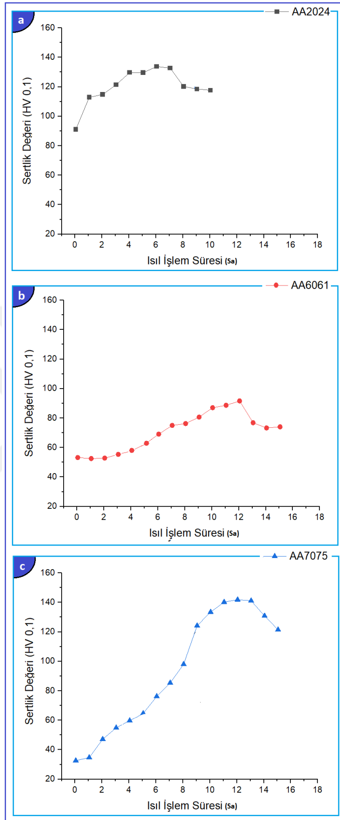
Şekil 5.1: Al alaşımlarına uygulanan ısıt işlem sonrası sertlik değerleri, a) AA2024 Al alaşıma ait sertlik değerleri, b) AA6061 Alaşıma ait sertlik değeri, c) AA7075 Al alaşıma ait sertlik değeri.
