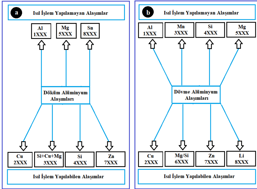
Şekil 2.7: Al alaşımları ısıtılabilirlik özellikleri a) Dövme Al alaşımlarında ısıtılabilirlik özellikleri, b) Dökme Al alaşımlarında ısıtılabilirlik özellikleri.
