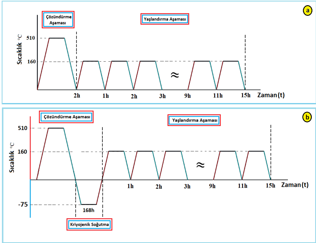
Şekil 4.7: AA2024, AA6061 ve AA7075 Al alaşımlarına uygulanan ısıtım işlem basamakları, (a) Çözündürme sonrası yaşlandırma işlemi, (b) Çözündürme sonrası sıf-kriyojenik soğutma ve yaşlandırma ısıtım işlem basamakları.
