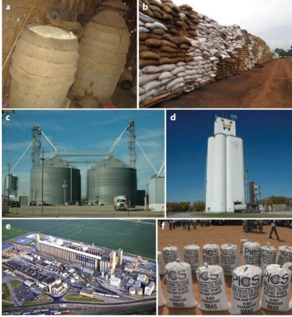
Şekil 1.1 Çeşitli Depolama Sistemleri. (a) Afrikalı Küçük Toprak Sahipleri Tarafından Kullanılan ve "gota" Olarak Adlandırılan Kerpiç Kaplar; (b) Dış Mekan Çuval İstifleri; (c) Havalandırılmalı ve Fumigant Devridaimli Çelik Depolar; (d) Beton Elevatör (Asansör); (e) İşleme ve Nakliye ile Birlikte Büyük Beton Asansör Sistemi; ve (f) Hermetik (Hava Geçirmez) Küçük Torba Saklama Yöntemi (Hagstrum ve Phillips, 2017)
