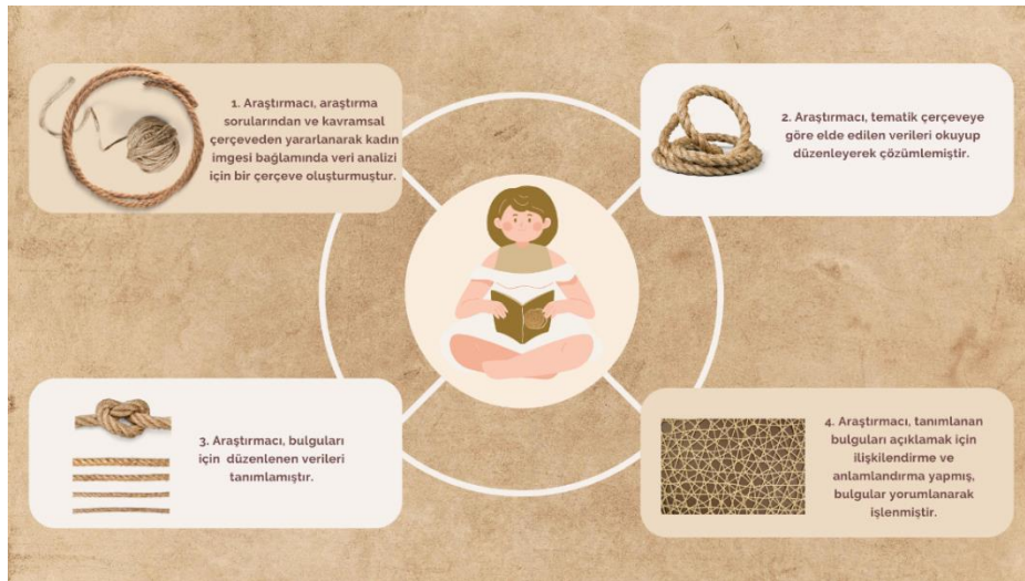
Şekil 3.3. Betimsel analize uygun analiz sürecinin ikonografik görüntüsü
