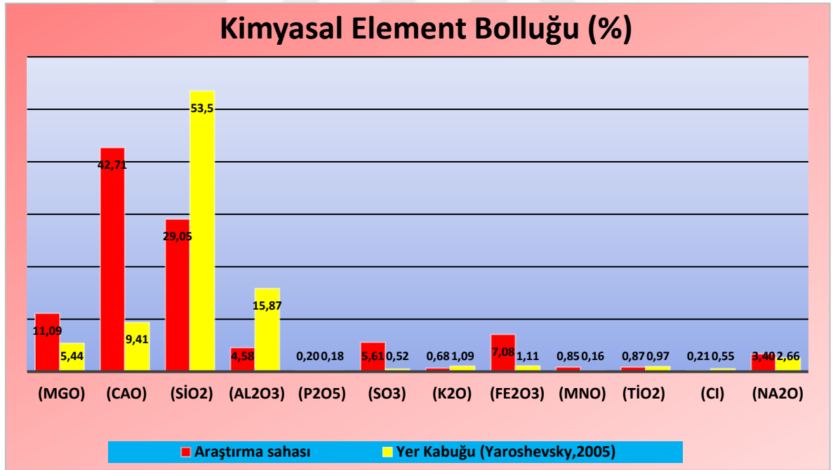
Grafik 21. Çalışma Sahasının Kımyasal Element Bollluğu
