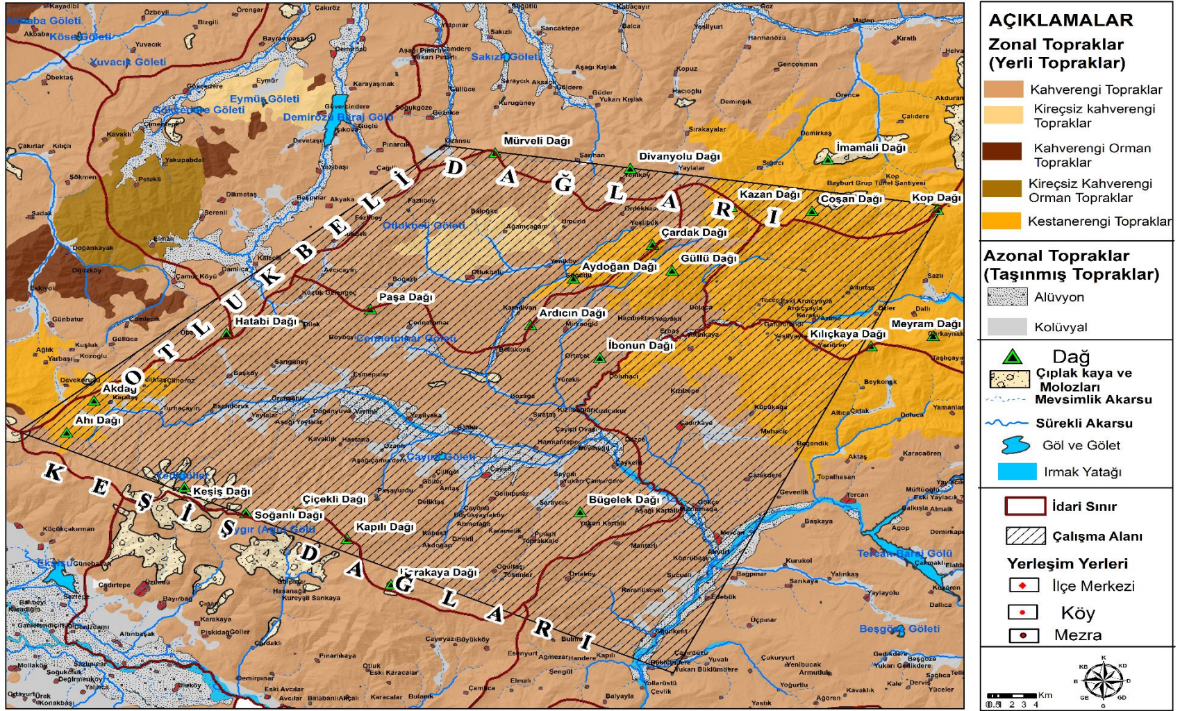
Harita 14. Çalışma Sahasının Toprak Haritası
