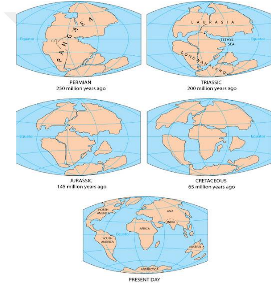
Şekil 4. Jeolojik Zamanlarda Oluşan Kıtalar (Url 3)
