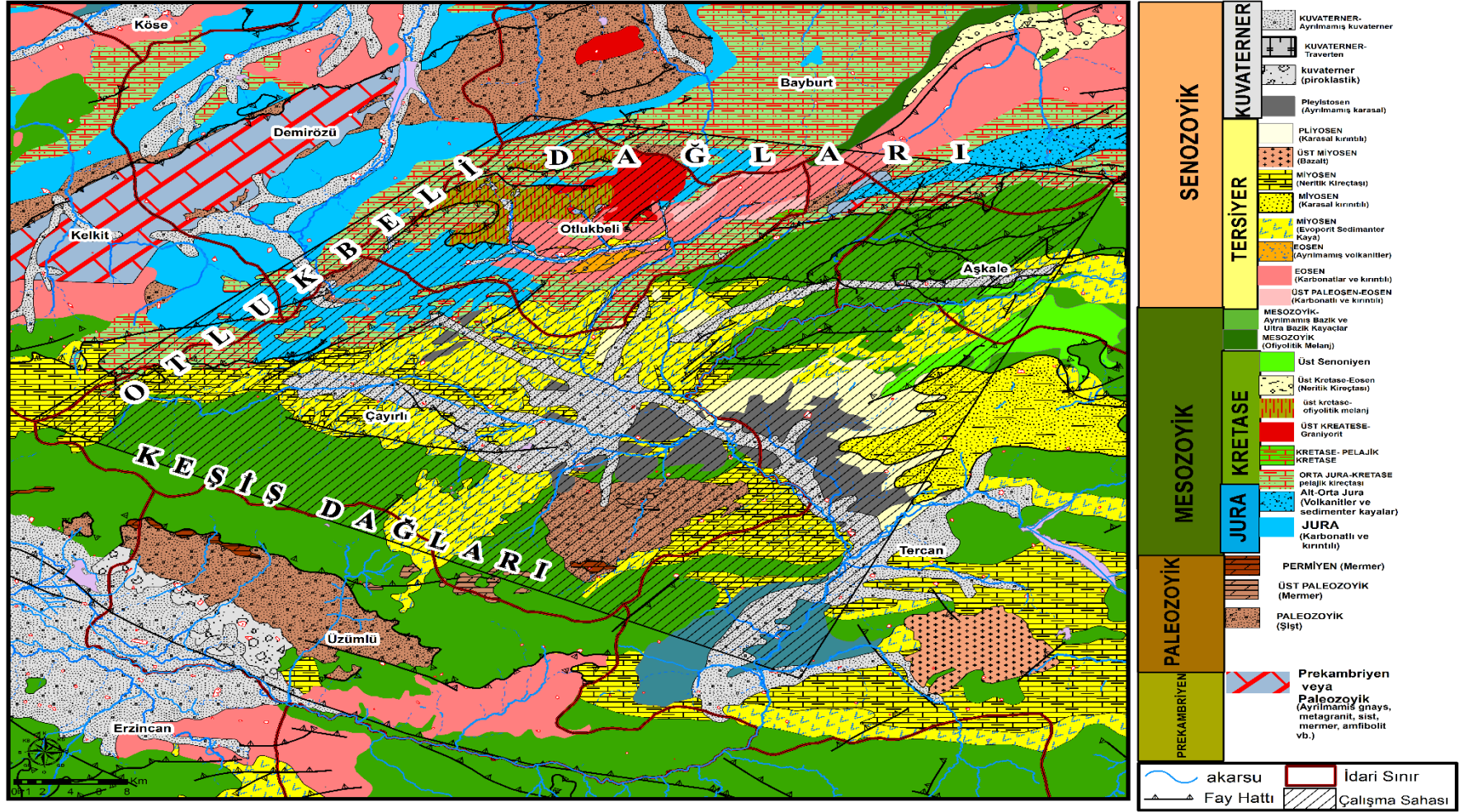
Harita 2. Çalışma Sahasının Jeoloji Haritası
