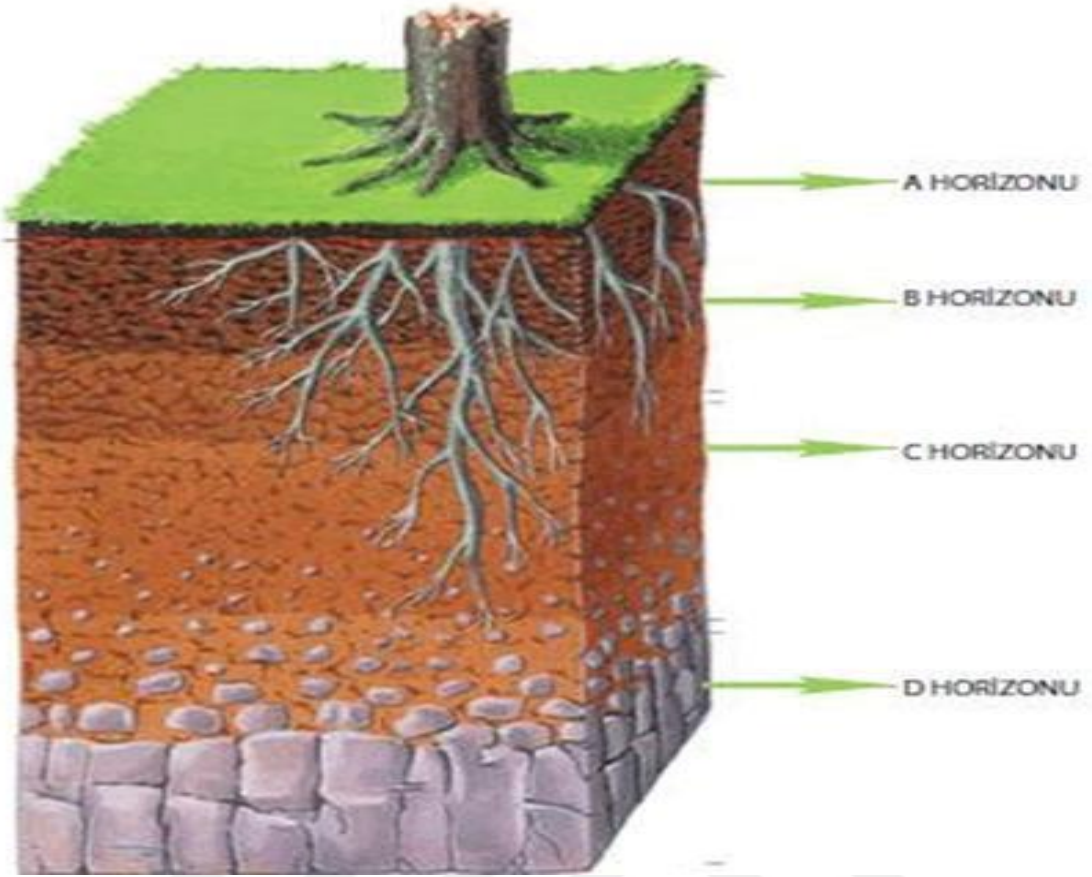
Şekil 2: Anakaya ve ana materyal üzerinde toprak oluşumu
