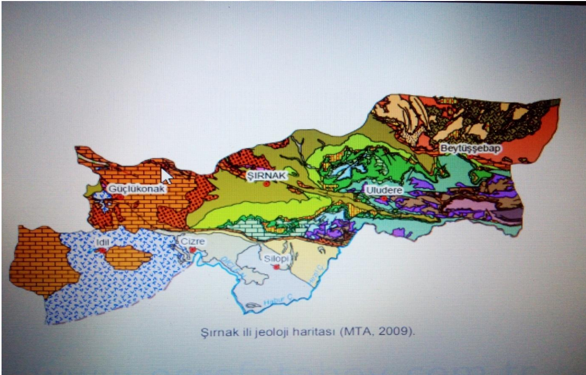
Şekil 1: Şırnak ilinin jeolojik haritası (Irmak vd., 2021: 366)
