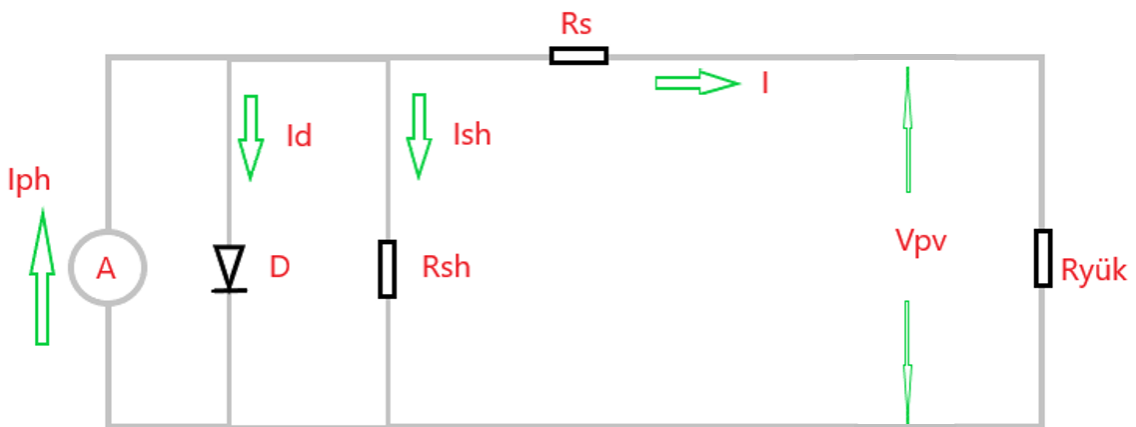
Şekil 2.4. Eşdeğer devre modeli
