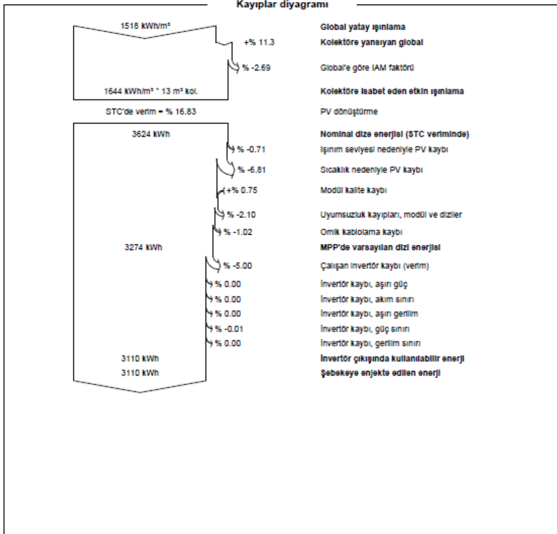
Şekil 4.36. Kayıp diyagramı
