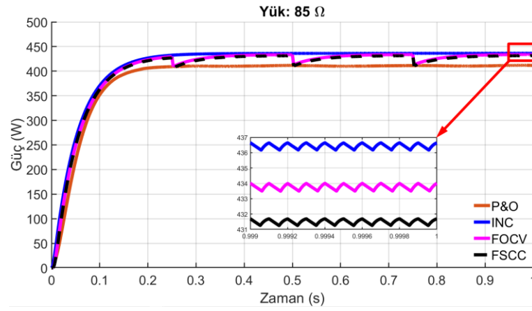
Şekil 4.5.8 T_C = 30^\circ\text{C} , T_H = 200^\circ\text{C} , R_L = 85 \Omega
