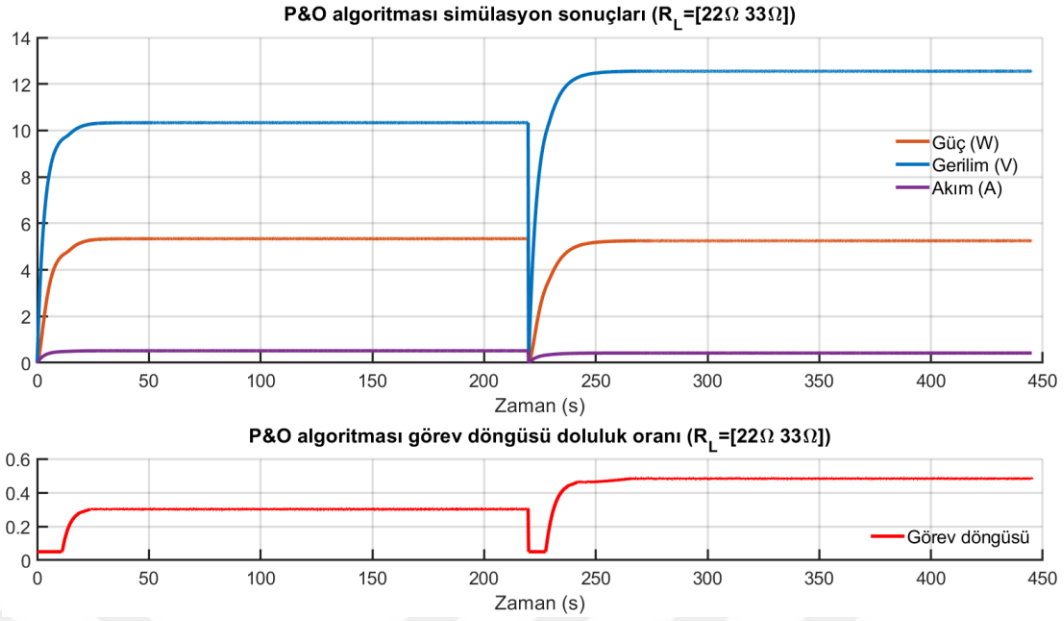
Şekil 4.14. P&O algoritması simülasyon sonuçları grafikleri
