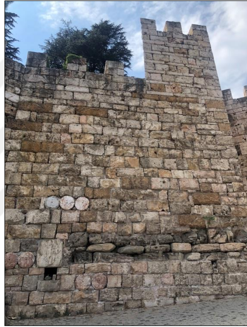
Şekil 43. Saltanat Kapı çevresindeki surlardaki orijinal olan ve olmayan taşlar
