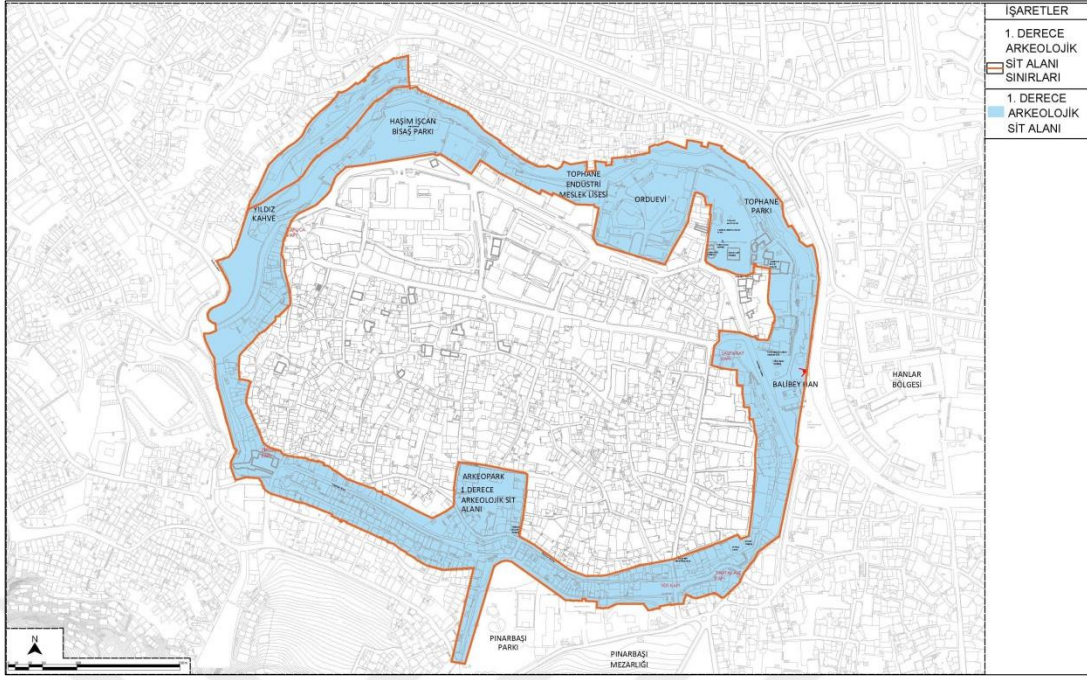
Şekil 30. Hisar Bölgesi I. Derece Arkeolojik Sit Alanı Haritası
