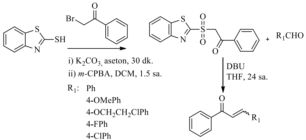
Şekil 2.22. Julia-Kocienski olefinasyonu ile kalkon sentezi.
