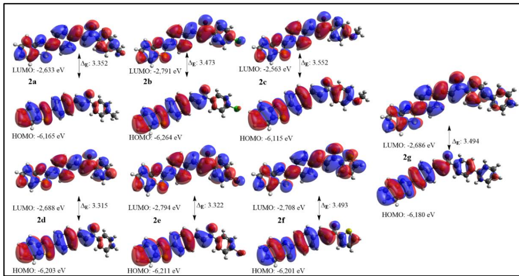
Şekil 4.9. Benzotriyazol kalkon (2a-g) HOMO-LUMO orbital diyagramı.
