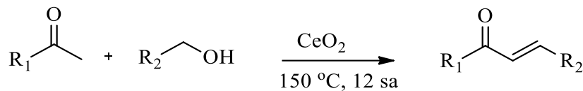
Şekil 2.15. Kalkon bileşiklerinin \text{CeO}_2 katalizli oksidatif sentezi.
