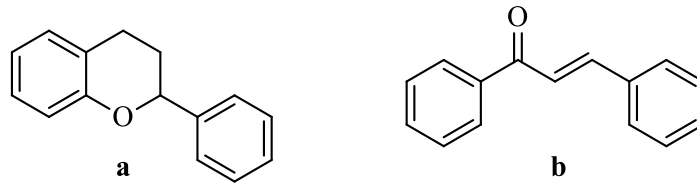
Şekil 1.2. Flavon (a) ve kalkonun (b) genel kimyasal formülü.
