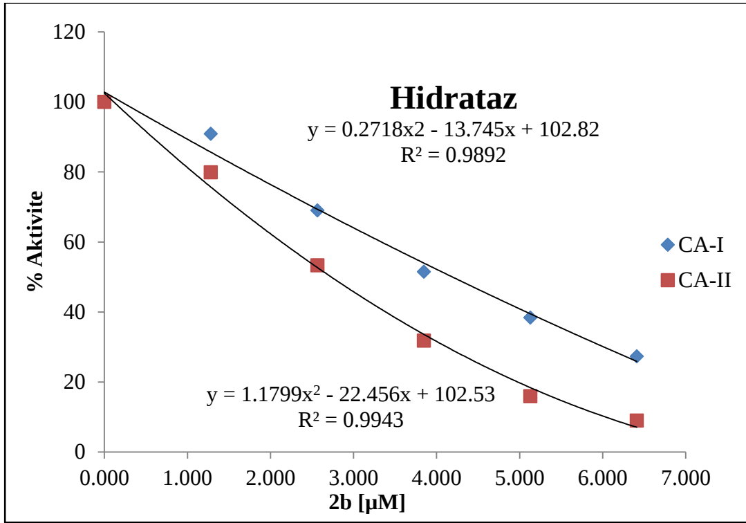
Şekil C.3. 2b'nin hCA-I, hCA-II enzimleri üzerindeki inhibisyon eğrisi (Hidrataz).
