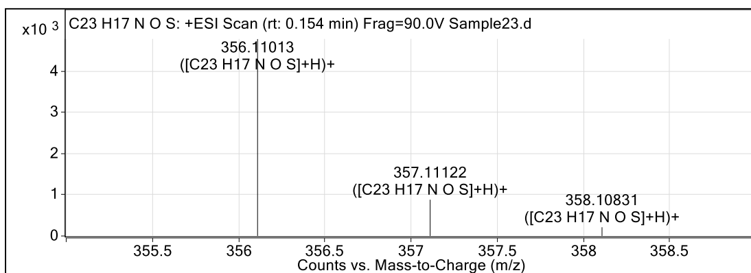
Şekil A.4. 2a bileşiğinin HRMS spektrumu.
