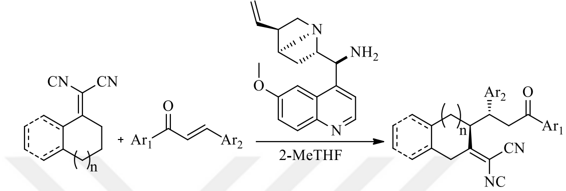
Şekil 2.26. \alpha,\alpha -Disiyanoolefinlerin kalkon bileşiklerine asimetrik katılması.
