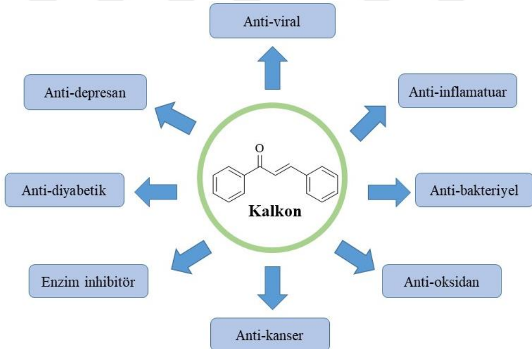
Şekil 2.39. Kalkonların genel biyolojik ve farmokolojik özellikleri.
