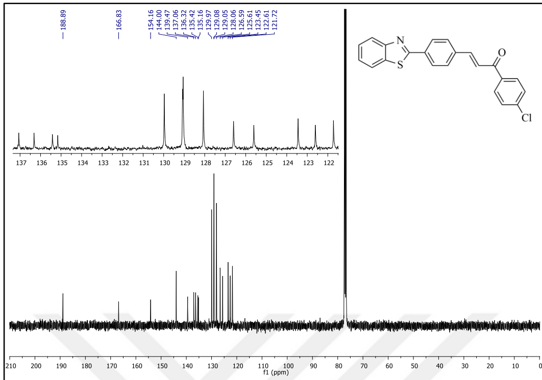
Şekil 4.5. 2b bileşiğine ait ^{13}\text{C} -NMR spektrumu.
