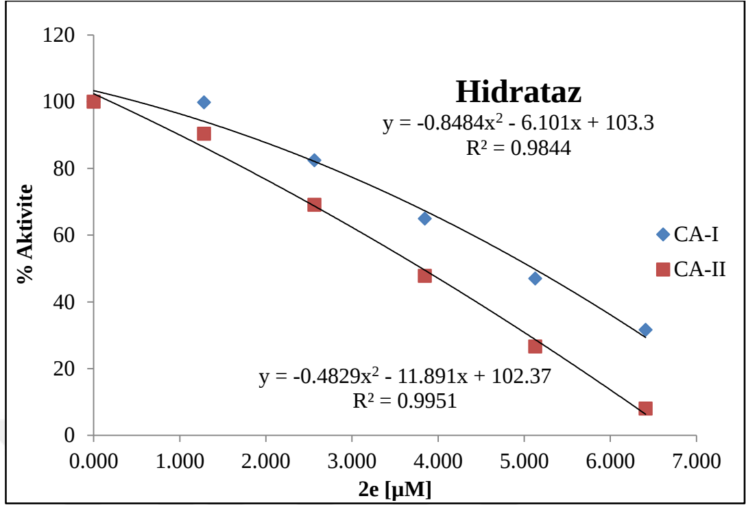
Şekil C.9. 2e'nin hCA-I, hCA-II enzimleri üzerindeki inhibisyon eğrisi (Hidratase).
