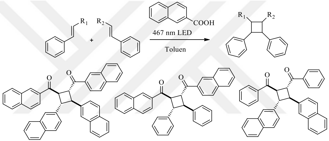
Şekil 2.35. Kalkon bileşiklerinin (2+2) siklokatılma reaksiyonu.
