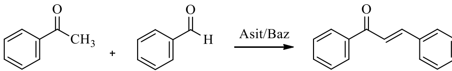
Şekil 2.3. Claisen-Schmidt kondenzasyonu.
