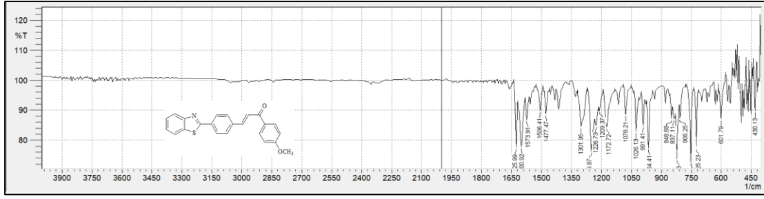
Şekil A.11. 2c bileşiğinin FT-IR spektrumu.
