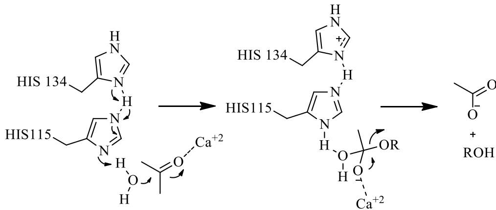
Şekil 2.79. Paraoksonaz enzimin etki mekanizması.
