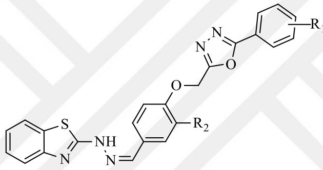
Şekil 2.67. Sentezlenen benzotiyazol bileşiklerinin genel yapısı.
