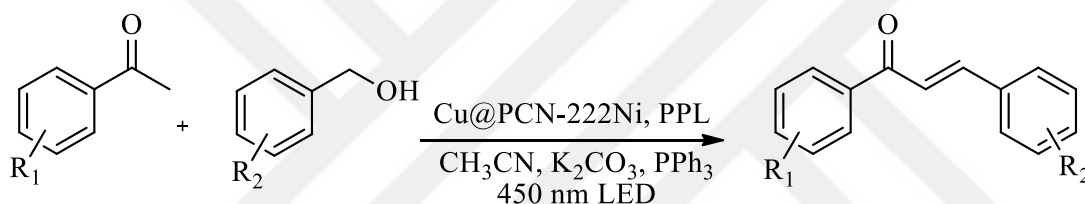
Şekil 2.16. Kalkon bileşiklerinin fotokatalitik sentezi.
