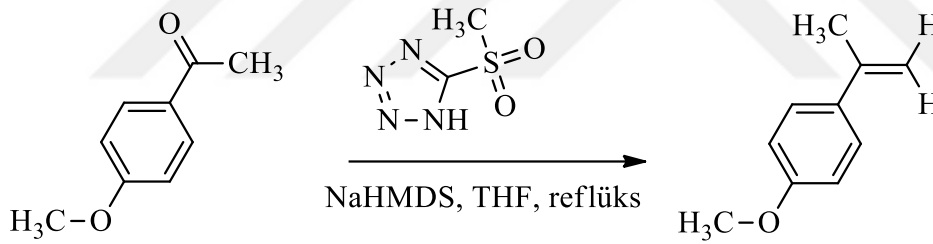
Şekil 2.21. Julia-Kocienski olefinizasyonunun şematik gösterimi.
