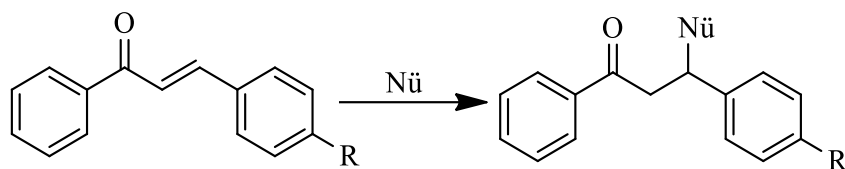
Şekil 2.23. Michael katılma reaksiyonun şematik gösterimi.
