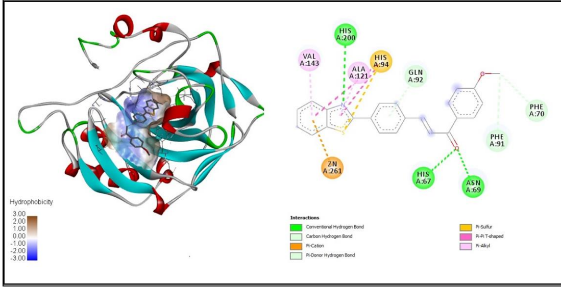
Şekil B.3. 2c'nin hCA-I 1AZM enziminin aktif bölgesindeki yerleştirme sonucu.
