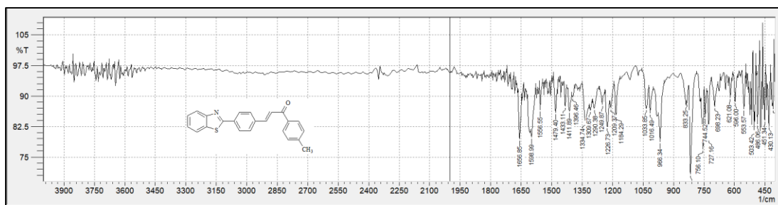
Şekil A.3. 2a bileşiğinin FT-IR spektrumu.
