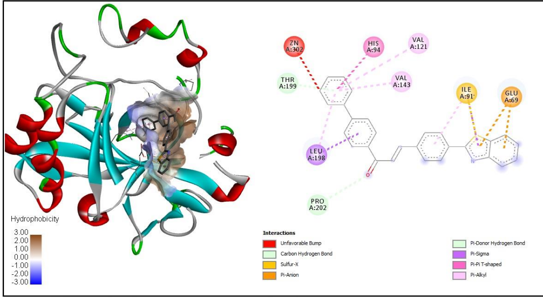
Şekil B.15. 2g'nin hCA-II 4IWZ enziminin aktif bölgesindeki yerleştirme sonucu.
