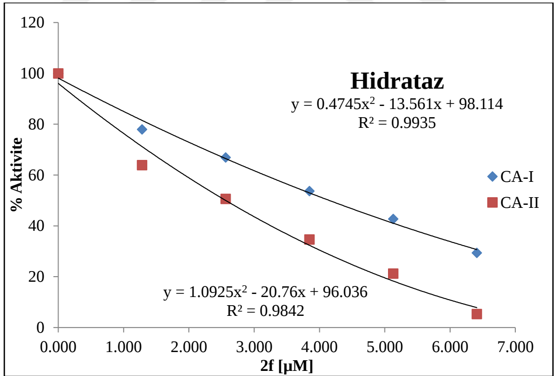
Şekil C.10. 2f'nin hCA-I, hCA-II enzimleri üzerindeki inhibisyon eğrisi (Hidratase).
