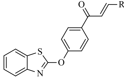
Şekil 2.61. Benzotiyazol-kalkon türevlerinin genel yapısı.
