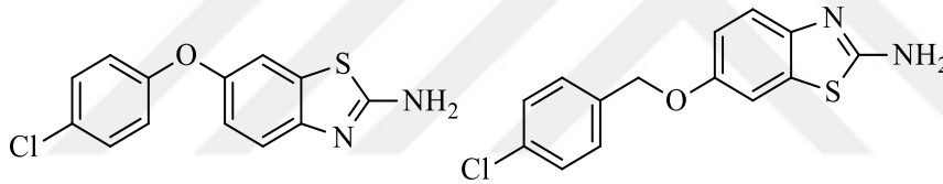
Şekil 2.63. 2-Amino-6-süstitüe benzo[d]tiyazol türevlerinin yapısı.
