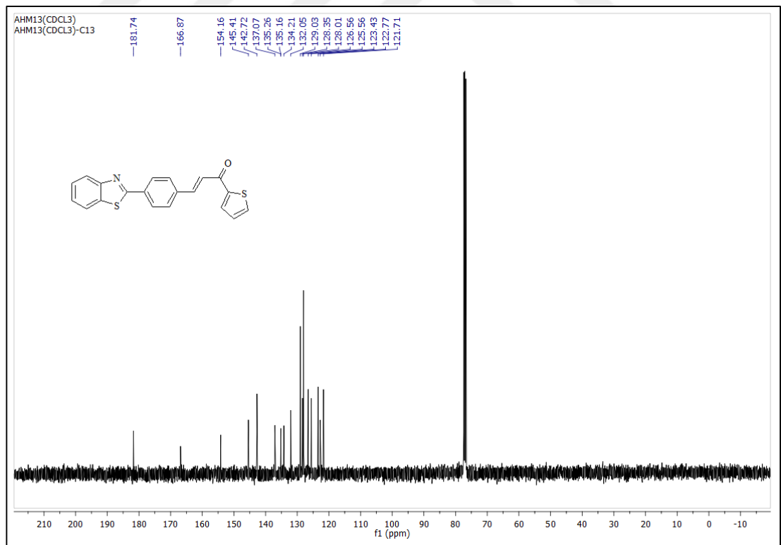
Şekil A.22. 2f bileşiğinin 13 C-NMR spektrumu (100 MHz, CDCl 3 ).
