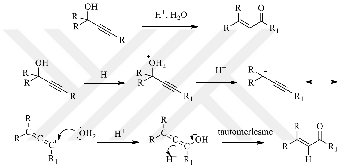
Şekil 2.14. Meyer-Schuster düzenlenmesinin mekanizması.
