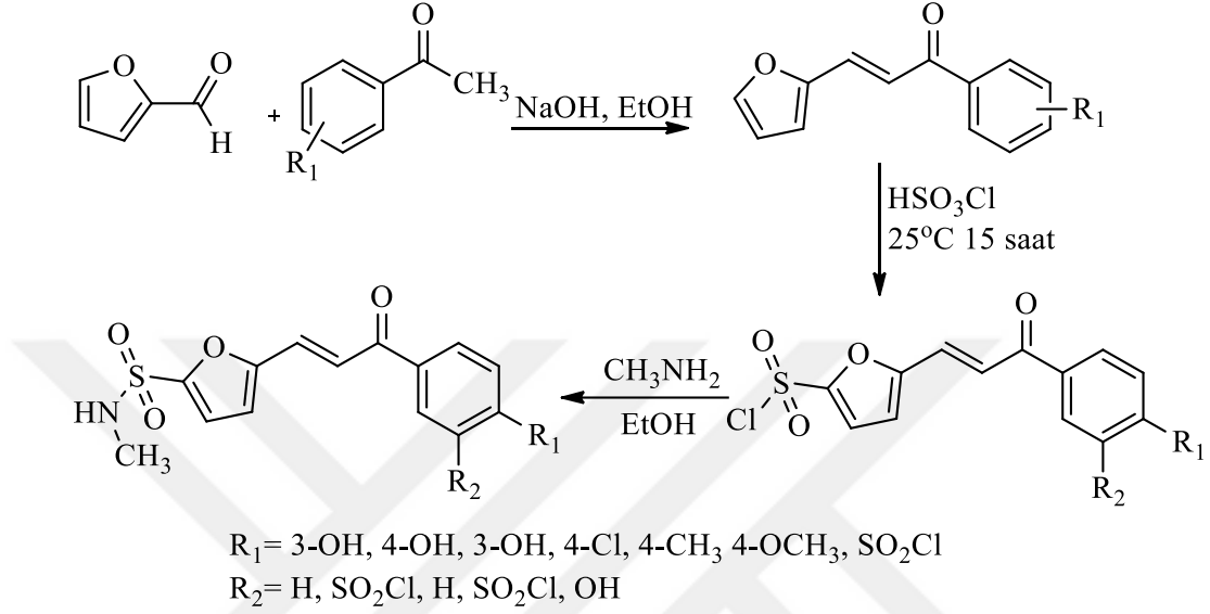
Şekil 2.46. Furfuril-kalkon türevlerinin sentezi.
