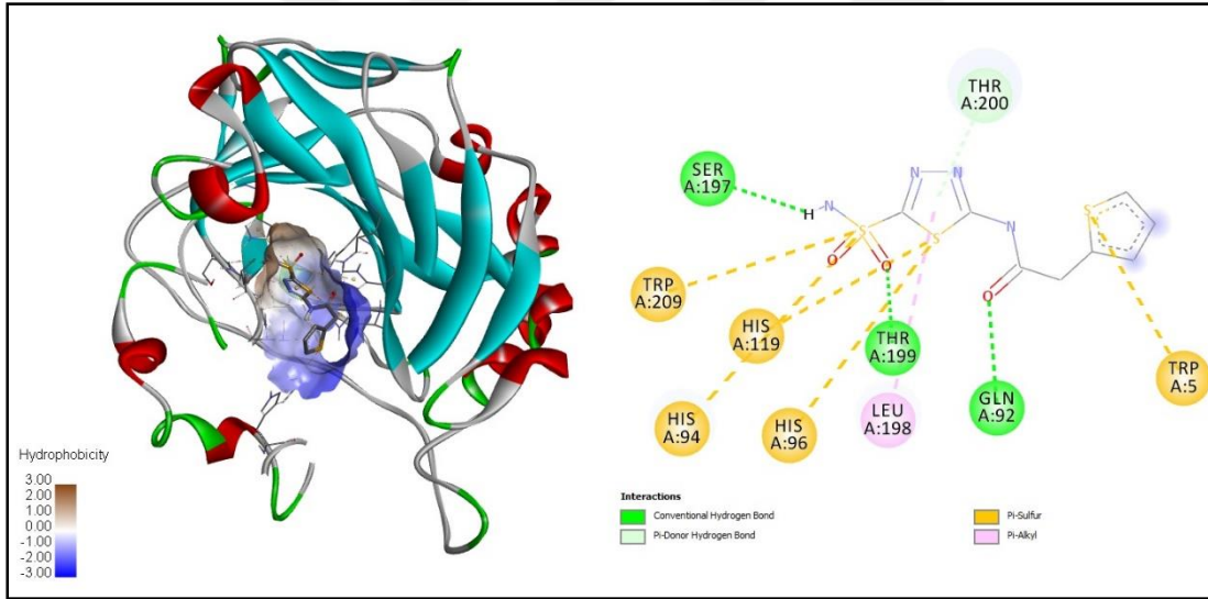
Şekil B.14. Kontrol bileşiğinin hCA-II 4IWZ enziminin aktif bölgesindeki yerleştirme sonucu.
