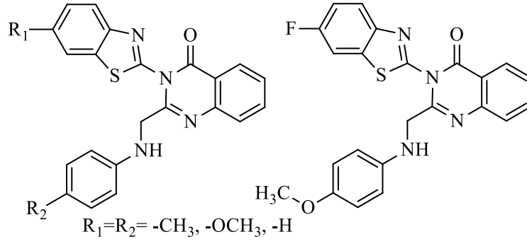
Şekil 2.64. Kinazolin ve benzotiyazol grupları içeren türevlerin genel yapısı.
