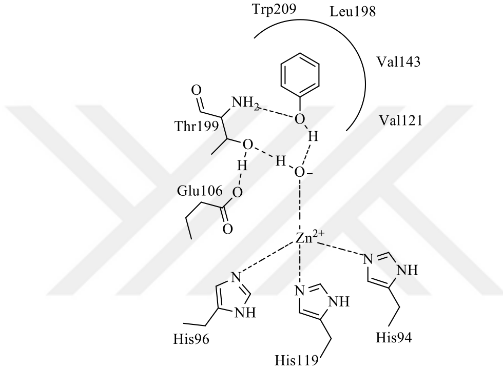
Şekil 2.73. Karbonik anhidraz enziminin aktif bölgesi.
