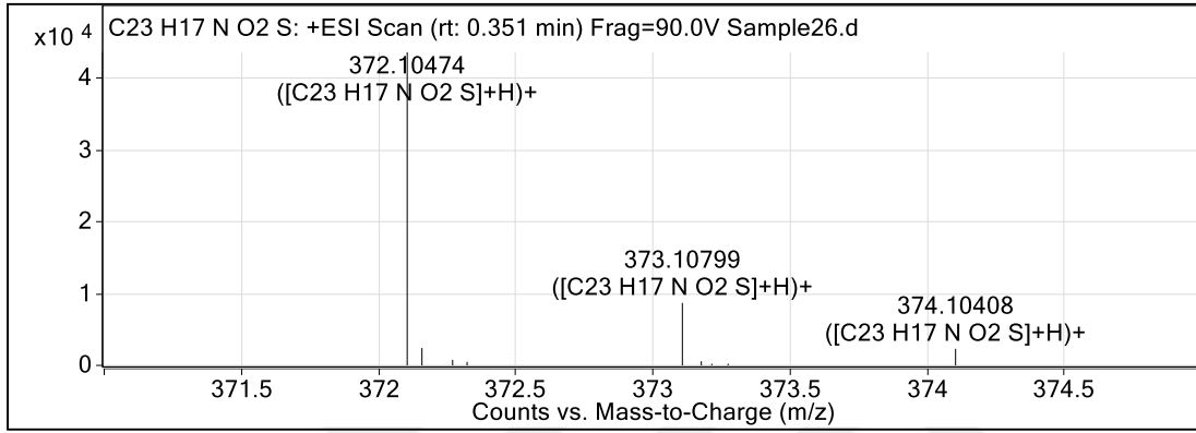
Şekil A.12. 2c bileşiğinin HRMS spektrumu.
