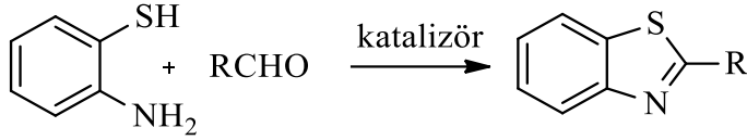
Şekil 2.50. 2-Aminotiyofenol ve aldehit bileşiklerinden benzotiyazol sentezi
