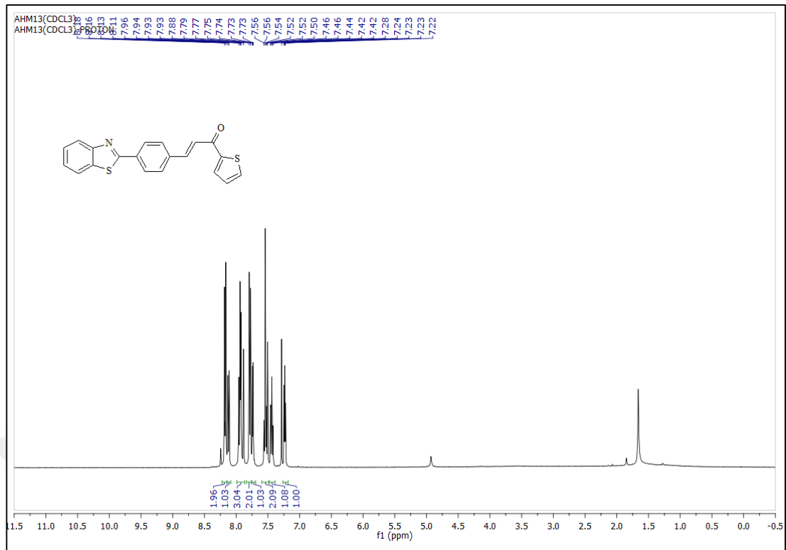
Şekil A.21. 2f bileşiğinin 1 H-NMR spektrumu (400 MHz, CDCl 3 ).
