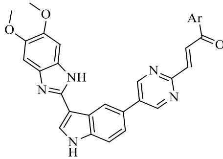
Şekil 2.43. İndol-pirimidin grubu içeren kalkon türevlerinin şematik gösterimi.
