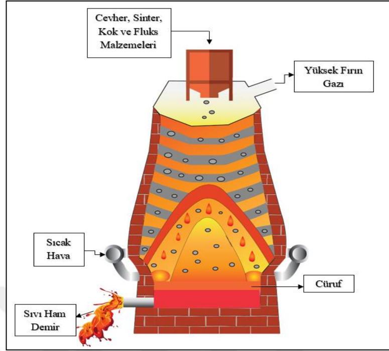
Şekil 3.7. Yüksek Fırın Çalışma Prosesi.
