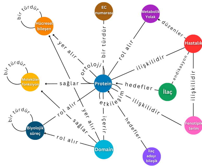
Şekil 3.1. Heterojen çizge verisinde yer alan düğüm ve kenar tipleri.
