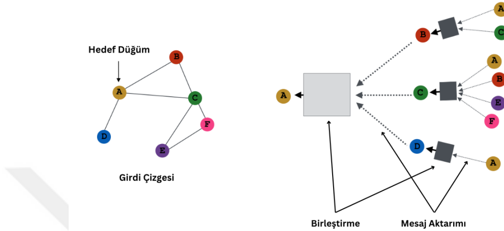
Şekil 2.4. Bir örnek çizge üzerinde A hedef düğümü için temel çizge sinir ağı operasyonlarının gösterimi (38).
