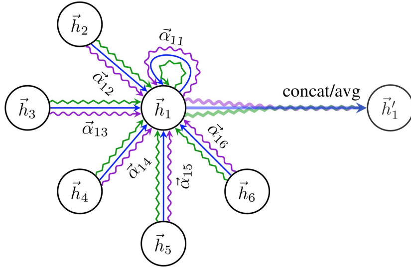
Şekil 2.5. Çizge dikkat ağlarında birleştirme adımının Düğüm 1 ve komşu düğümleri üzerinden gösterimi (40). Farklı çizgi renkleri farklı dikkat hesaplamalarını ifade etmektedir, her bir komşu düğüm için birden fazla “dikkat kafası” hesaplamak mümkündür. Bu örnekte 3 dikkat kafası mevcuttur. \bar{\alpha} , komşu düğümlerin Düğüm 1 üzerindeki önemini ifade eden öğrenilebilir ağırlıklardır. Bunlarla ağırlıklandırılmış komşu öznitelik vektörlerinin birleştirilmesi (concat/avg) sonucu Düğüm 1’in güncellenmiş öznitelik vektörü oluşur.
