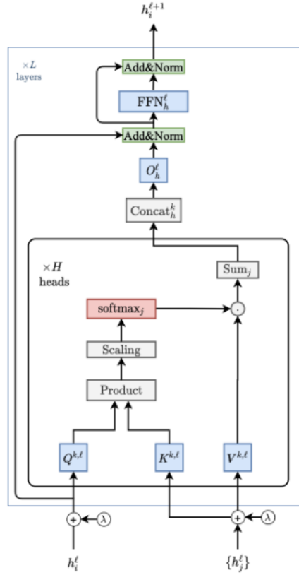
Şekil 2.6. Temel çizge dönüştürücü mimarisi gösterimi (47). \lambda , düğüm özniteliklerine ilk katmana girmeden önce eklenen pozisyonel gömme vektörleridir. h_i^l hedef düğümün, \{h_j^l\} ise komşu düğümlerin l katmanındaki gömme vektörlerini ifade eder. Hedef düğüm üzerinde komşu düğümlerin önemi üzerinden hesaplanan tüm dikkat değerleri toplanır. Her bir dikkat kafasından (“head”) çıkan değer birbirine eklenmesinin ardından bu çıktı bir tam bağlı ağdan geçirilerek hedef düğümün güncellenmiş gömmesi ( h^{l+1}_i ) elde edilir.
