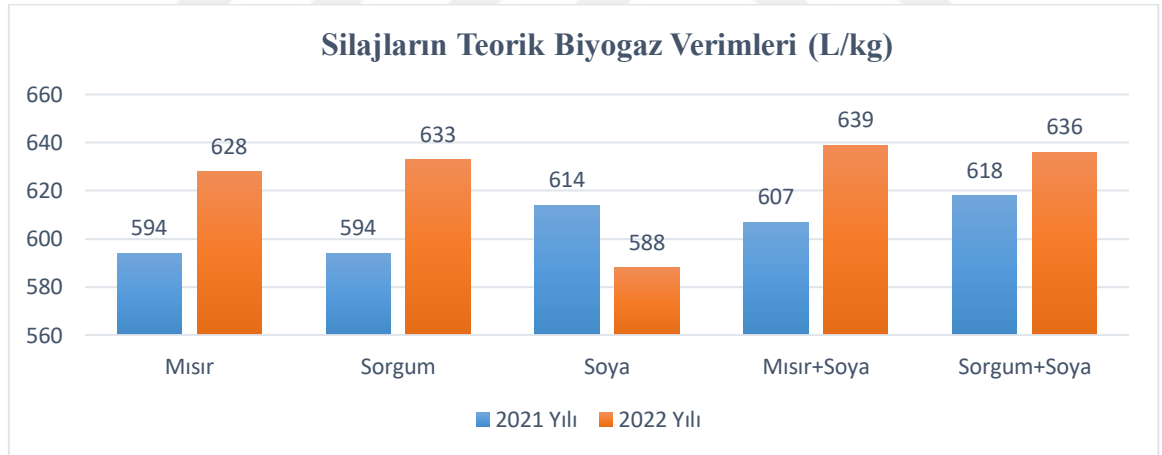
Şekil 4.25. Bitkilere ve yıllara göre silajların teorik biyogaz verimleri
