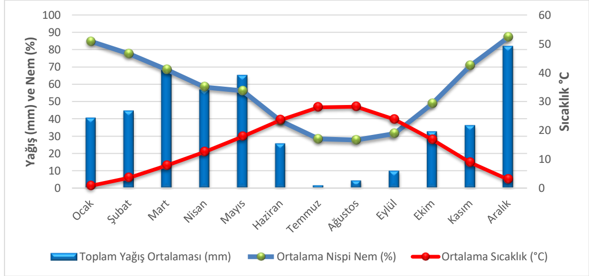
Şekil 3.2. Elâzığ ili Merkez Çöteli Köyü uzun yıllar (1939-2021) iklim verilerine ait diyagram
