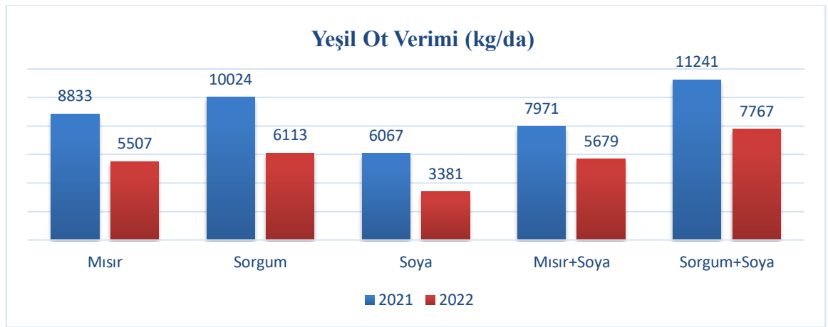
Şekil 4.1. Bitkilere ve yıllara göre elde edilen yeşil ot verimleri (kg/da)
