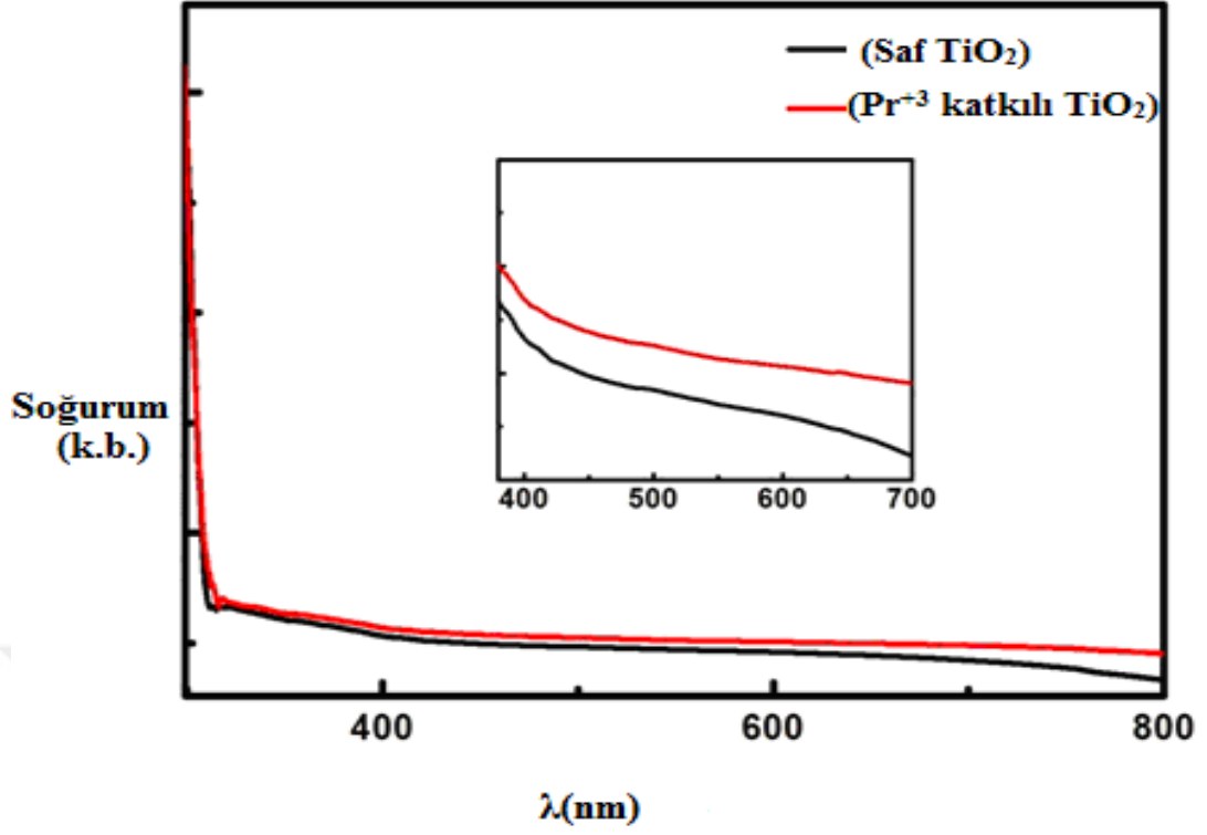
Şekil 5.5. Saf ve \text{Pr}^{+3} katkılı foto-anotların soğurma spektrumu
