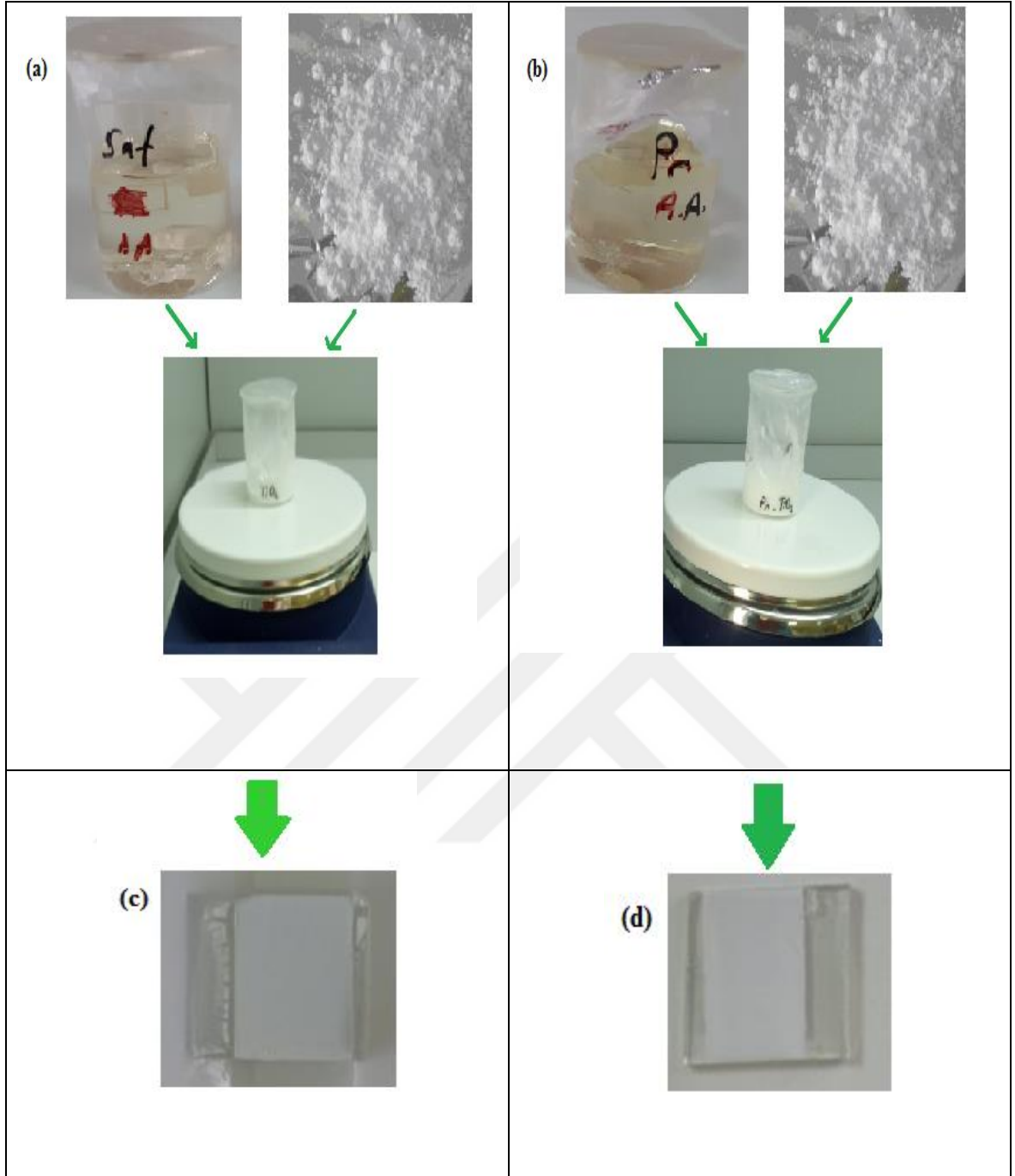
Şekil 4.3.a) Saf sentezin \text{TiO}_2 nano toz ile karıştırılması, b) \text{Pr}^{+3} katkılı sentezin \text{TiO}_2 nano toz ile karıştırılması, c) Hazırlanan saf pastaların doctor blade yöntemi ile FTO üzerinde sürülmüş hallerinin gösterimi d) \text{Pr}^{+3} katkılı pastaların doctor blade yöntemi ile FTO üzerine sürülmüş halleri
