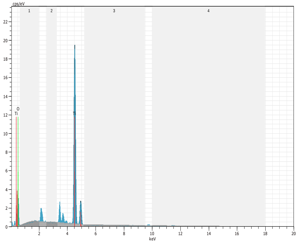
Şekil 5.2. Saf \text{TiO}_2 filmin EDX analizi
