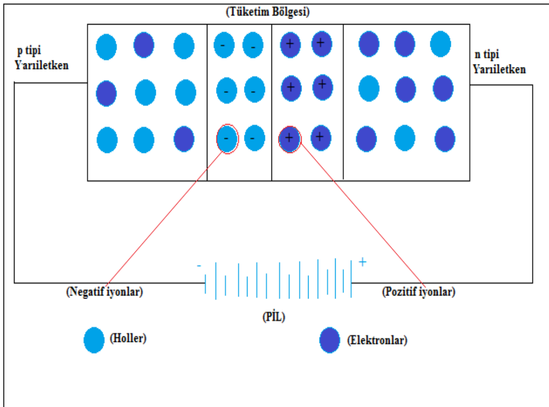
Şekil 2.3. Ters besleme durumundaki p-n eklem şematik görüntüsü
