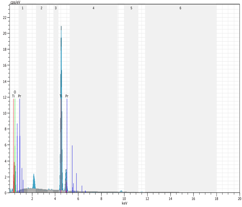
Şekil 5.3. \text{Pr}^{+3} katkılı \text{TiO}_2 filmin EDX analizi
