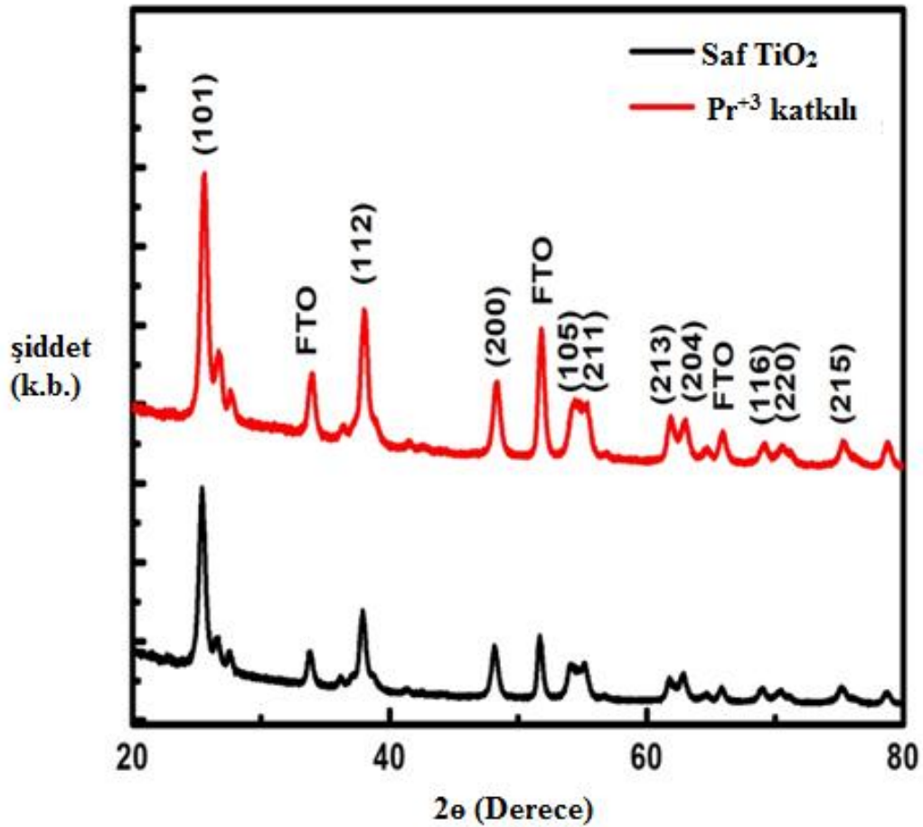
Şekil 5.1. Sol-jel yöntemi ile hazırlanan saf ve \text{Pr}^{+3} katkılı \text{TiO}_2 pastaların XRD analizi
