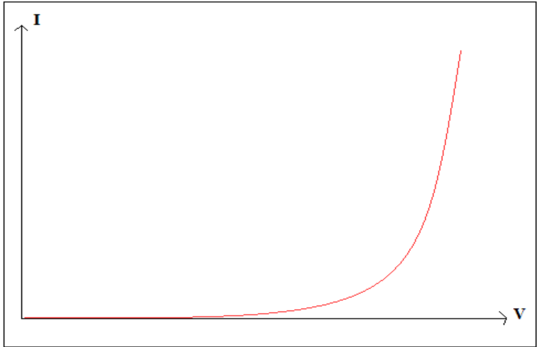
Şekil 2.6. ileri beslemede p-n eklem I-V karakteristik eğrisi
