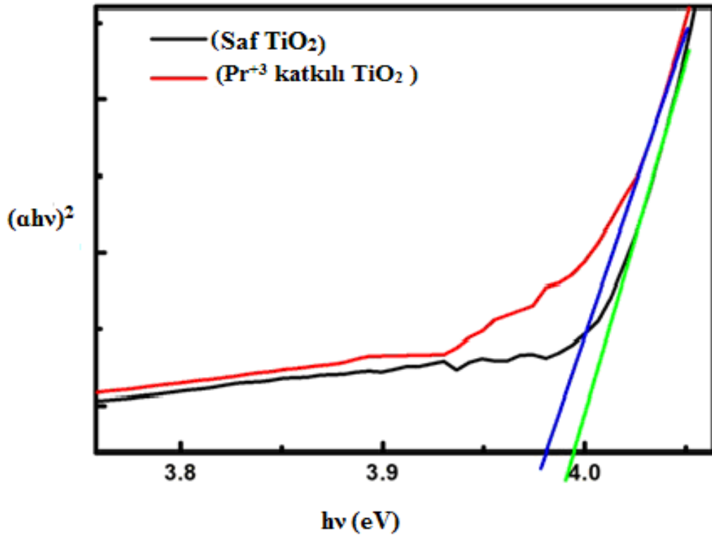
Şekil 5.6. Saf ve \text{Pr}^{+3} katkılı \text{TiO}_2 foto-anotlar için (\alpha h\nu)^2 - h\nu grafiği
