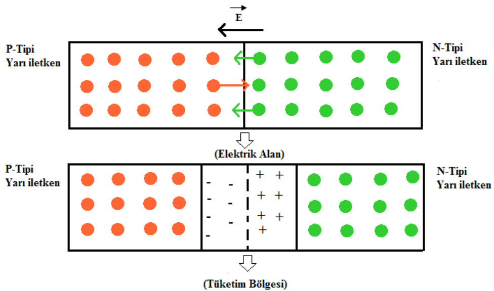
Şekil 2.2 P-n eklem tüketim bölgesi
