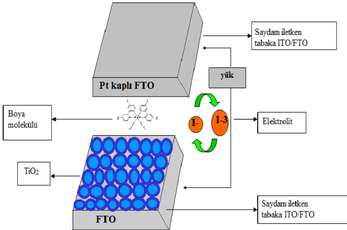
Şekil 3.1. Boya duyarlı güneş pilinin temel görüntüsü
