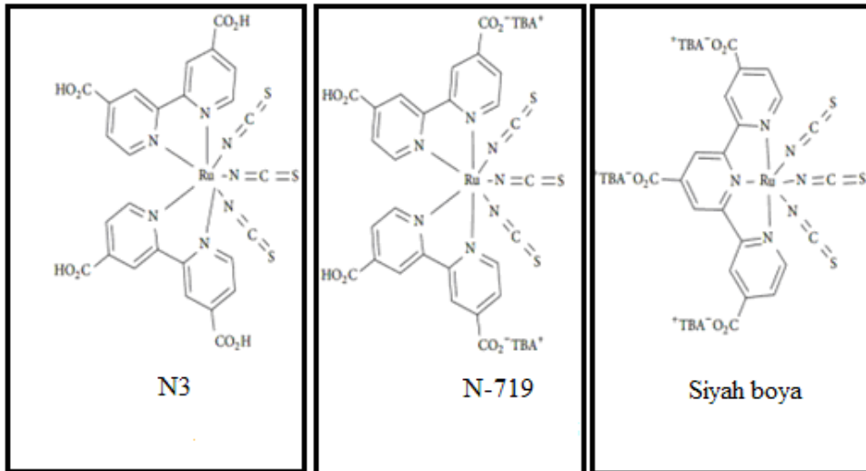
Şekil 3.3. Ru bazlı N3, N719 ve siyah boyar maddenin kimyasal yapısı
