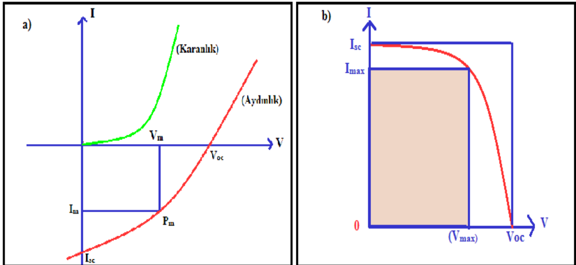
Şekil 2.8 a) Karanlıkta ve aydınlanma altında p-n eklem I-V karakteristik eğrileri, b) Güneş pillerinin bazı karakteristik parametrelerinin I-V eğrisi üzerinde gösterimi
