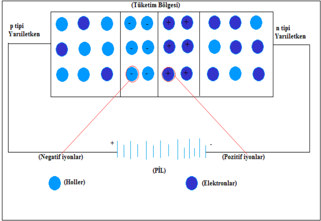
Şekil 2.5. İleri beslemede p-n eklem şematik görüntüsü
