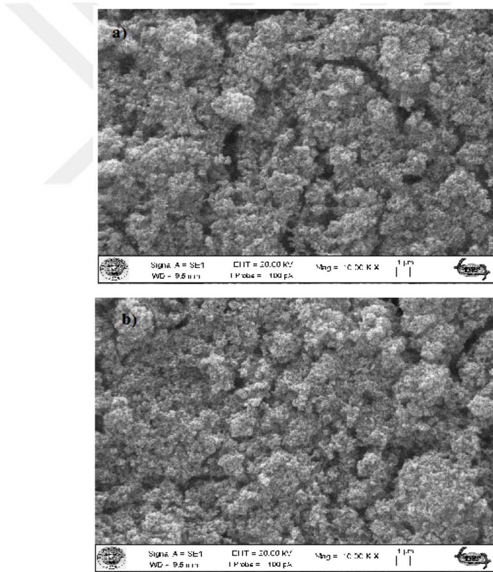
Şekil 5.4. SEM analizi, (a) Saf \text{TiO}_2 , (b) %1 (M) \text{Pr}^{+3} katkılı \text{TiO}_2 filmlerin SEM görüntüsü
