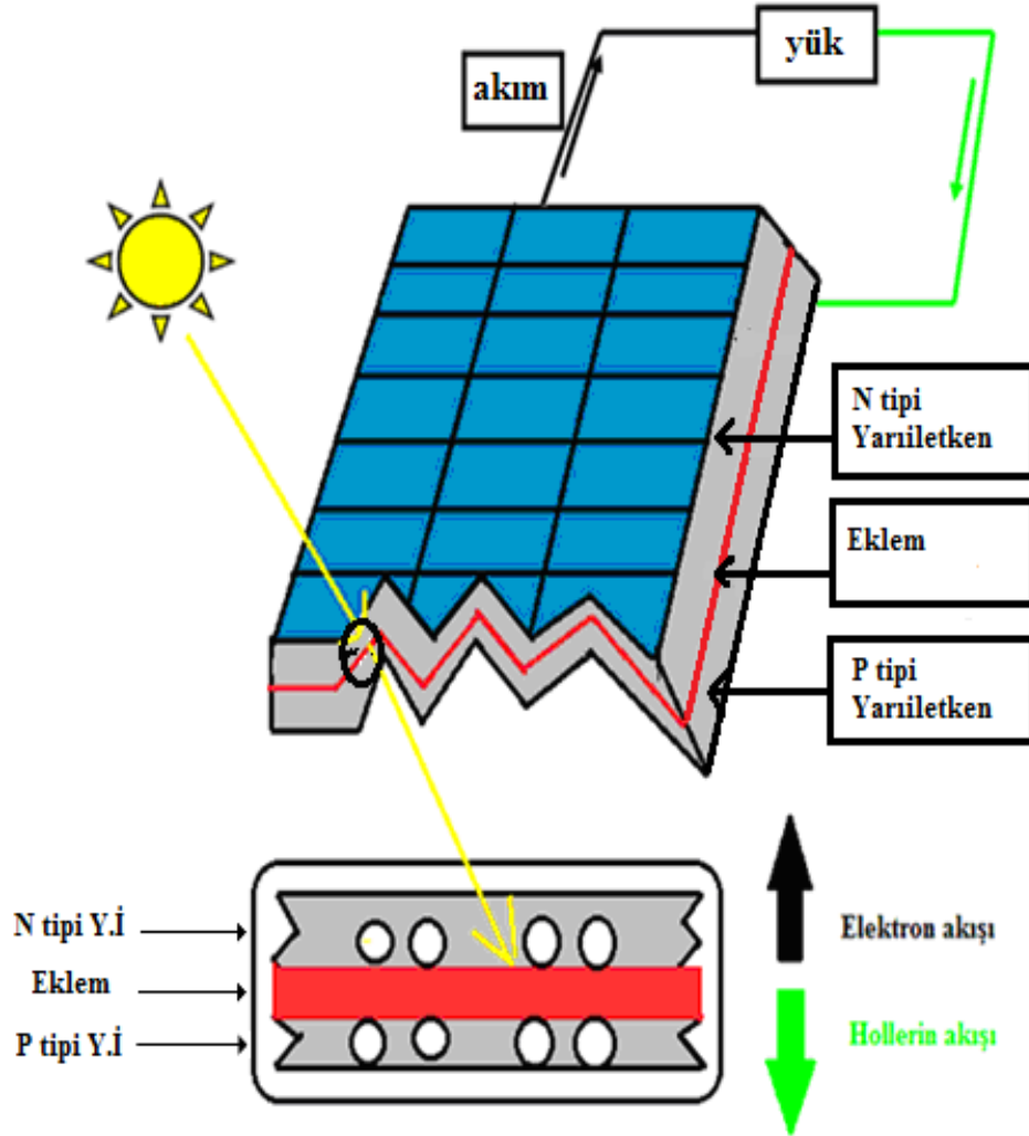
Şekil 2.7 P-n eklem aracılığıyla oluşturulmuş güneş pili
