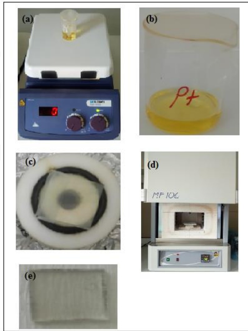
Şekil 4.4.a) Pt çözeltisi sentez aşaması, b) Sentez sonrası Pt çözeltisi, c) FTO camın Pt çözeltisiyle kaplanması, d) Pt kaplı filmlerin fırınlama aşaması, e) Fırınlama sonrası Pt kaplı foto katotlar
