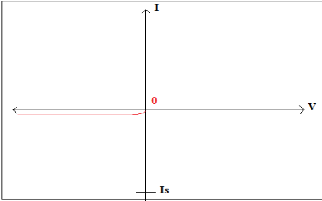
Şekil 2.4. Ters besleme durumundaki p-n eklemnin I-V karakteristiği
