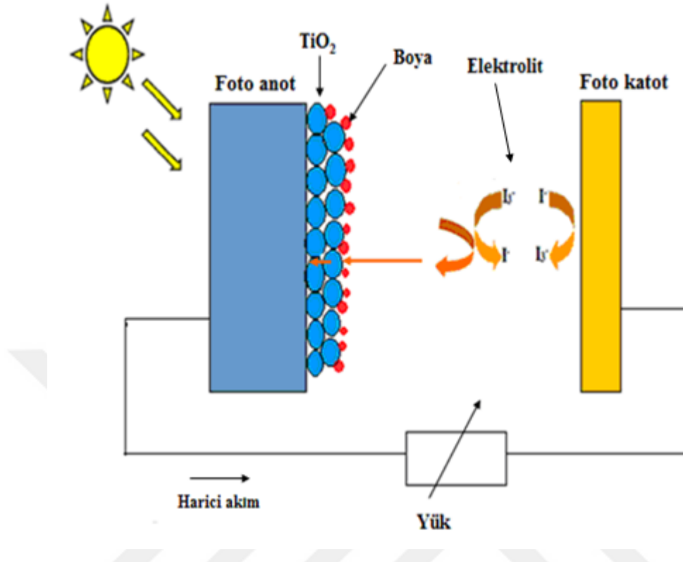
Şekil 3.4. Boya duyarlı güneş pilinin çalışma prensibi
