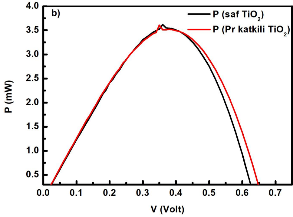
Şekil 5.7. Saf ve Pr +3 katkılı TiO 2 numunelerin a) Akım yoğunluğu (J)-(V) Voltaj eğrisi, b) Güç(P)-Voltaj(V) değişim eğrisi
