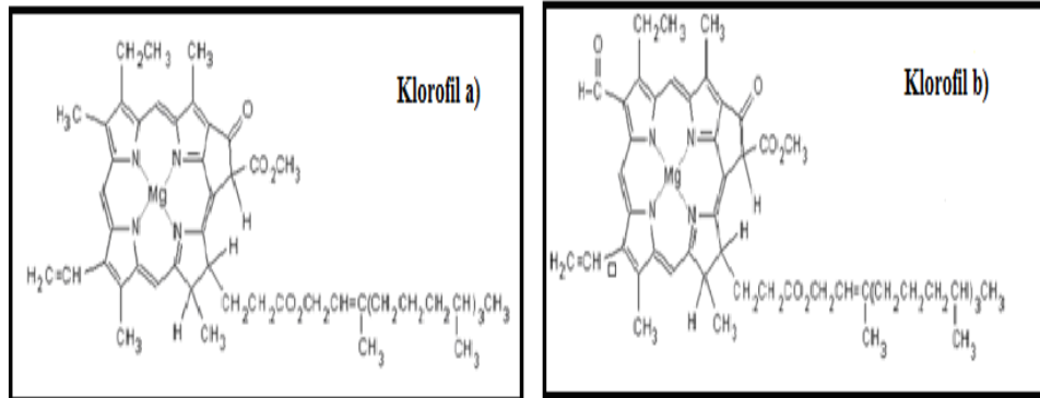
c) Klorofil a ve klorofil b'nin kimyasal yapısı
