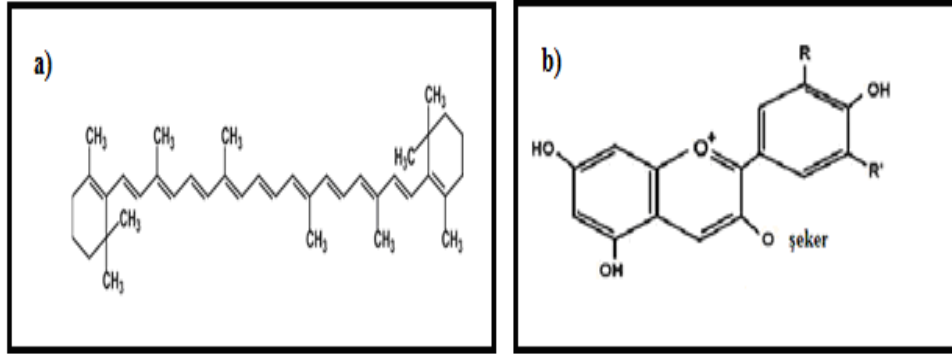
Şekil 3.2. a) Karotenoidlerin kimyasal yapısı, b) Antosiyaninlerin kimyasal yapısı,
