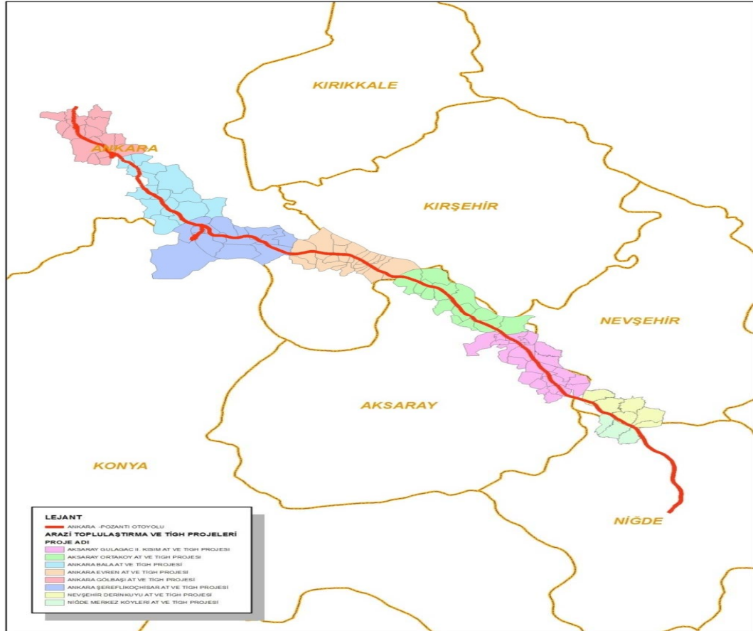
Şekil 5.1. Ankara-Niğde otoyolu güzergâhında bulunan AT projeleri.
