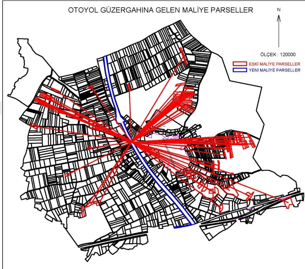
Şekil 6.4. Alayhan köyü otoyol güzergâhı üzerine gelen maliye parselleri.
