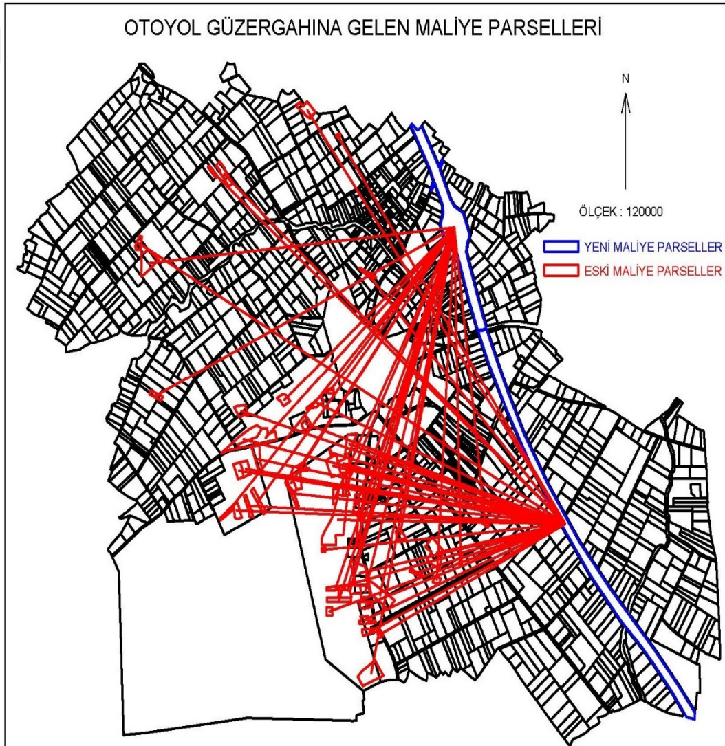
Şekil 6.5. Babakonağı köyü otoyol güzergâhı üzerine gelen maliye parselleri.
