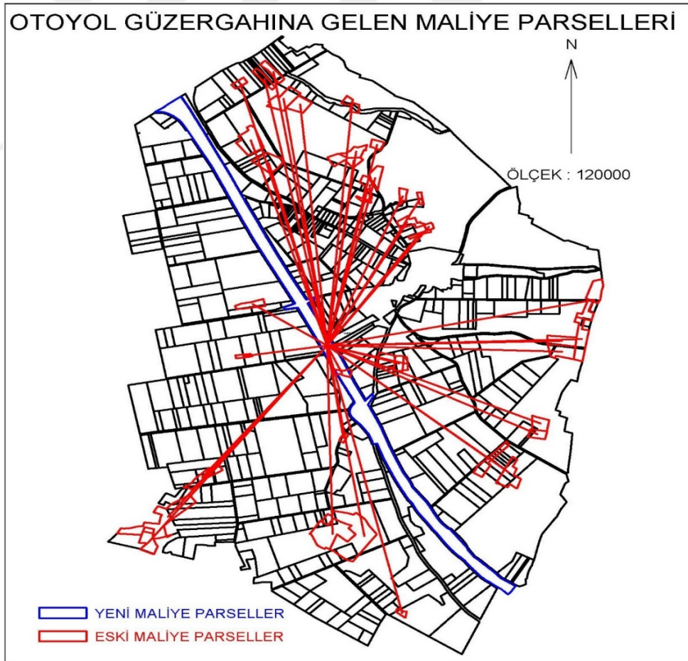
Şekil 6.8. Düğüz köyü otoyol güzergâhı üzerine gelen maliye parselleri.
