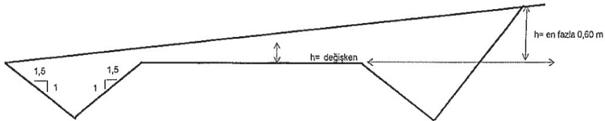
YOL KAZISI KESİTİ PLATFORM GENİŞLİĞİ 4 ve 6 m
