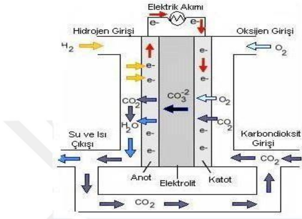
Şekil 4.7. Erimiş karbonat yapıdaki yakıt pilinin çalışma şeması (Appleby ve Foulkes, 1989)
