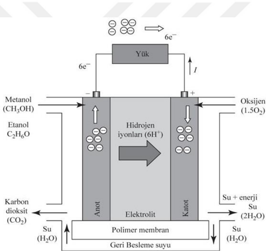
Şekil 4.4 Doğrudan Metanollü Yakıt Pili ( slideplayer.biz.tr )
