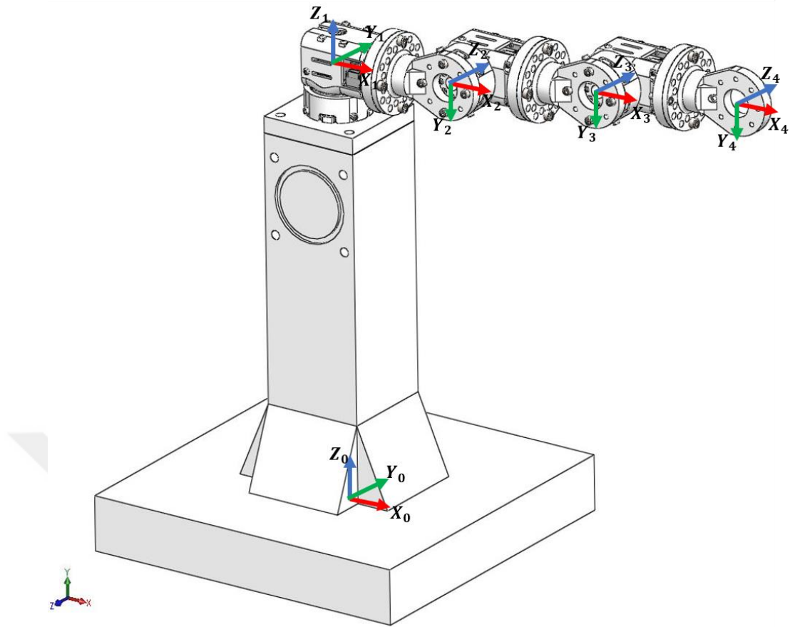
Figure 2.7 : DH coordinate frames.
