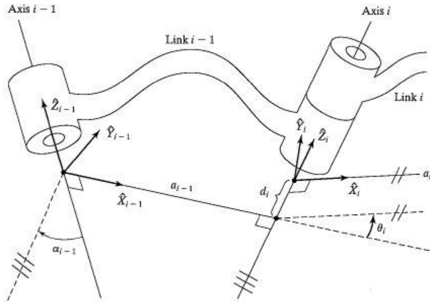
Figure 2.6 : DH convention [28].
