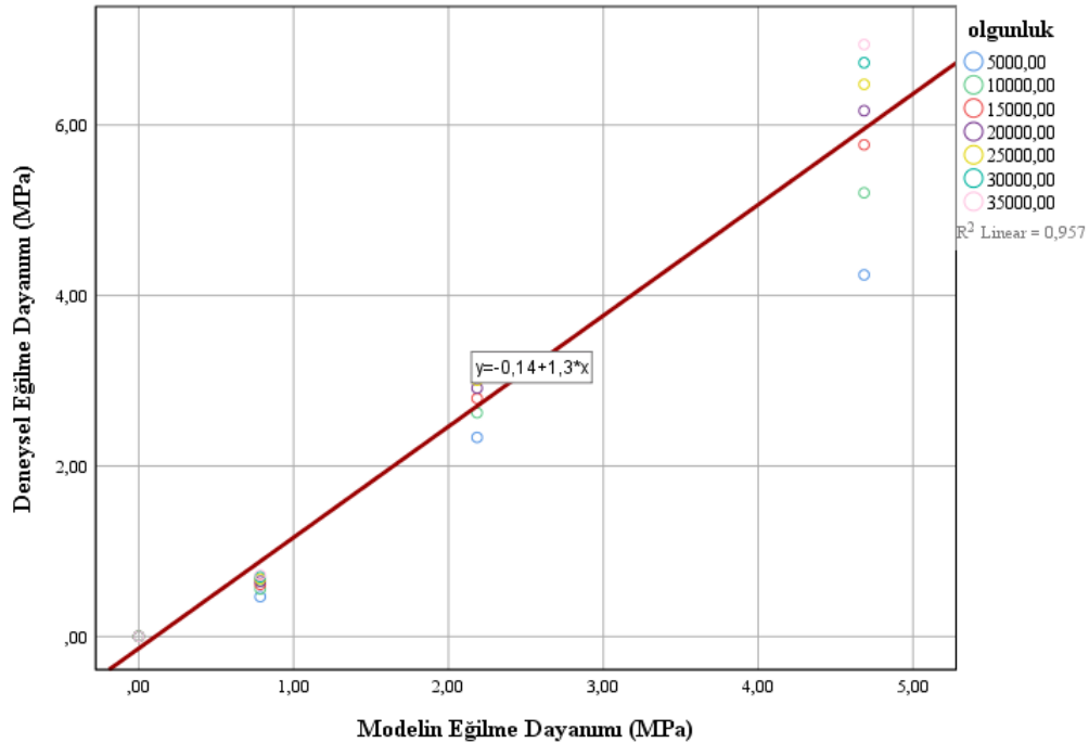
Şekil 4.20. Model-deneysel eğilme dayanımı ilişkisi.
