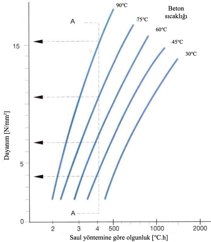
Şekil 2.65. Saul yöntemine göre farklı sıcaklıklardaki olgunluk gelişimi [120].
