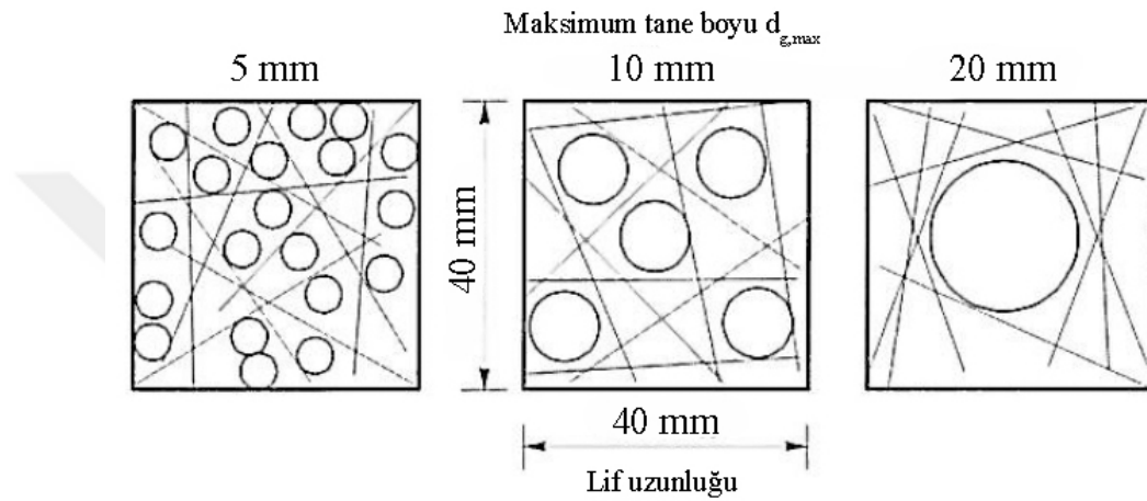
Şekil 2.2. Agreganın en büyük tane boyutunun lif dağılımına etkisi [15].
