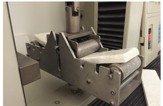
(d) Testin numune üzerinde uygulanması.
