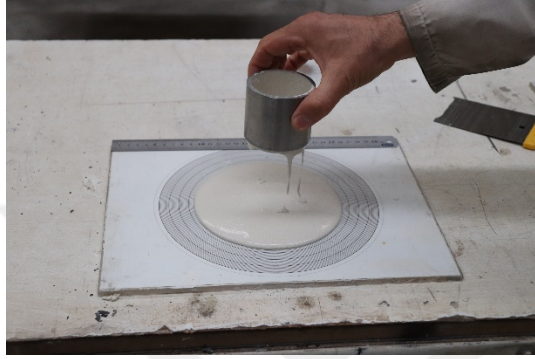
(c) Halkanın kaldırılması.
