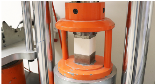
(a) Deney cihazı.
