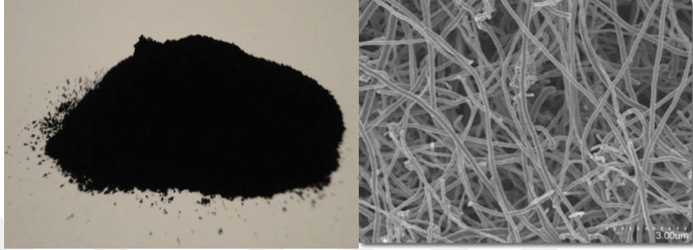
řekil 2.9. CNF'lerin toz formda ve SEM g r nt s  (3 m aralık) [31].
