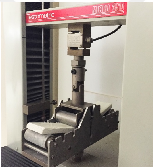
(a) Deney cihazı.
