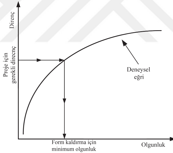
Şekil 2.67. Direnç-olgunluk ilişkisi [127].
