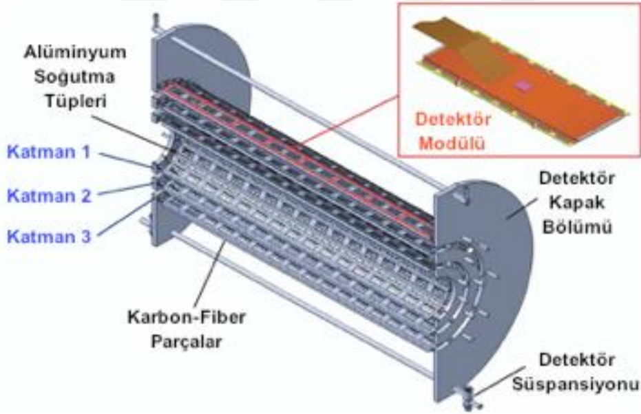
Şekil 2.5. CMS İzleyici Sisteminin İlk 3 Katmanı
