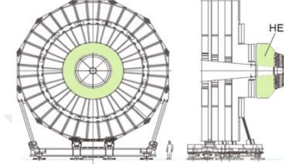
Şekil 2.7. Hadronik kapak kalorimetresi (HE)
